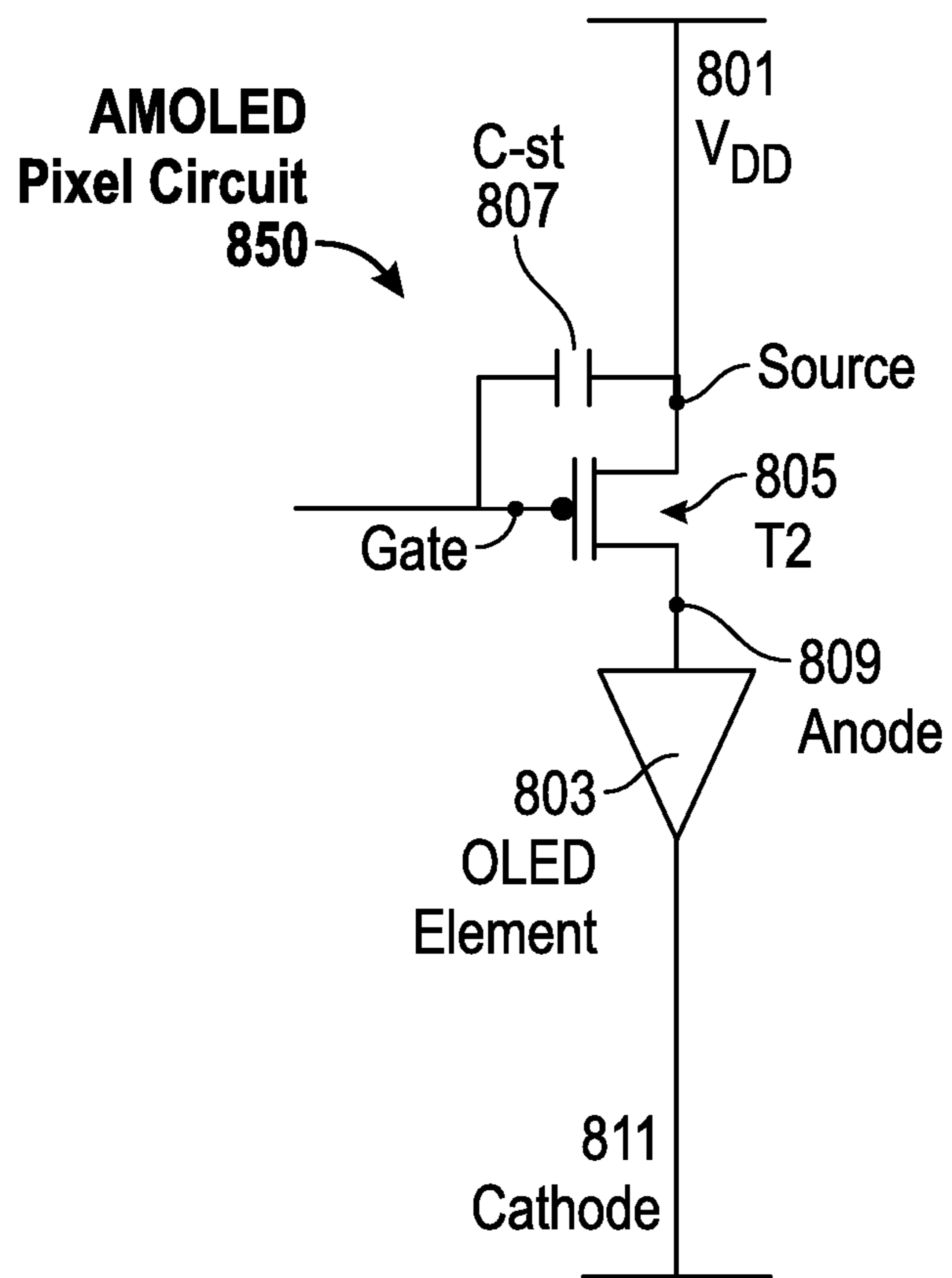
FIG. 8B
