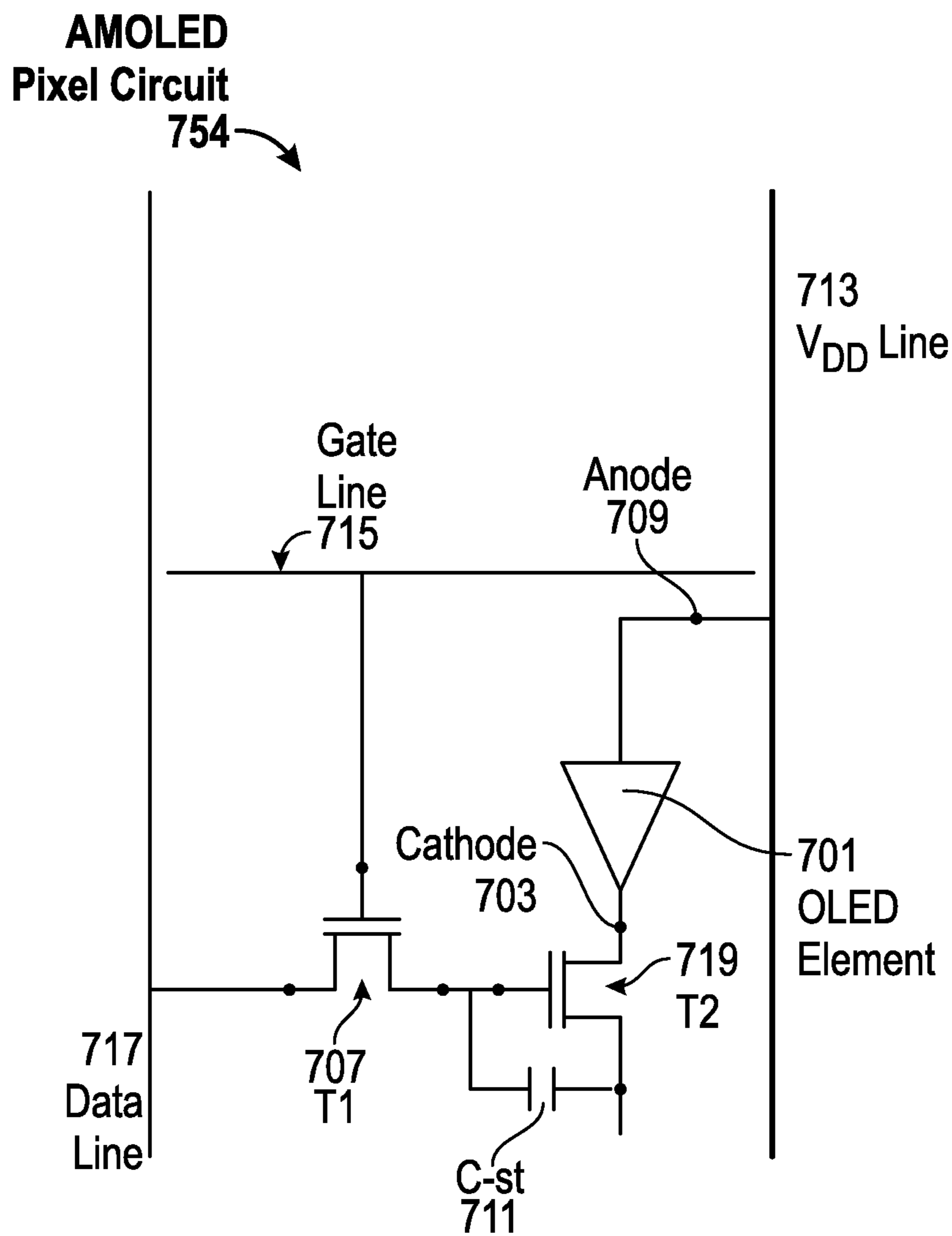
FIG. 7C
