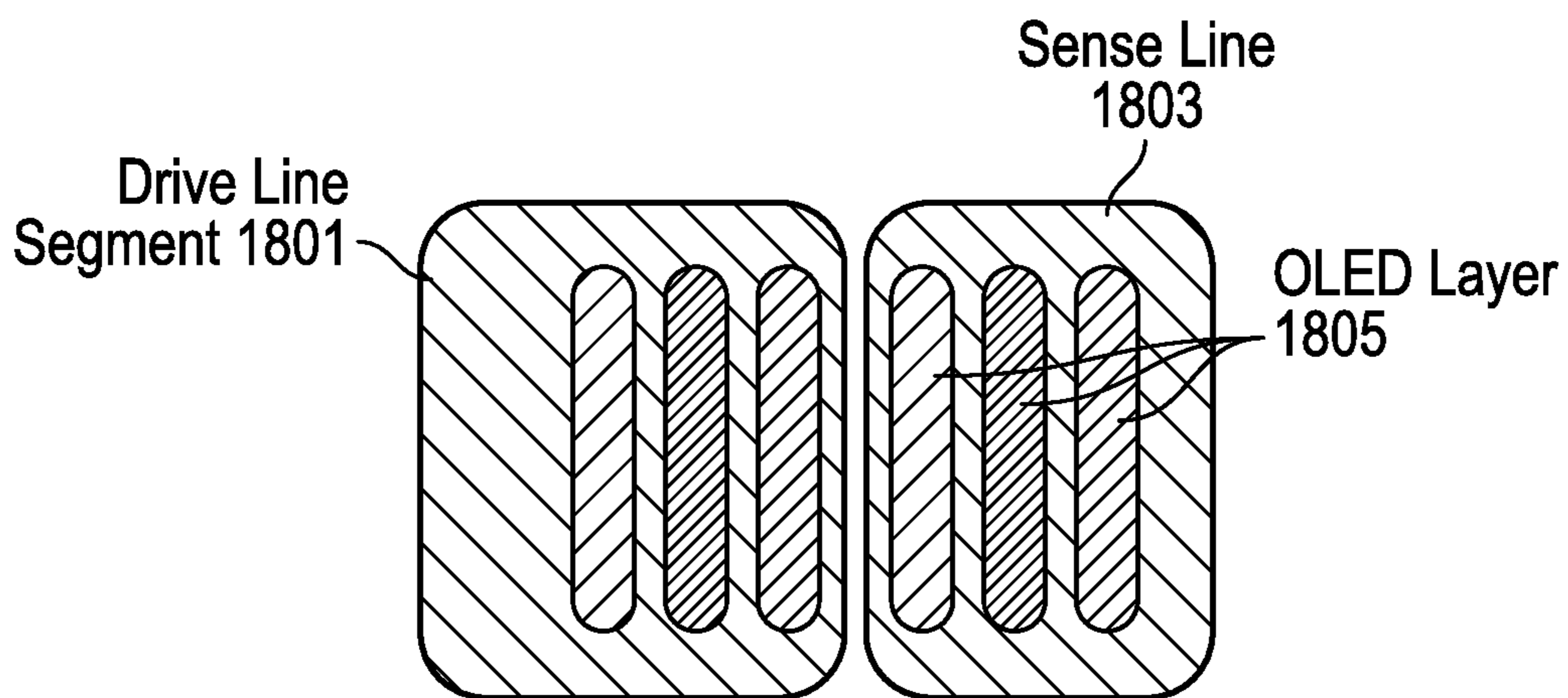
FIG. 18A
