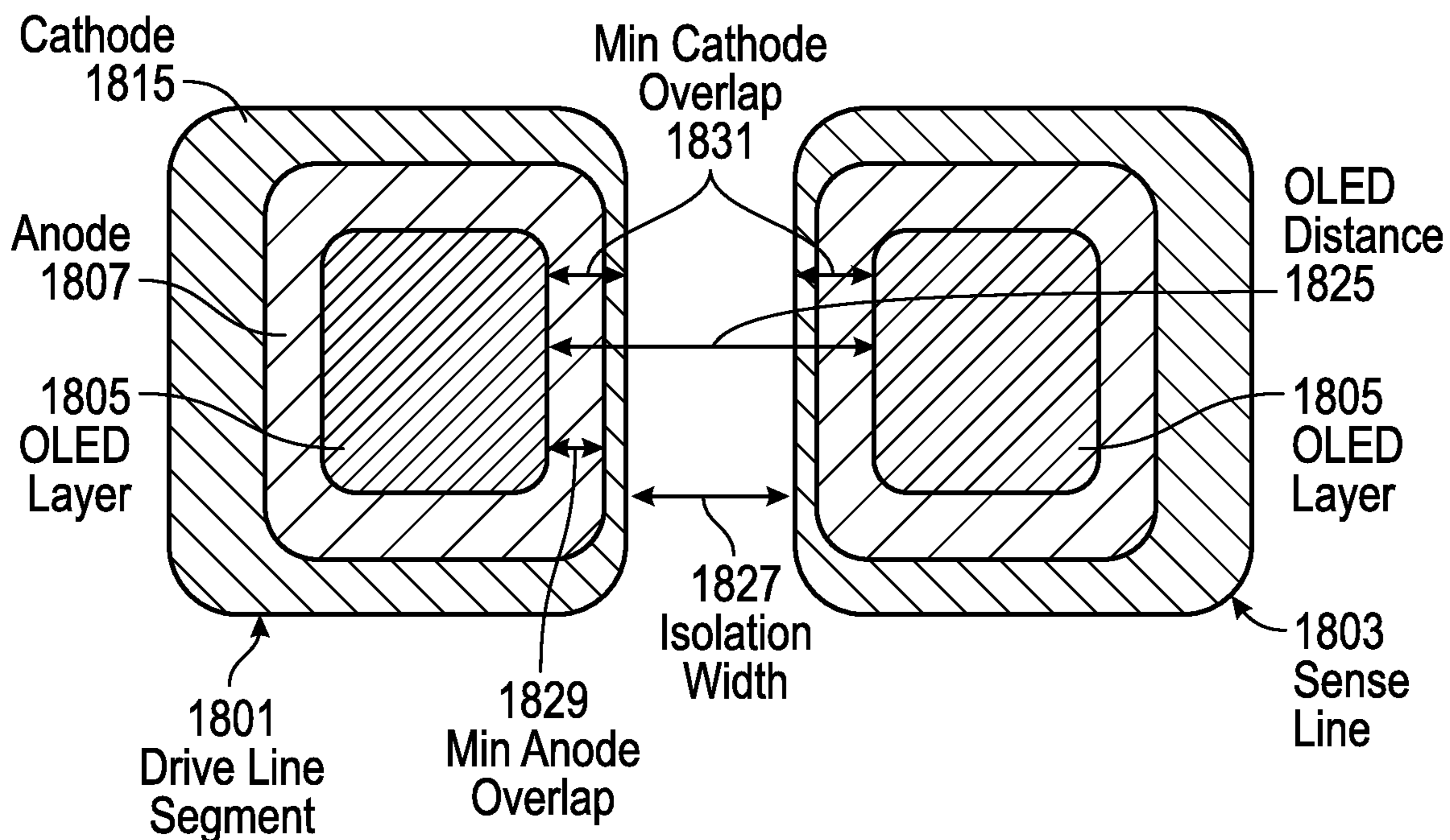
FIG. 18B
