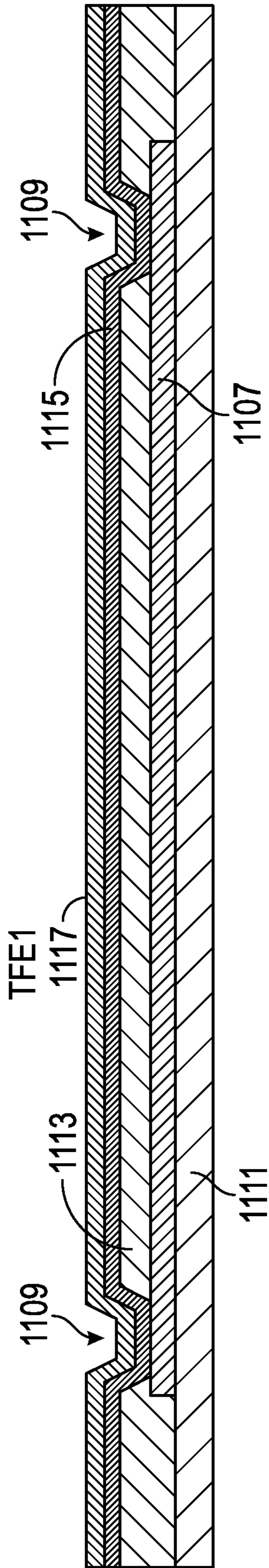
FIG. 11B-2
