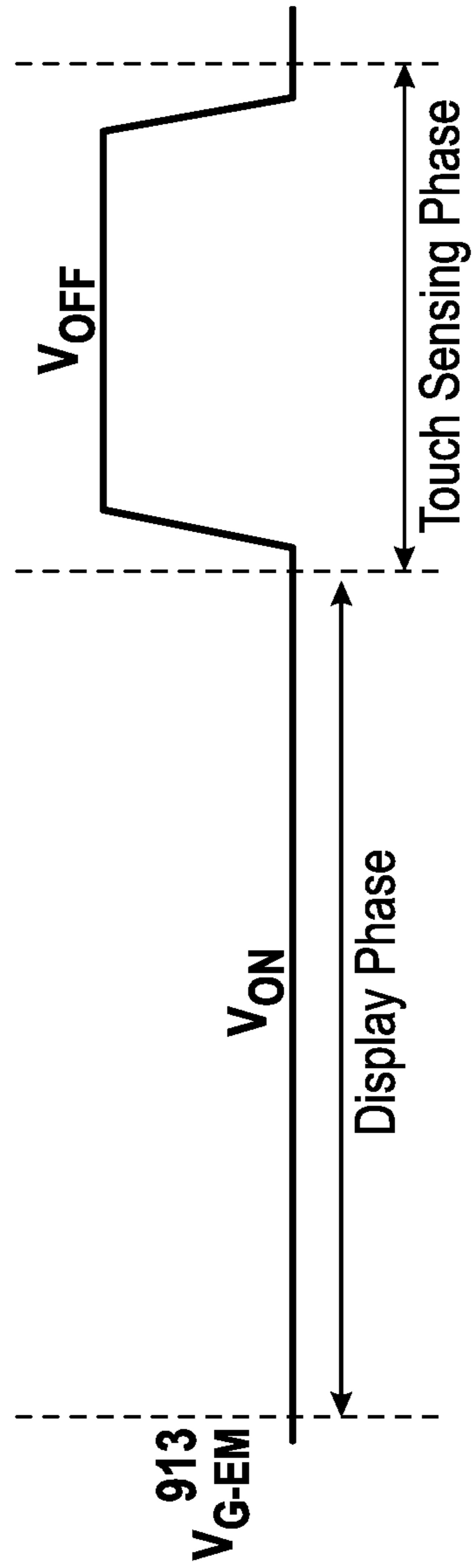
FIG. 9A
