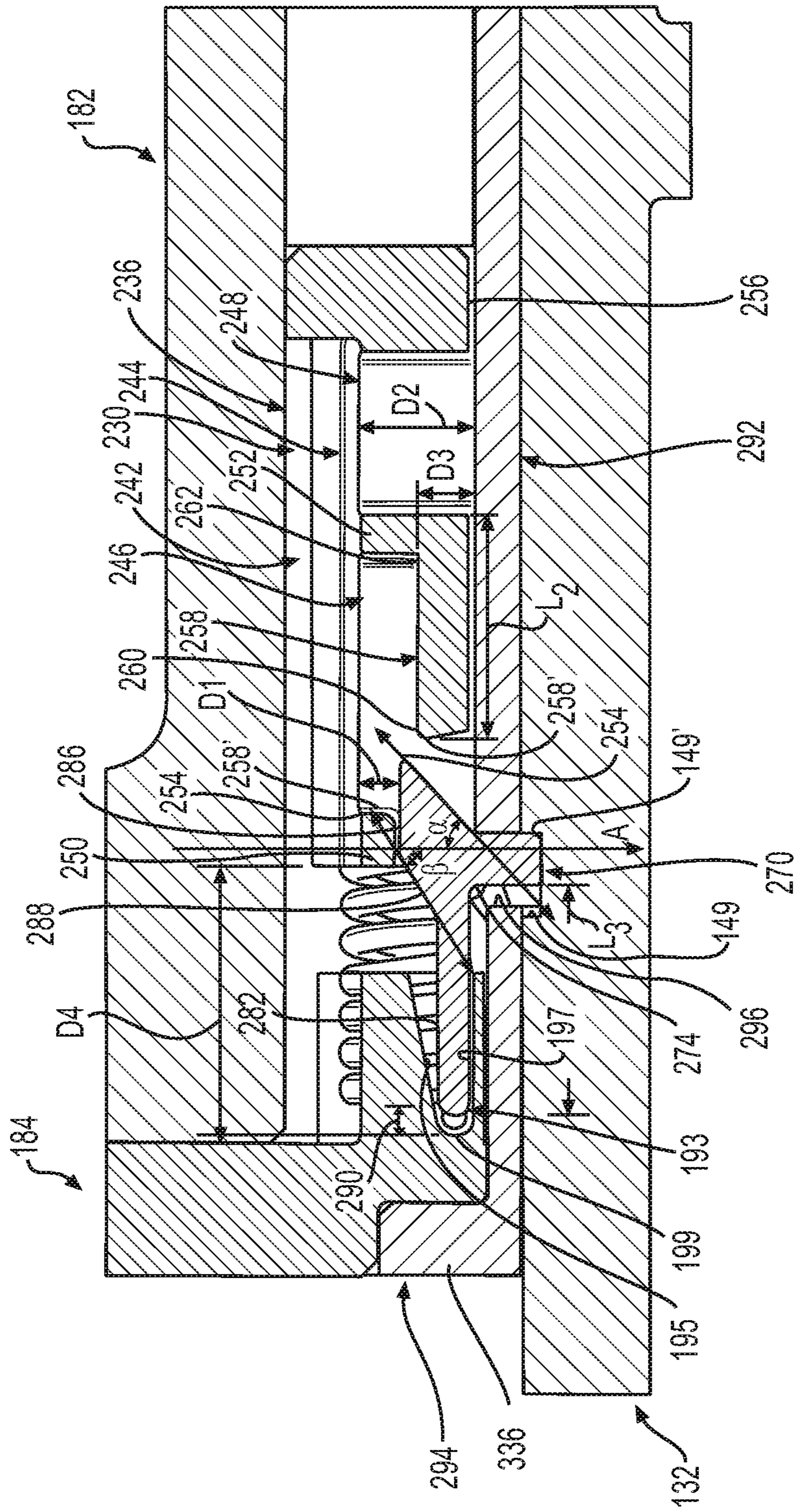
FIG. 7
