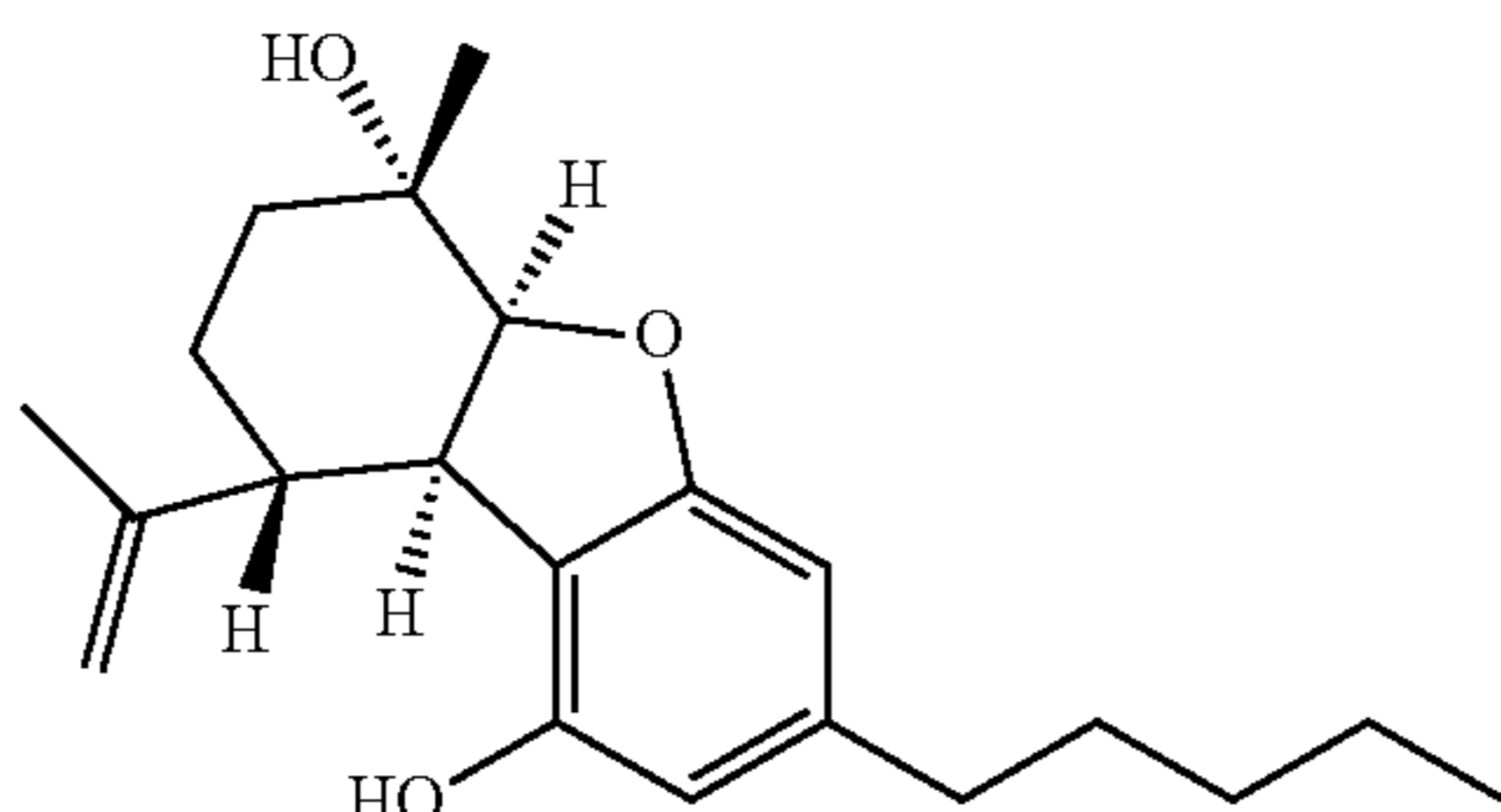
(5aS, 6S, 9R, 9aR)-cannabielsoin [CBE]
