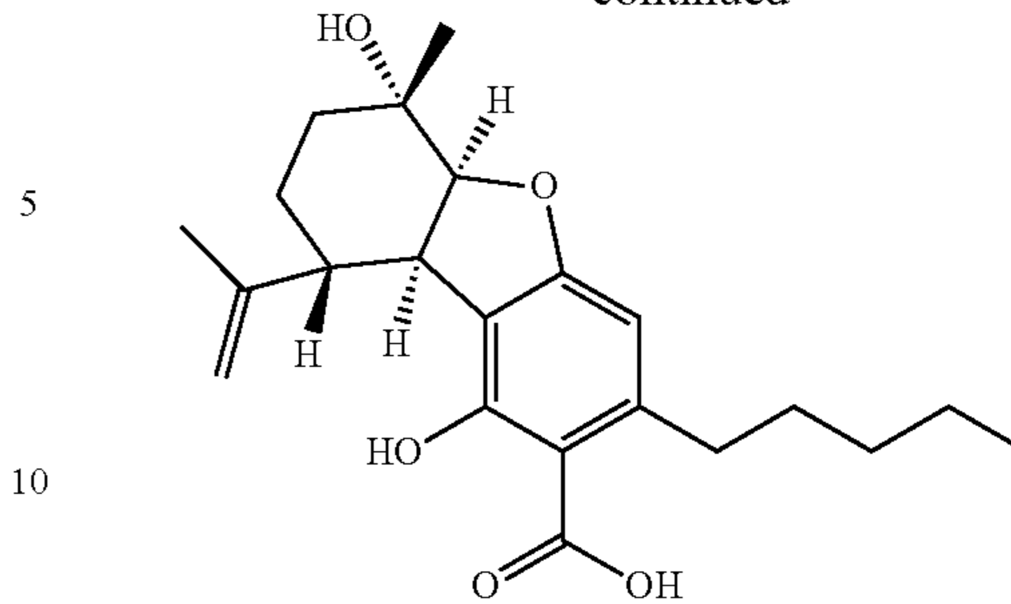
(5aS, 6S, 9R, 9aR)-cannabielsoic acid B [CBEA B]
