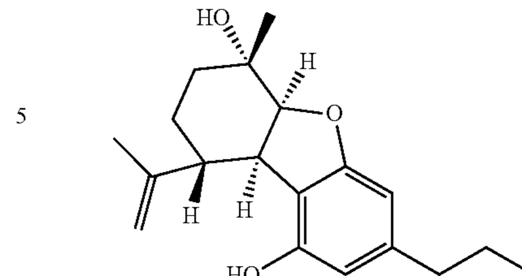
(5aS, 6S, 9R, 9aR)-C 3 -cannabielsoin [CBE-C 3 ]
