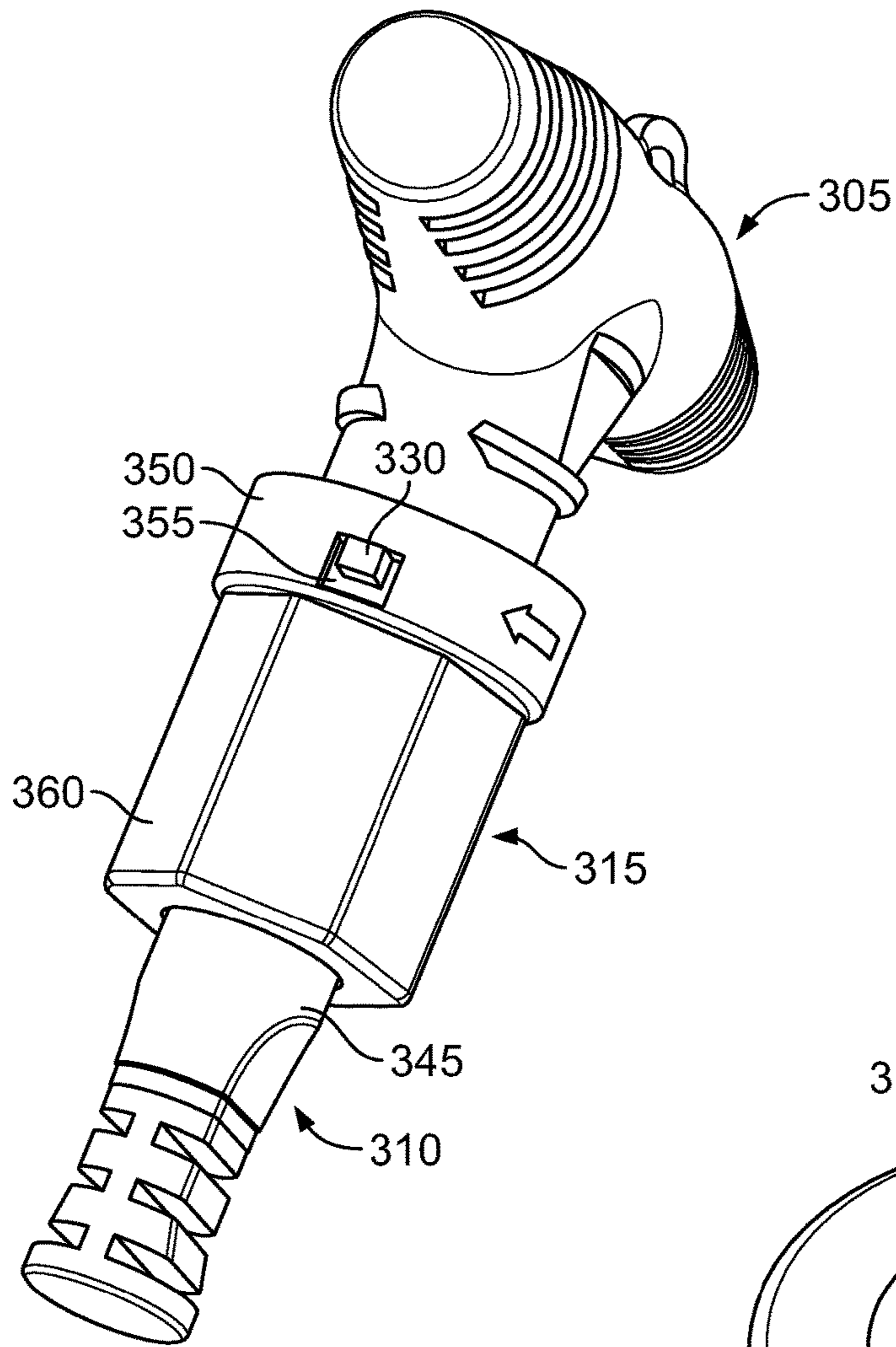
FIG. 5
