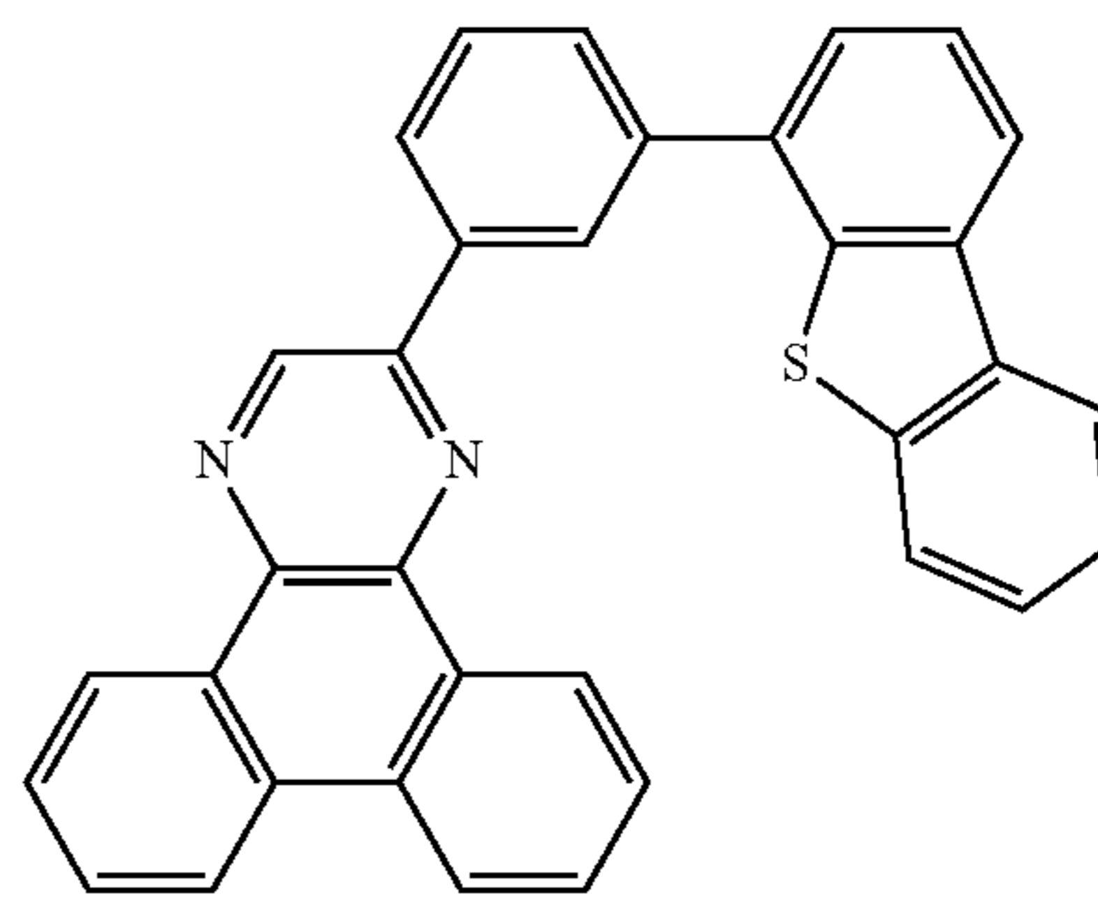
2mDBTPDBq-II
