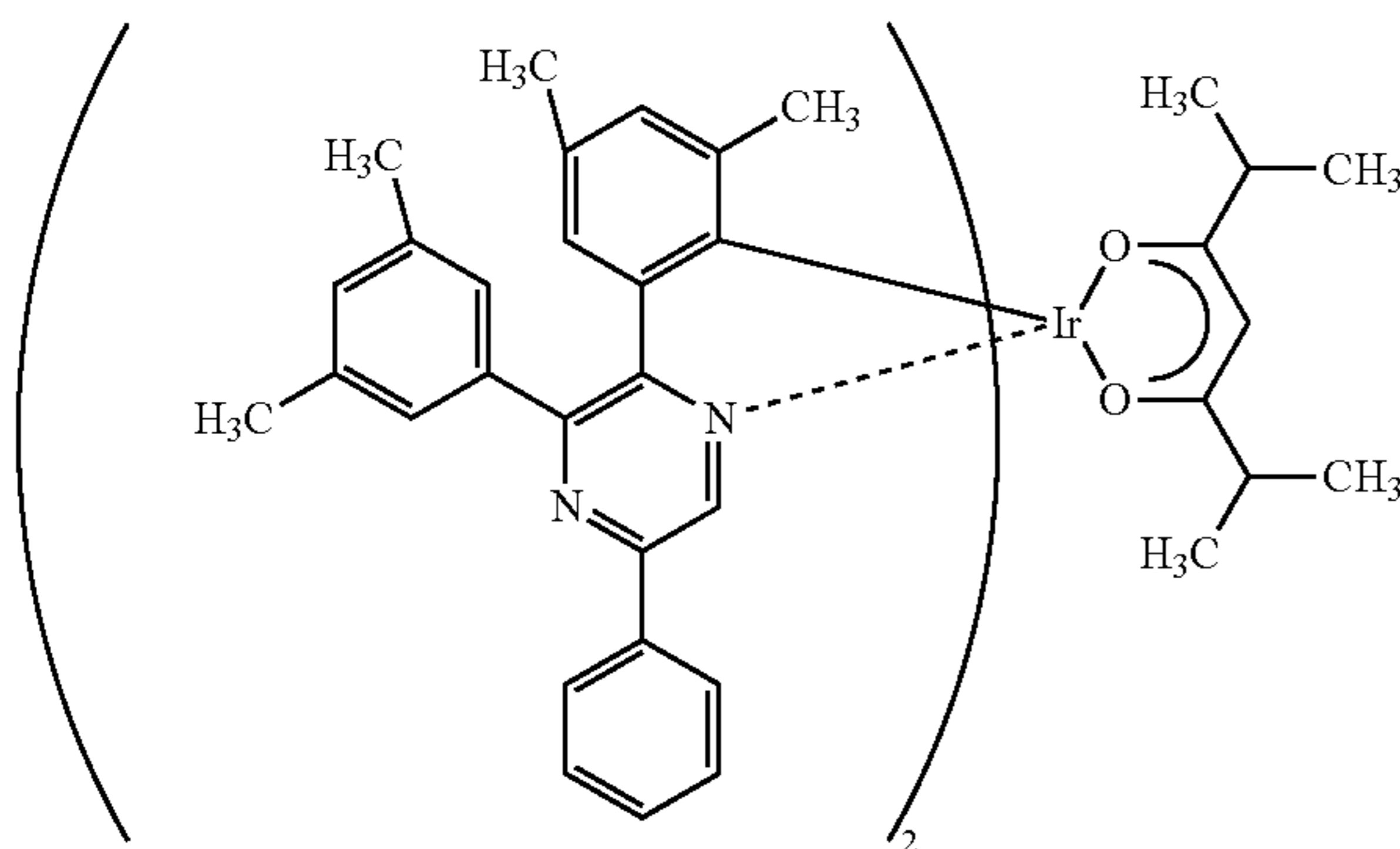
Ir(dmdppr-P) 2 (dibm)
