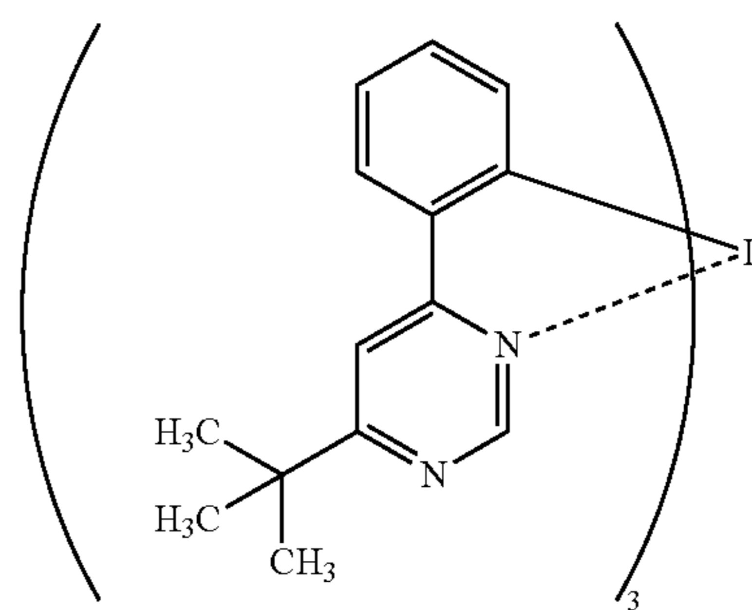
Ir(tBuppm) 3
