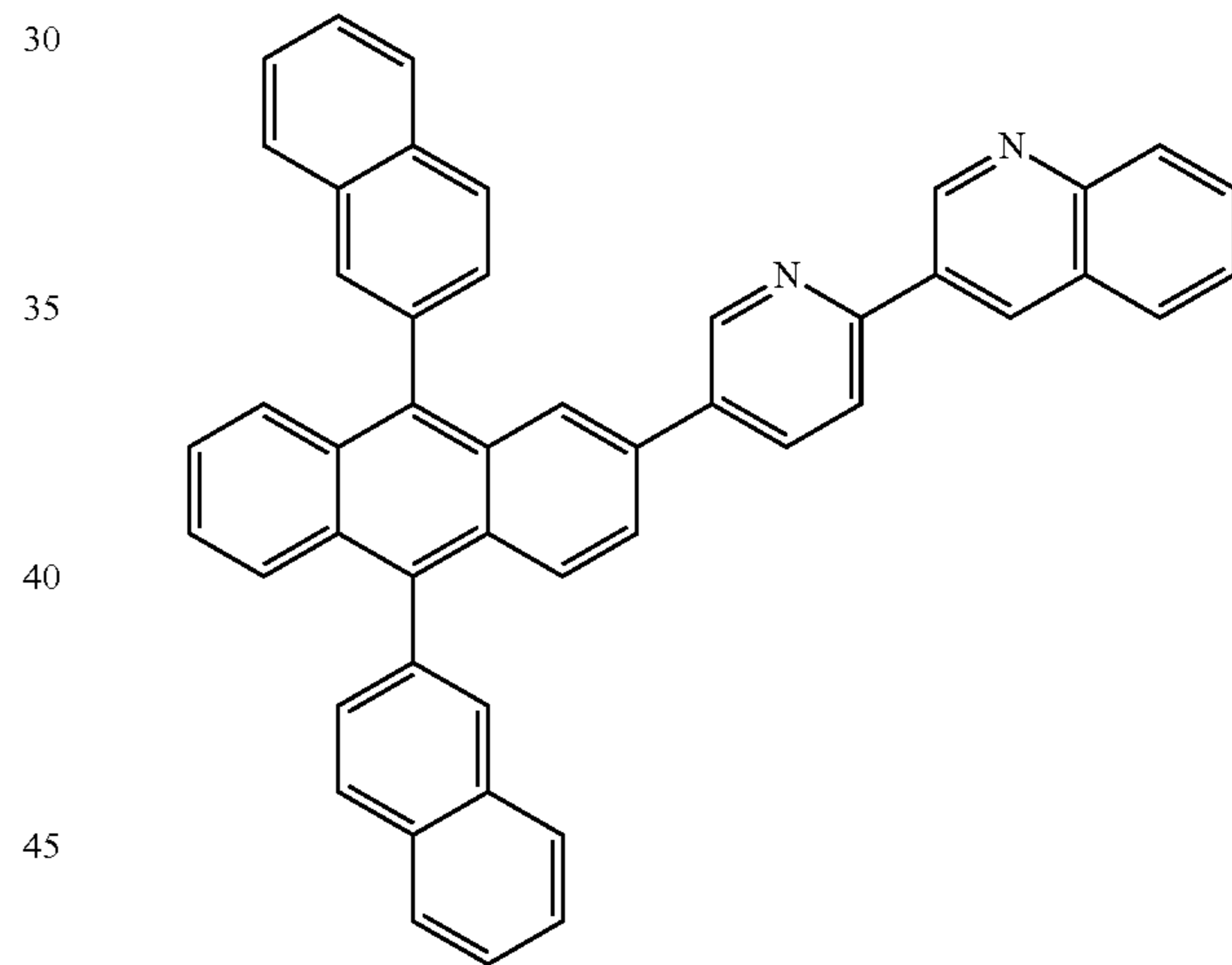
ET2
