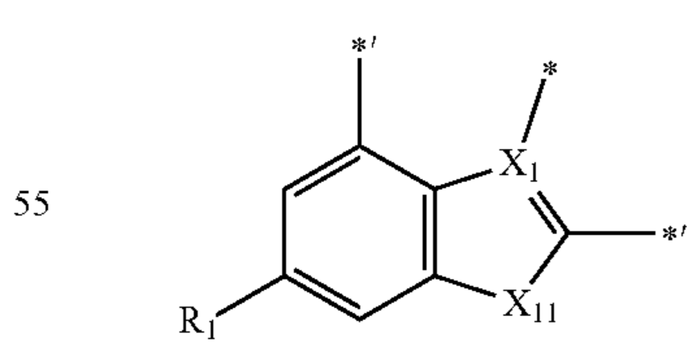
Formula A4-1(35)
