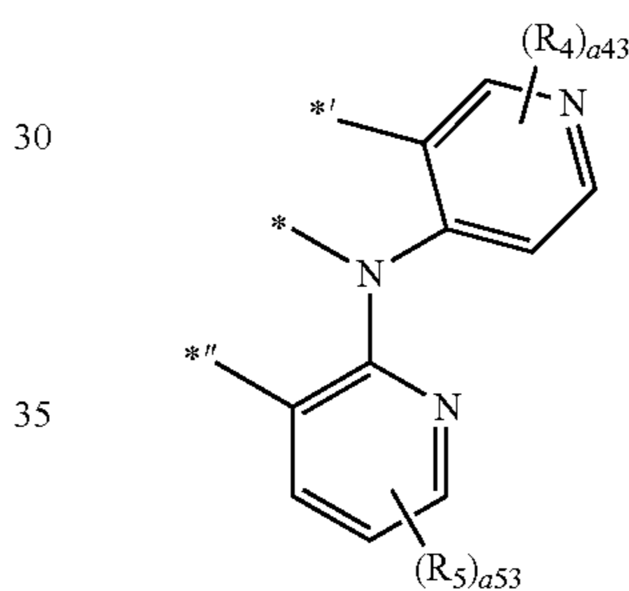
Formula A4-1(3)
