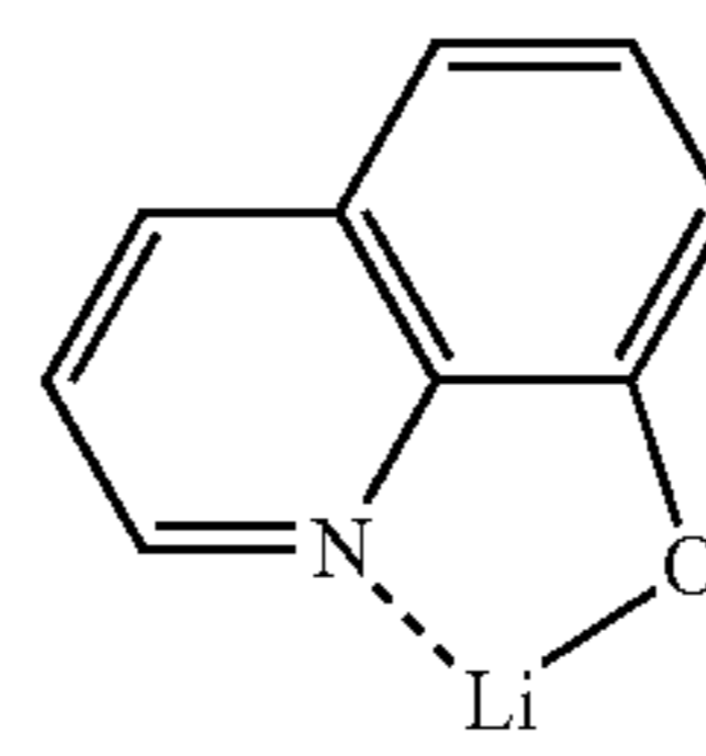
ET-D1
