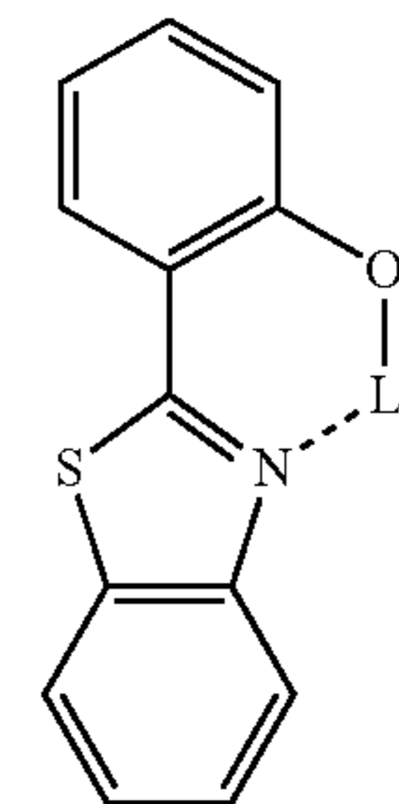
ET-D2
