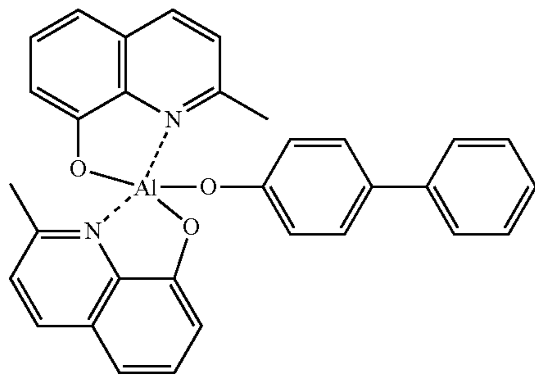
BAlq
