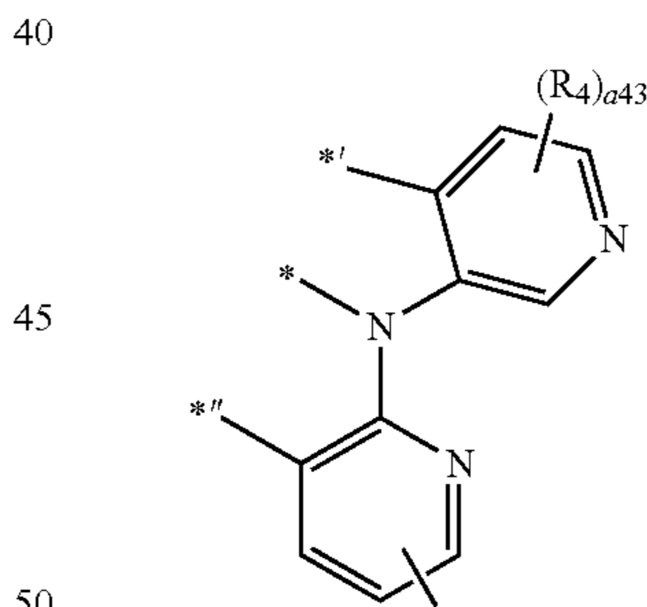
Formula A4-1(4)
