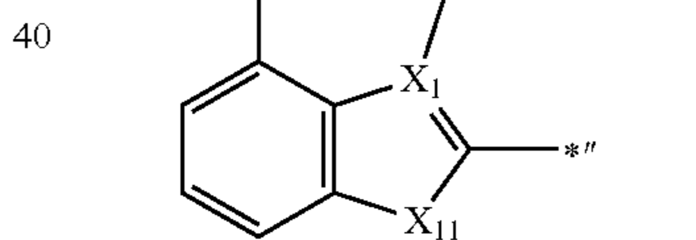
Formula A4-1(34)
