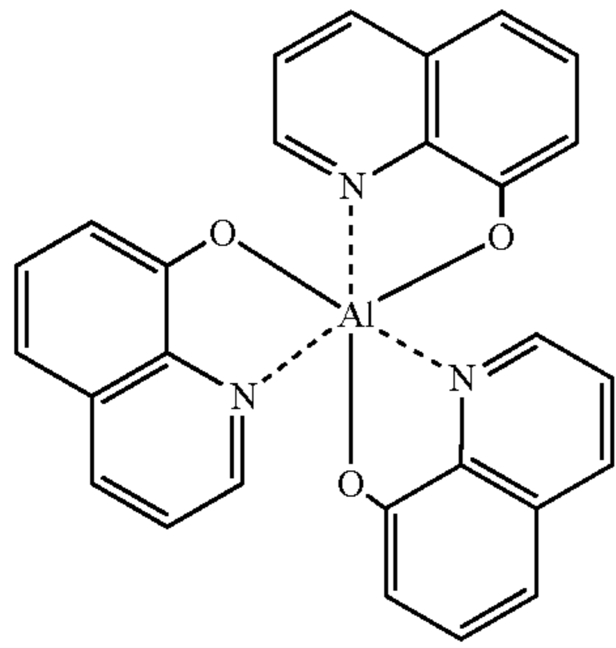
Alq 3
