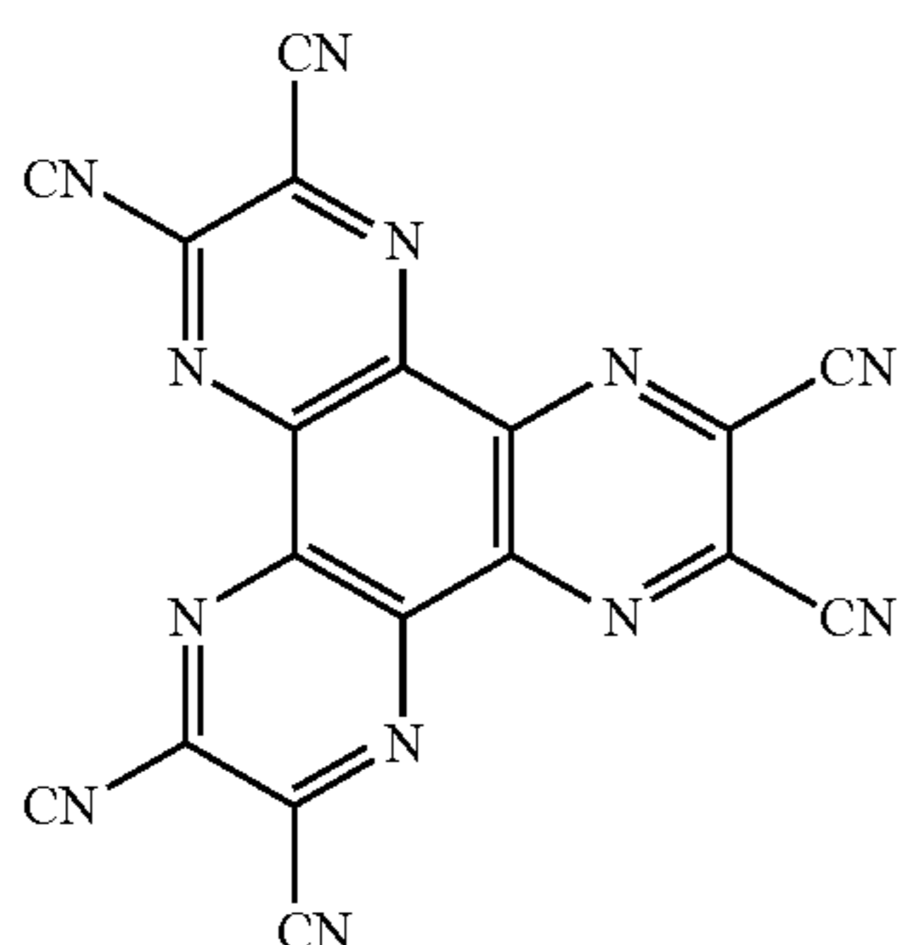
HT-D1
