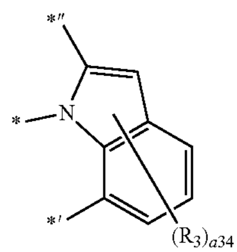
Formula A3-1(18)
