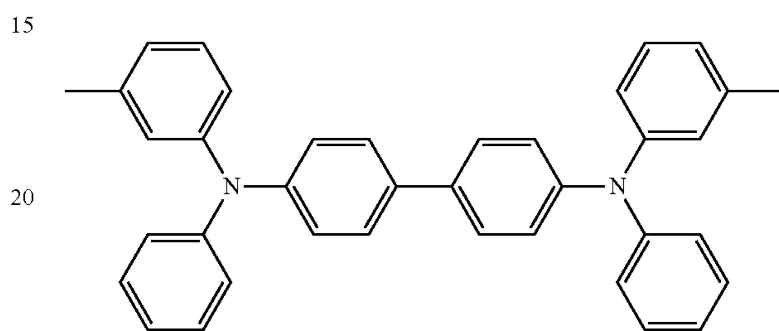
TPD
