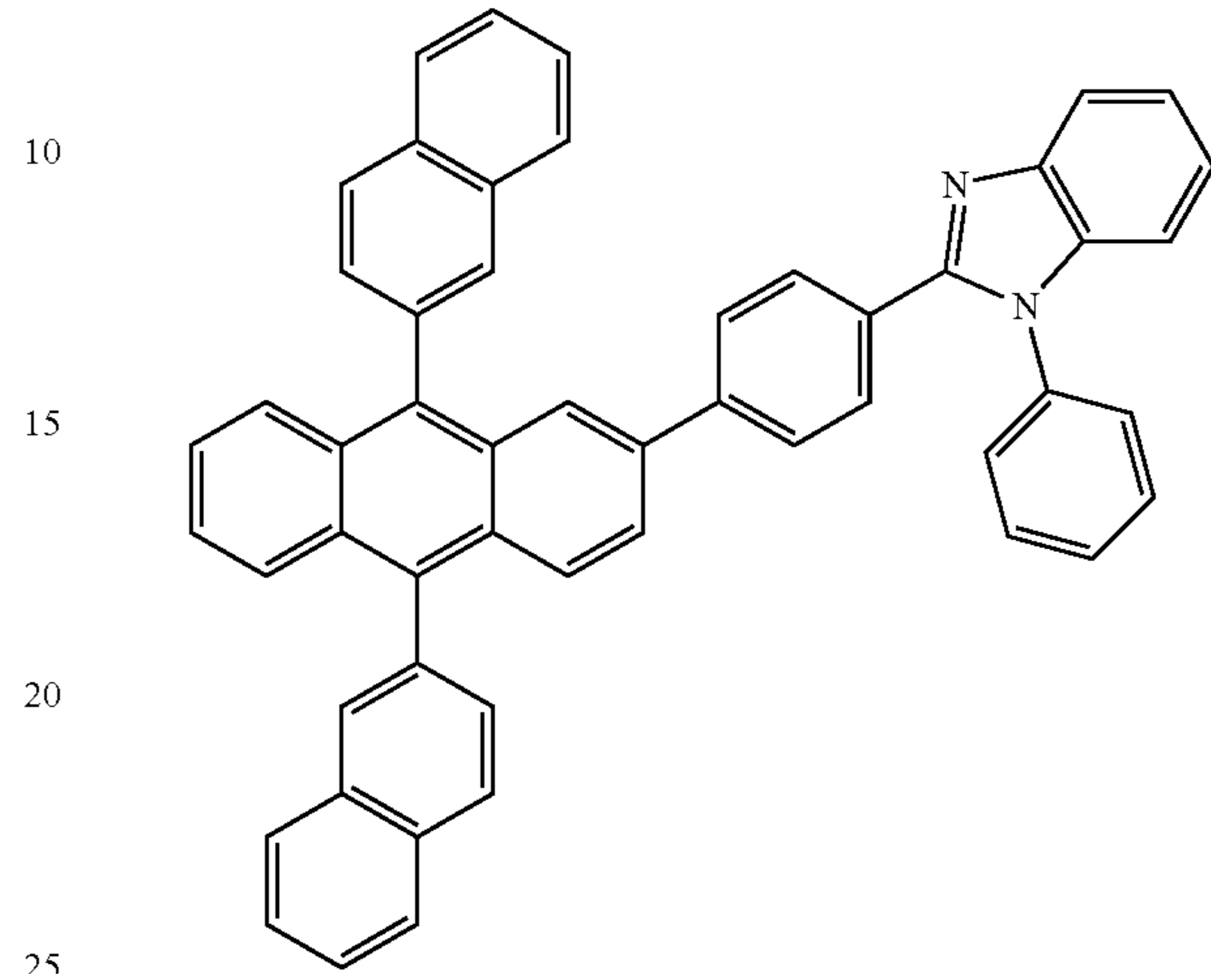
ET1
