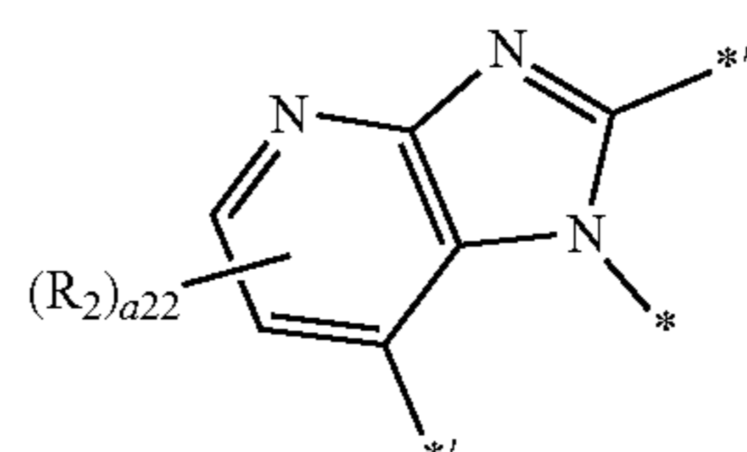
Formula A2-2(57)
