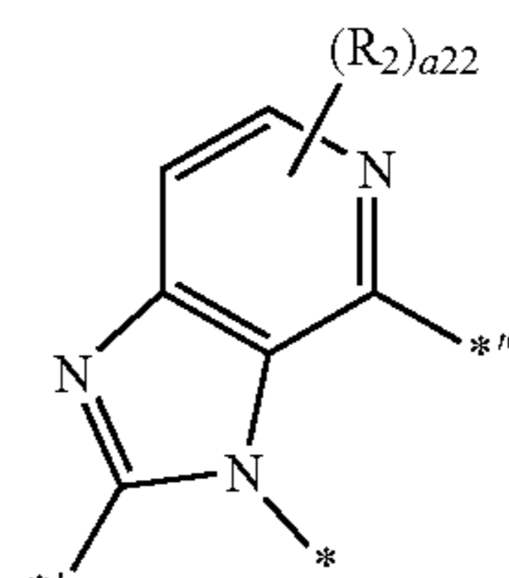
Formula A2-2(1)
