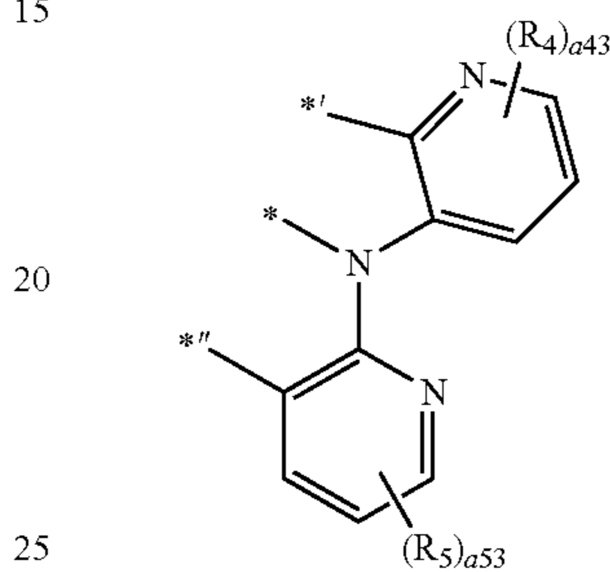
Formula A4-1(2)
