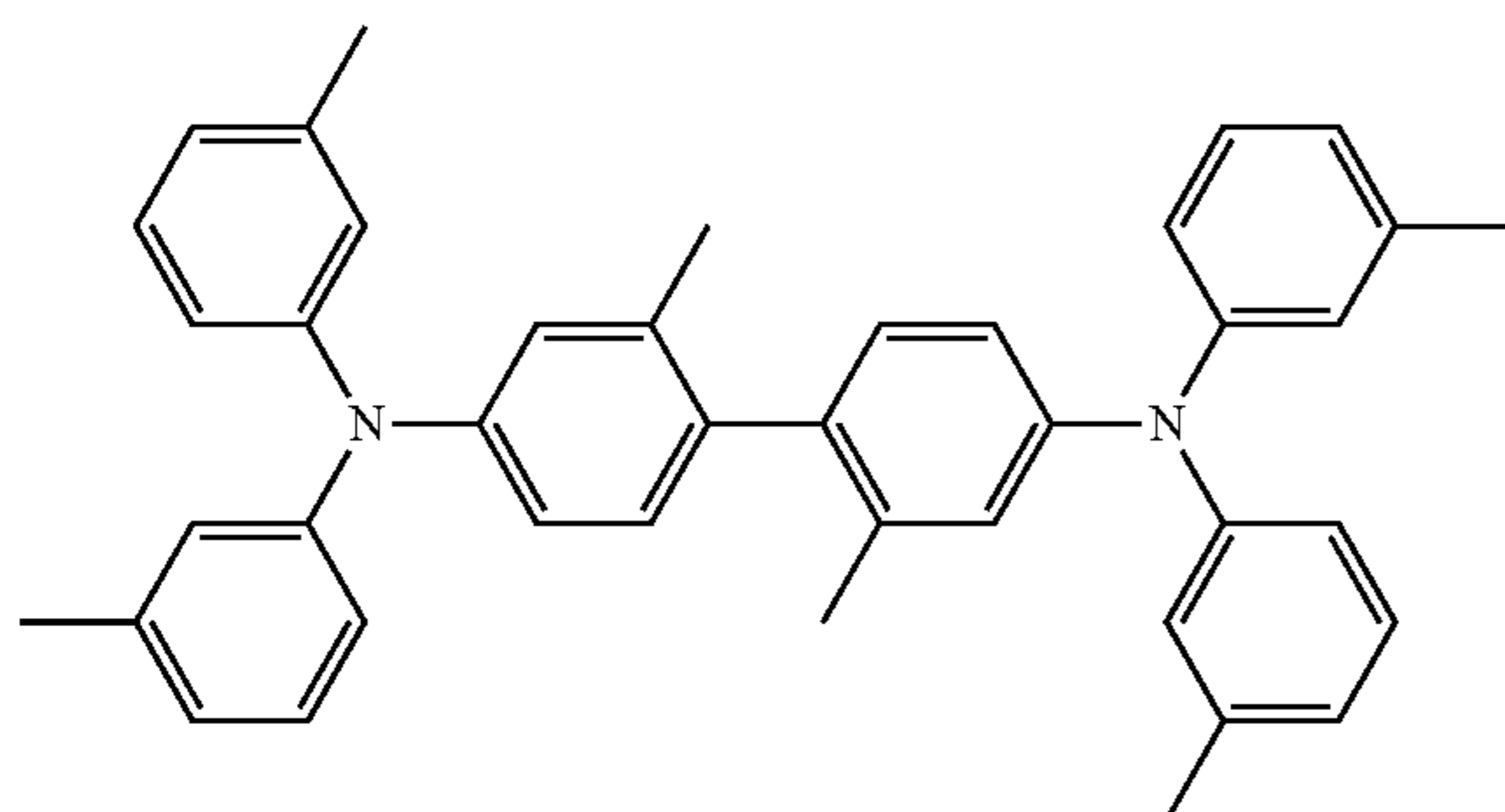
HMTPD
