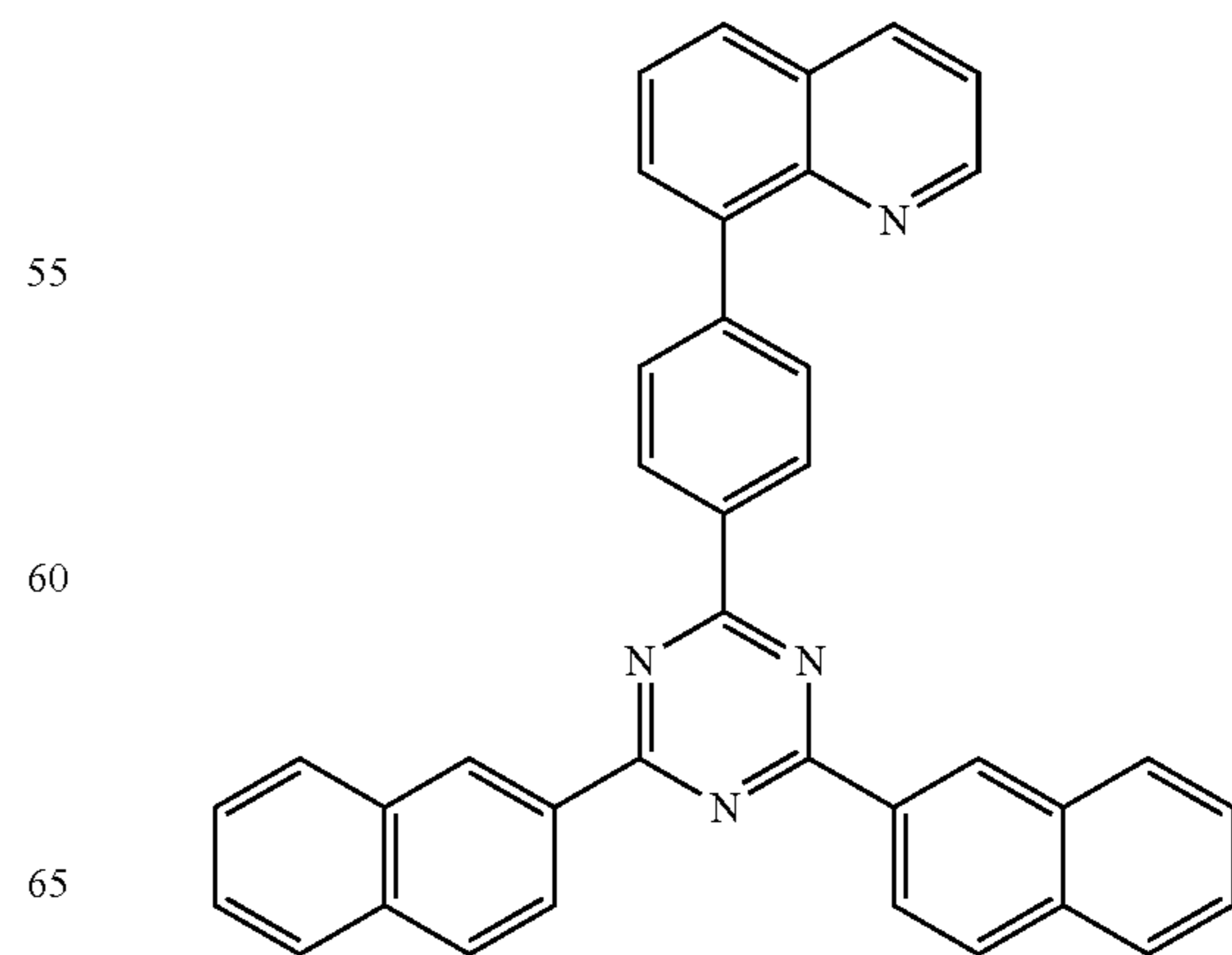
ET3
