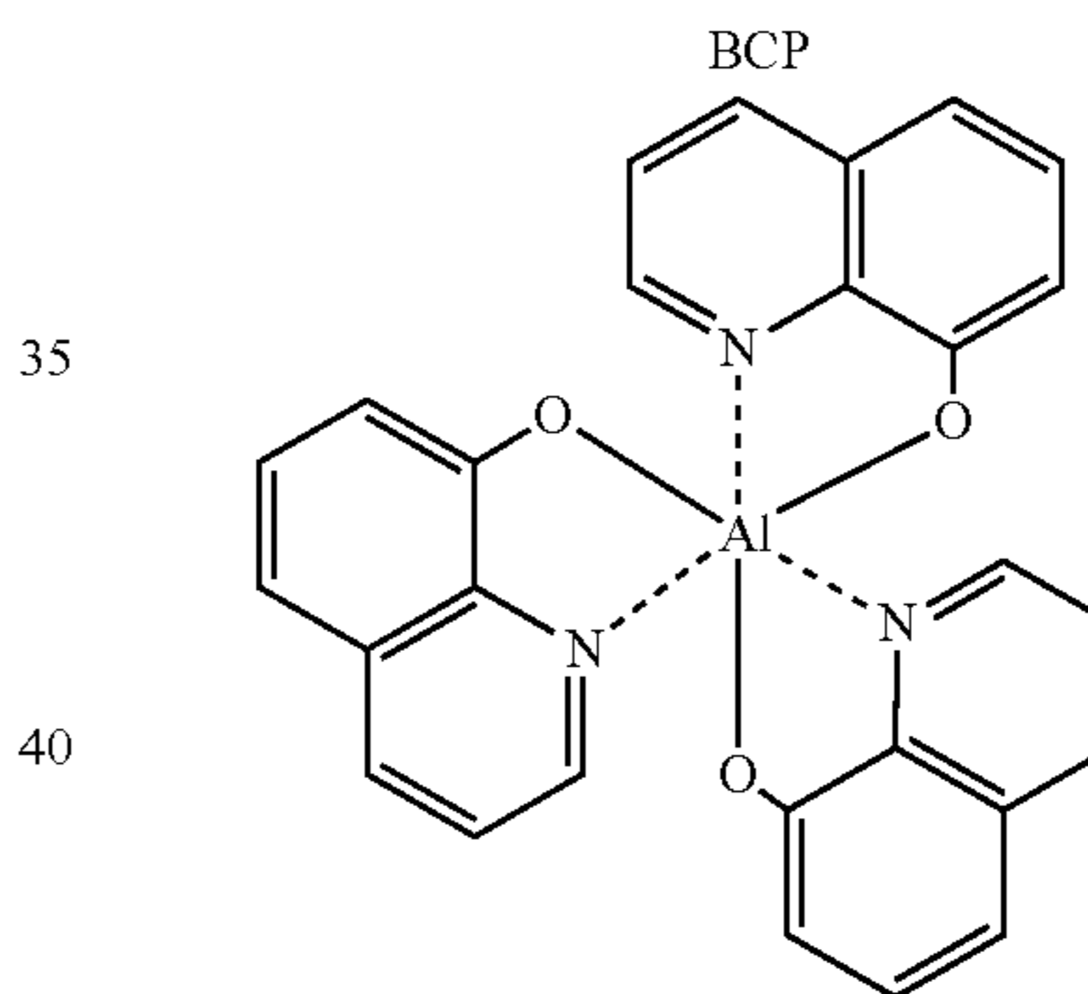
Alq 3
