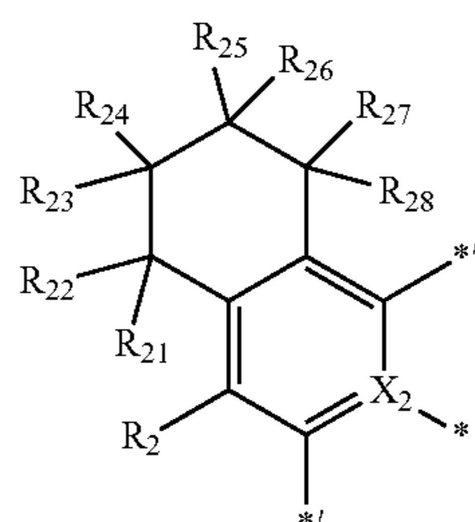
Formula A2-1(1)
