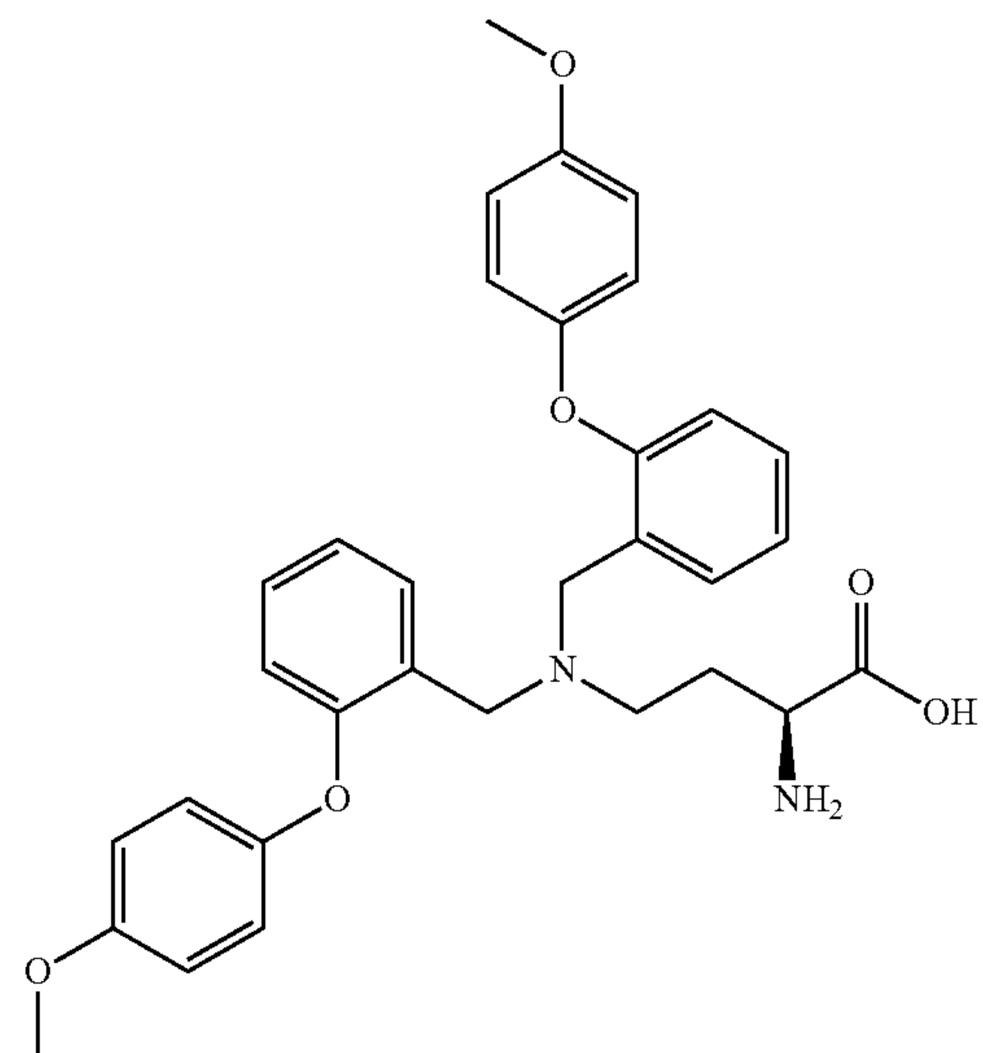
MLS-A-148-14 rat IC 50 = 8.7 μM human IC 50 = 11.9 μM
