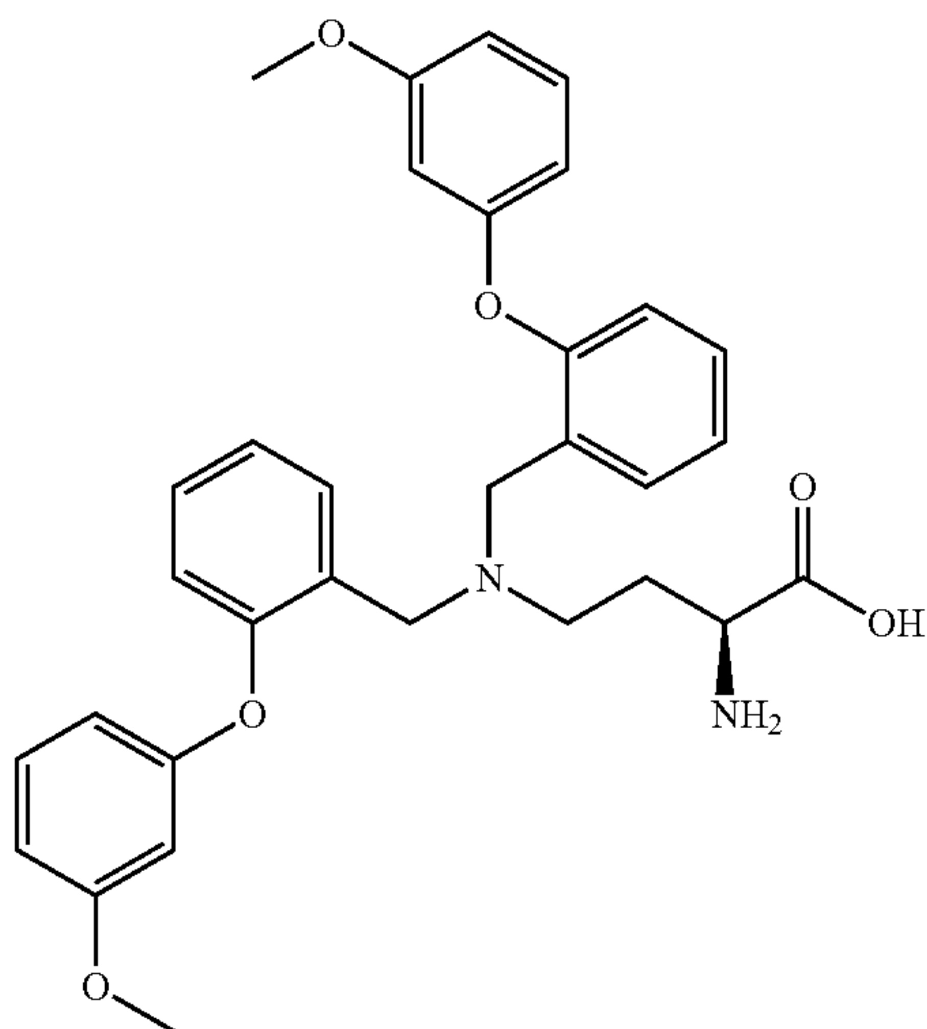
MLS-A-148-13 rat IC 50 = 1.3 μM human IC 50 = 57.2 μM
