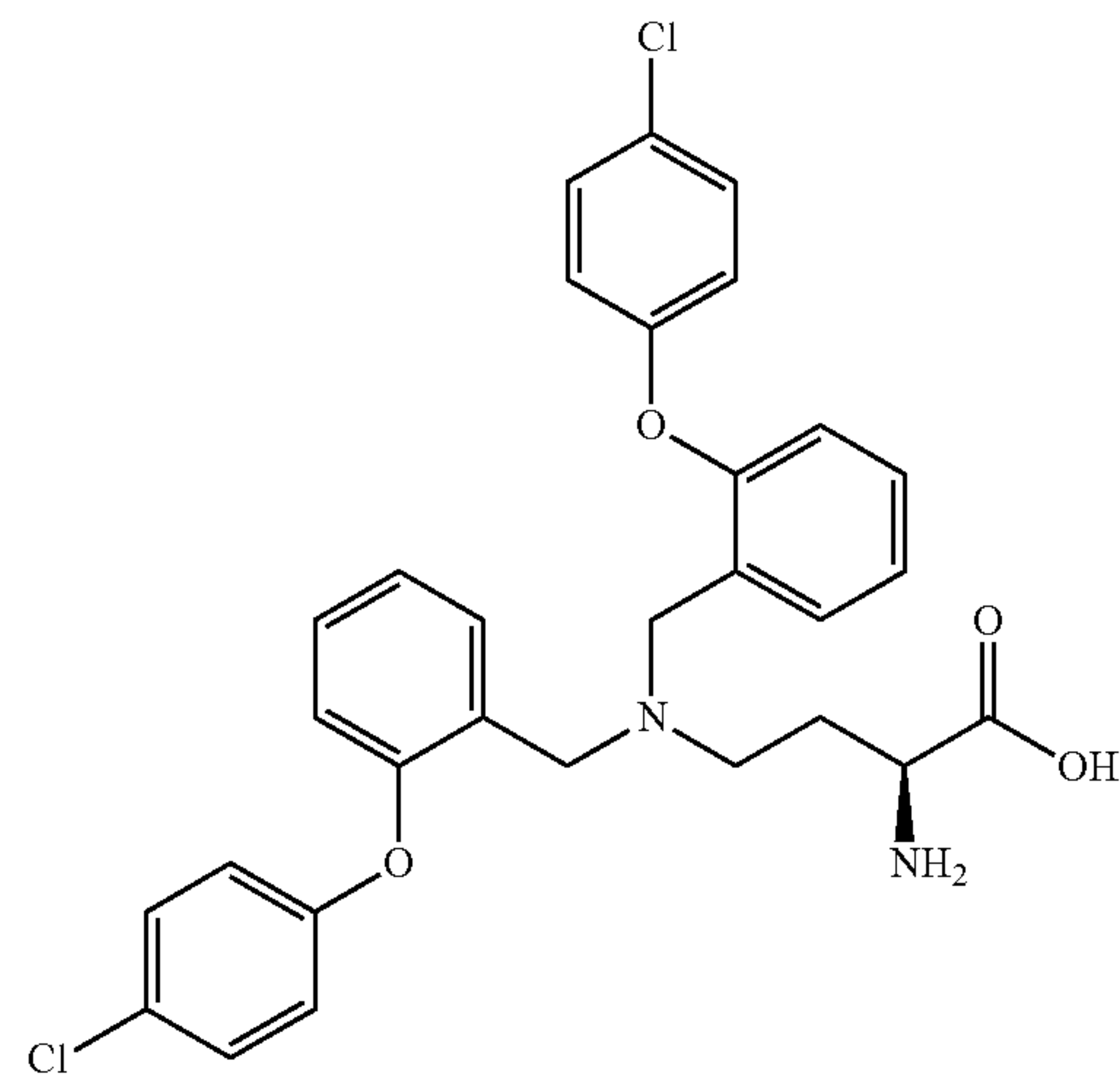
MLS-A-148-15 rat IC 50 = 24.3 μM human IC 50 = 26.0 μM
