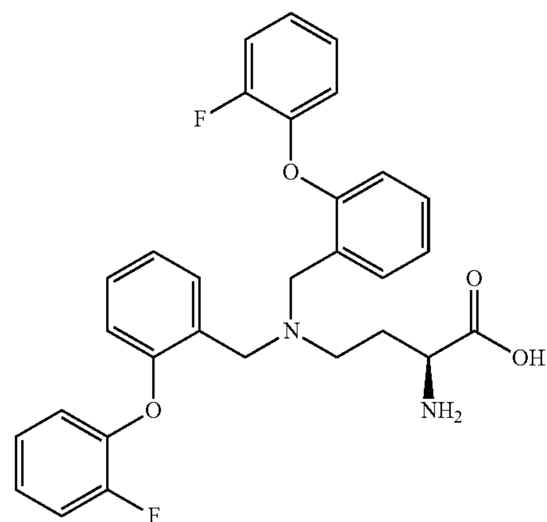
MLS-A-148-16 rat IC 50 = 1.8 μM human IC 50 = 33.8 μM
