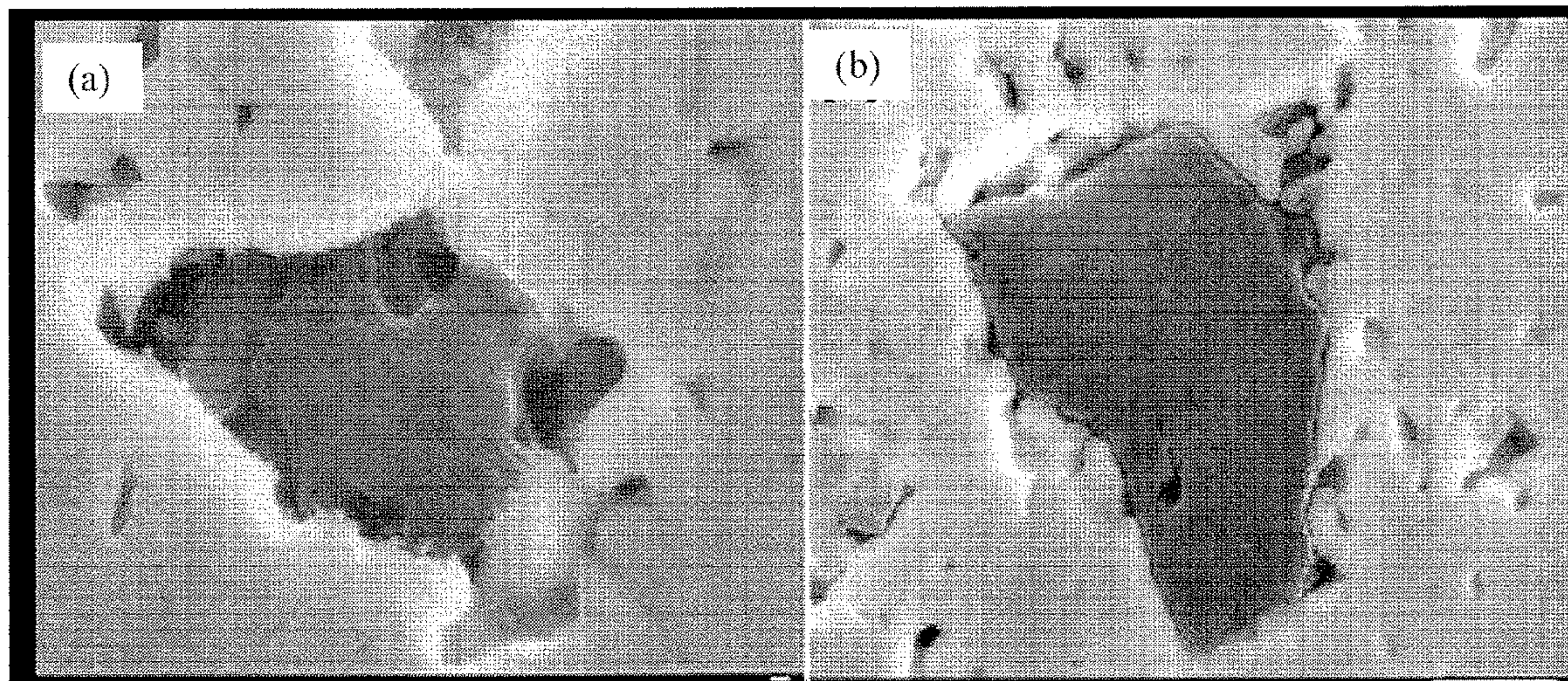
MAIC SEI 15.0kV X30,000 WD15.0mm 100nm
