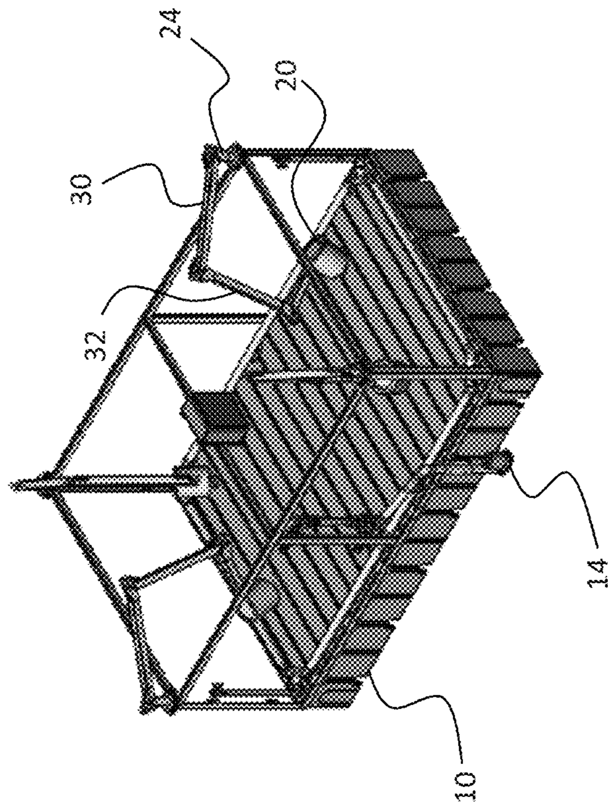
Fig. 4A
