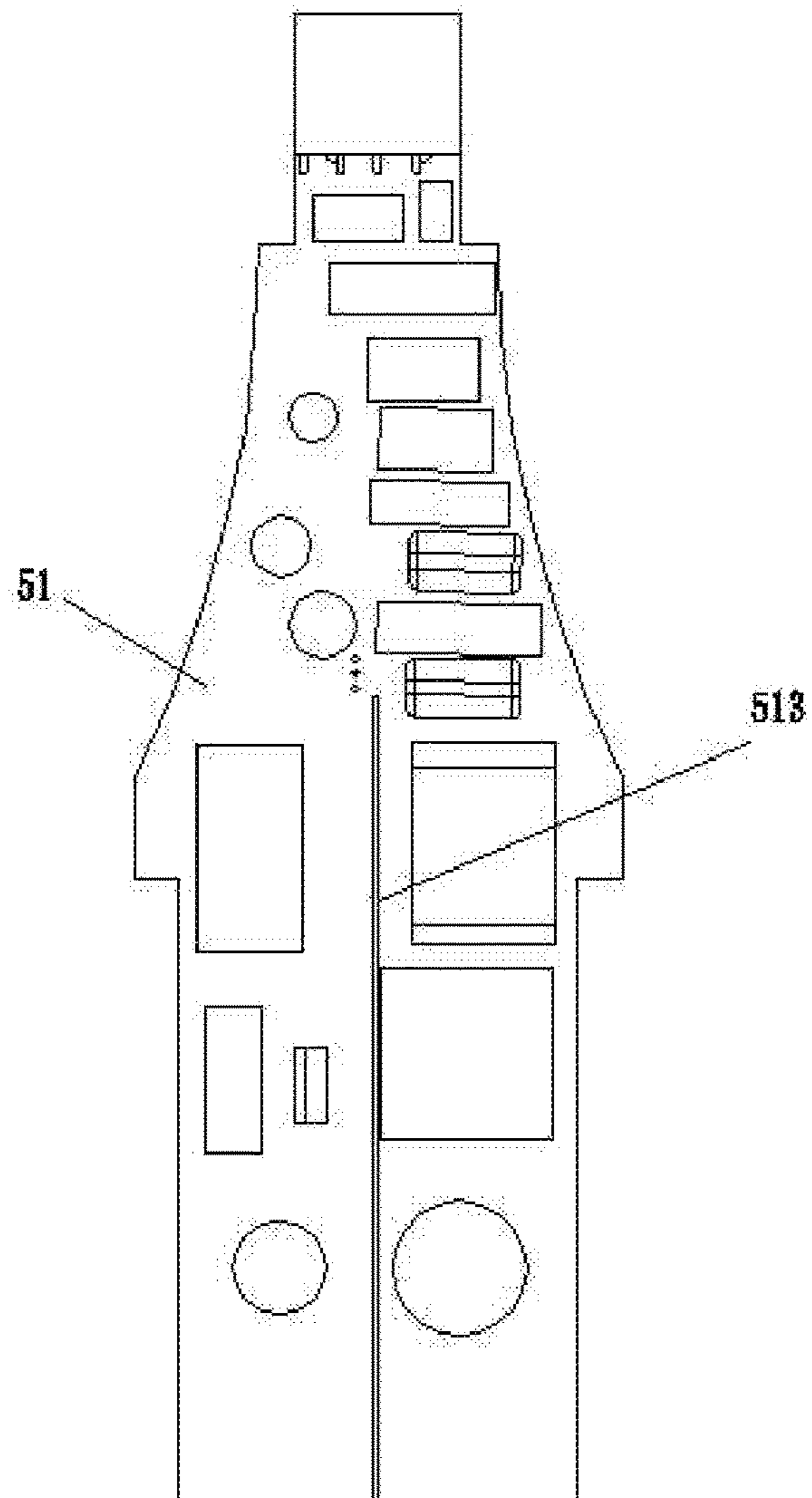
FIG. 33
