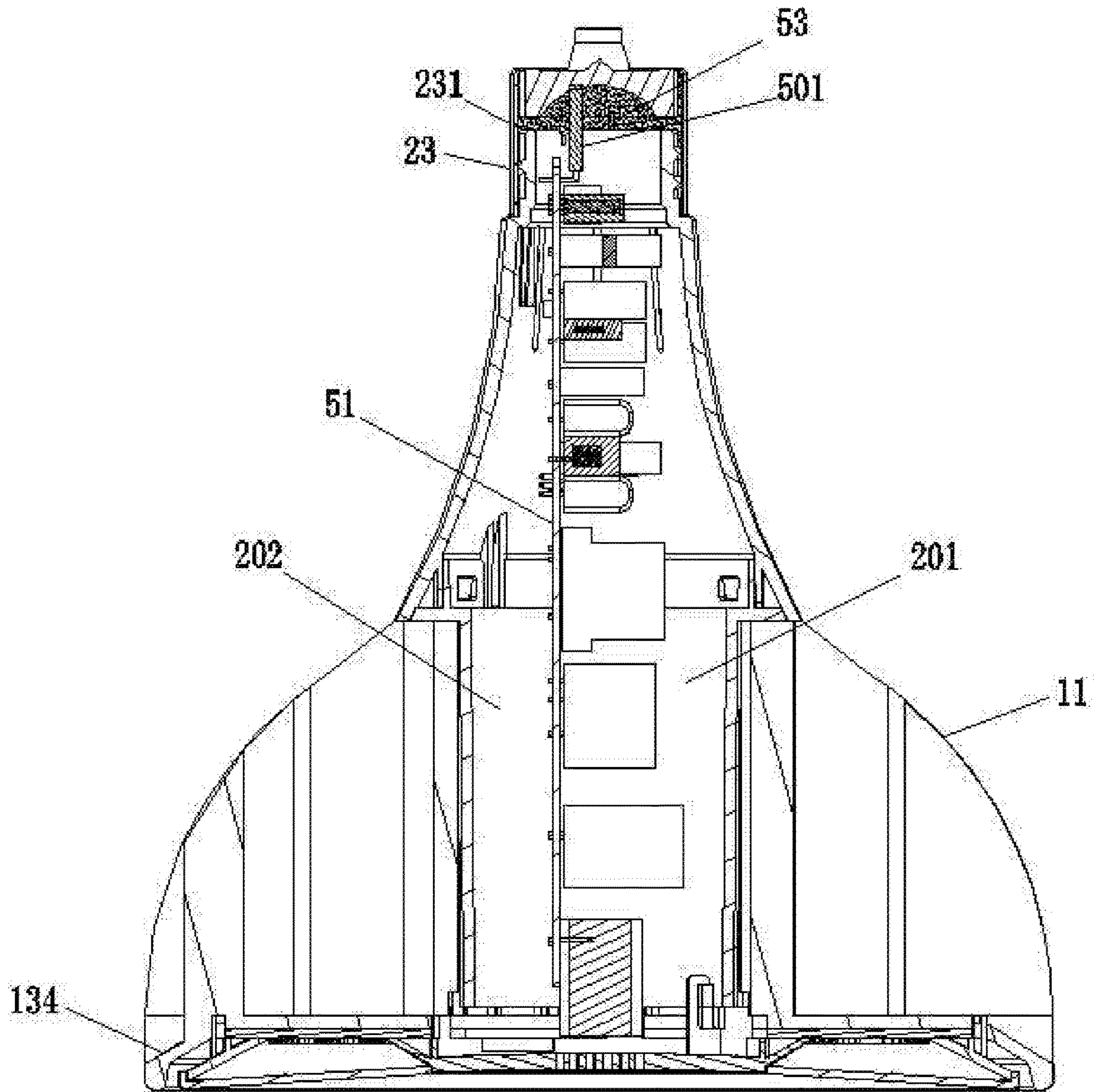
FIG. 15
