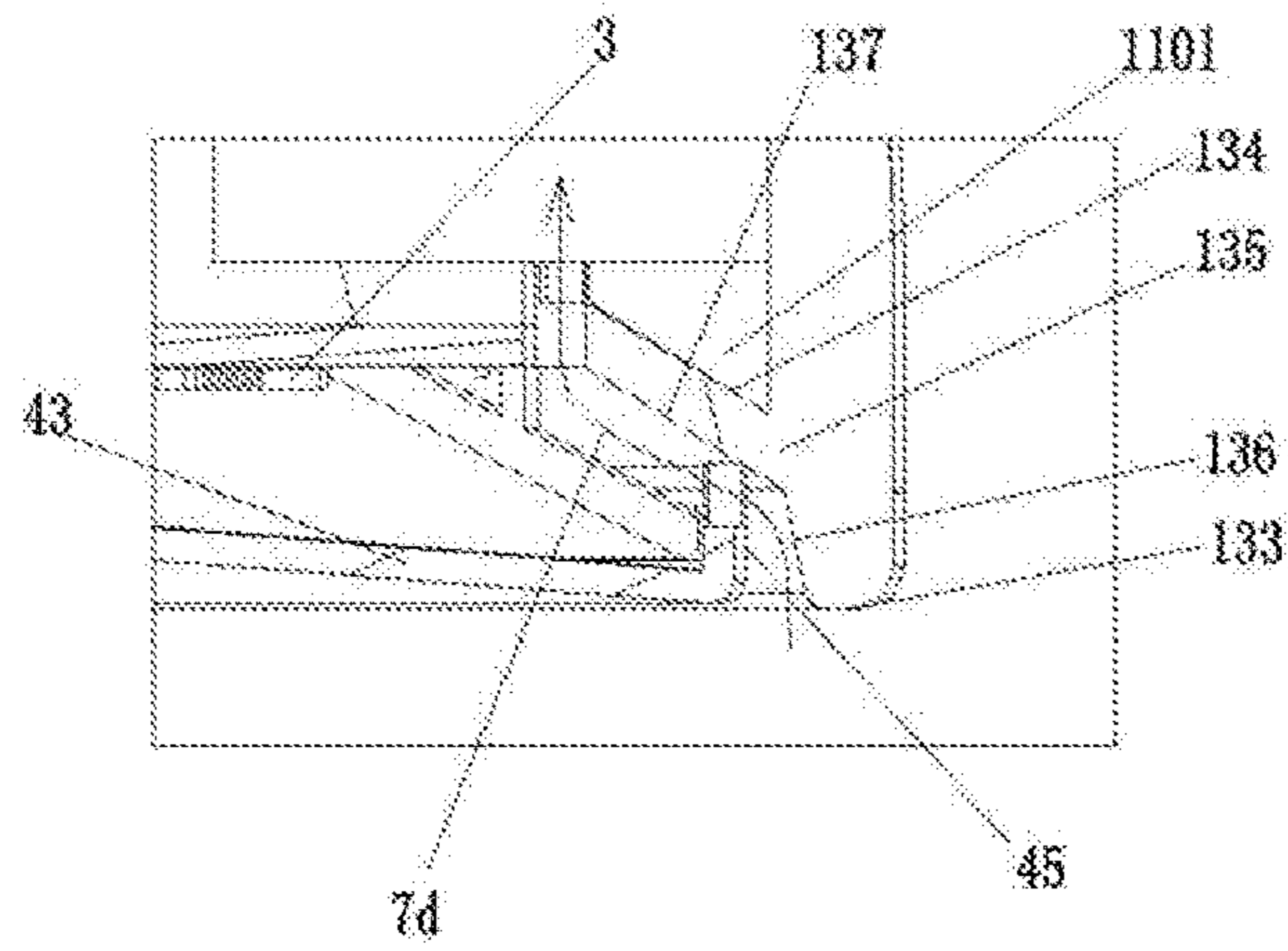
FIG. 23
