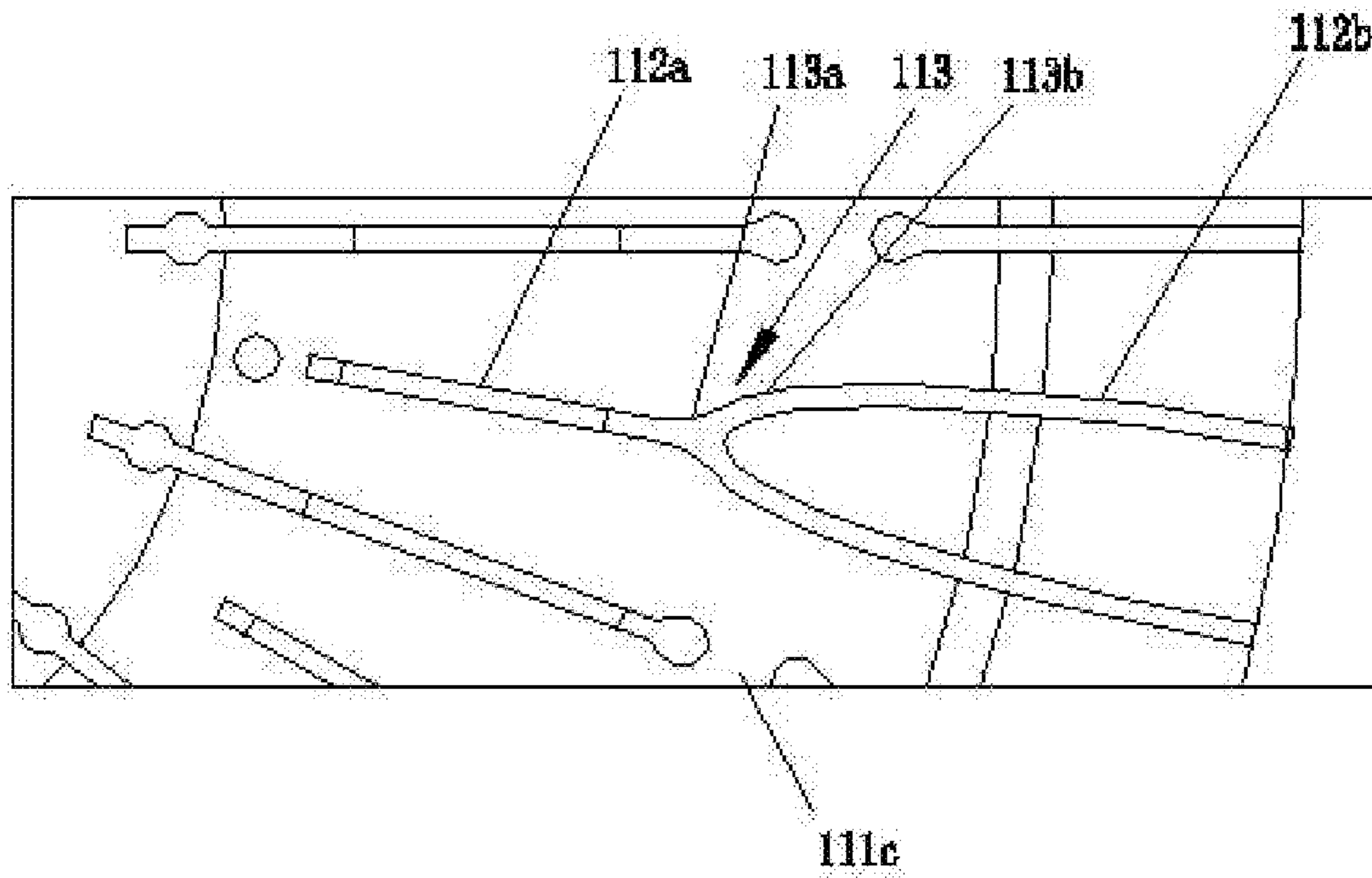
FIG. 19
