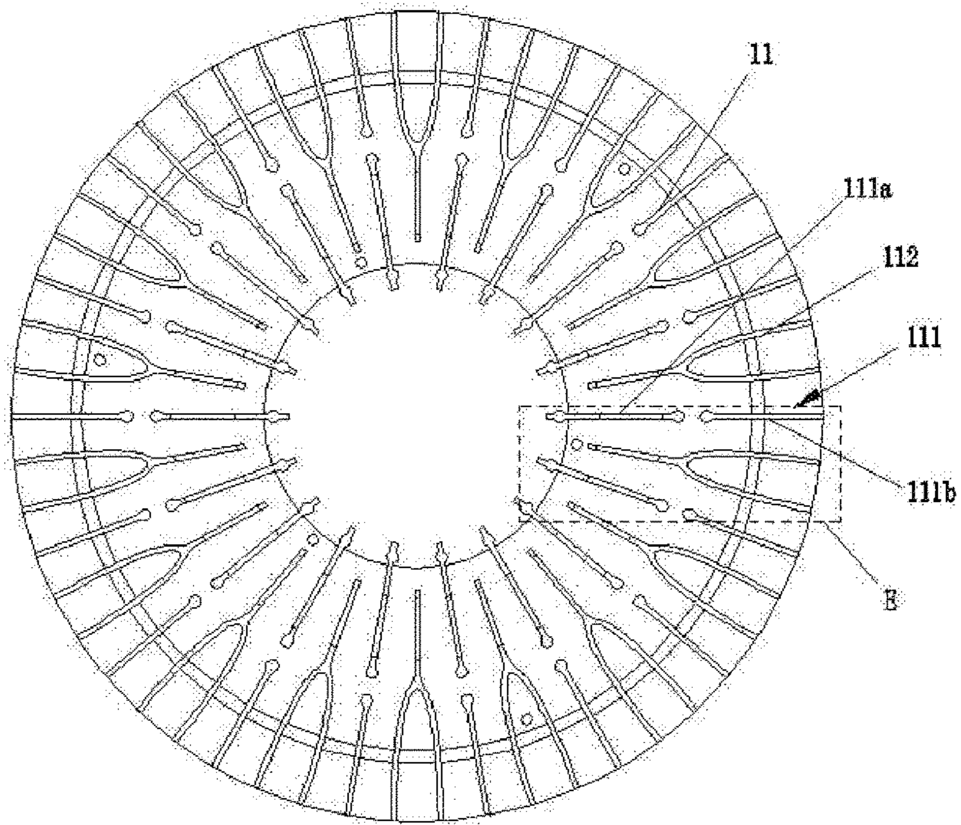
FIG. 16
