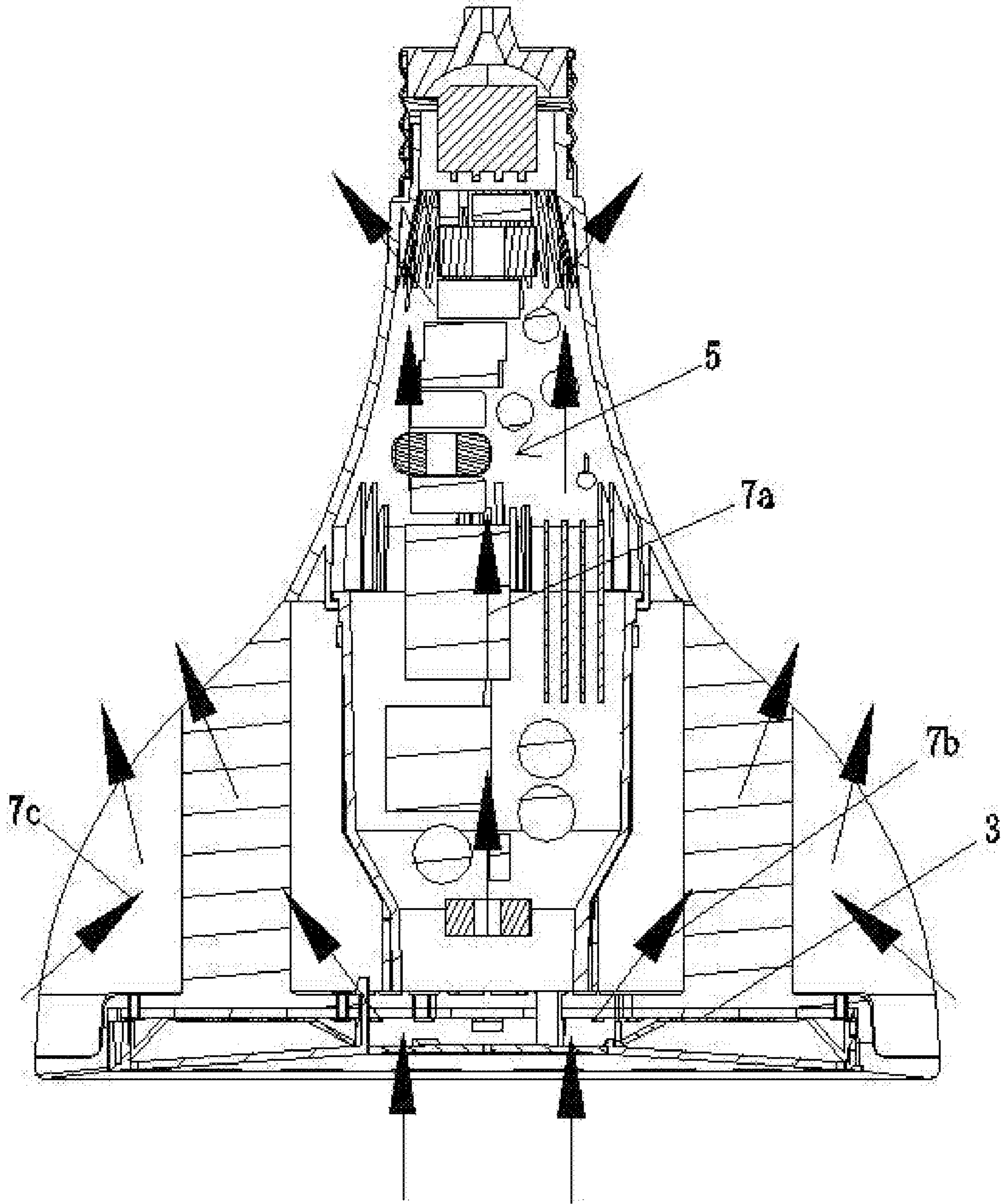
FIG. 37
