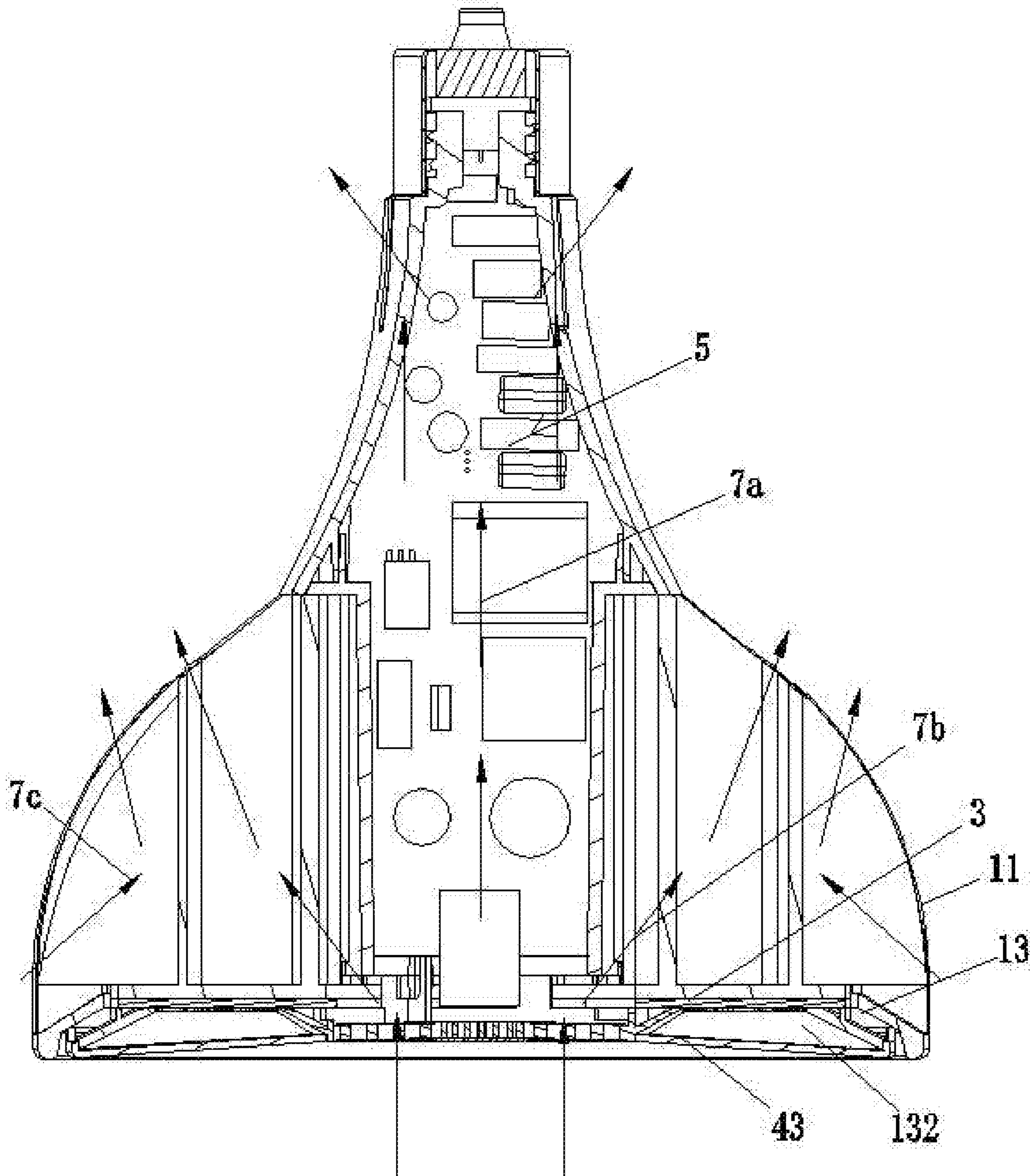
FIG. 4
