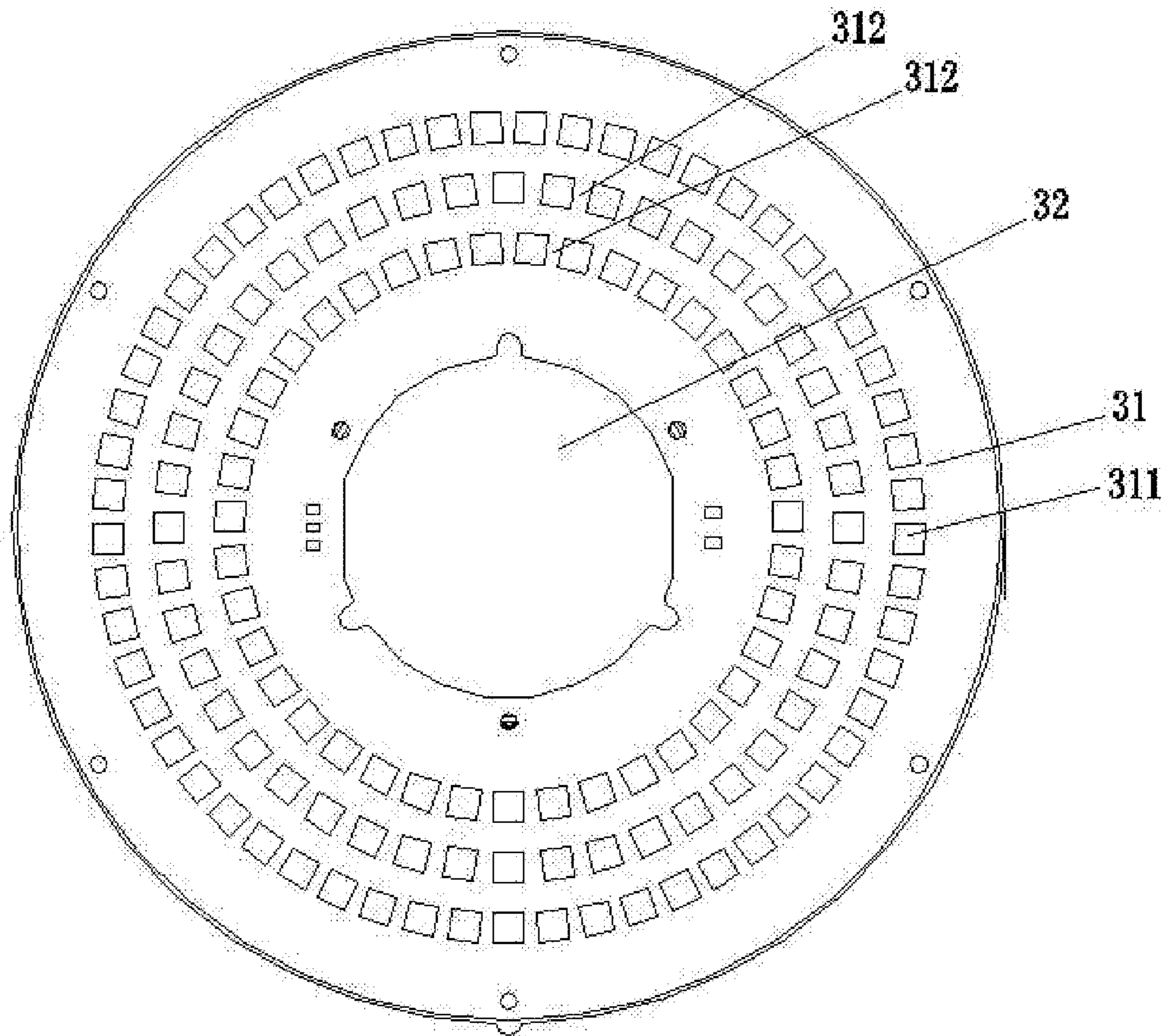
FIG. 27
