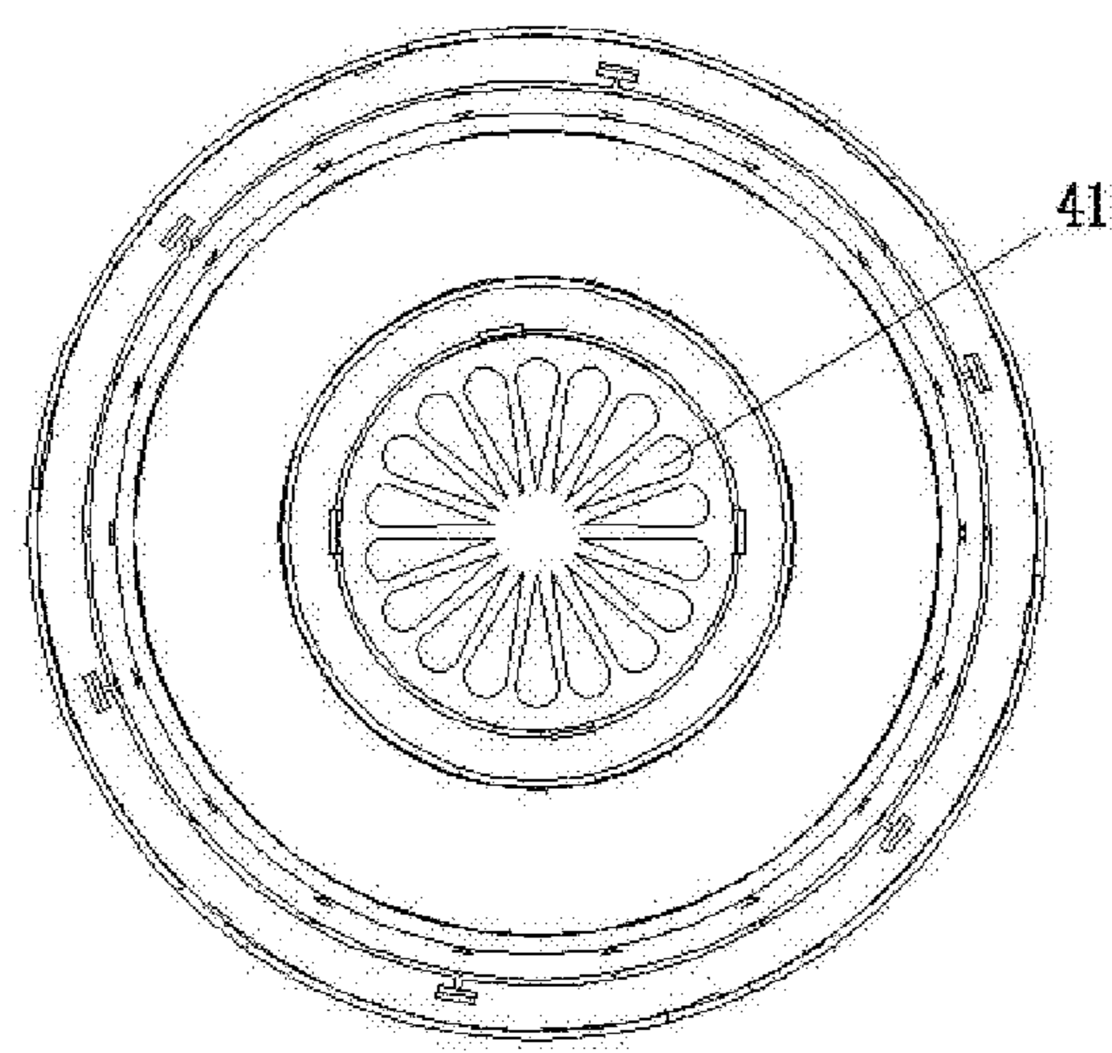
FIG. 12G
