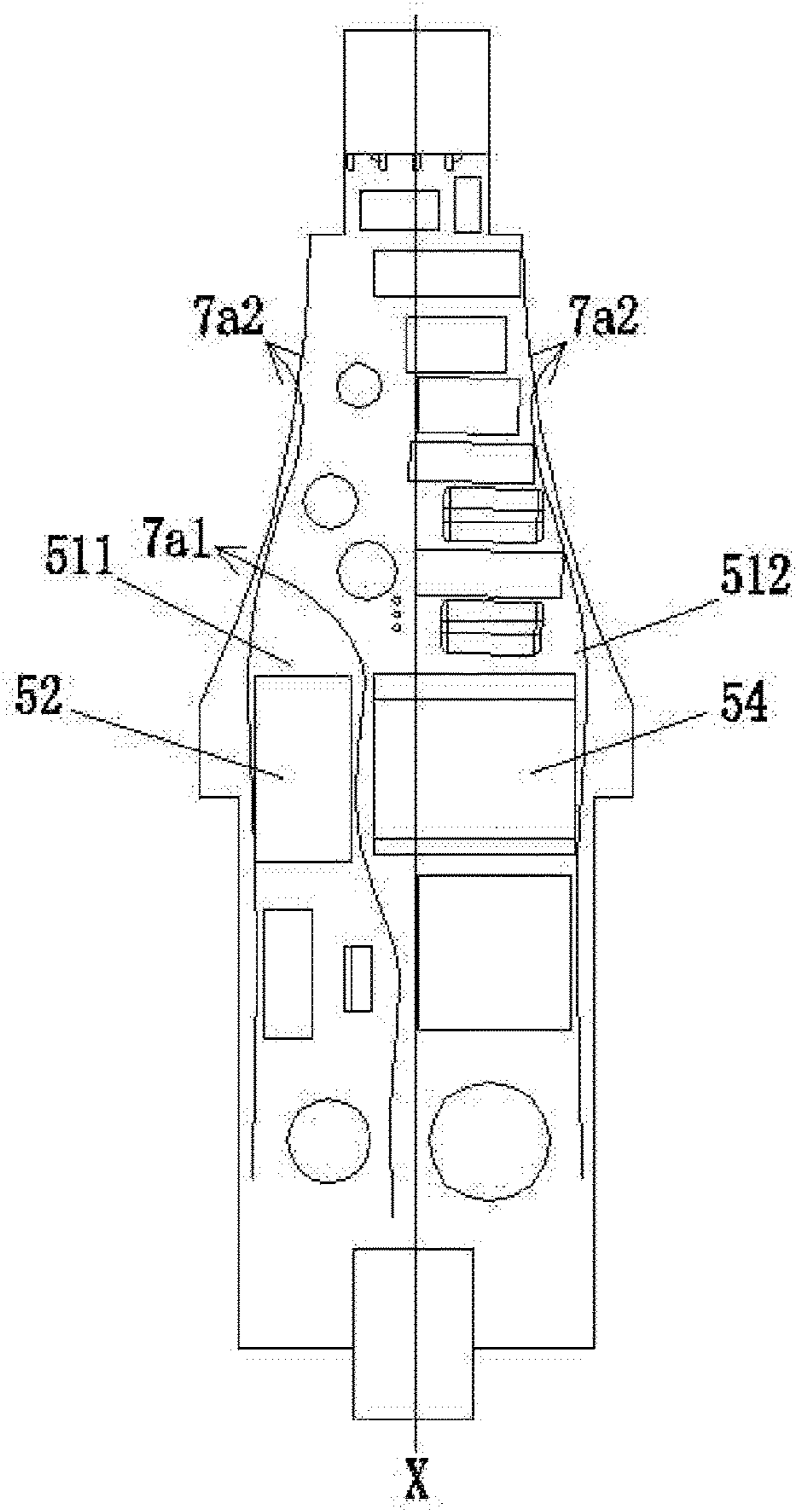
FIG. 29
