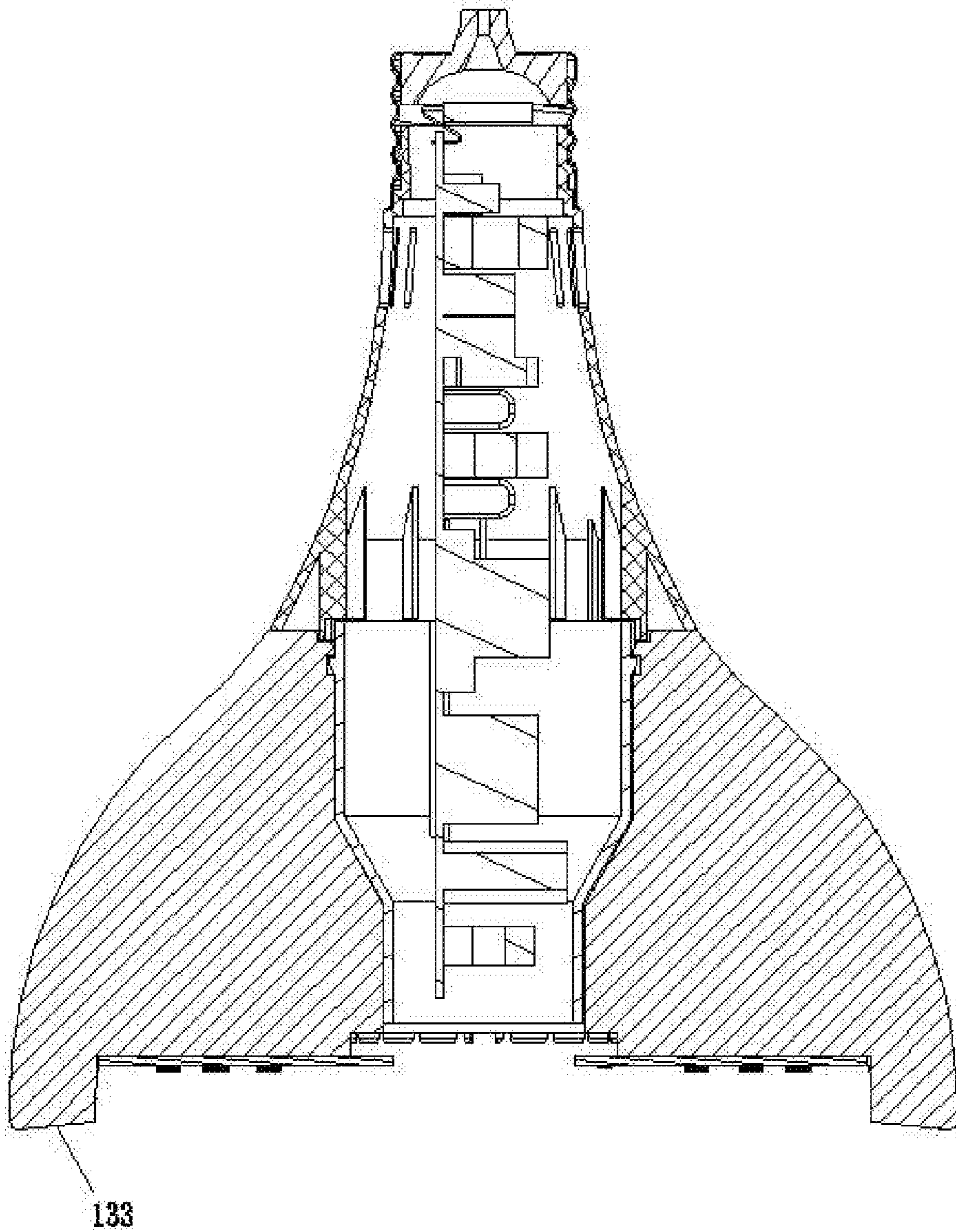
FIG. 13
