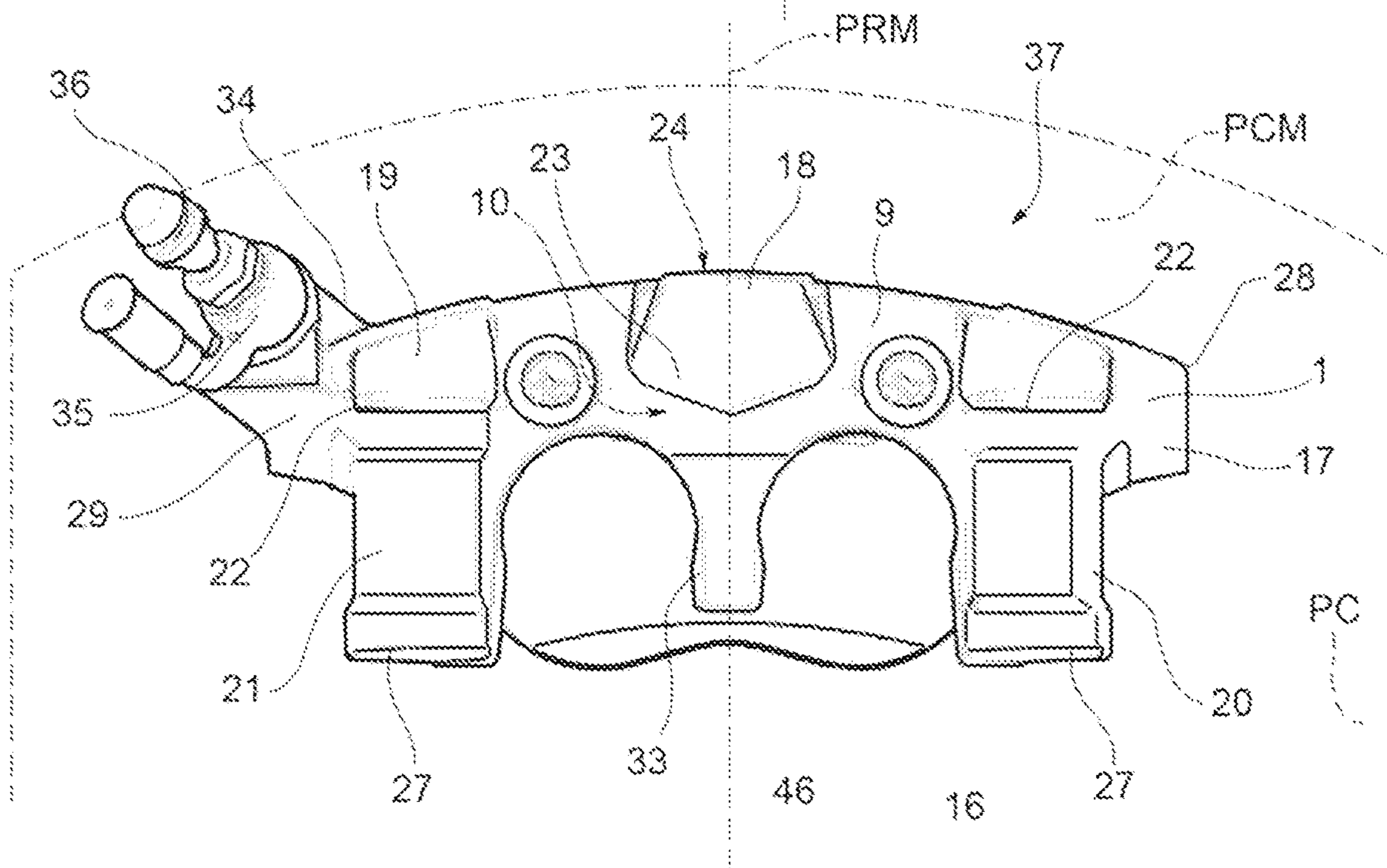
Fig. 2
