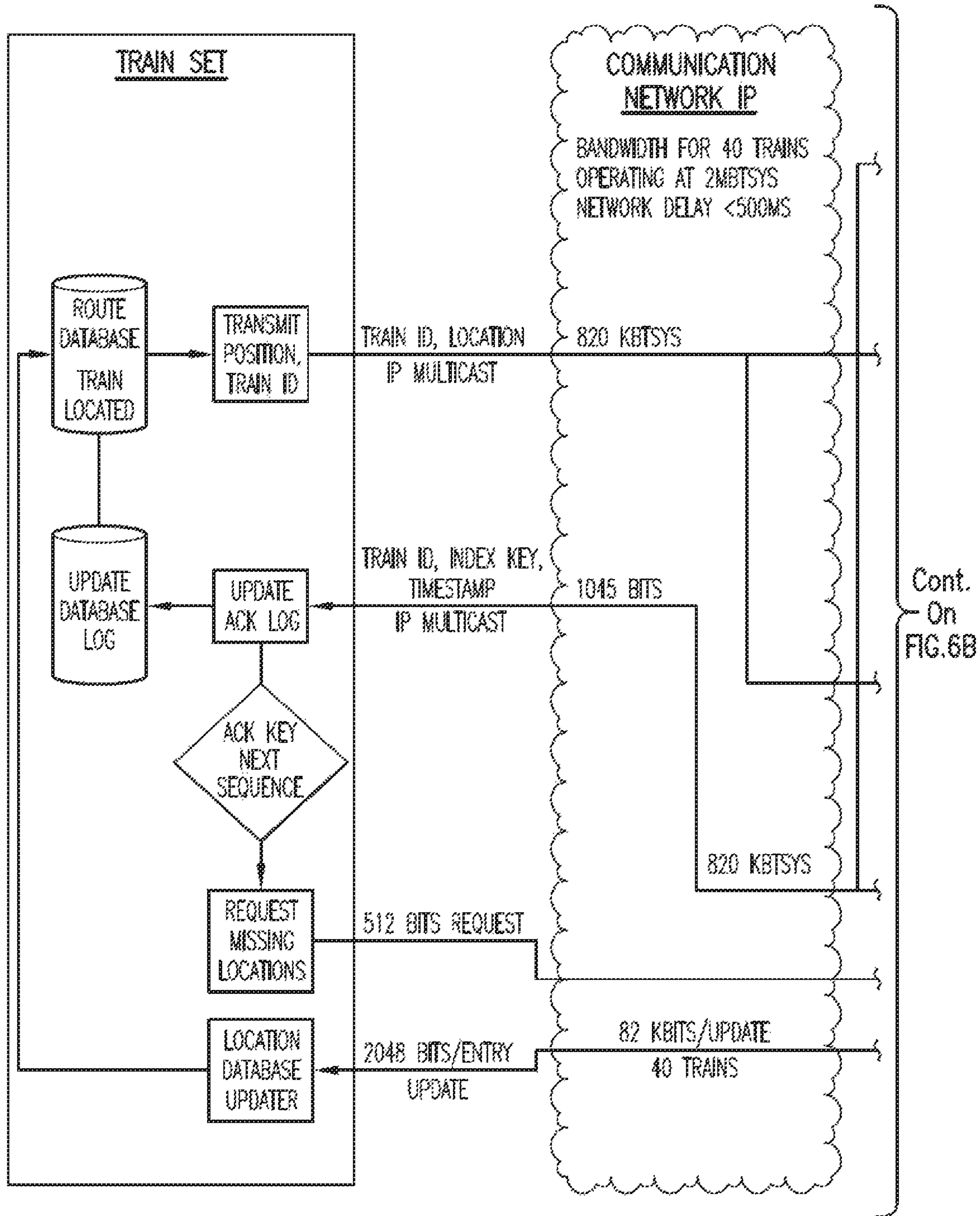
FIG. 6A
