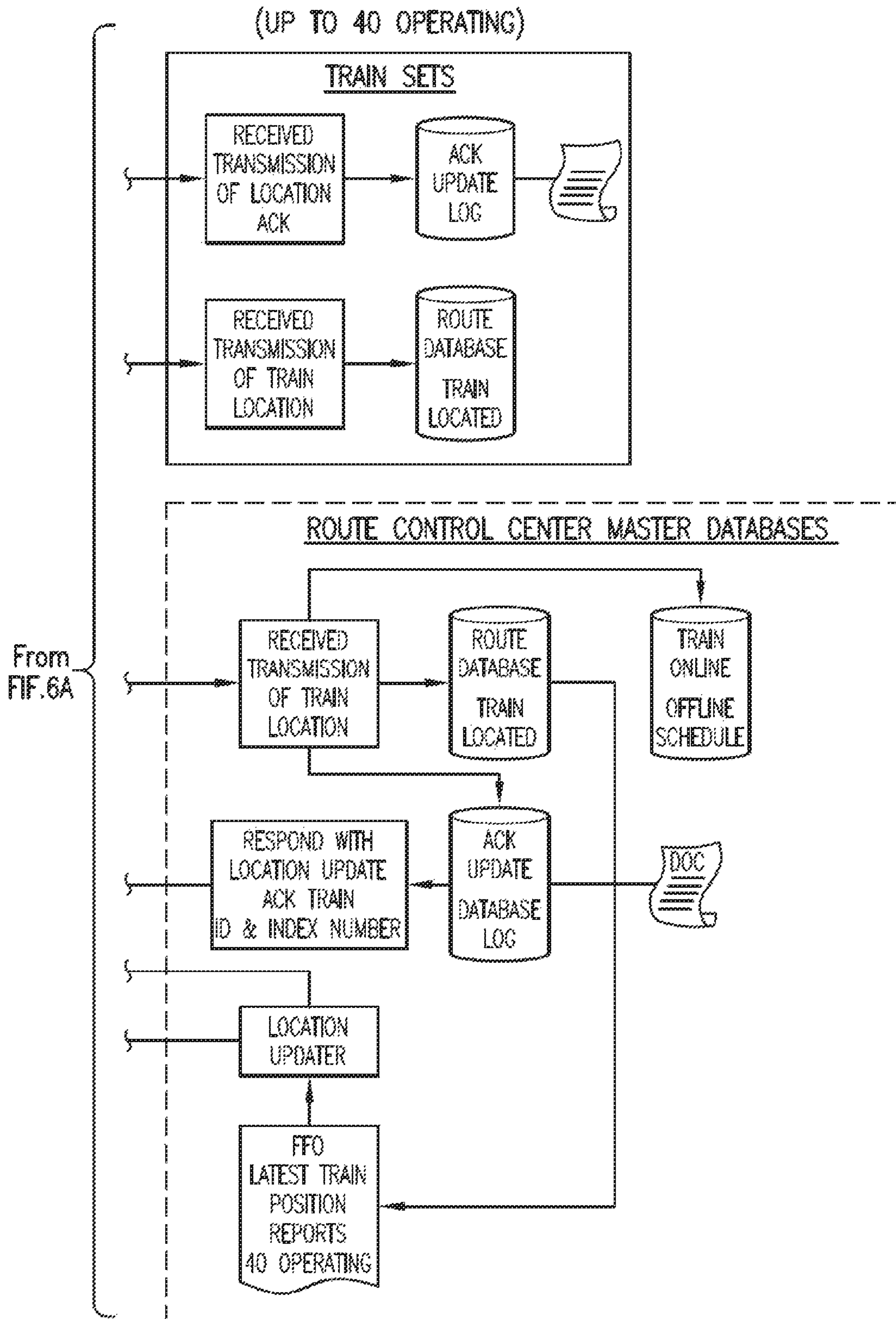
FIG. 6B
