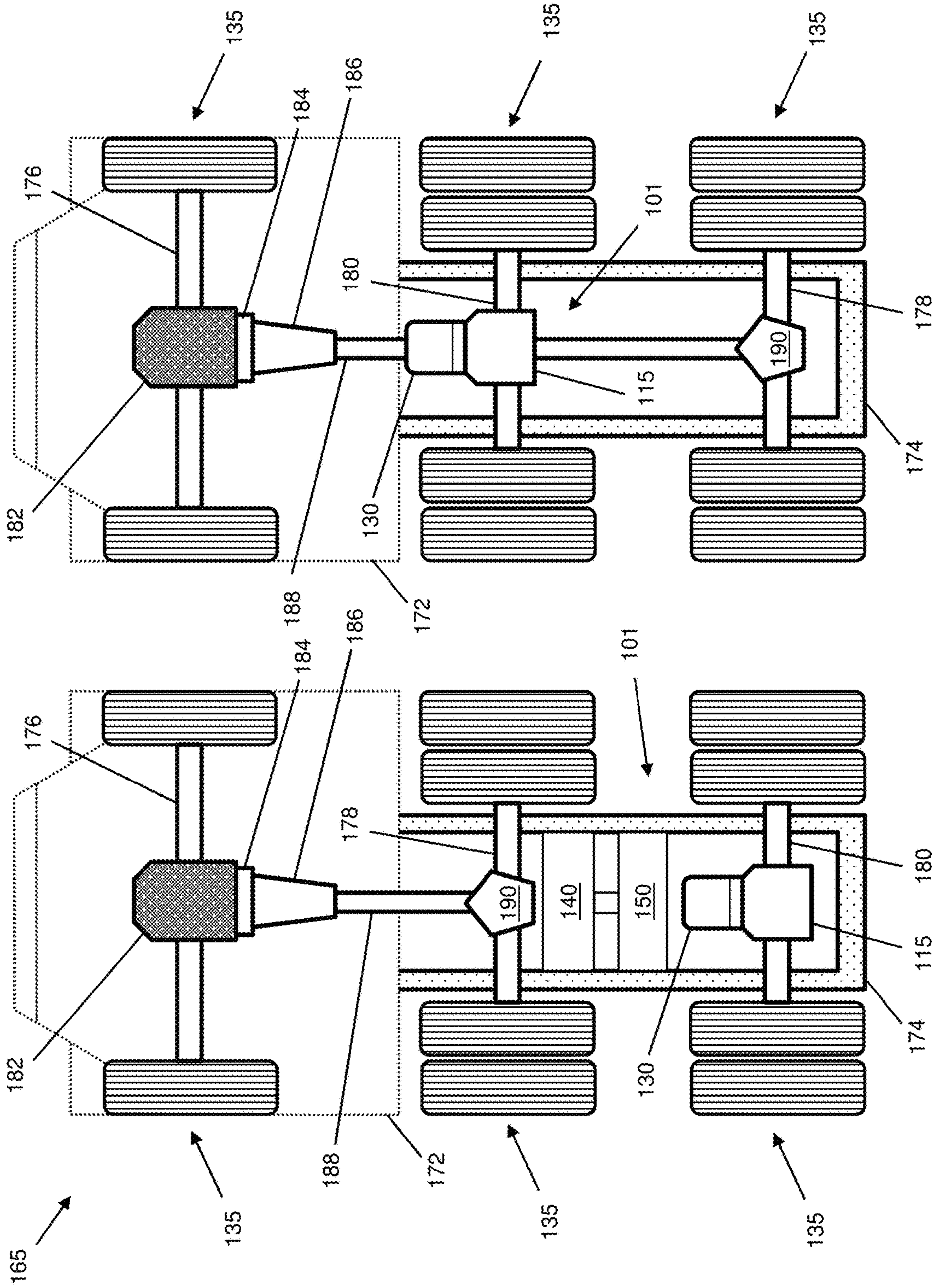
FIG. 1E
