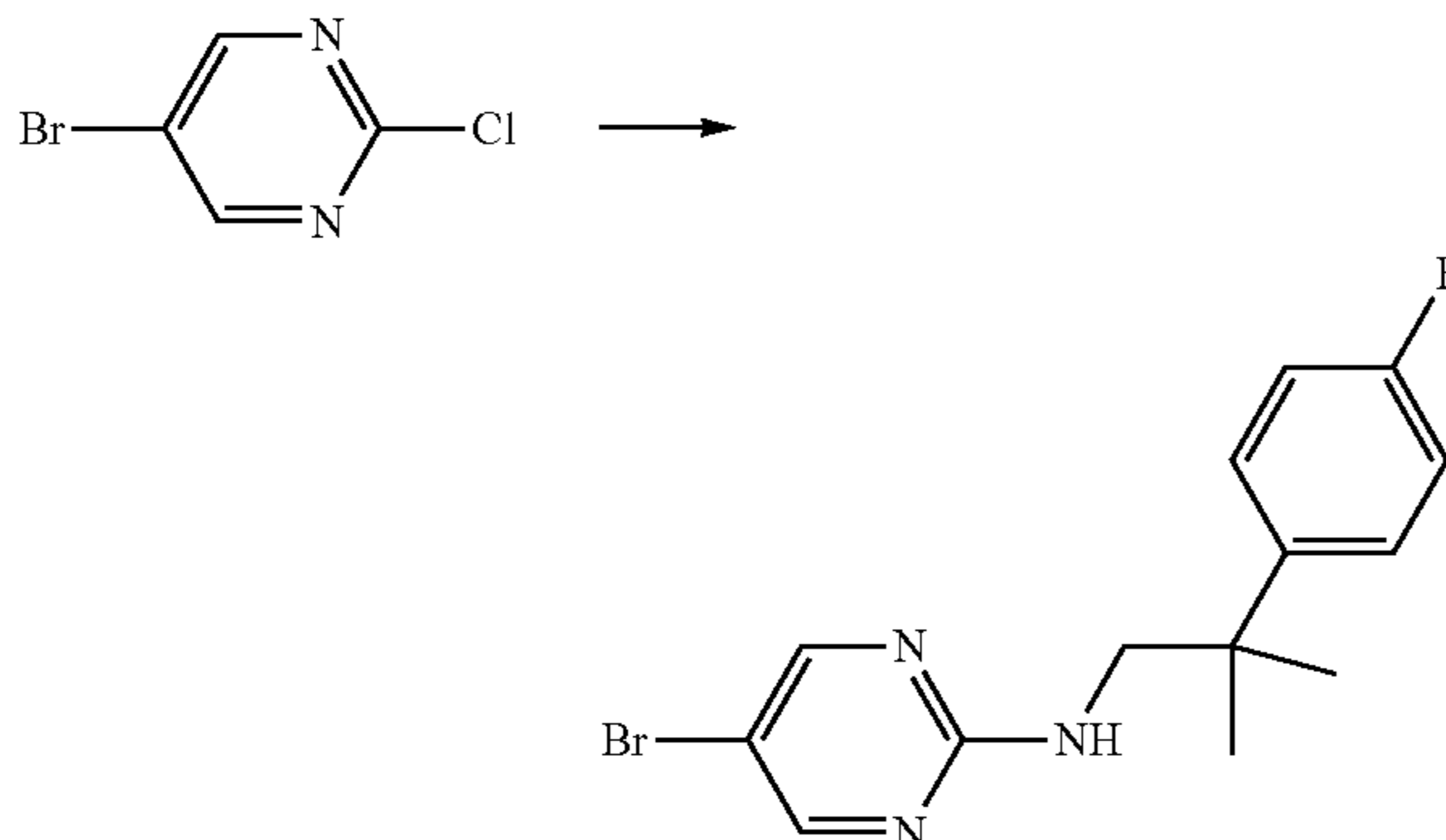
5-Bromo-N-(2-(4-fluorophenyl)-2-methylpropyl)pyrimidin-2-amine
