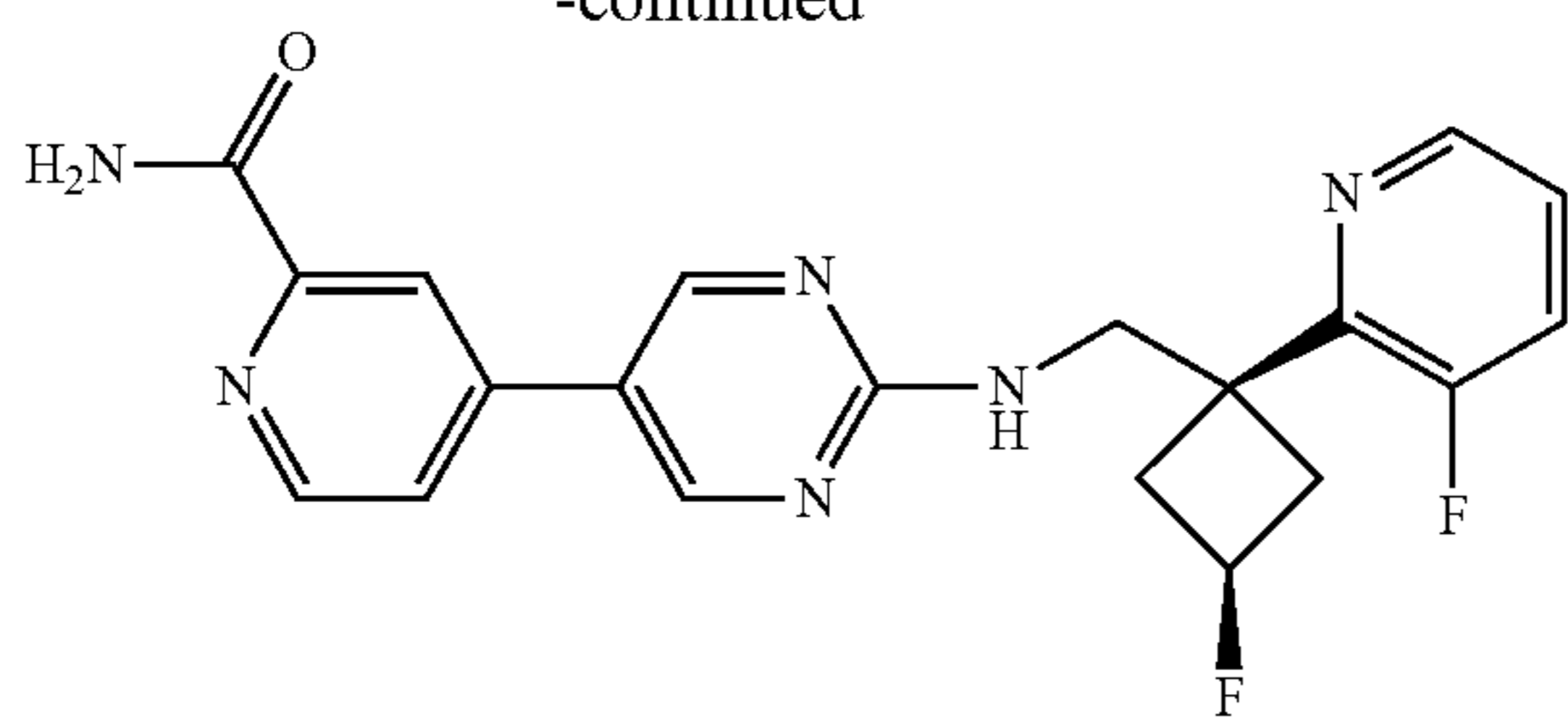
4-(2-(((cis)-3-fluoro-1-(3-fluoropyridin-2-yl)cyclobutyl)methylamino)pyrimidin-5-yl)picolinamide
