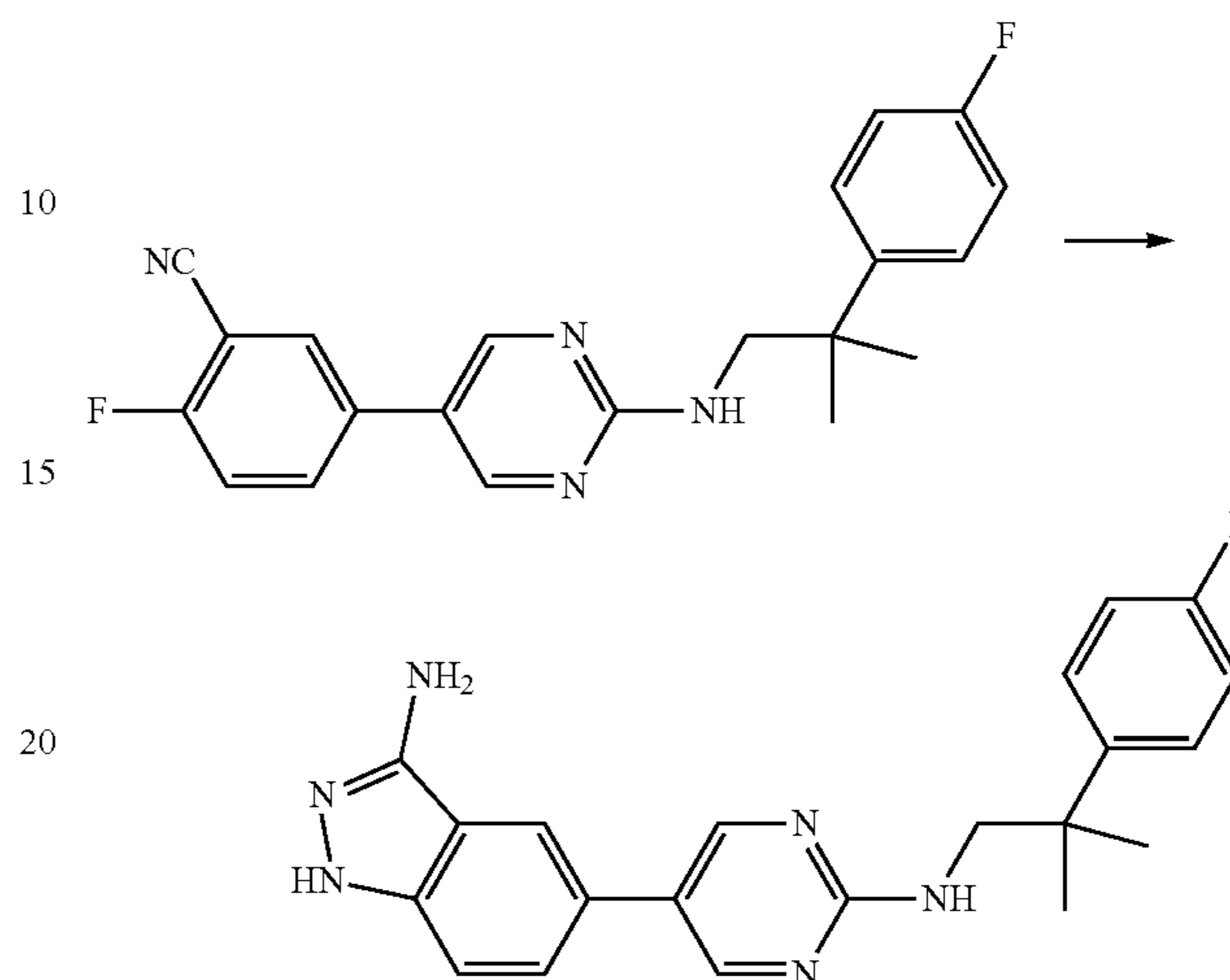
5-(2-(2-(4-Fluorophenyl)-2-methylpropylamino)pyrimidin-5-yl)-1H-indazol-3-amine
