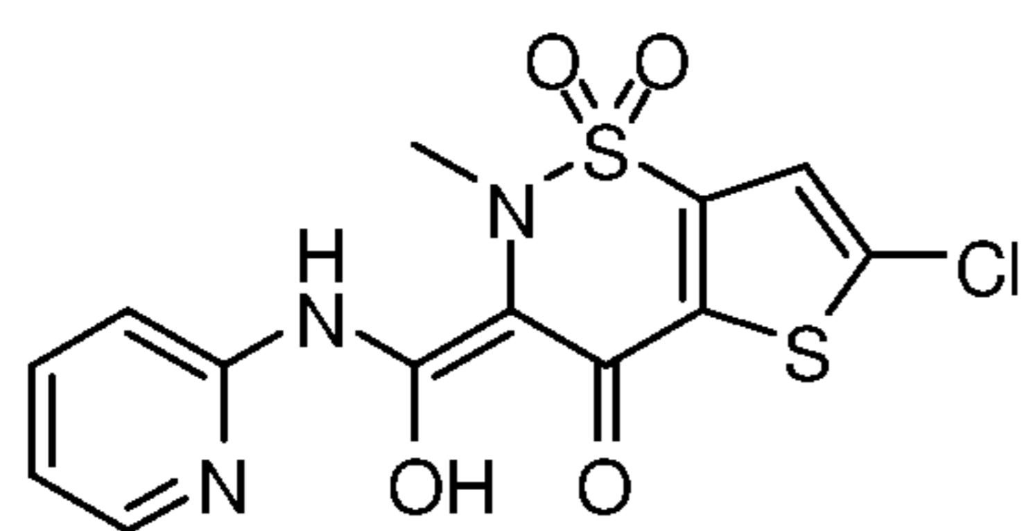
Lornoxicam
