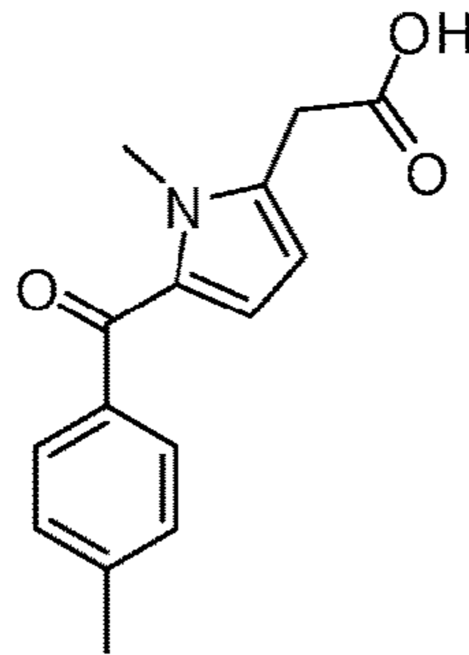
Tolmetin
