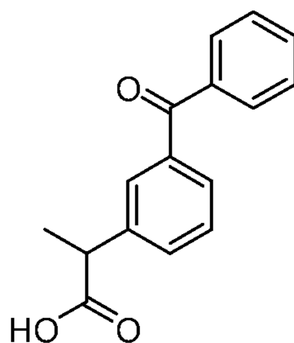
Ketoprofen
