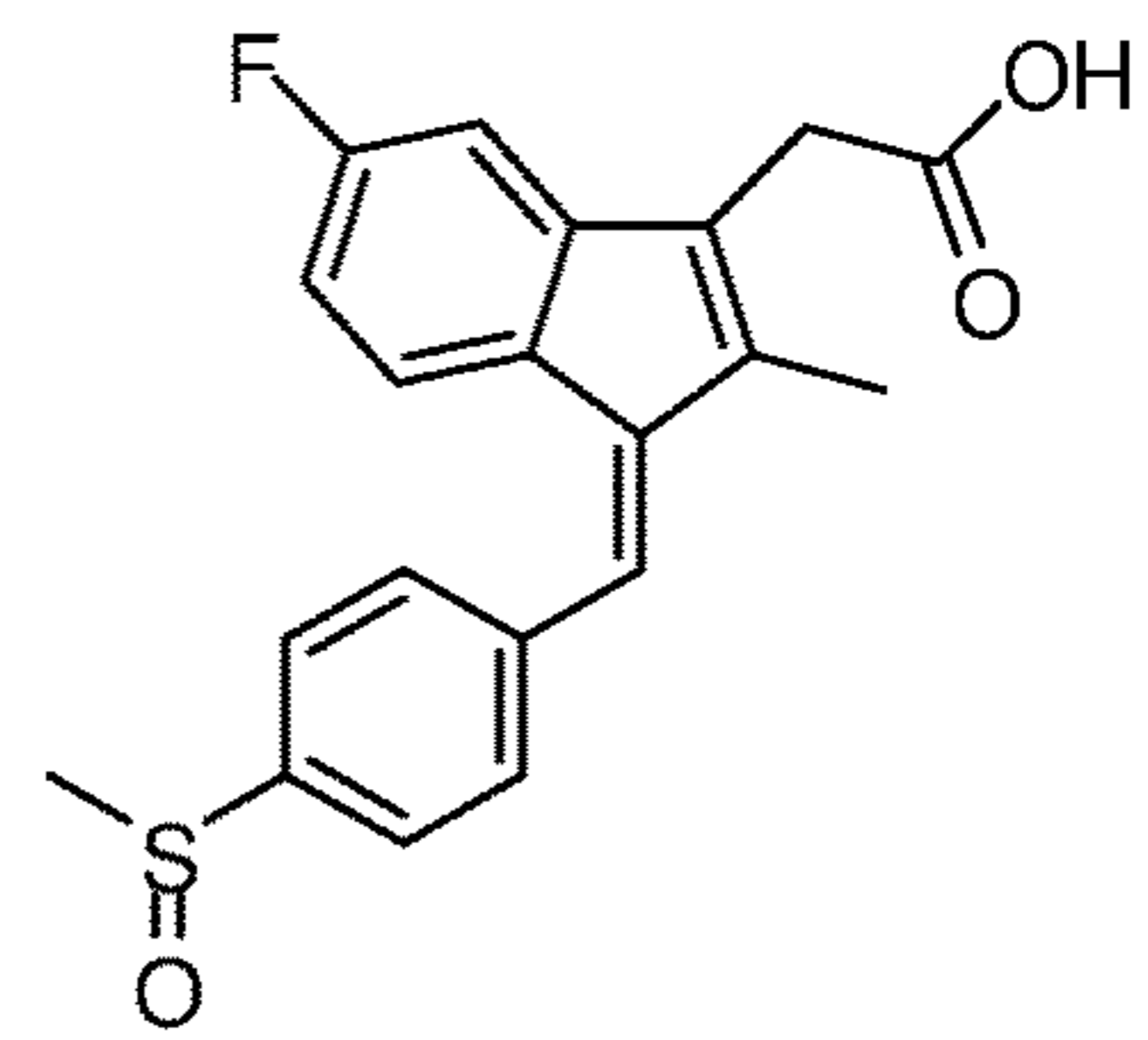
Sulindac
