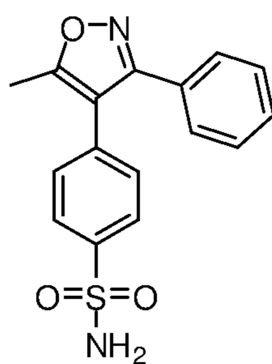
Valdecoxib
