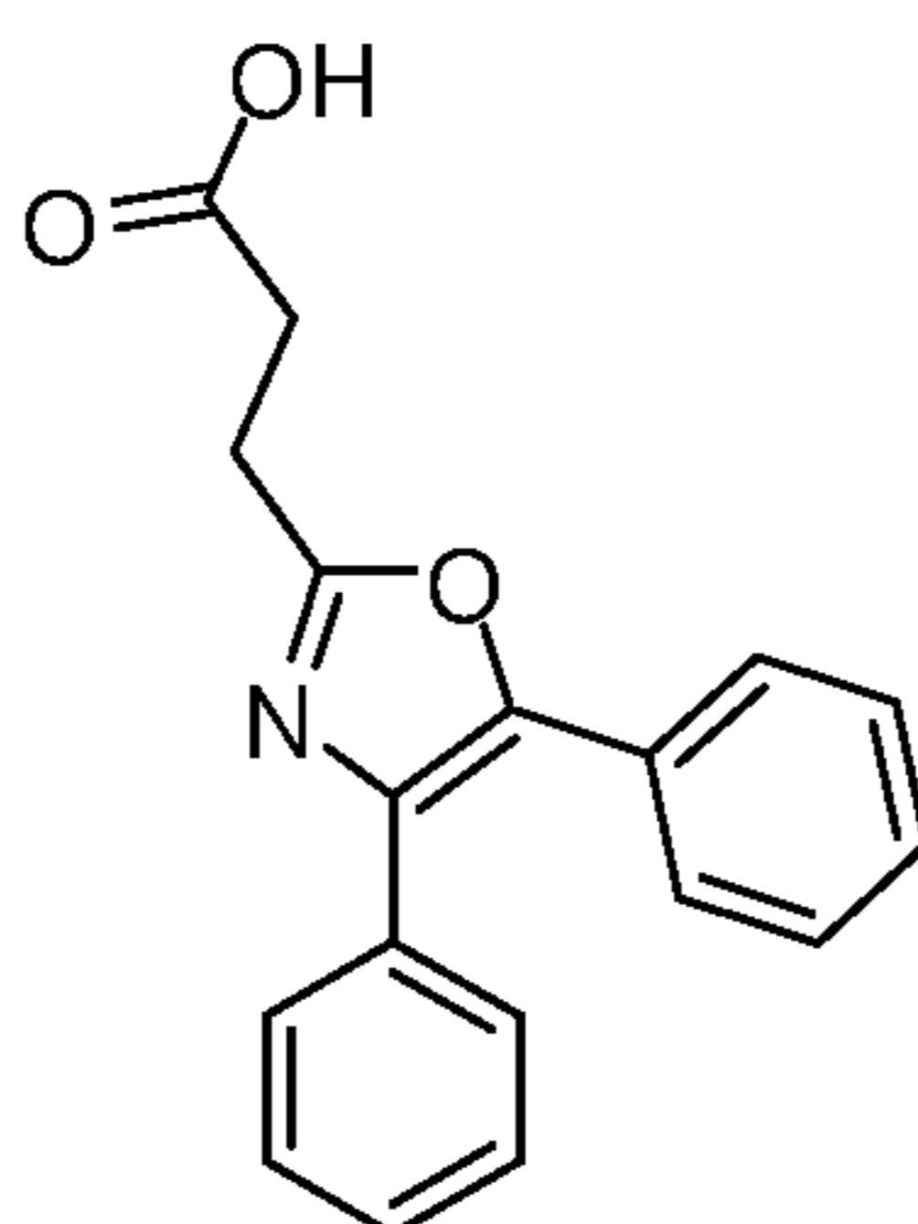
Oxaprozin
