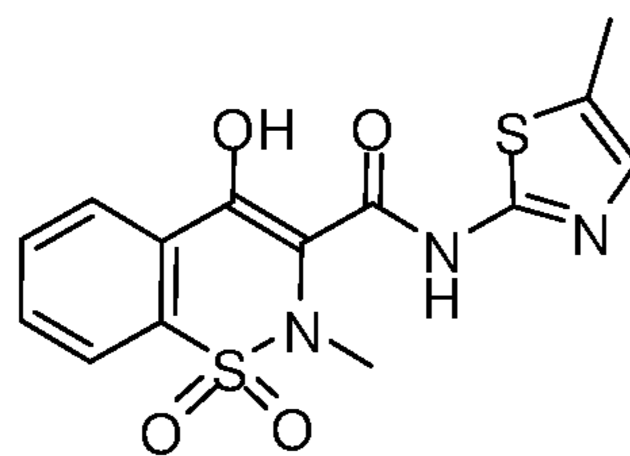
Meloxicam
