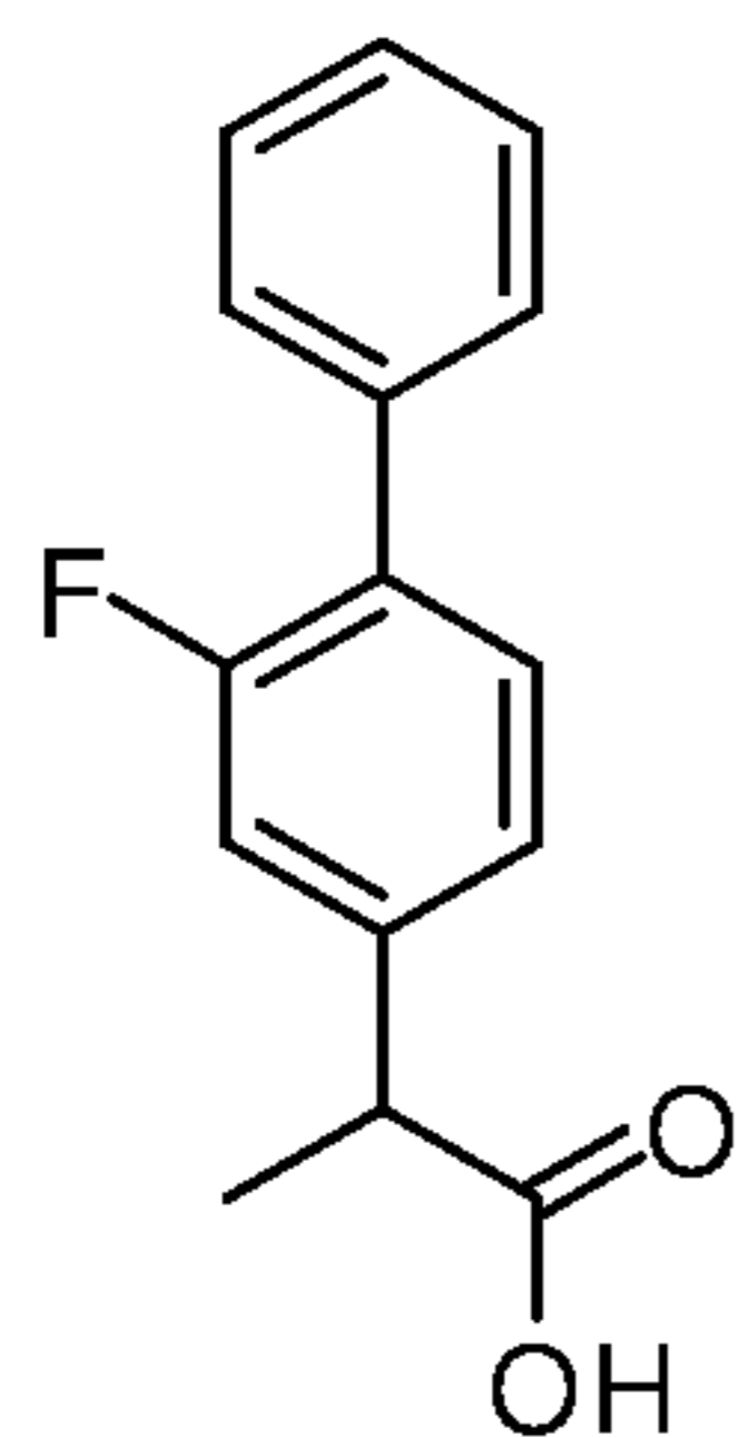
Flurbiprofen
