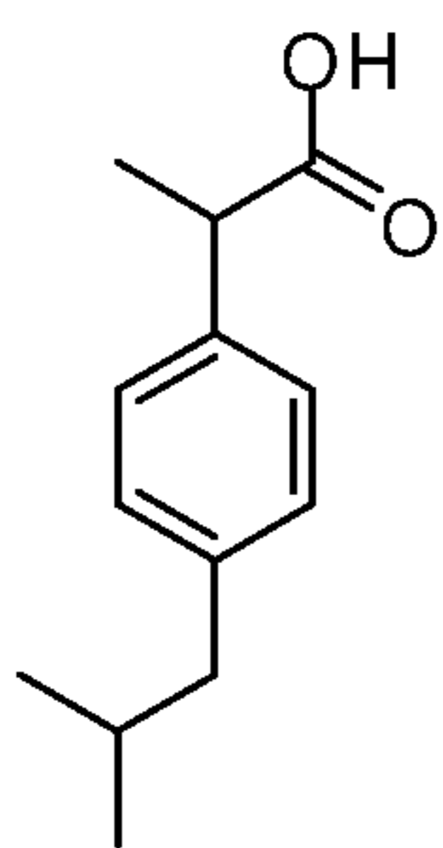
Ibuprofen
