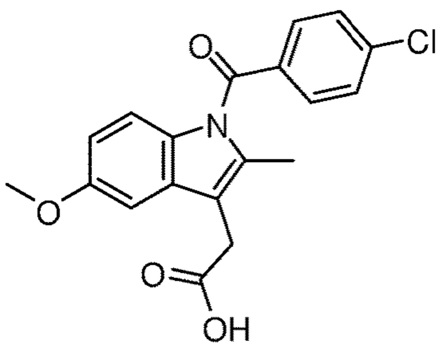
Indomethacin
