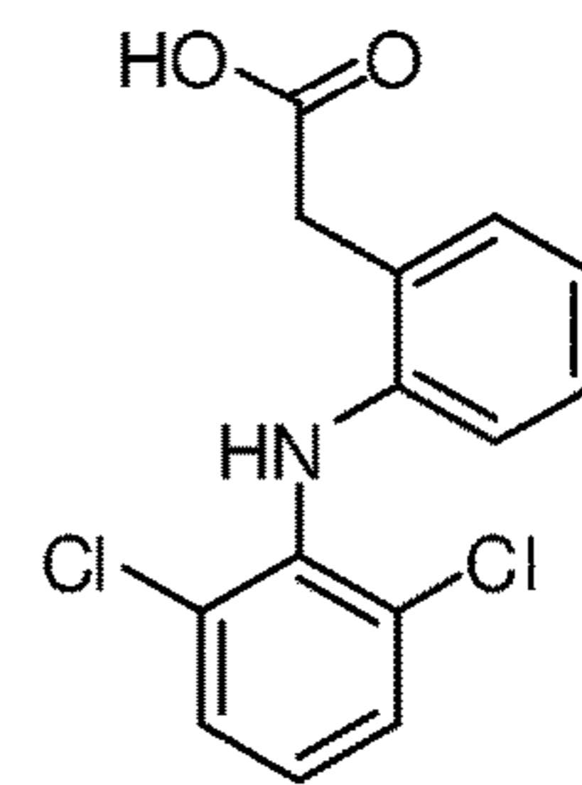
Diclofenac
