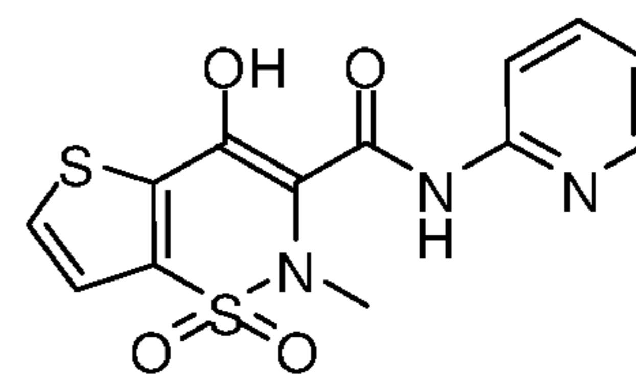
Tenoxicam
