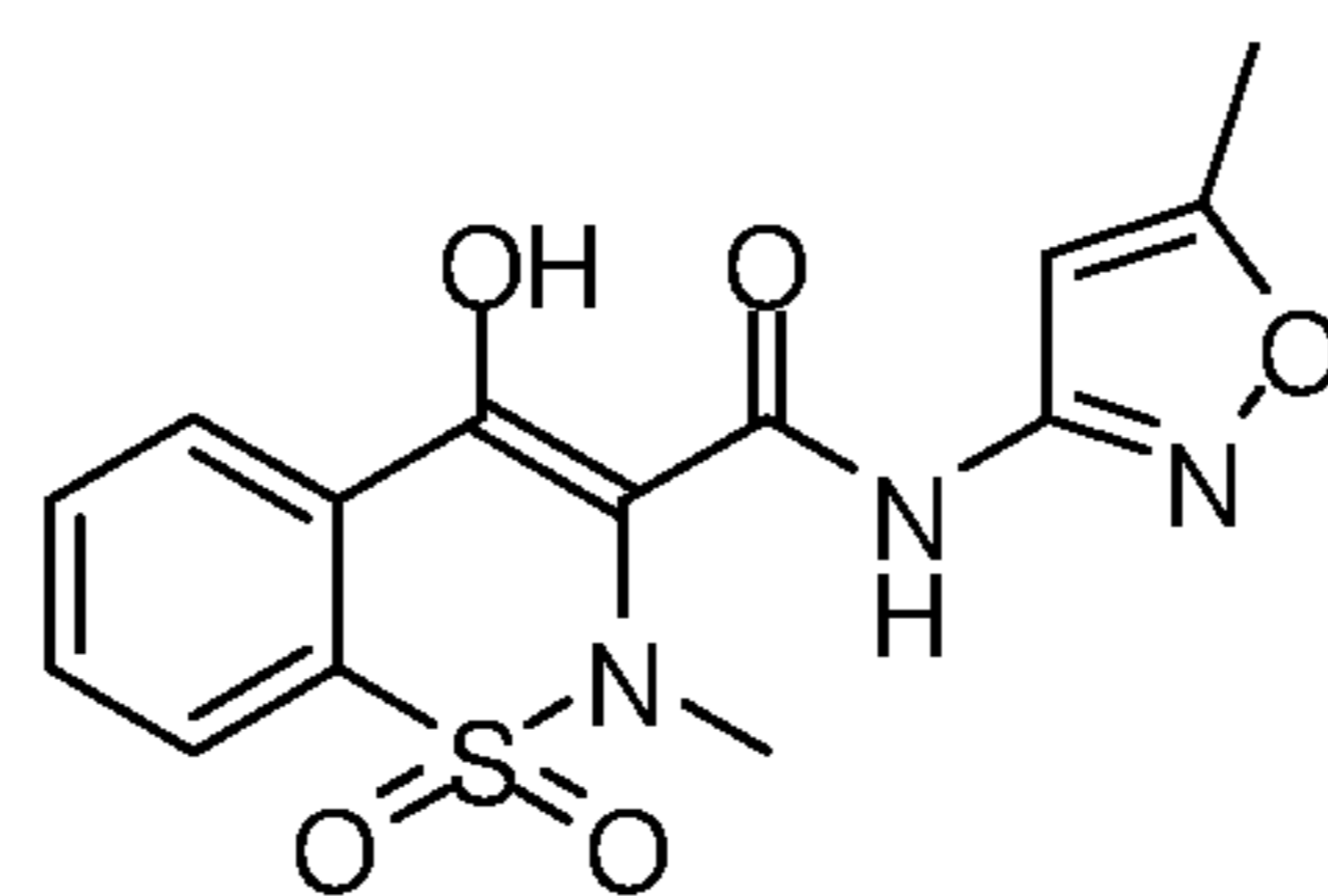
Isoxicam
