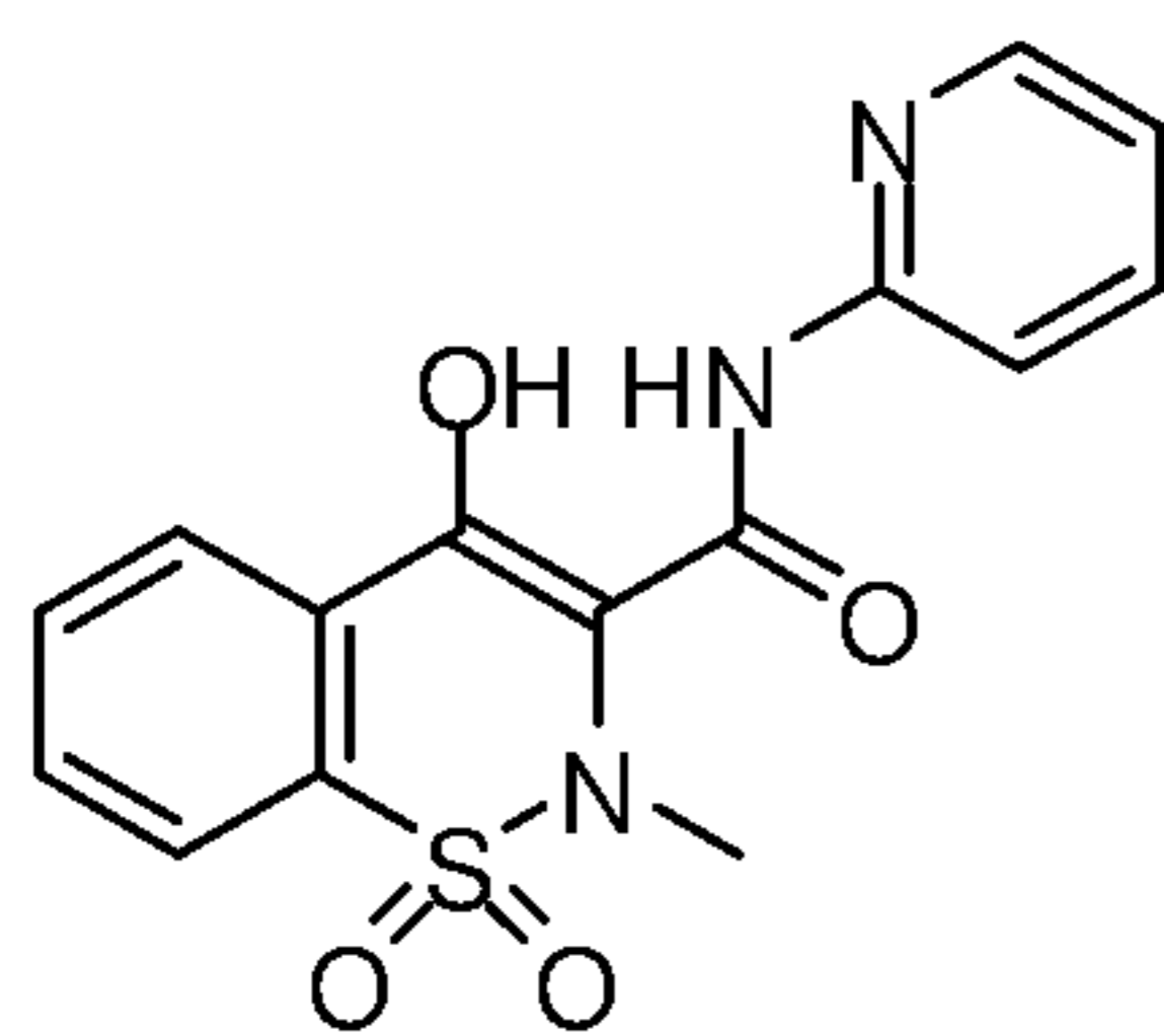
Piroxicam
