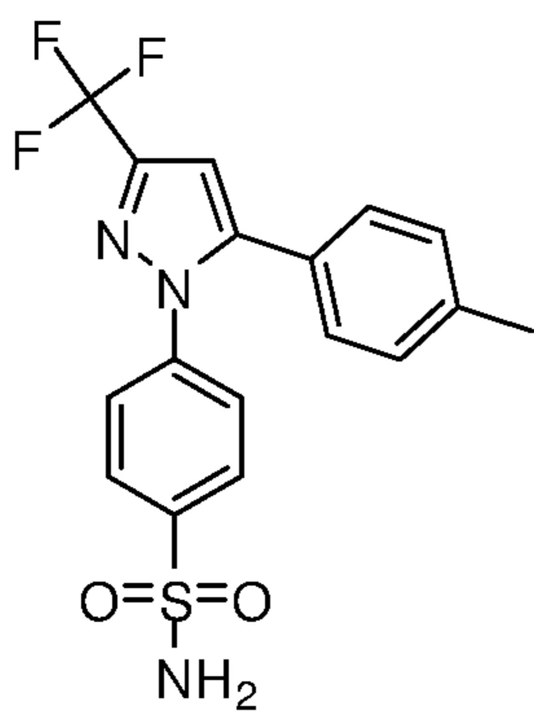
Celecoxib
