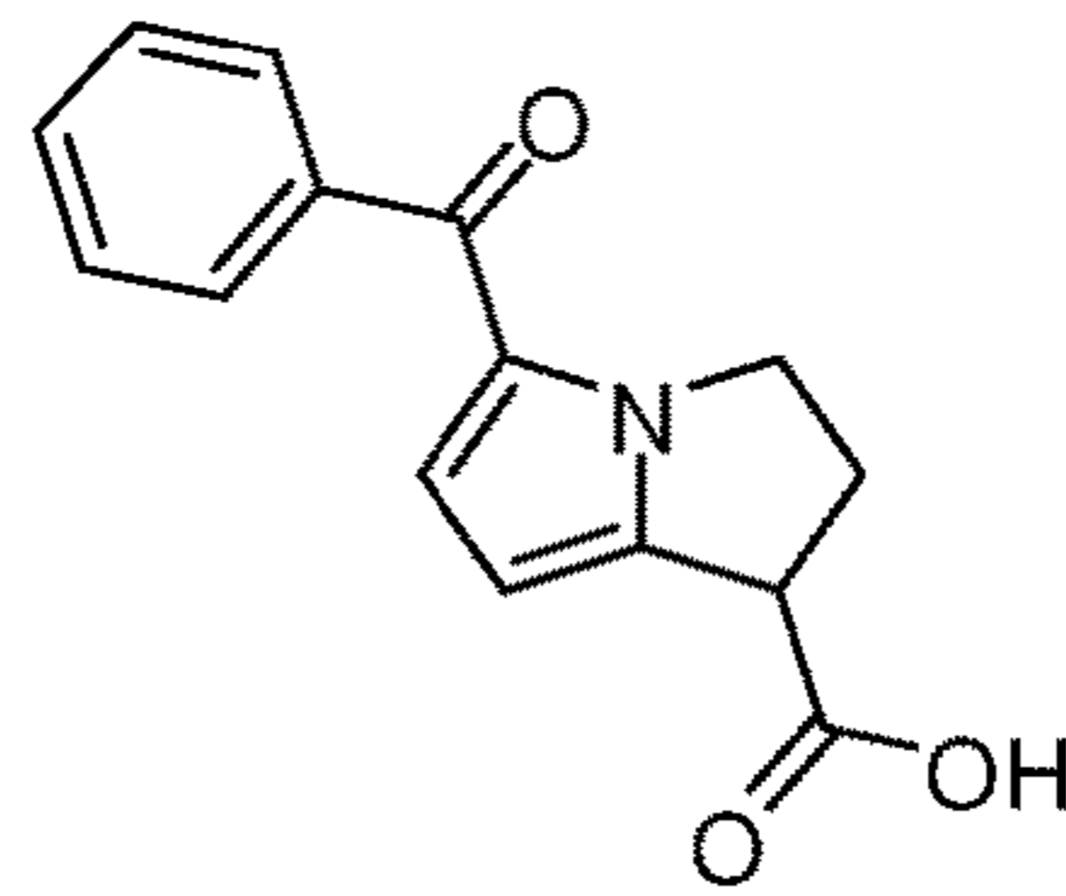
Ketorolac
