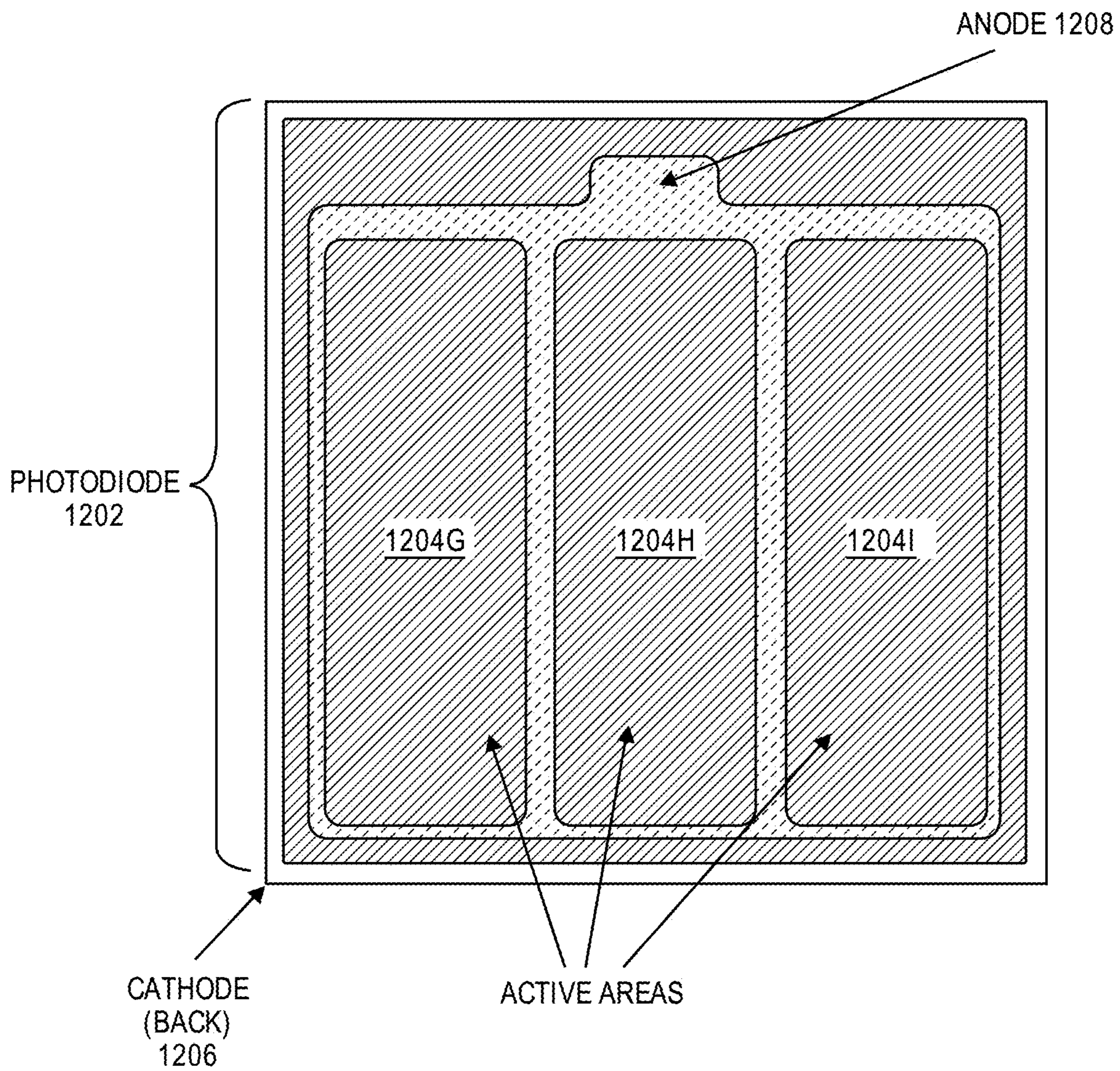
FIG. 12G
