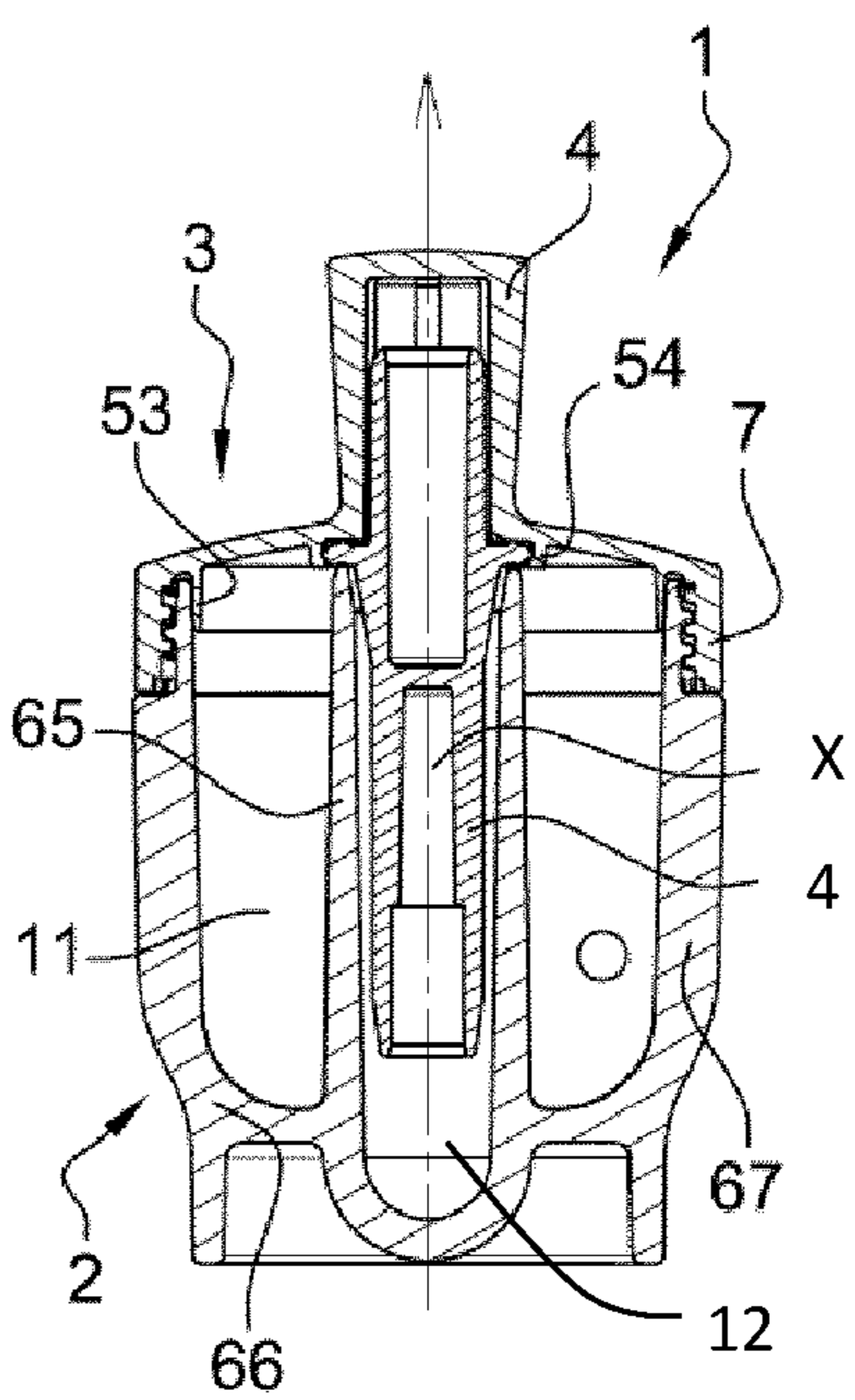
Fig. 5 Section B-B
