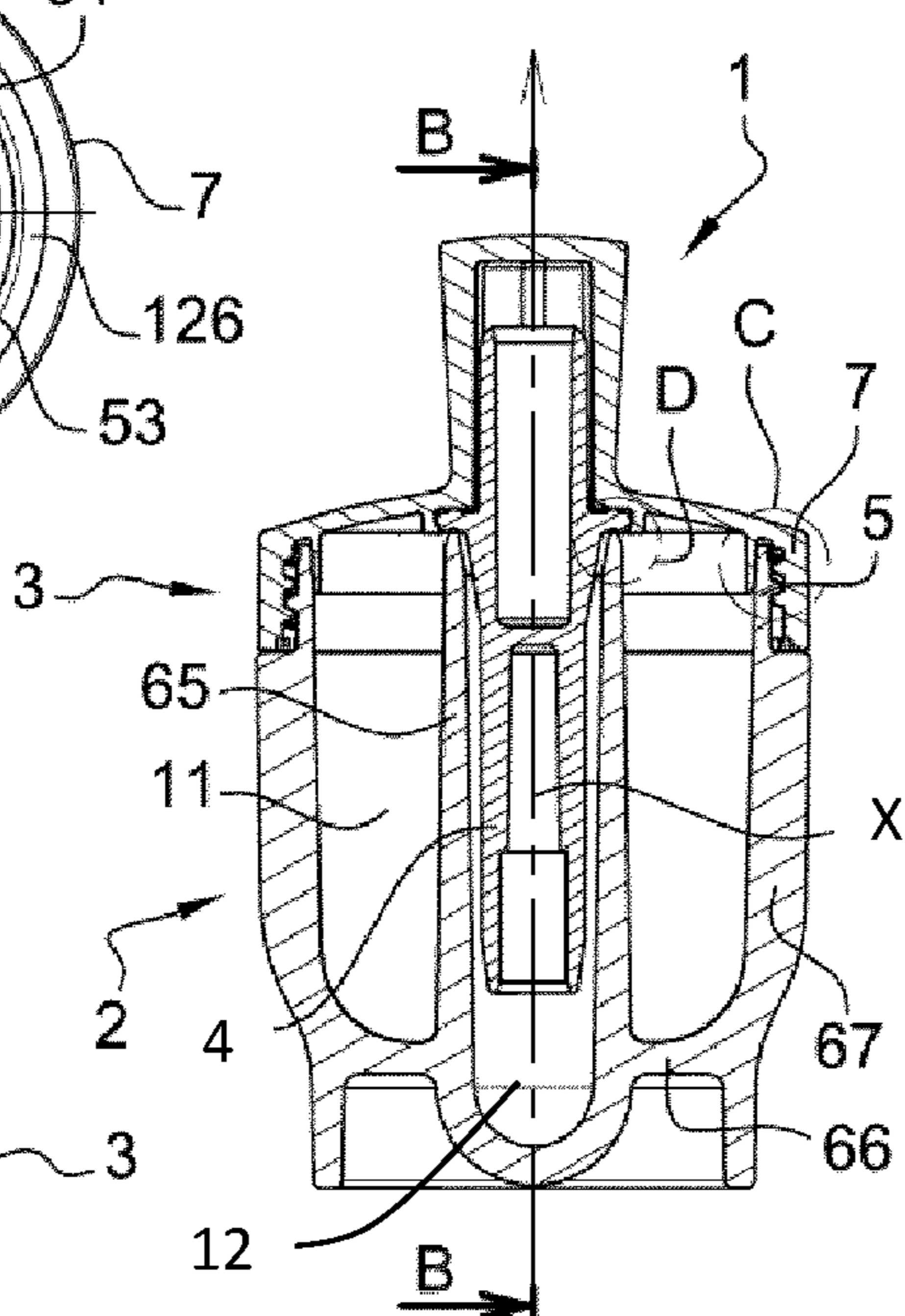
Fig. 4 Section A-A
