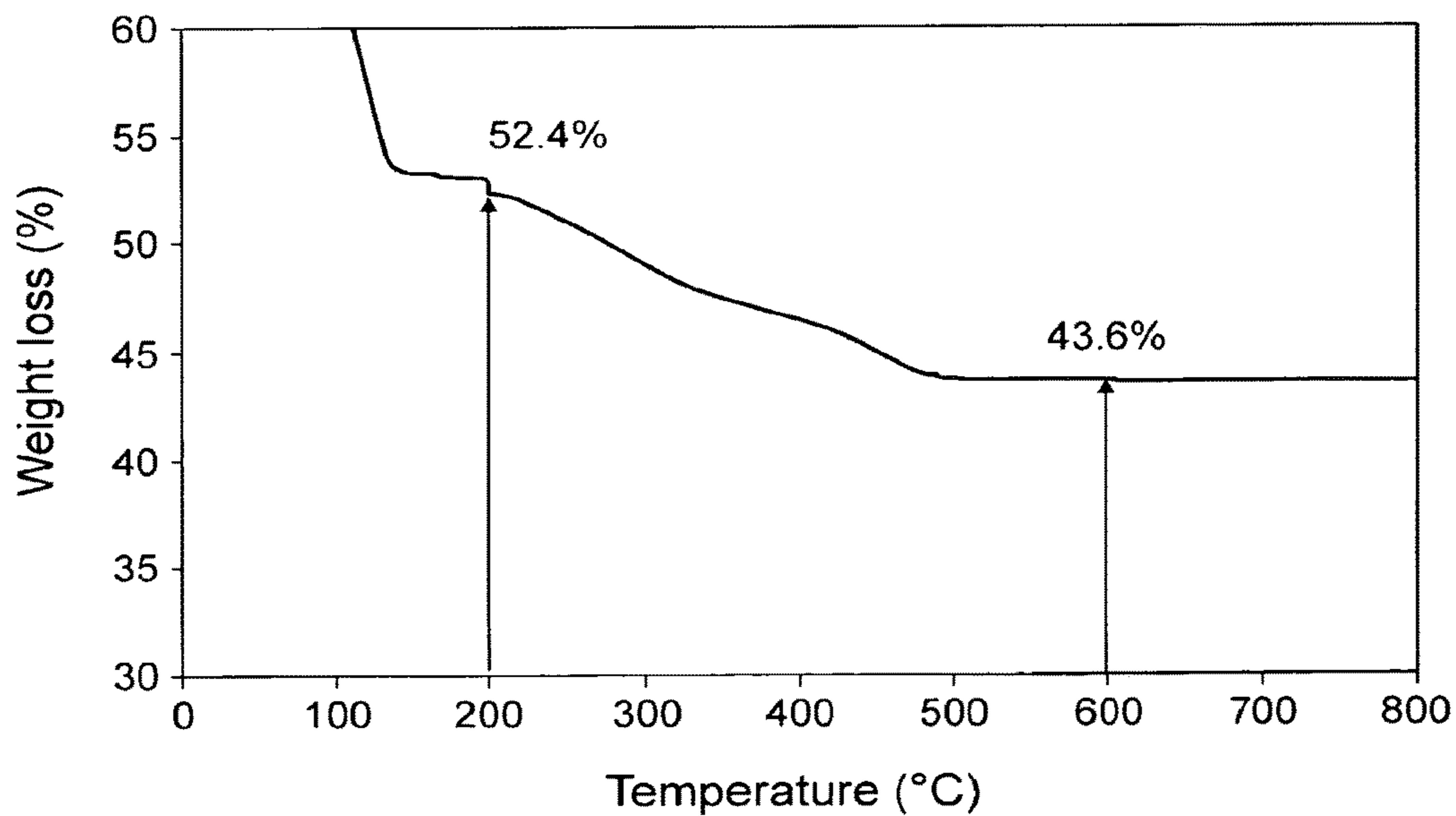
FIG. 24
