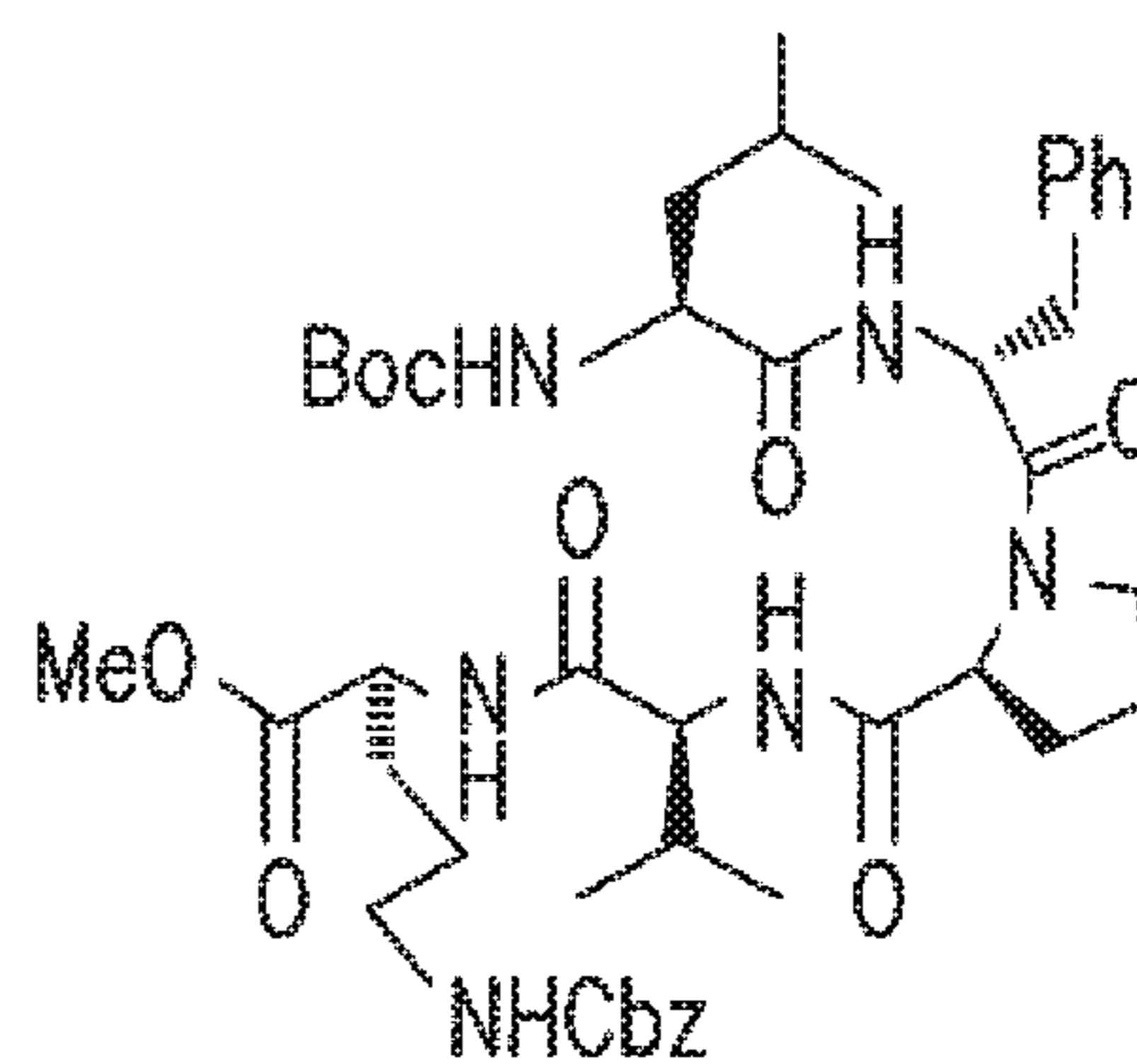
XJB-2-70
