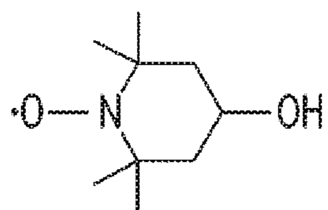
TEMPOL
