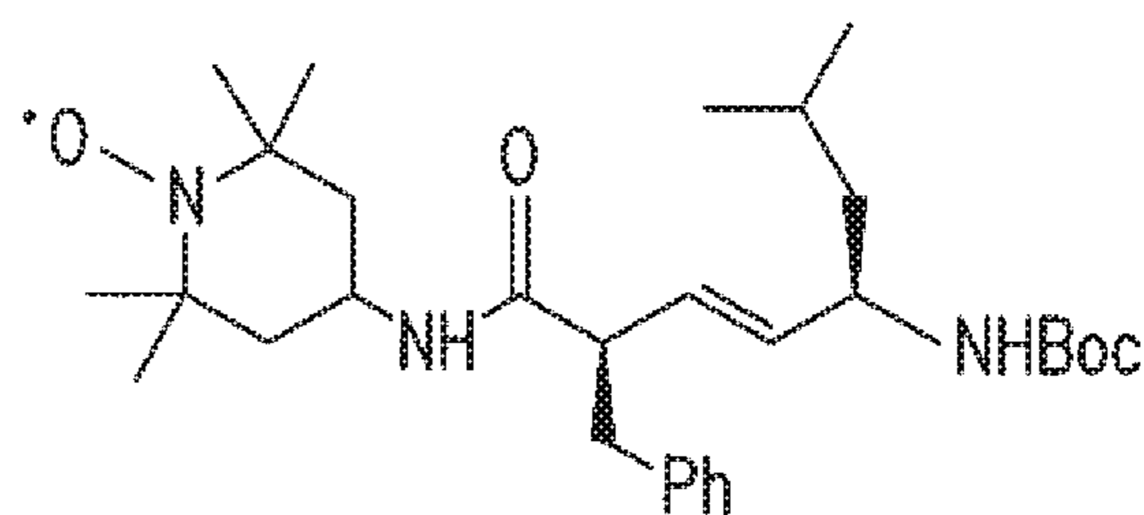
XJB-5-208
