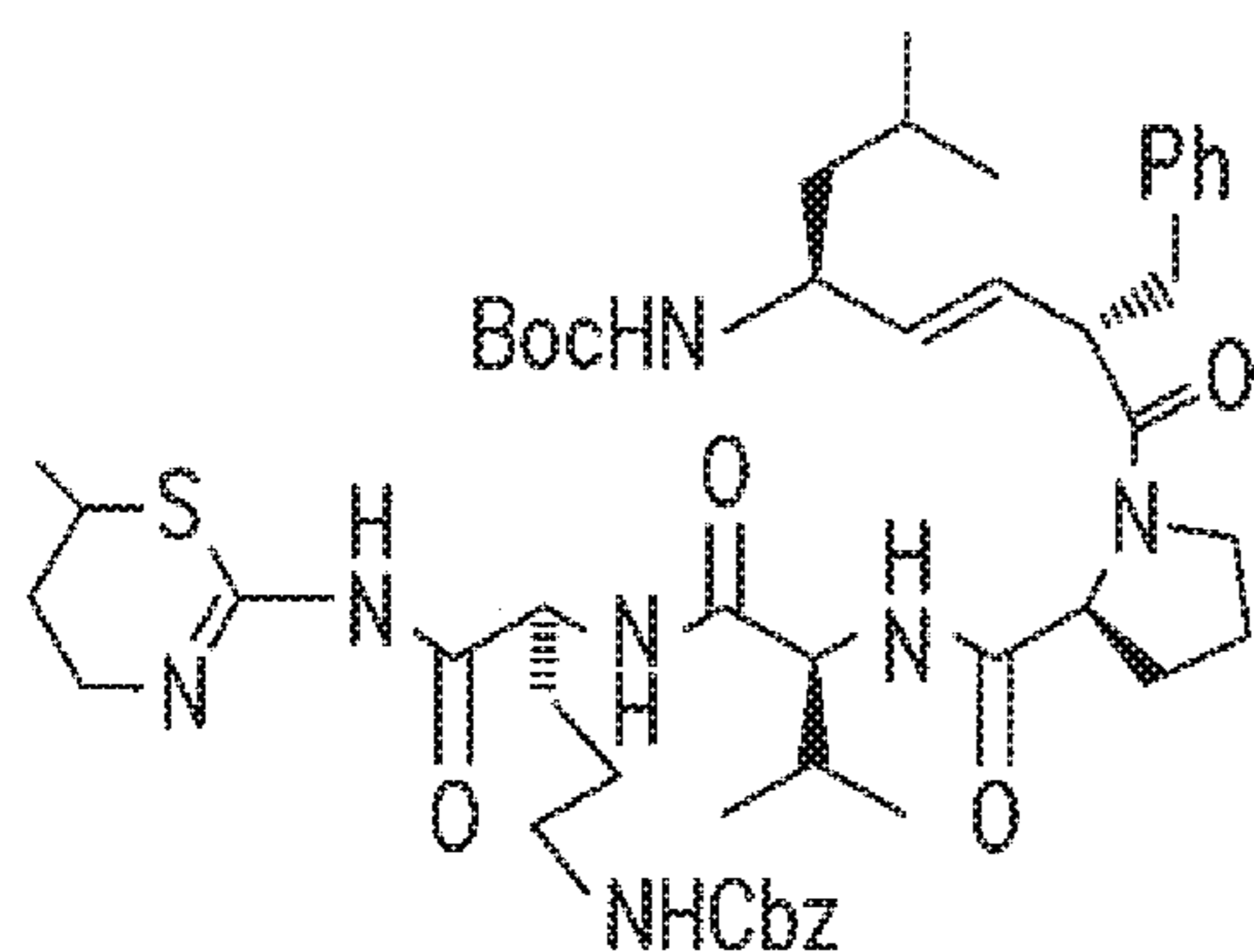
XJB-5-133
