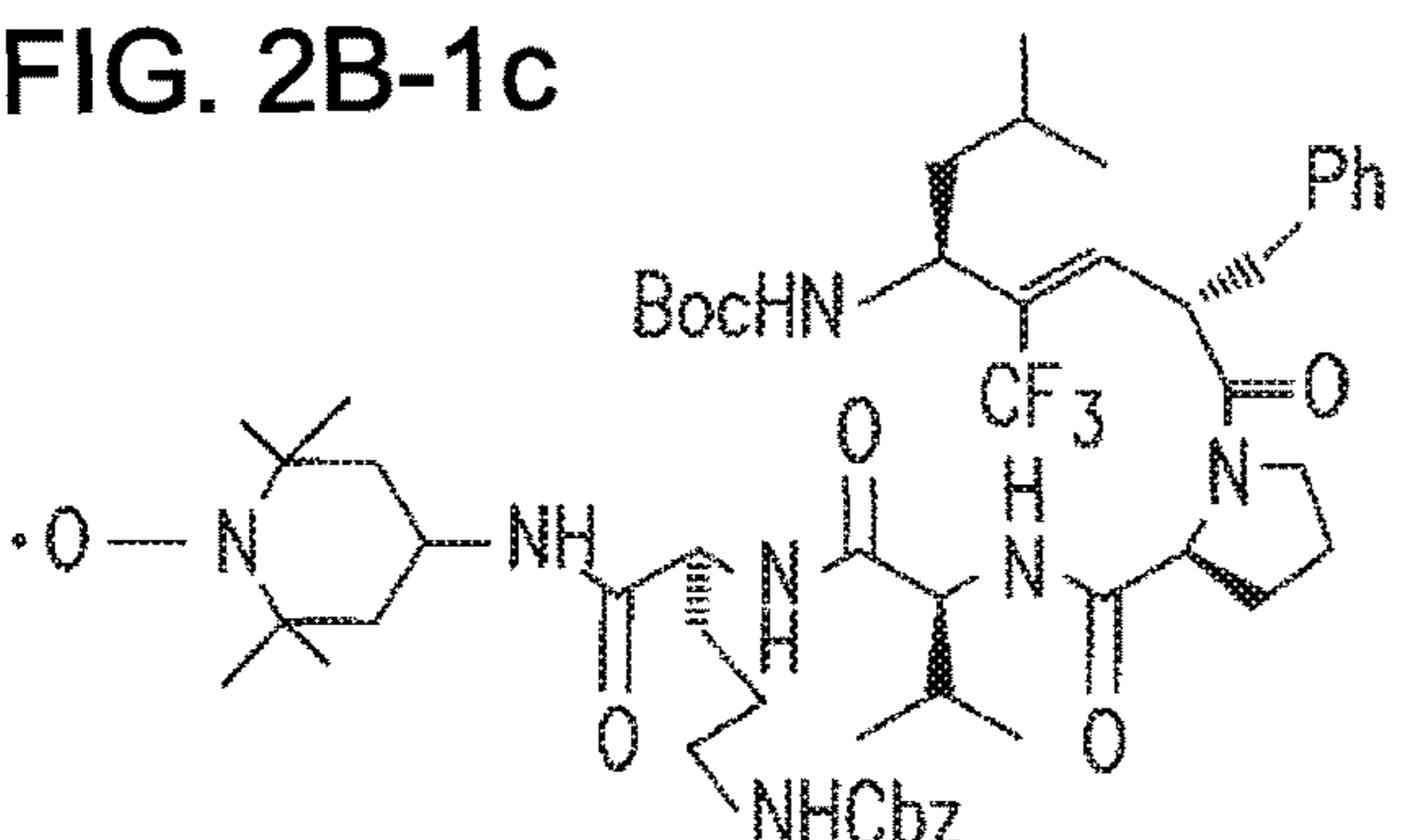
XJB-7-55
