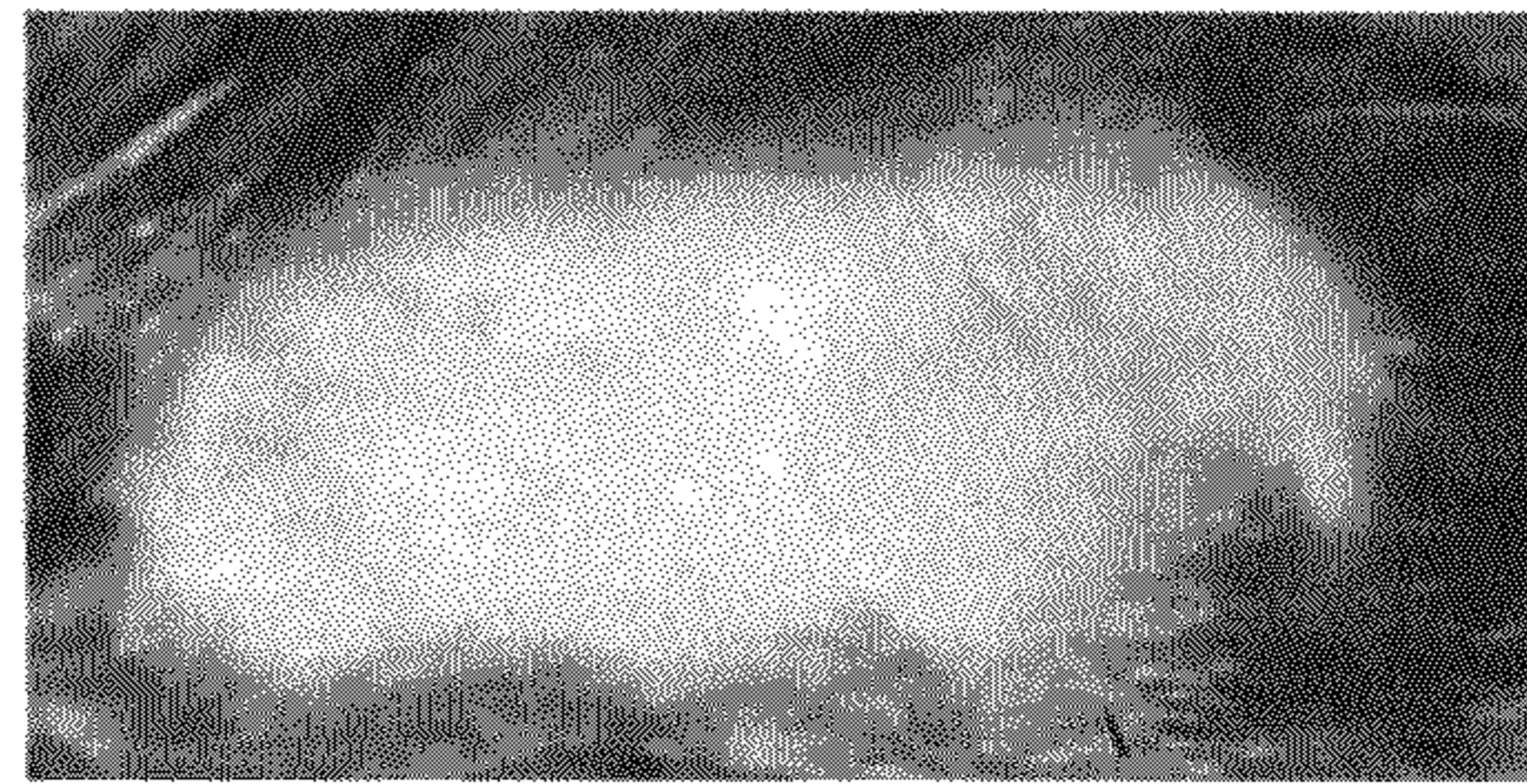
XJB-5-131
