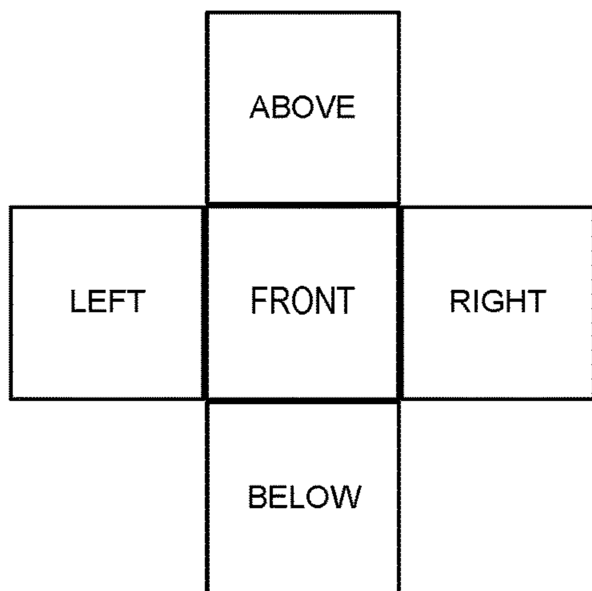
CUBEMAP
