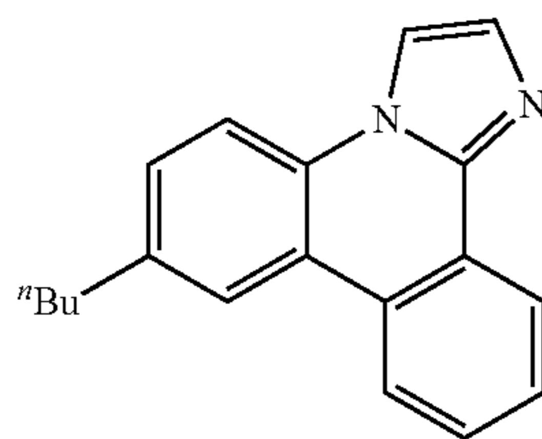
es15 ligand
