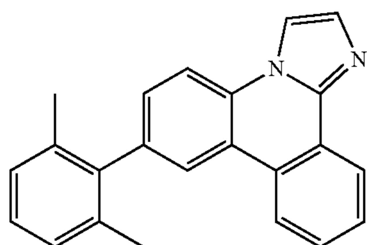
es13 ligand
