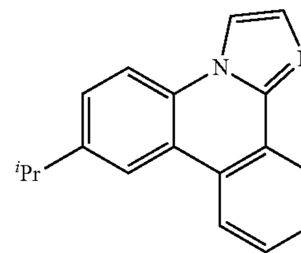
es6 ligand
