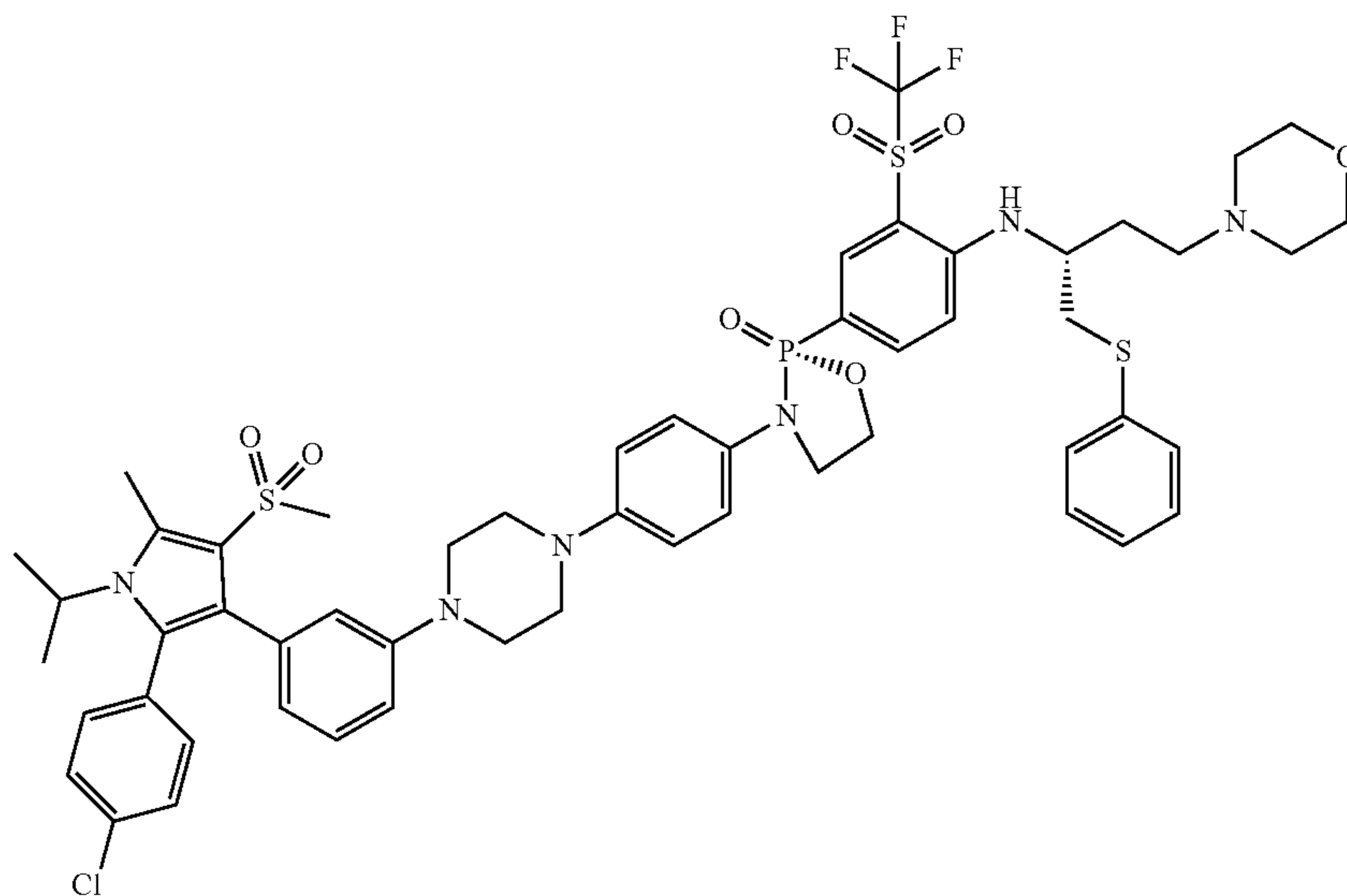
(R)-3-(4-(4-(3-(2-(4-chlorophenyl)-1-isopropyl-5-methyl-4-(methylsulfonyl)-1H-pyrrol-3-yl)phenyl)piperazin-1-yl)phenyl)-2-(4-(((R)-4-morpholino-1-(phenylthio)butan-2-yl)amino)-3-((trifluoromethyl)sulfonyl)phenyl)-1,3,2-oxazaphospholidine 2-oxide
