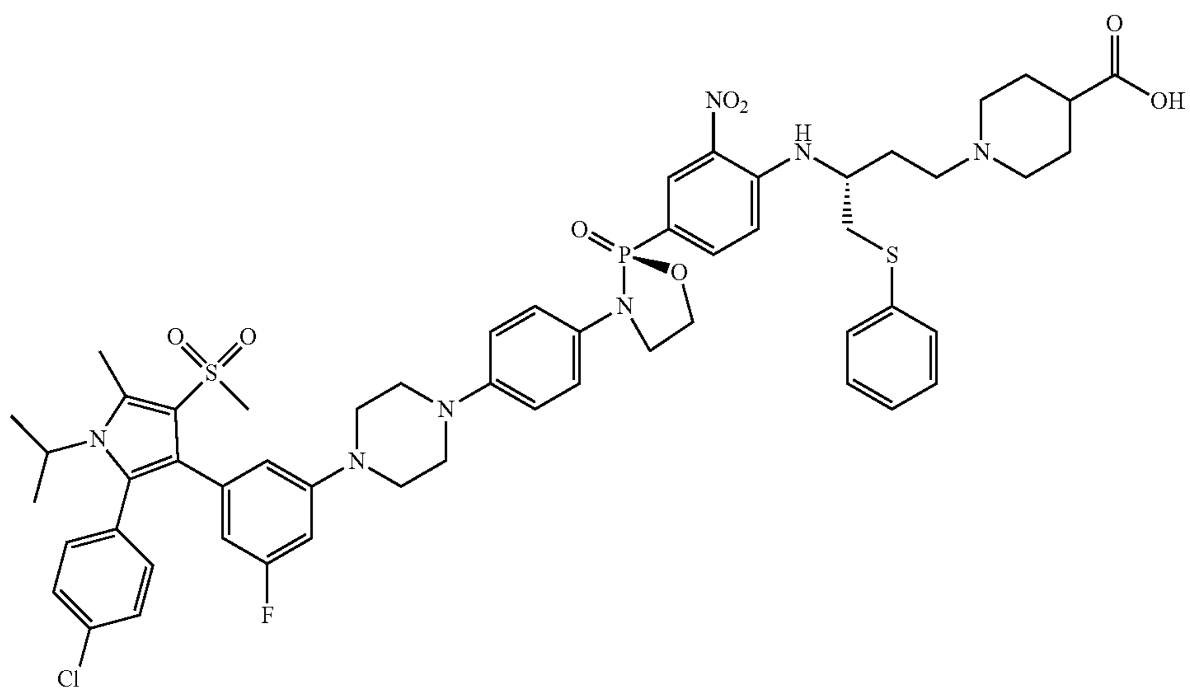
1-((S)-3-((4-((S)-3-(4-(4-(3-(2-(4-chlorophenyl)-1-isopropyl-5-methyl-4-(methylsulfonyl)-1H-pyrrol-3-yl)-5-fluorophenyl)piperazin-1-yl)phenyl)-2-oxido-1,3,2-oxazaphospholidin-2-yl)-2-nitrophenyl)amino)-4-(phenylthio)butyl)piperidine-4-carboxylic acid
