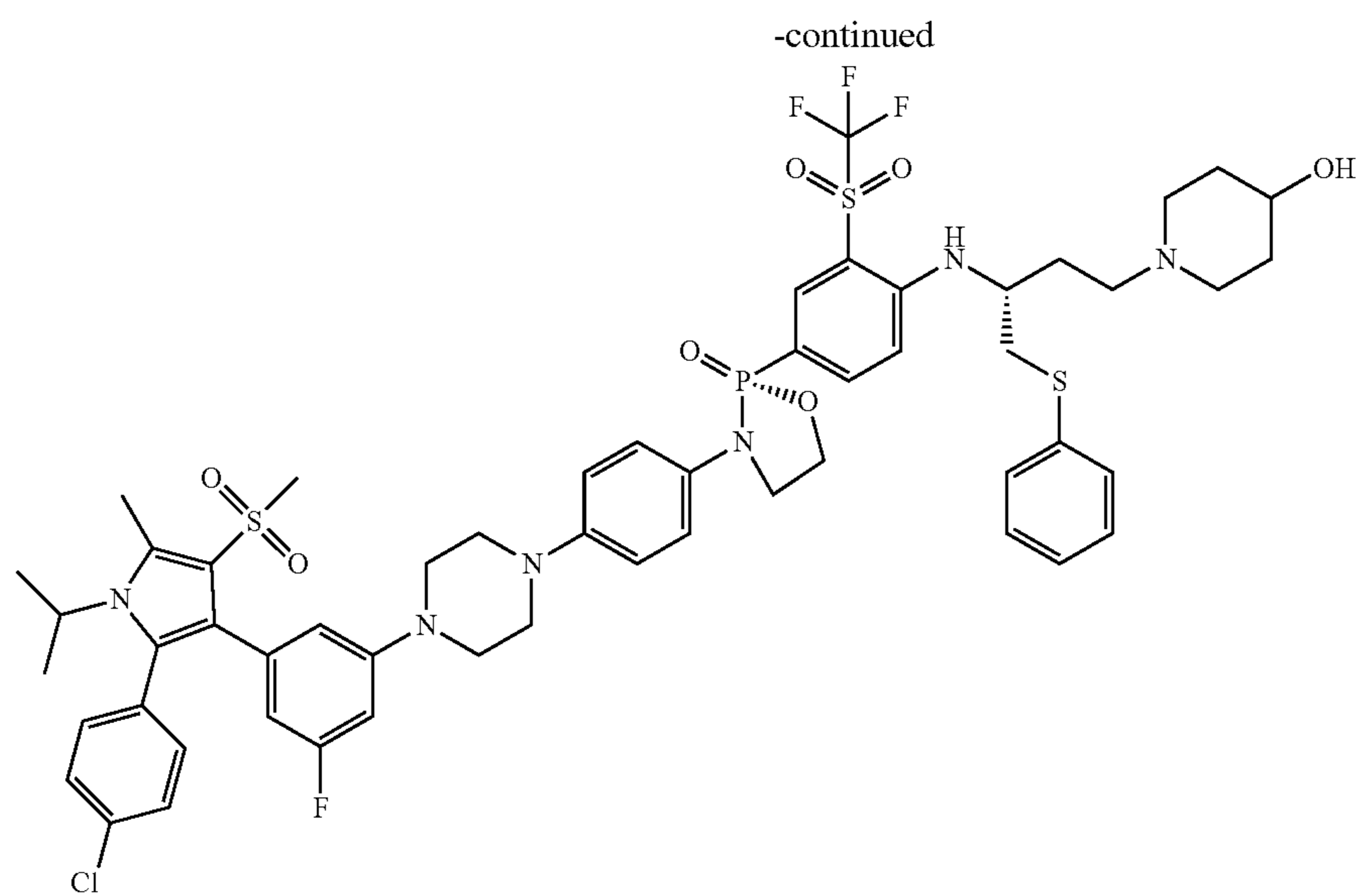
(R)-3-(4-(4-(3-(2-(4-chlorophenyl)-1-isopropyl-5-methyl-4-(methylsulfonyl)-1H-pyrrol-3-yl)-5-fluorophenyl)piperazin-1-yl)phenyl)-2-(4-(((R)-4-(4-hydroxypiperidin-1-yl)-1-(phenylthio)butan-2-yl)amino)-3-((trifluoromethyl)sulfonyl)phenyl)-1,3,2-oxazaphospholidine 2-oxide
