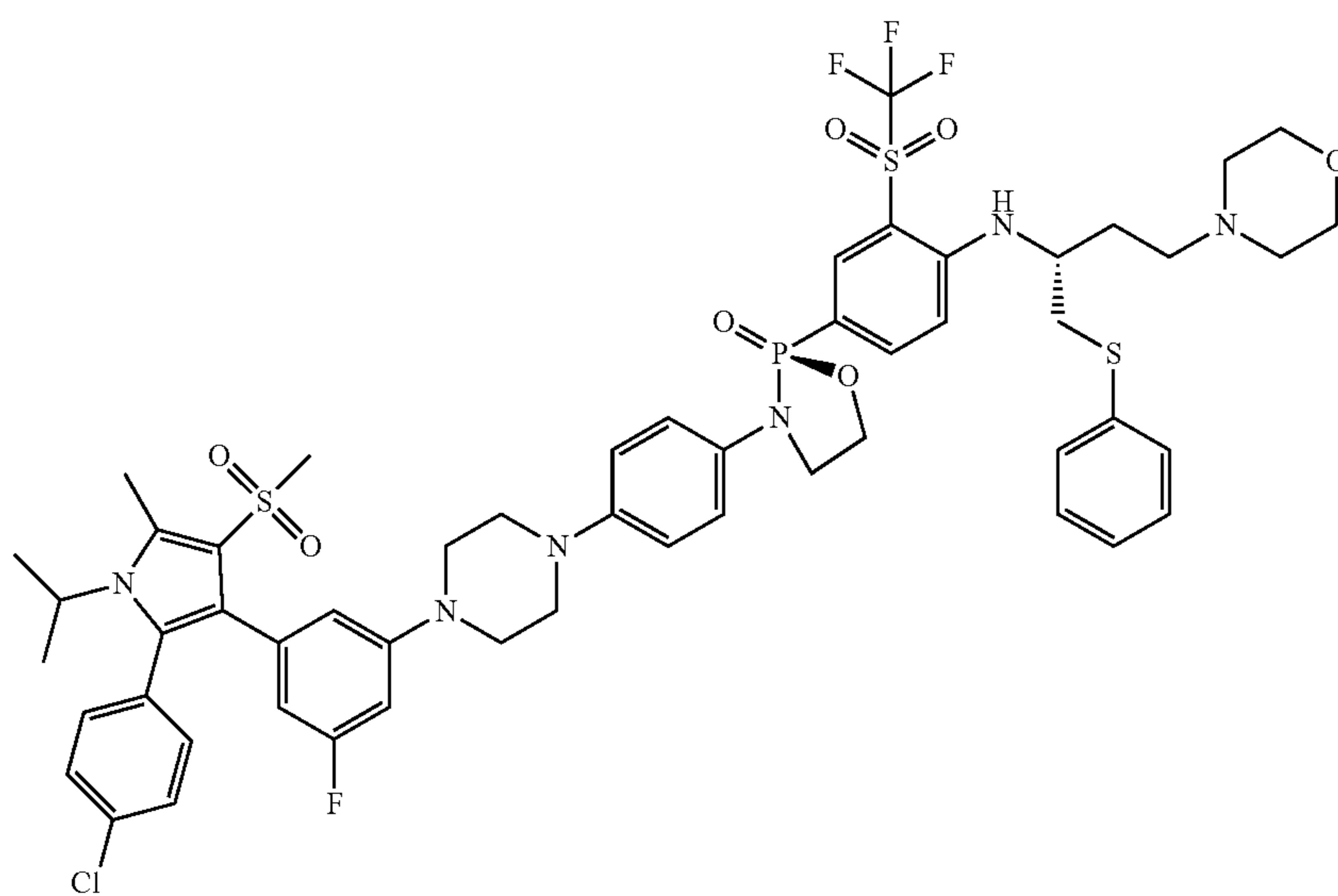
(S)-3-(4-(4-(3-(2-(4-chlorophenyl)-1-isopropyl-5-methyl-4-(methylsulfonyl)-1H-pyrrol-3-yl)-5-fluorophenyl)piperazin-1-yl)phenyl)-2-(4-(((R)-4-morpholino-1-(phenylthio)butan-2-yl)amino)-3-(trifluoromethyl)sulfonyl)phenyl)-1,3,2-oxazaphospholidine 2-oxide
