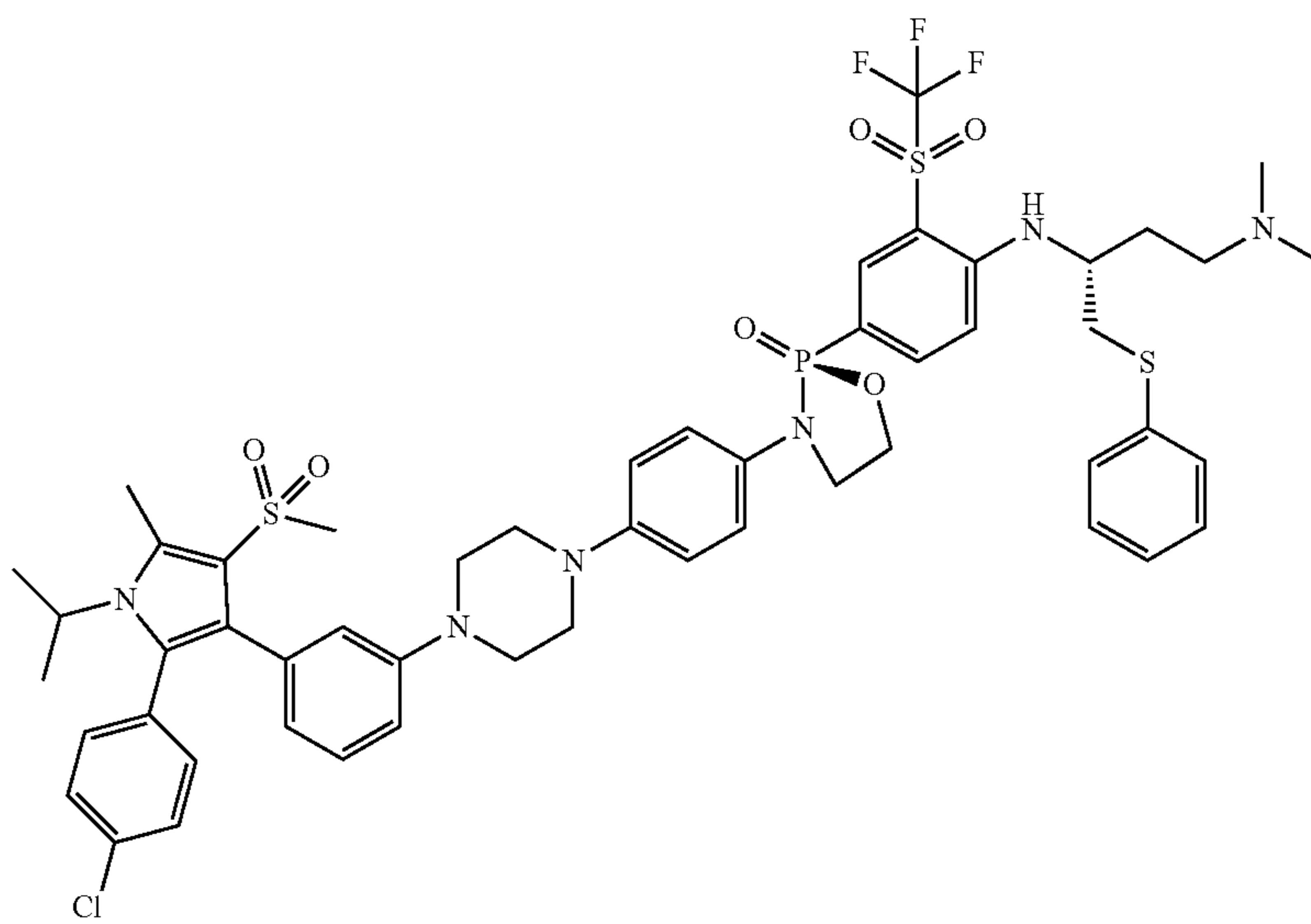
(S)-3-(4-(4-(3-(2-(4-chlorophenyl)-1-isopropyl-5-methyl-4-(methylsulfonyl)-1H-pyrrol-3-yl)phenyl)piperazin-1-yl)phenyl)-2-(4-(((R)-4-(dimethylamino)-1-(phenylthio)butan-2-yl)amino)-3-((trifluoromethyl)sulfonyl)phenyl)-1,3,2-oxazaphospholidine 2-oxide
