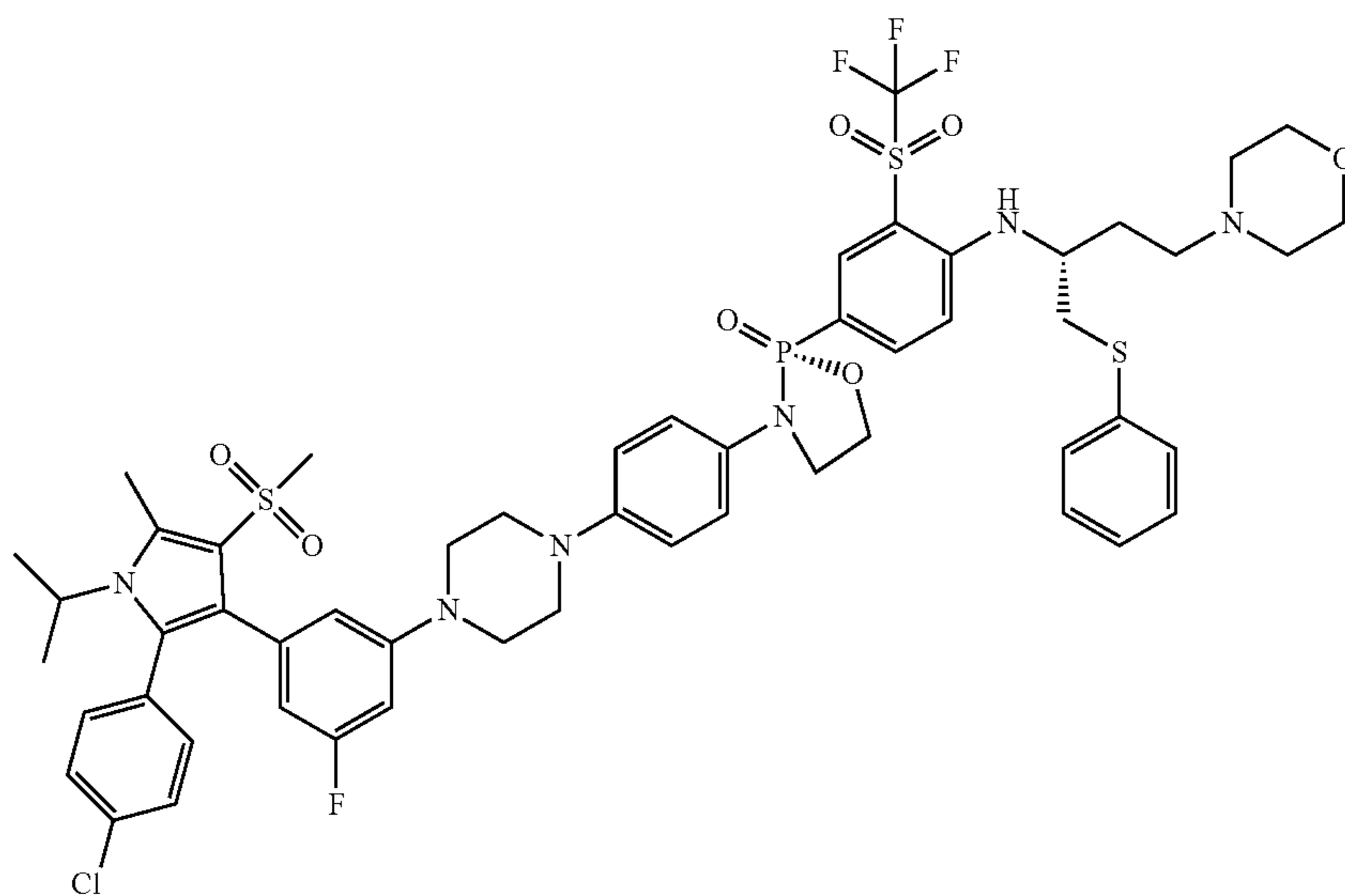
(R)-3-(4-(4-(3-(2-(4-chlorophenyl)-1-isopropyl-5-methyl-4-(methylsulfonyl)-1H-pyrrol-3-yl)-5-fluorophenyl)piperazin-1-yl)phenyl)-2-(4-(((R)-4-morpholino-1-(phenylthio)butan-2-yl)amino)-3-(trifluoromethyl)sulfonyl)phenyl)-1,3,2-oxazaphospholidine 2-oxide
