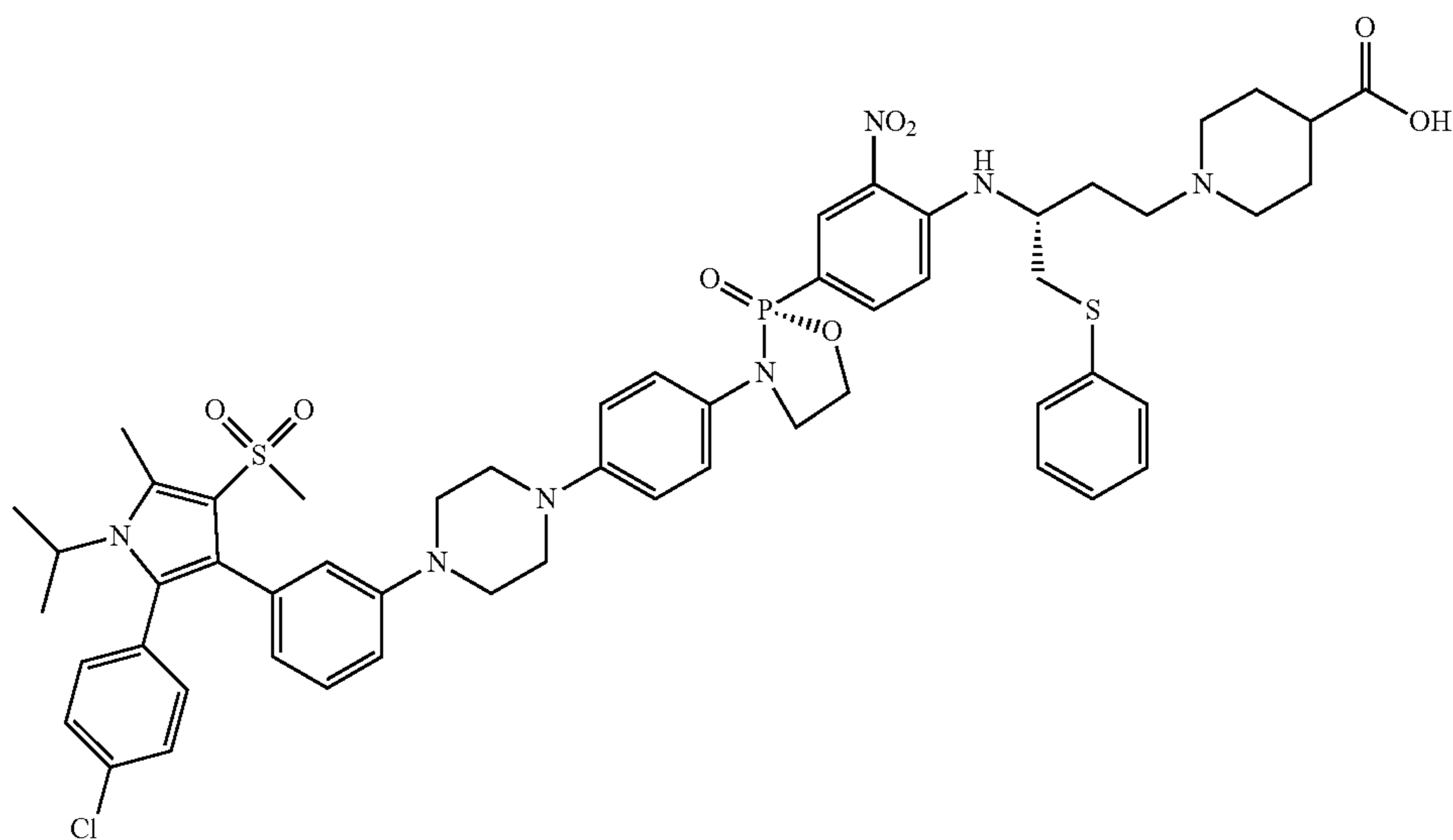
1-((R)-3-((4-((R)-3-(4-(4-(3-(2-(4-chlorophenyl)-1-isopropyl-5-methyl-4-(methylsulfonyl)-1H-pyrrol-3-yl)phenyl)piperazin-1-yl)phenyl)-2-oxido-1,3,2-oxazaphospholidin-2-yl)-2-nitrophenyl)amino)-4-(phenylthio)butyl)piperidine-4-carboxylic acid
