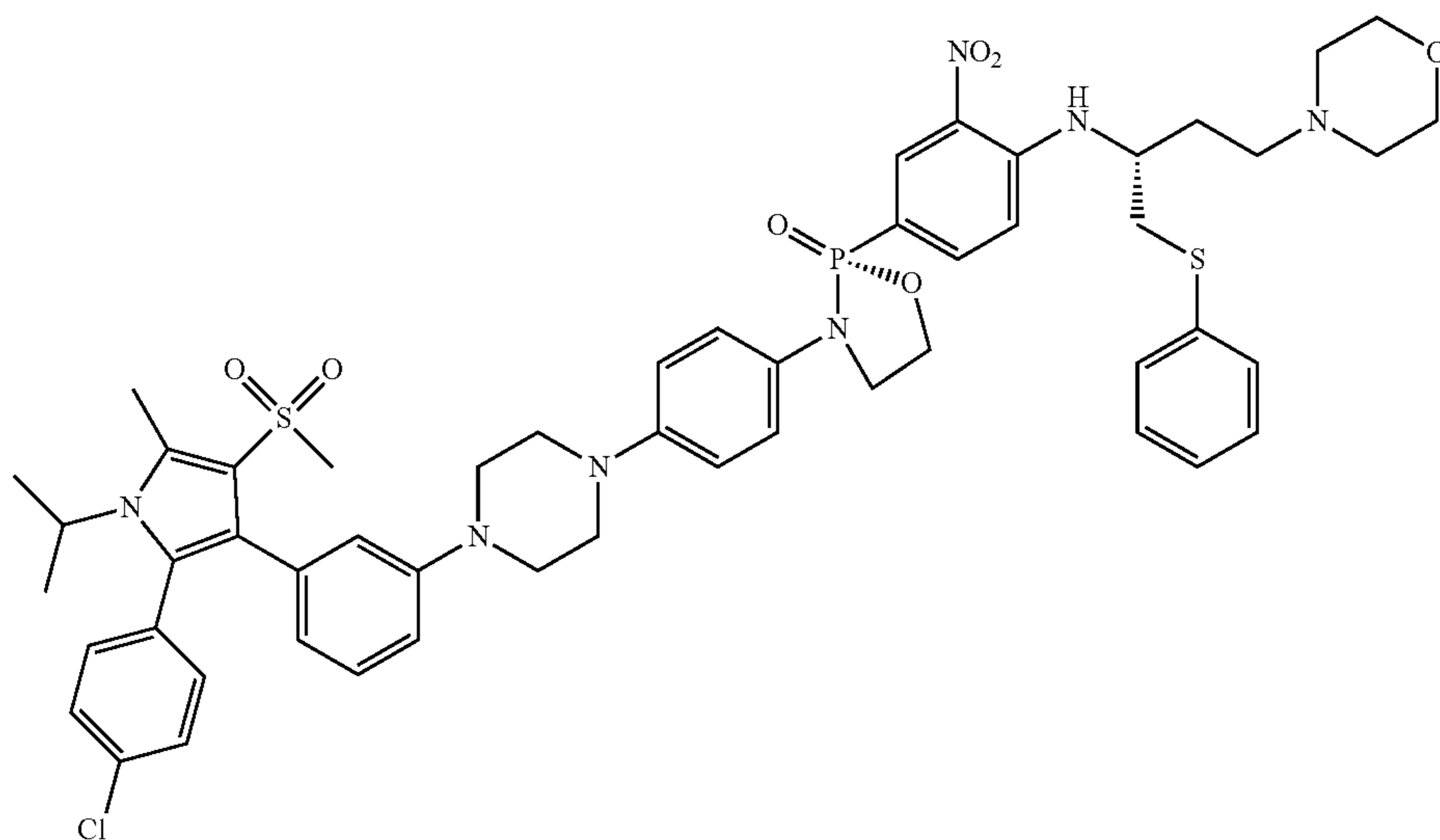
(R)-3-(4-(4-(3-(2-(4-chlorophenyl)-1-isopropyl-5-methyl-4-(methylsulfonyl)-1H-pyrrol-3-yl)phenyl)piperazin-1-yl)phenyl)-2-(4-(((R)-4-morpholino-1-(phenylthio)butan-2-yl)amino)-3-nitrophenyl)-1,3,2-oxazaphospholidine 2-oxide
