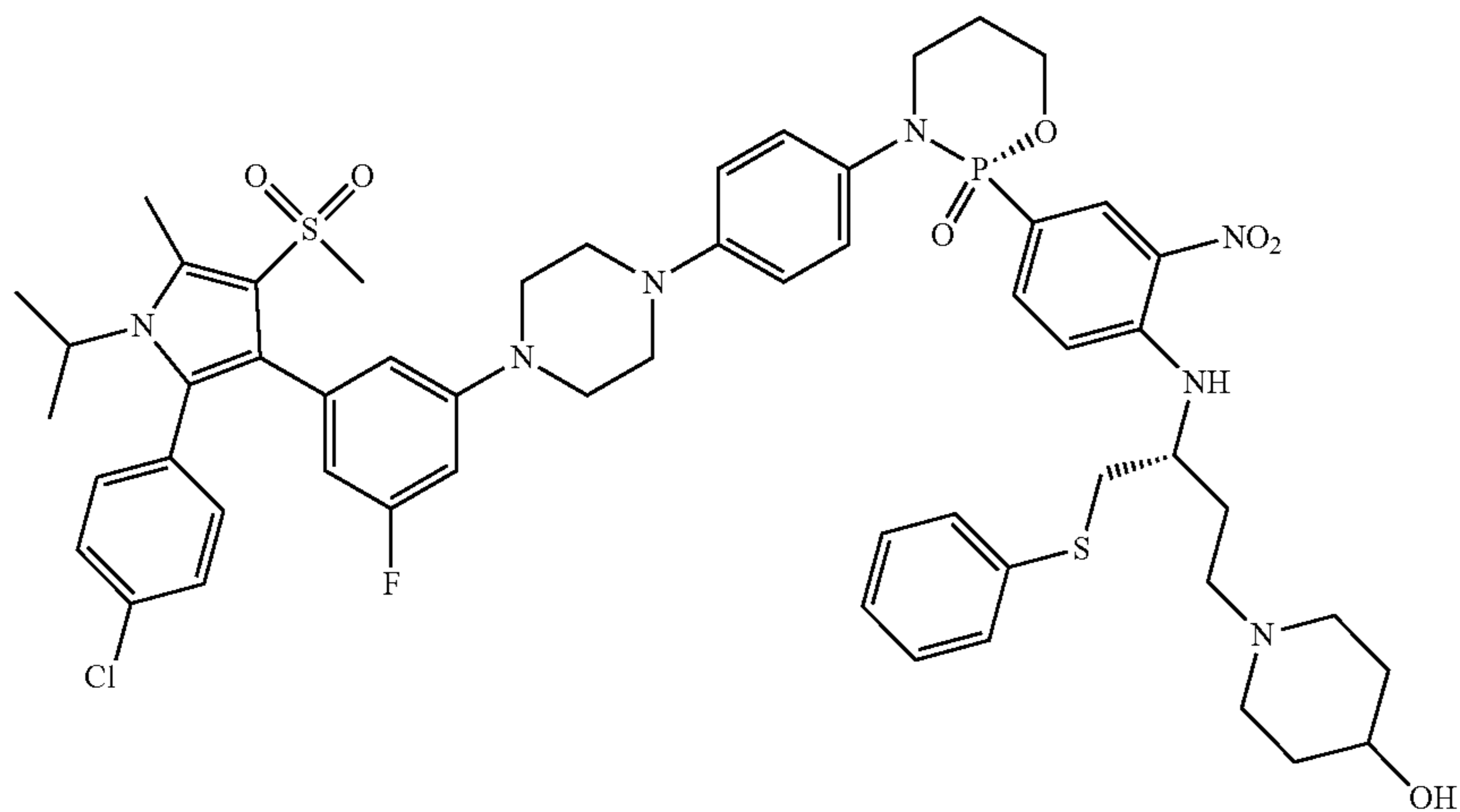
(S)-3-(4-(4-(3-(2-(4-chlorophenyl)-1-isopropyl-5-methyl-4-(methylsulfonyl)-1H-pyrrol-3-yl)-5-fluorophenyl)piperazin-1-yl)phenyl)-2-(4-(((R)-4-(4-hydroxypiperidin-1-yl)-1-(phenylthio)butan-2-yl)amino)-3-nitrophenyl)-1,3,2-oxazaphosphinane 2-oxide
