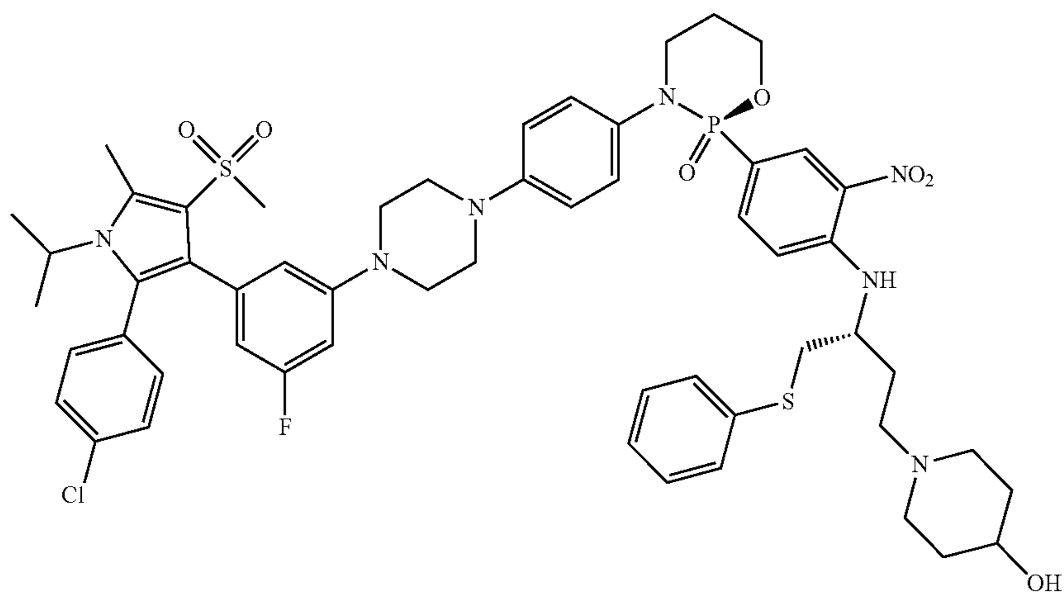
(R)-3-(4-(4-(3-(2-(4-chlorophenyl)-1-isopropyl-5-methyl-4-(methylsulfonyl)-1H-pyrrol-3-yl)-5-fluorophenyl)piperazin-1-yl)phenyl)-2-(4-(((R)-4-(4-hydroxypiperidin-1-yl)-1-(phenylthio)butan-2-yl)amino)-3-nitrophenyl)-1,3,2-oxazaphosphinane 2-oxide
