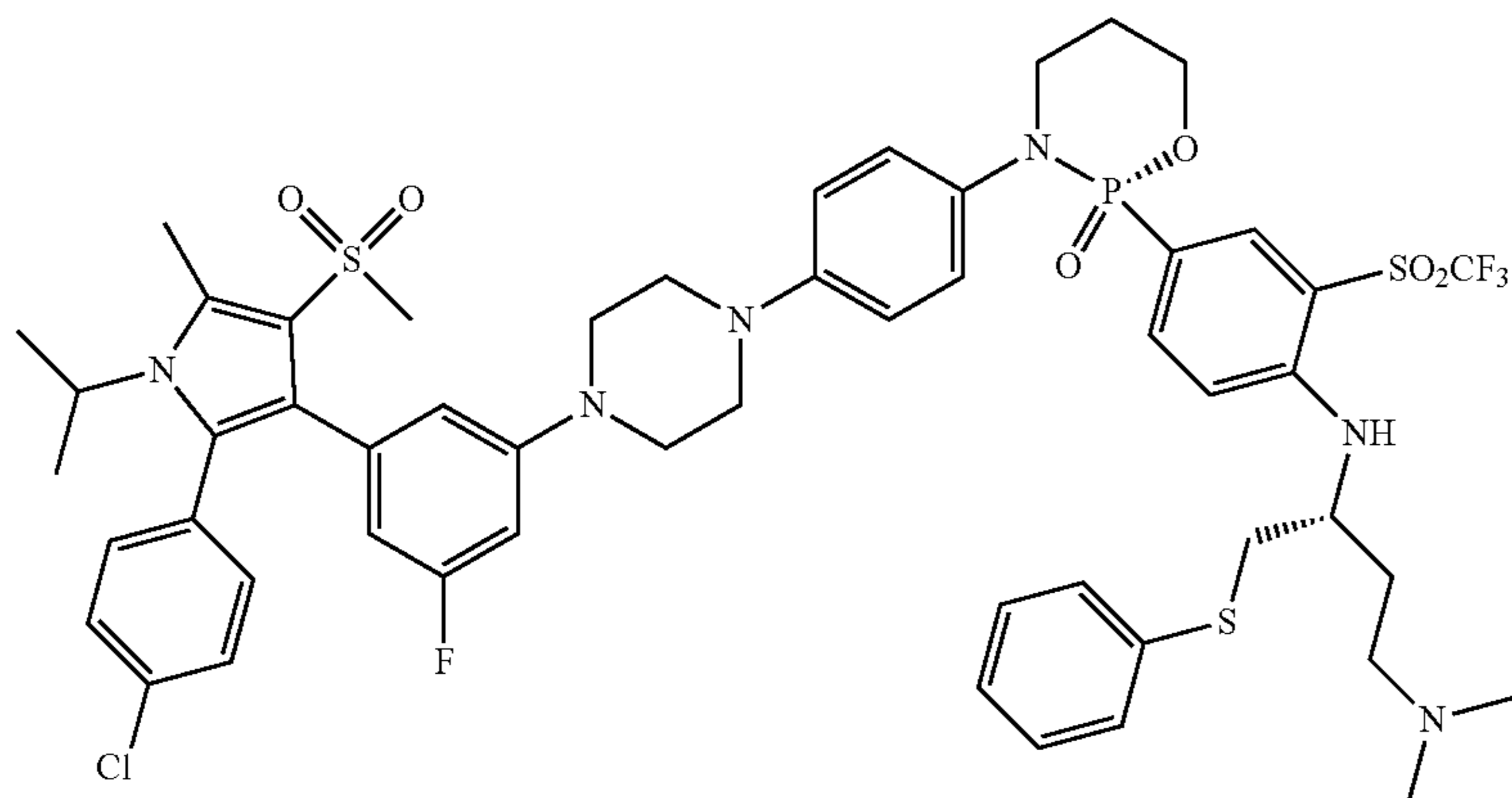
(S)-3-(4-(4-(3-(2-(4-chlorophenyl)-1-isopropyl-5-methyl-4-(methylsulfonyl)-1H-pyrrol-3-yl)-5-fluorophenyl)piperazin-1-yl)phenyl)-2-(4-(((R)-4-(dimethylamino)-1-(phenylthio)butan-2-yl)amino)-3-((trifluoromethyl)sulfonyl)phenyl)-1,3,2-oxazaphosphinane 2-oxide
