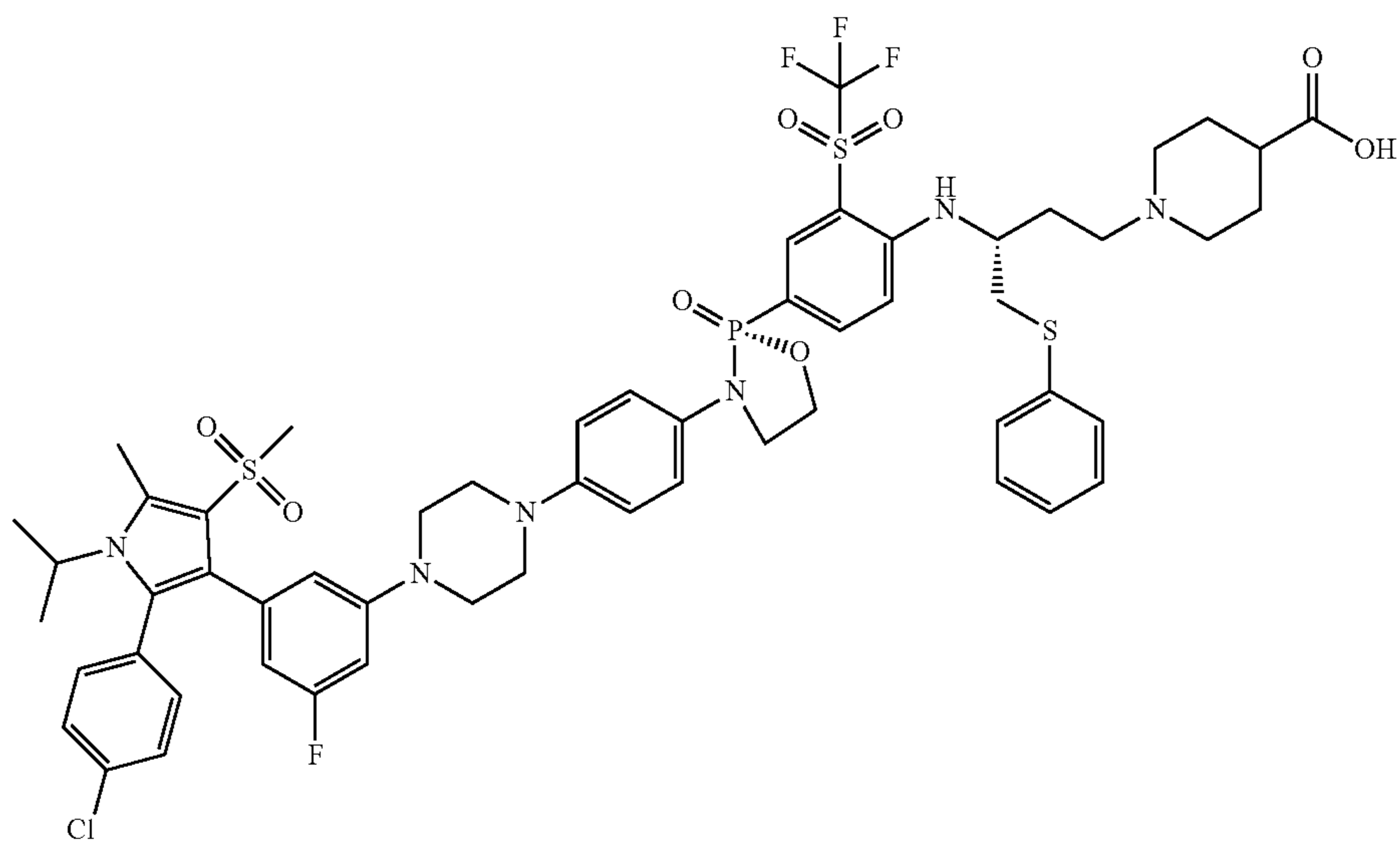
1-((R)-3-((4-((R)-3-(4-(4-(3-(2-(4-chlorophenyl)-1-isopropyl-5-methyl-4-(methylsulfonyl)-1H-pyrrol-3-yl)-5-fluorophenyl)piperazin-1-yl)phenyl)-2-oxido-1,3,2-oxazaphospholidin-2-yl)-2-(trifluoromethyl)sulfonyl)phenyl)amino)-4-(phenylthio)butyl)piperidine-4-carboxylic acid
