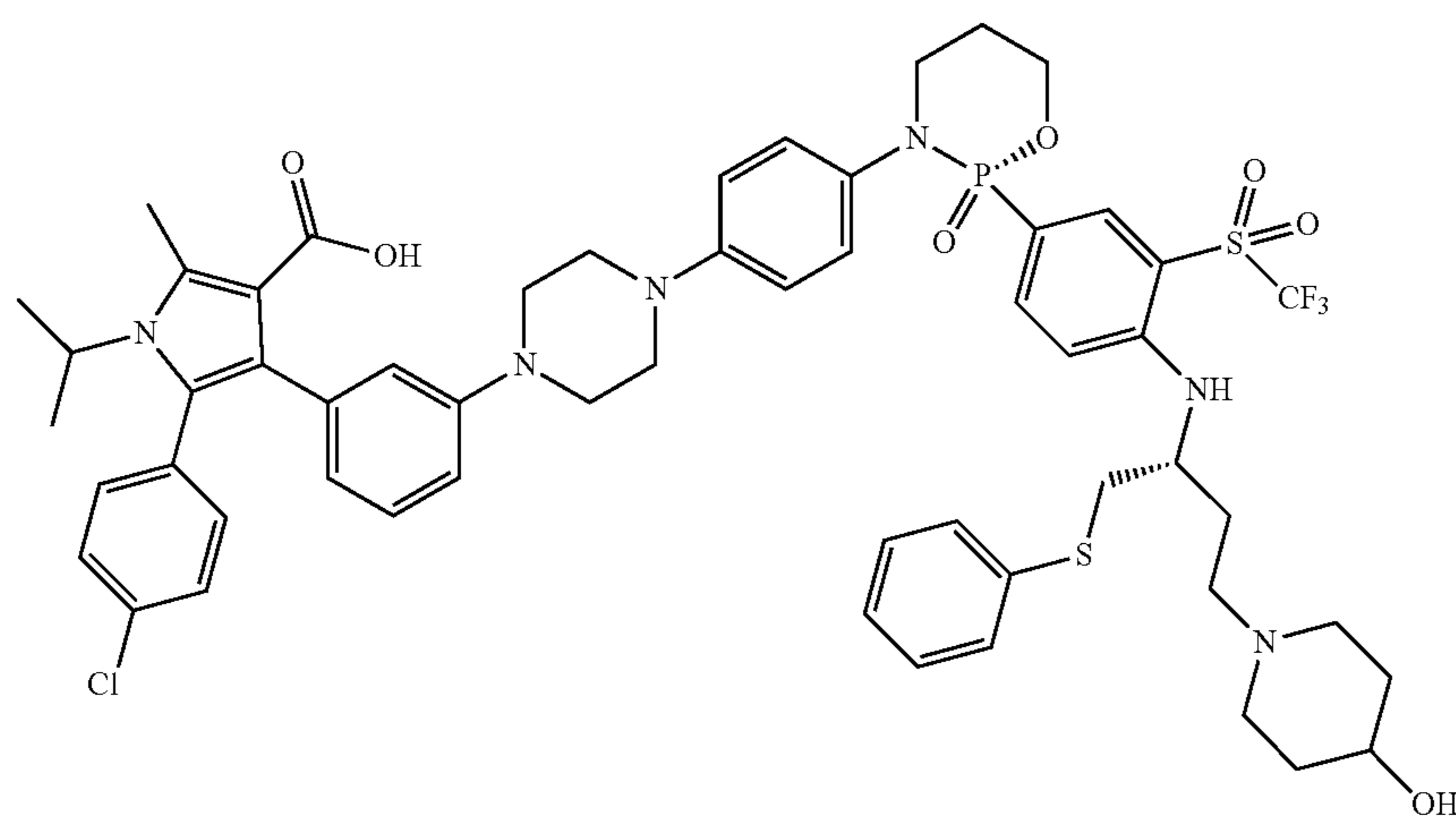
5-(4-chlorophenyl)-4-(3-(4-(4-((S)-2-4-(((R)-4-(4-hydroxypiperidin-1-yl)-1-(phenylthio)butan-2-yl)amino)-3-((trifluoromethyl)sulfonyl)phenyl)-2-oxido-1,3,2-oxazaphosphinan-3-yl)phenyl)piperazin-1-yl)phenyl)-1-isopropyl-2-methyl-1H-pyrrole-3-carboxylic acid
