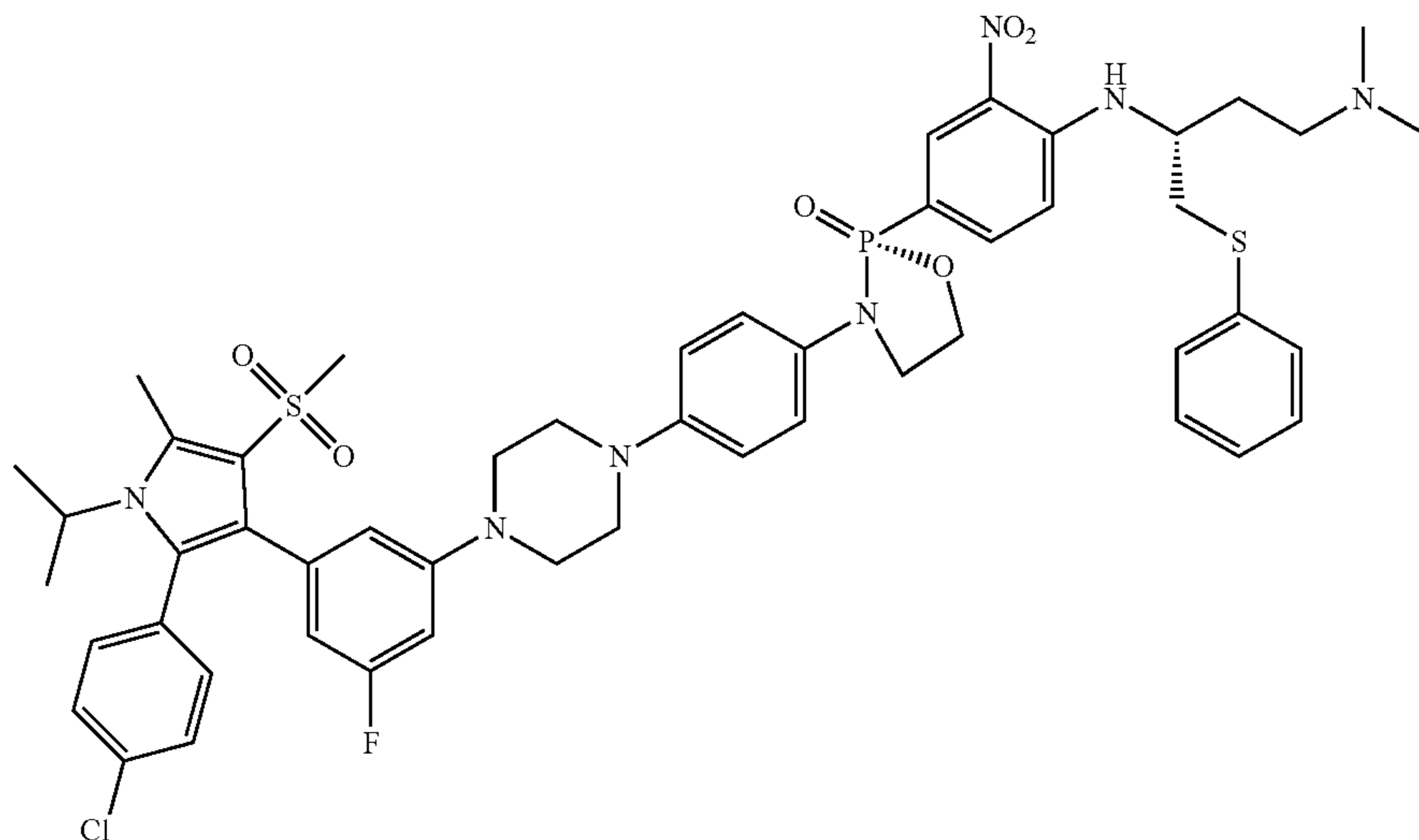
(R)-3-(4-(4-(3-(2-(4-chlorophenyl)-1-isopropyl-5-methyl-4-(methylsulfonyl)-1H-pyrrol-3-yl)-5-fluorophenyl)piperazin-1-yl)phenyl)-2-(4-(((R)-4-(dimethylamino)-1-(phenylthio)butan-2-yl)amino))-3-nitrophenyl)-1,3,2-oxazaphospholidine 2-oxide
