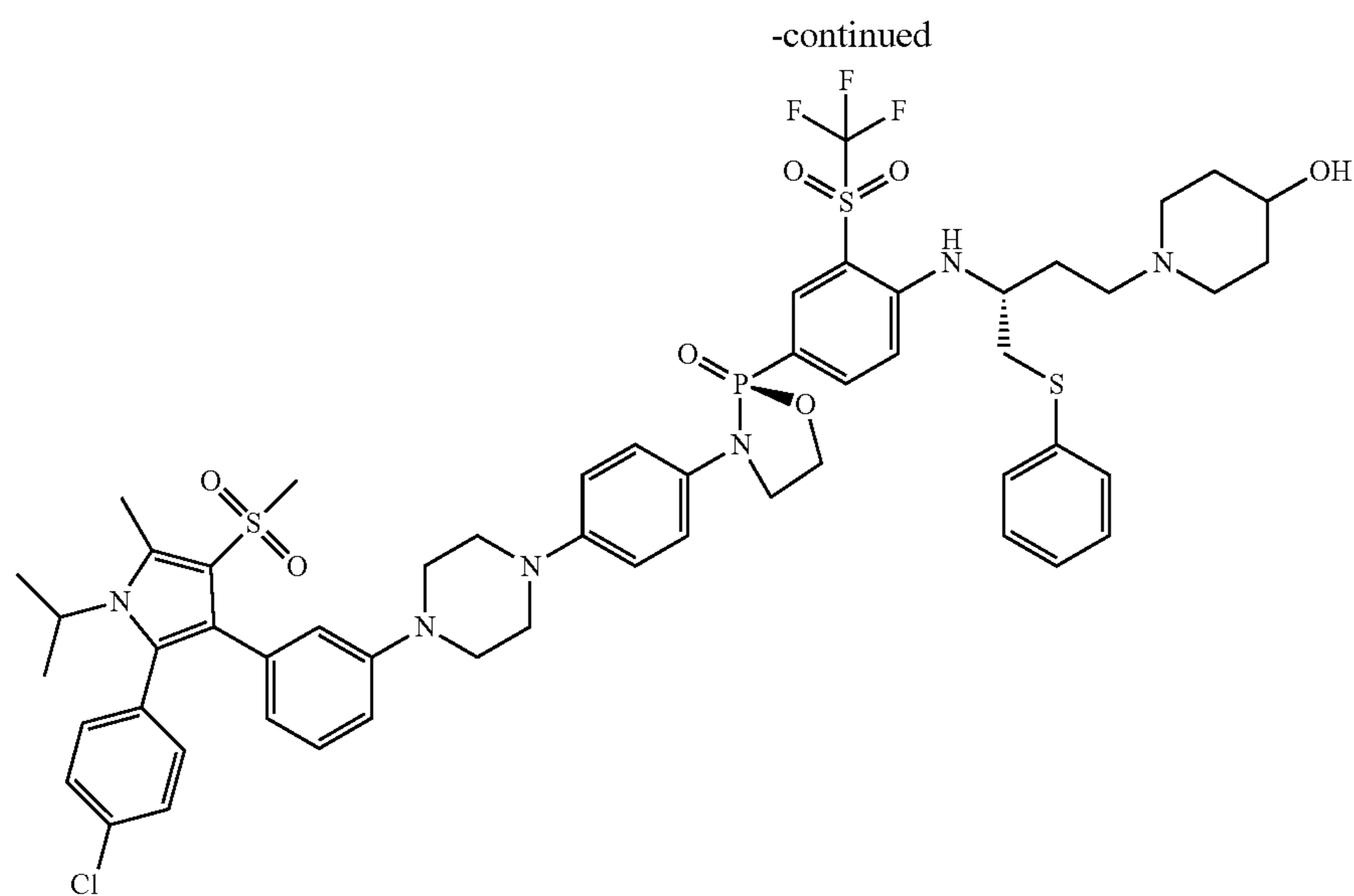
(S)-3-(4-(4-(3-(2-(4-chlorophenyl)-1-isopropyl-5-methyl-4-(methylsulfonyl)-1H-pyrrol-3-yl)phenyl)piperazin-1-yl)phenyl)-2-(4-((R)-4-(4-hydroxypiperidin-1-yl)-1-(phenylthio)butan-2-yl)amino)-3-(trifluoromethyl)sulfonyl)phenyl)-1,3,2-oxazaphospholidine 2-oxide
