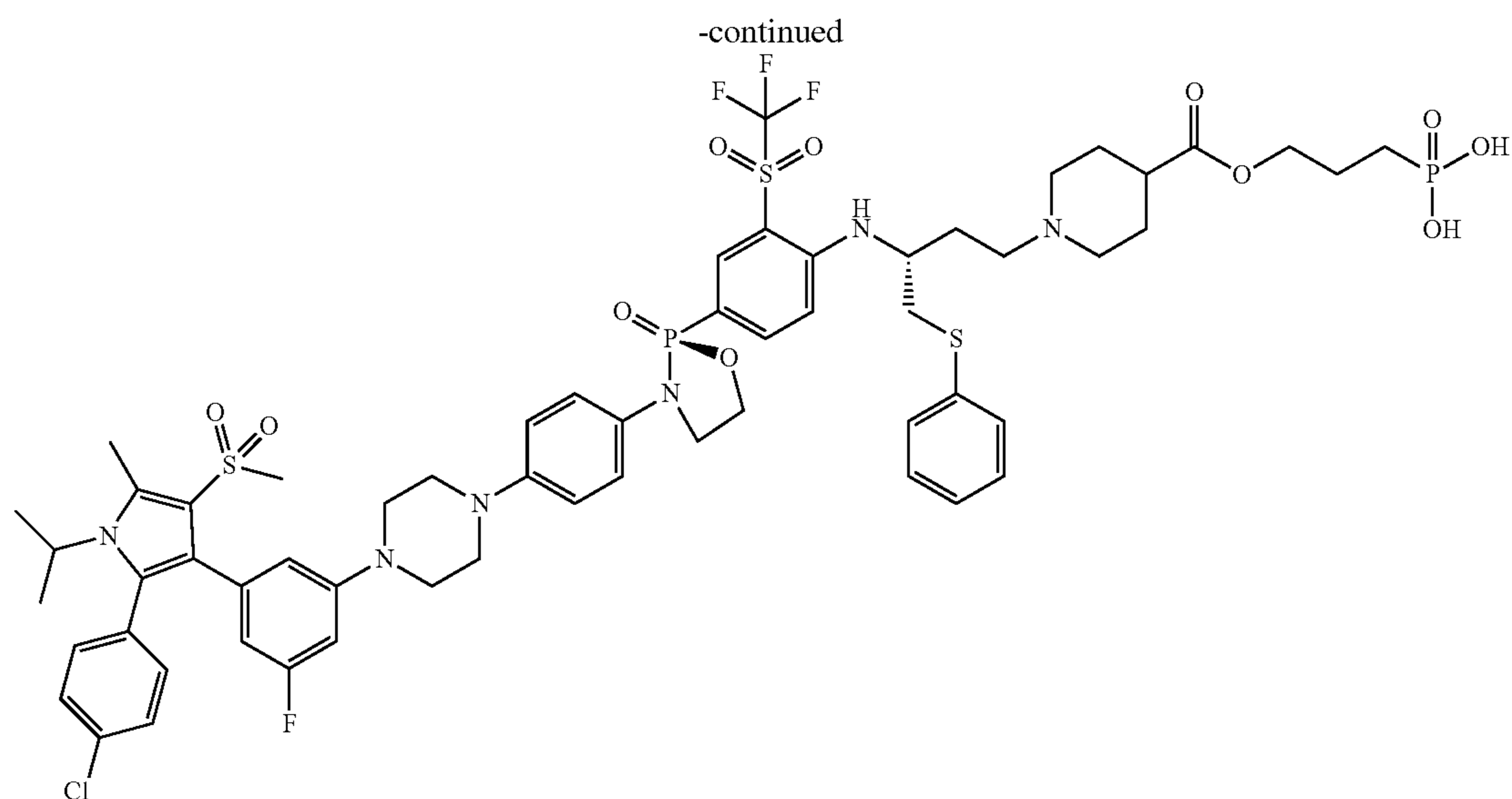
(3-((1-((R)-3-((4-((S)-3-(4-(3-(2-(4-chlorophenyl)-1-isopropyl-5-methyl-4-(methylsulfonyl)-1H-pyrrol-3-yl)-5-fluorophenyl)piperazin-1-yl)phenyl)-2-oxido-1,3,2-oxazaphospholidin-2-yl)-2-(trifluoromethylsulfonyl)phenyl)amino)-4-(phenylthio)butyl)piperidine-4-carbonyloxy)propyl)phosphonic acid
