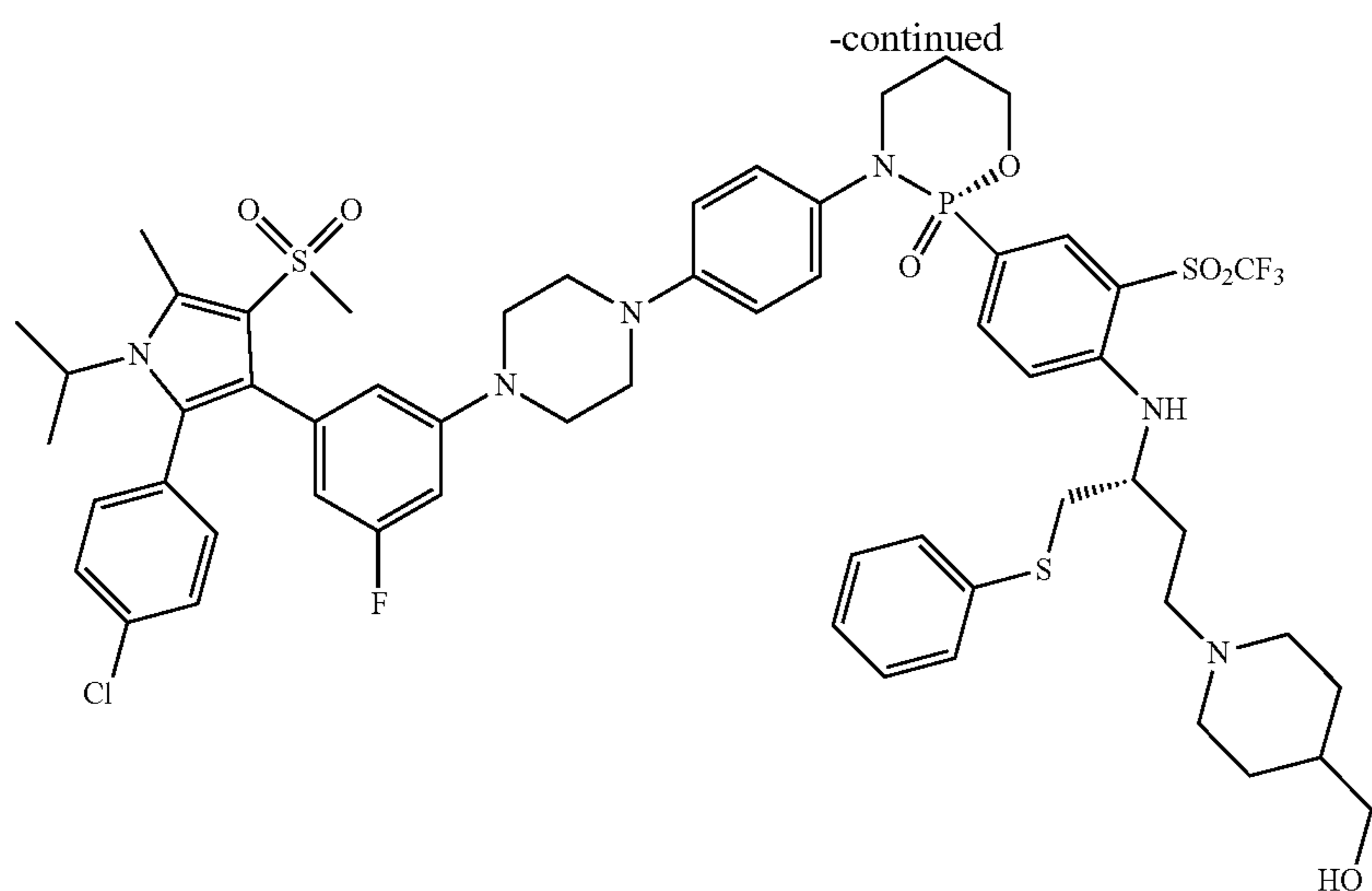
(S)-3-(4-(4-(3-(2-(4-chlorophenyl)-1-isopropyl-5-methyl-4-(methylsulfonyl)-1H-pyrrol-3-yl)-5-fluorophenyl)piperazin-1-yl)phenyl)-2-(4-(((R)-4-(4-hydroxymethyl)piperidin-1-yl)-1-(phenylthio)butan-2-yl)amino)-3-((trifluoromethyl)sulfonyl)phenyl)-1,3,2-oxazaphosphinane 2-oxide
