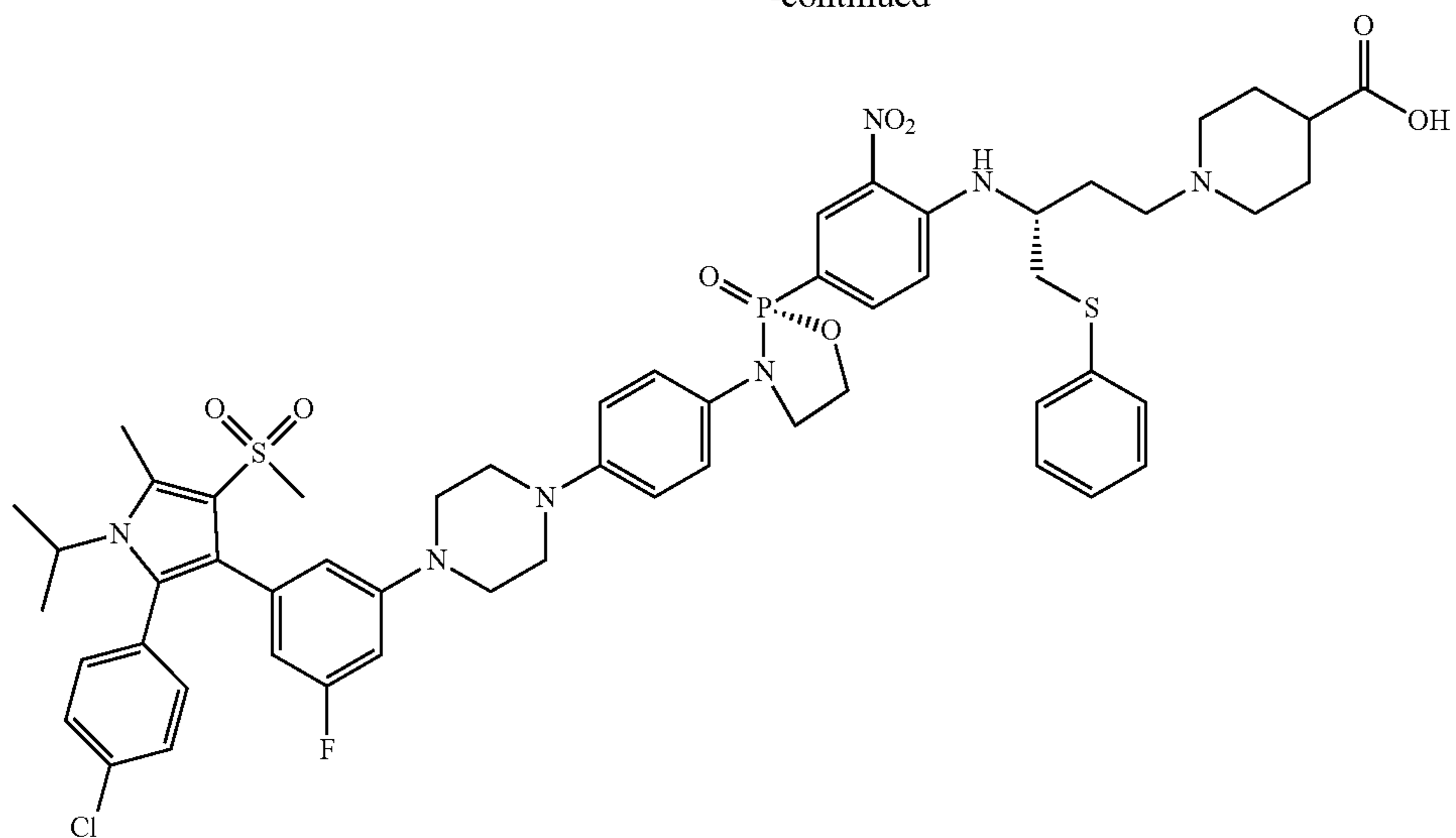
1-((R)-3-((4-((R)-3-(4-(4-(3-(2-(4-chlorophenyl)-1-isopropyl-5-methyl-4-(methylsulfonyl)-1H-pyrrol-3-yl)-5-fluorophenyl)piperazin-1-yl)phenyl)-2-oxido-1,3,2-oxazaphospholidin-2-yl)-2-nitrophenyl)amino)-4-(phenylthio)butyl)piperidine-4-carboxylic acid
