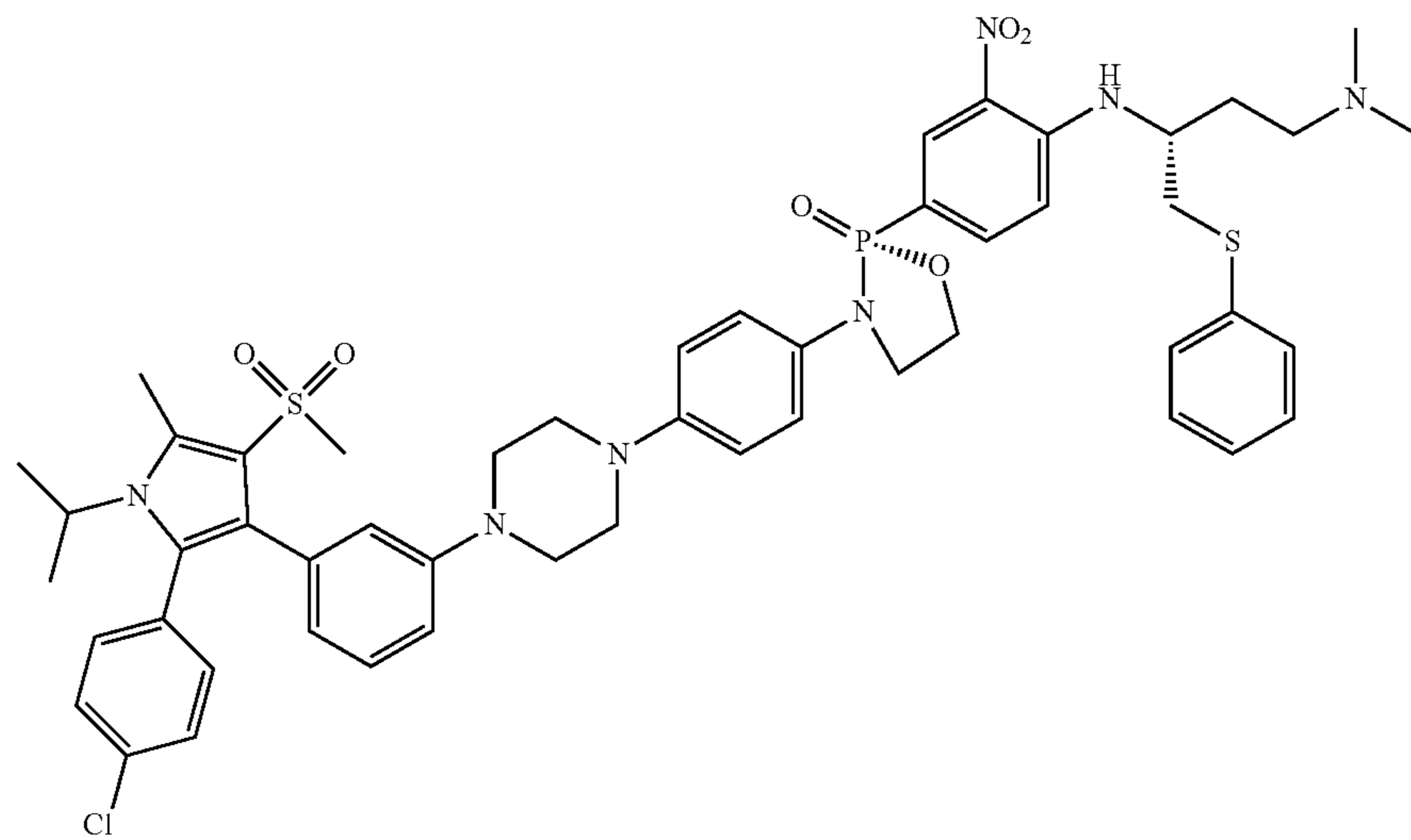
(R)-3-(4-(4-(3-(2-(4-chlorophenyl)-1-isopropyl-5-methyl-4-(methylsulfonyl)-1H-pyrrol-3-yl)phenyl)piperazin-1-yl)phenyl)-2-(4-(((R)-4-(dimethylamino)-1-(phenylthio)butan-2-yl)amino)-3-nitrophenyl)-1,3,2-oxazaphospholidine 2-oxide
