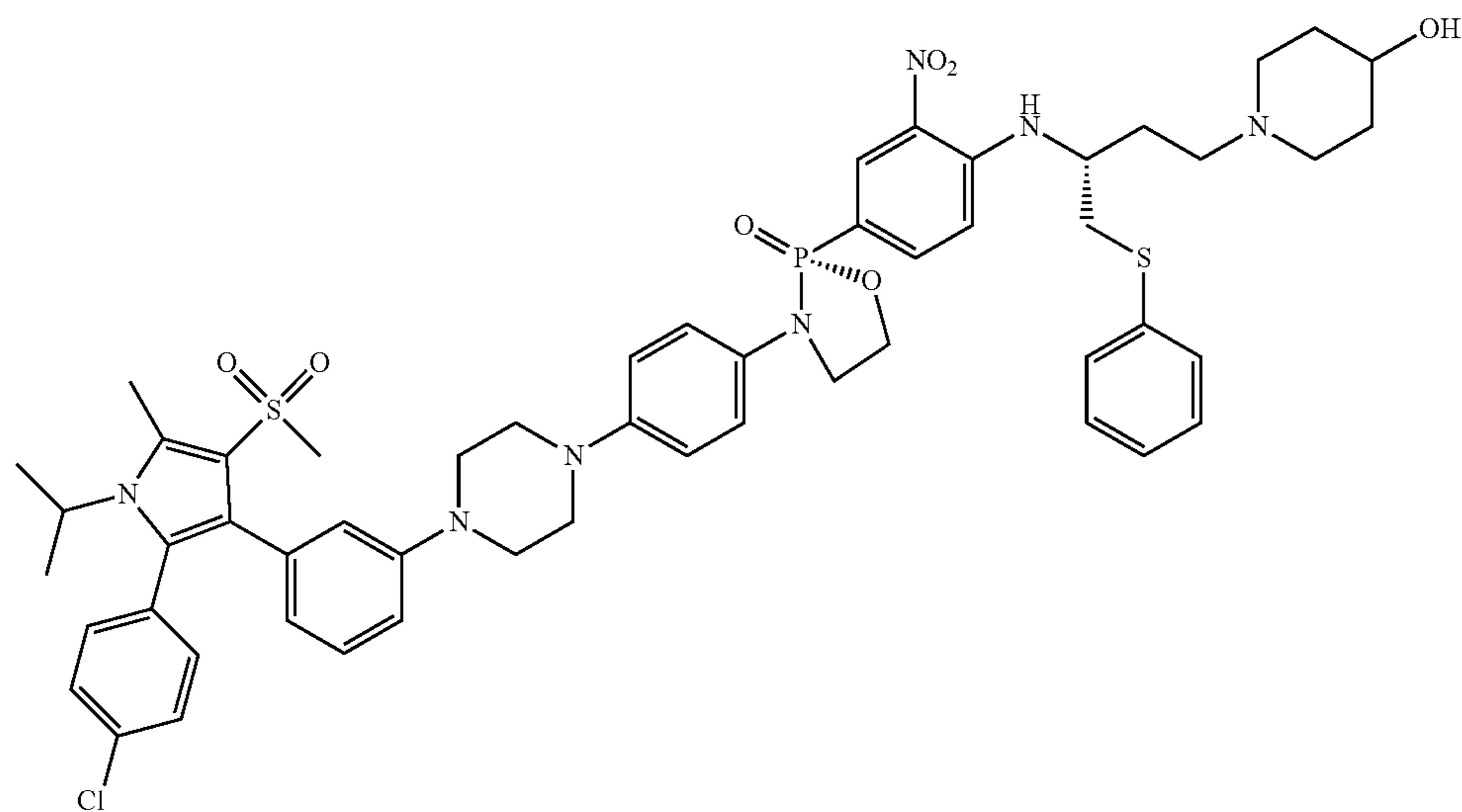
(R)-3-(4-(4-(3-(2-(4-chlorophenyl)-1-isopropyl-5-methyl-4-(methylsulfonyl)-1H-pyrrol-3-yl)-phenyl)piperazin-1-yl)phenyl)-2-(4-(((R)-4-(4-hydroxypiperidin-1-yl)-1-(phenylthio)butan-2-yl)amino)-3-nitrophenyl)-1,3,2-oxazaphospholidine 2-oxide
