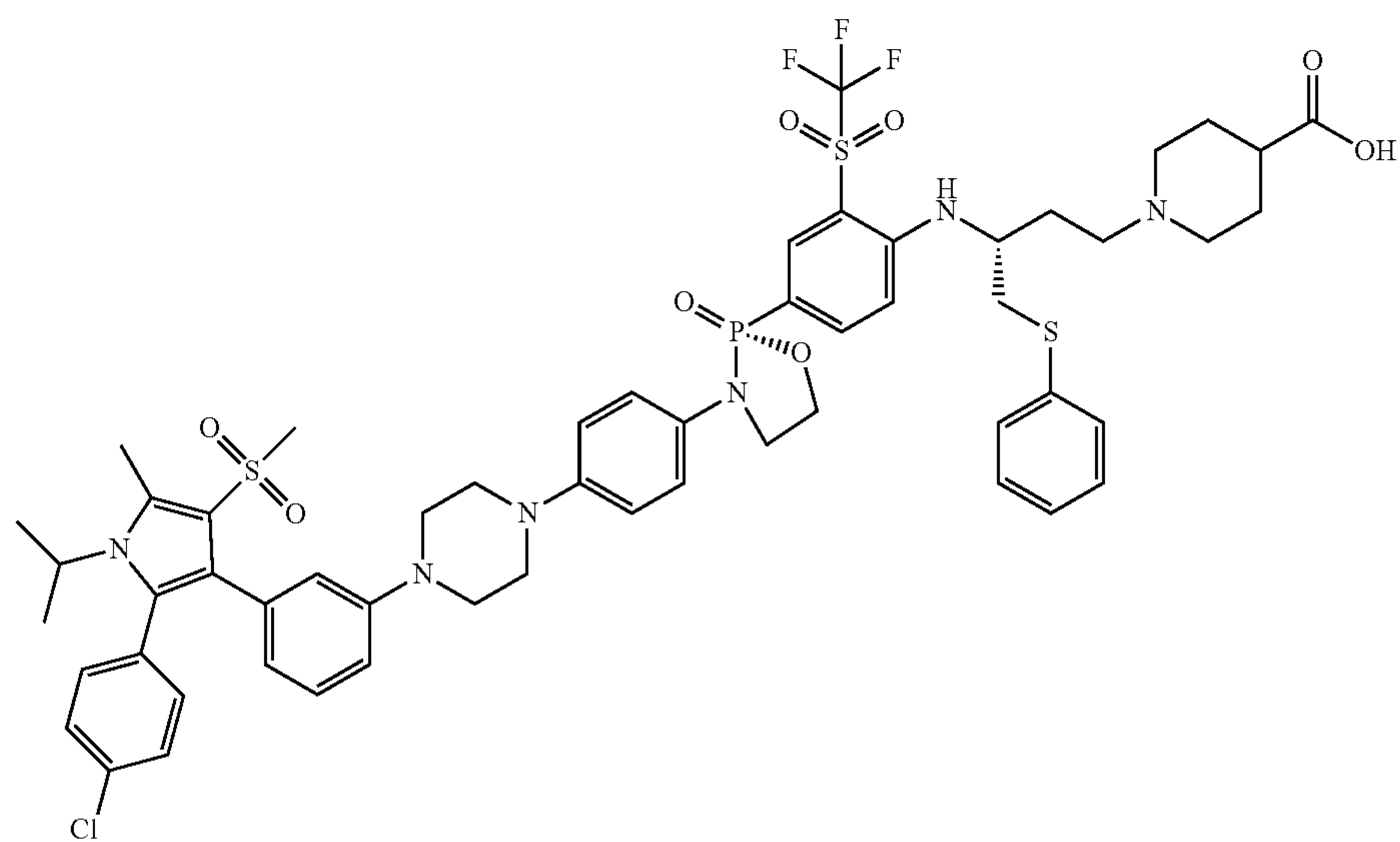
1-((R)-3-((4-((R)-3-(4-(4-(3-(2-(4-chlorophenyl)-1-isopropyl-5-methyl-4-(methylsulfonyl)-1H-pyrrol-3-yl)phenyl)piperazin-1-yl)phenyl)-2-oxido-1,3,2-oxazaphospholidin-2-yl)-2-(trifluoromethyl)sulfonyl)phenyl)amino)-4-(phenylthio)butyl)piperidine-4-carboxylic acid
