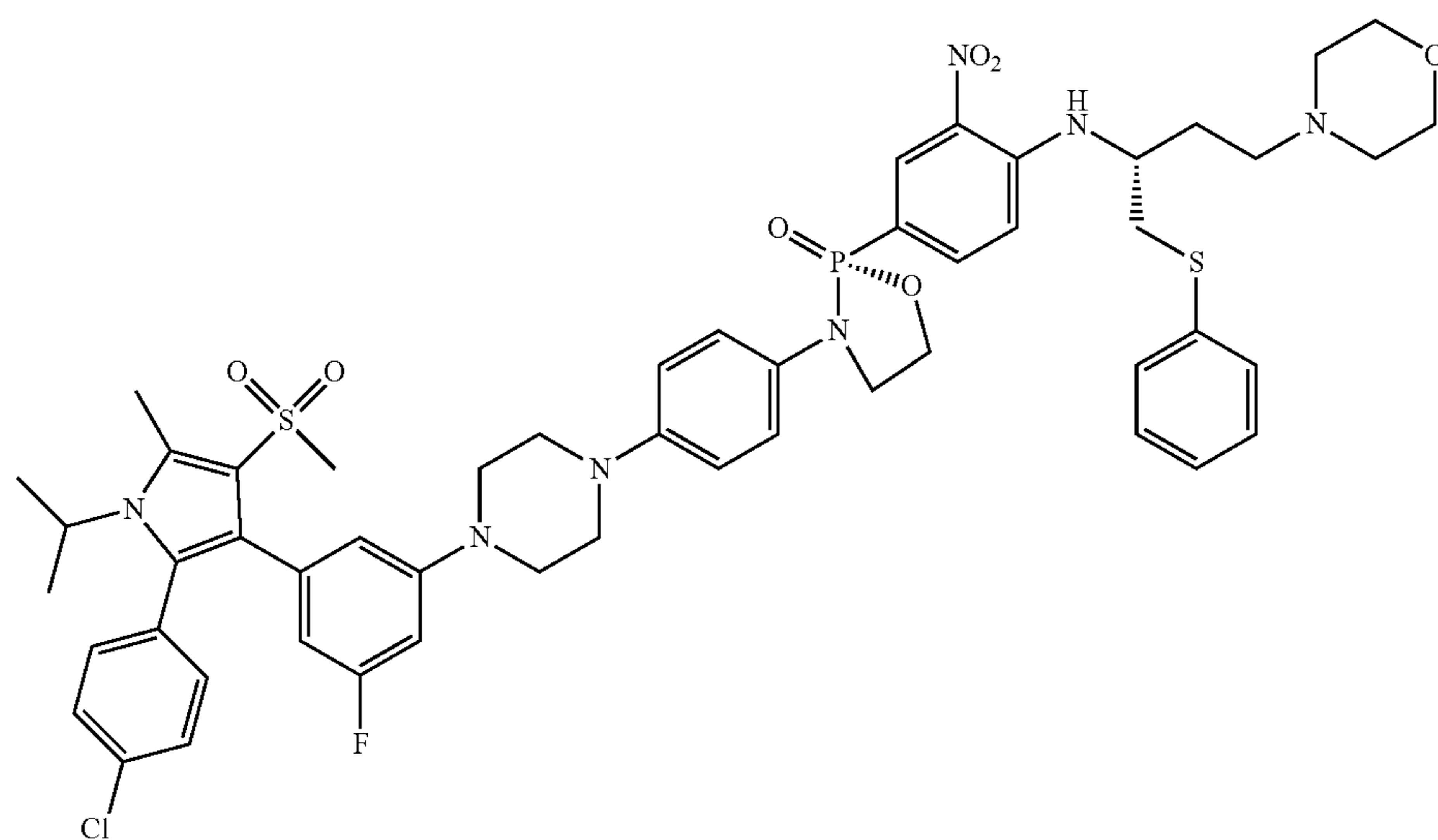
(R)-3-(4-(4-(3-(2-(4-chlorophenyl)-1-isopropyl-5-methyl-4-(methylsulfonyl)-1H-pyrrol-3-yl)-5-fluorophenyl)piperazin-1-yl)phenyl)-2-(4-(((R)-4-morpholino-1-(phenylthio)butan-2-yl)amino)-3-nitrophenyl)-1,3,2-oxazaphospholidine 2-oxide
