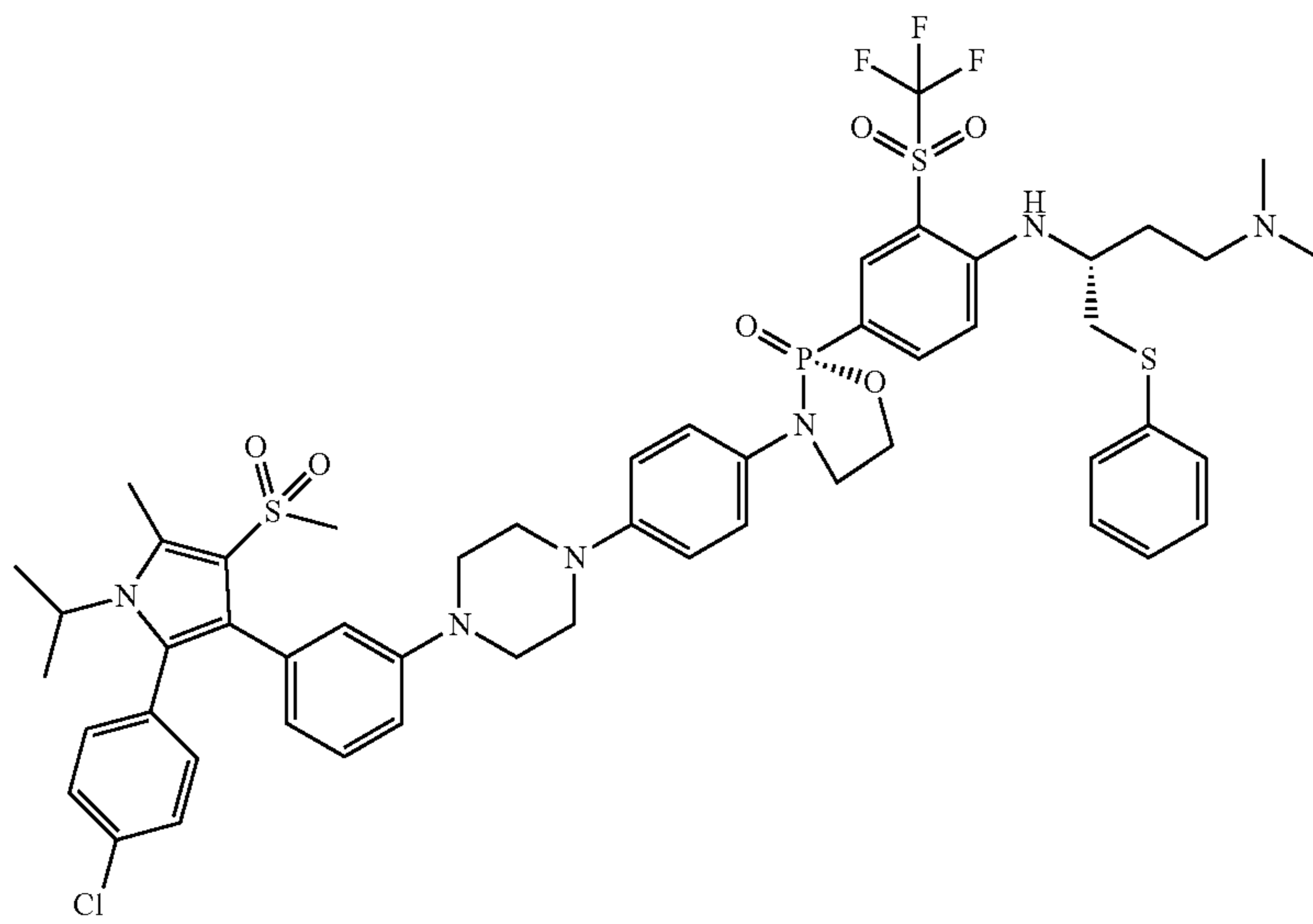
(R)-3-(4-(3-(2-(4-chlorophenyl)-1-isopropyl-5-methyl-4-(methylsulfonyl)-1H-pyrrol-3-yl)phenyl)piperazin-1-yl)phenyl-2-(4-(((R)-4-(dimethylamino)-1-(phenylthio)butan-2-yl)amino)-3-(trifluoromethyl)sulfonyl)phenyl)-1,3,2-oxazaphospholidine 2-oxide
