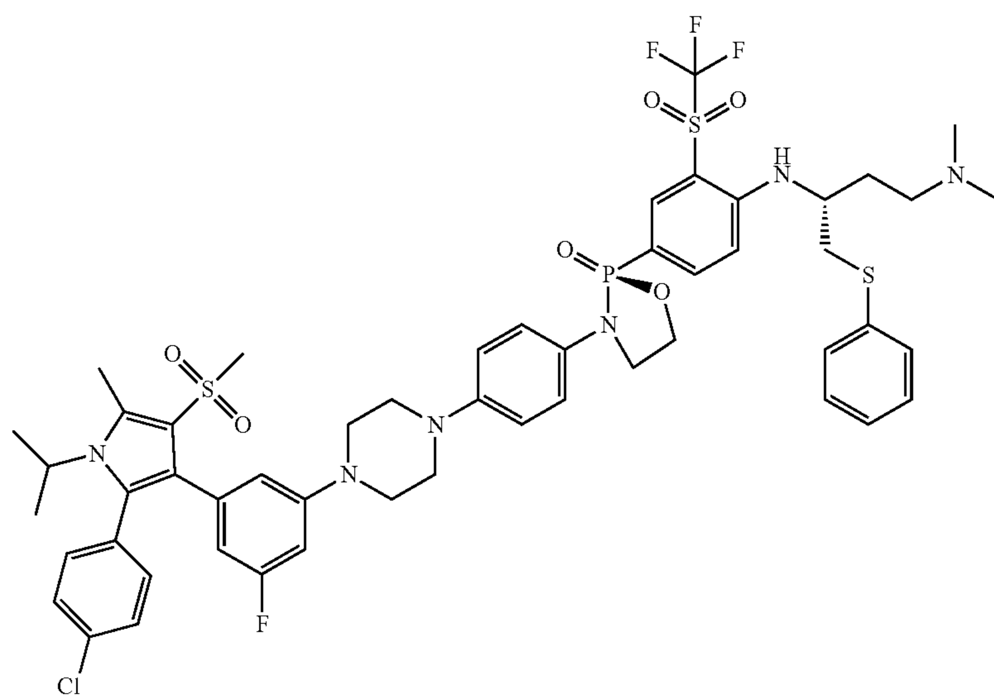
(S)-3-(4-(4-(3-(2-(4-chlorophenyl)-1-isopropyl-5-methyl-4-(methylsulfonyl)-1H-pyrrol-3-yl)-5-fluorophenyl)piperazin-1-yl)phenyl)-2-(4-((R)-4-(dimethylamino)-1-(phenylthio)butan-2-yl)amino)-3-(trifluoromethylsulfonyl)phenyl)-1,3,2-oxazaphospholidine 2-oxide
