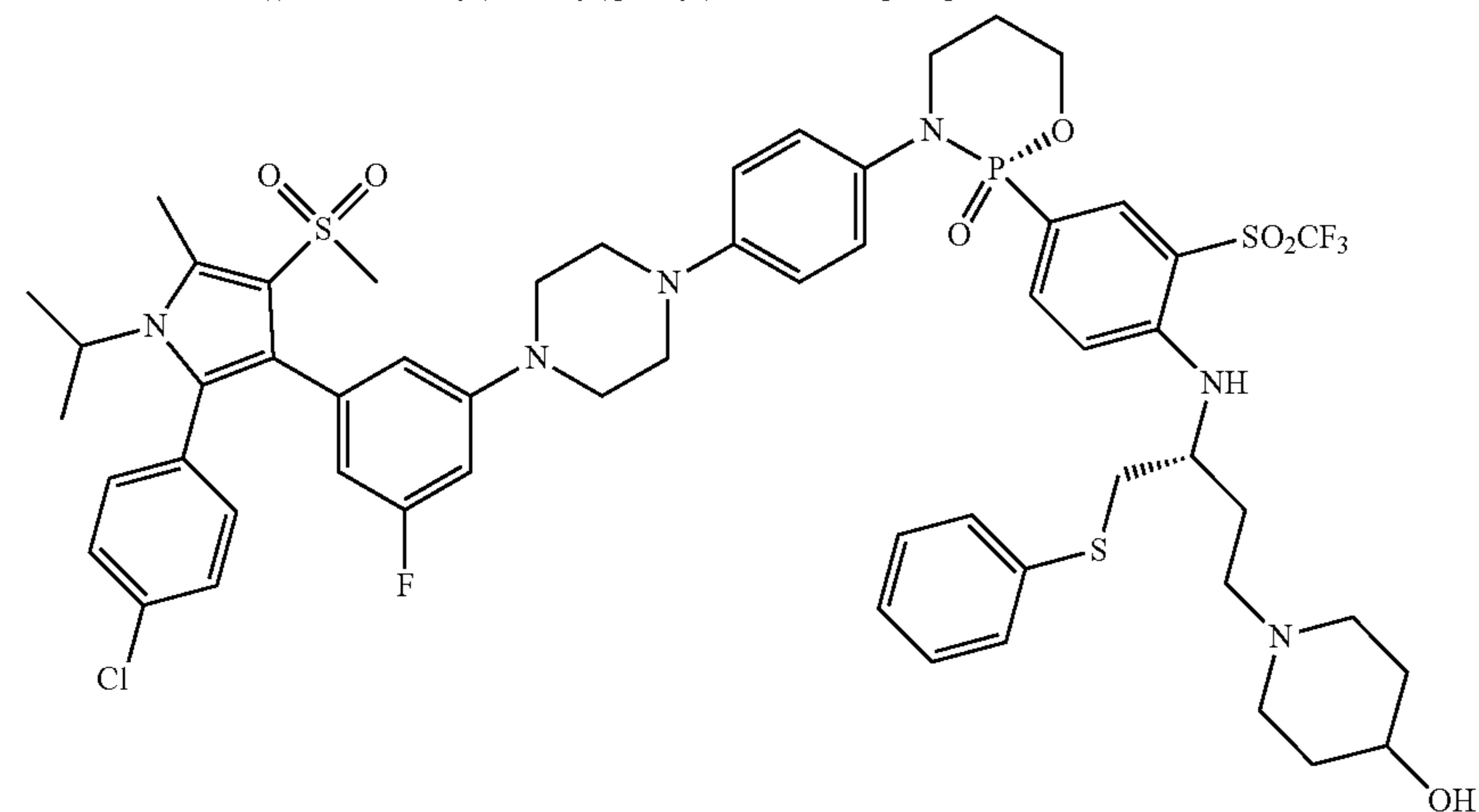
(R)-3-(4-(4-(3-(2-(4-chlorophenyl)-1-isopropyl-5-methyl-4-(methylsulfonyl)-1H-pyrrol-3-yl)-5-fluorophenyl)piperazin-1-yl)phenyl)-2-(4-(((R)-4-(dimethylamino)-1-(phenylthio)butan-2-yl)amino)-3-((trifluoromethyl)sulfonyl)phenyl)-1,3,2-oxazaphosphinane 2-oxide
