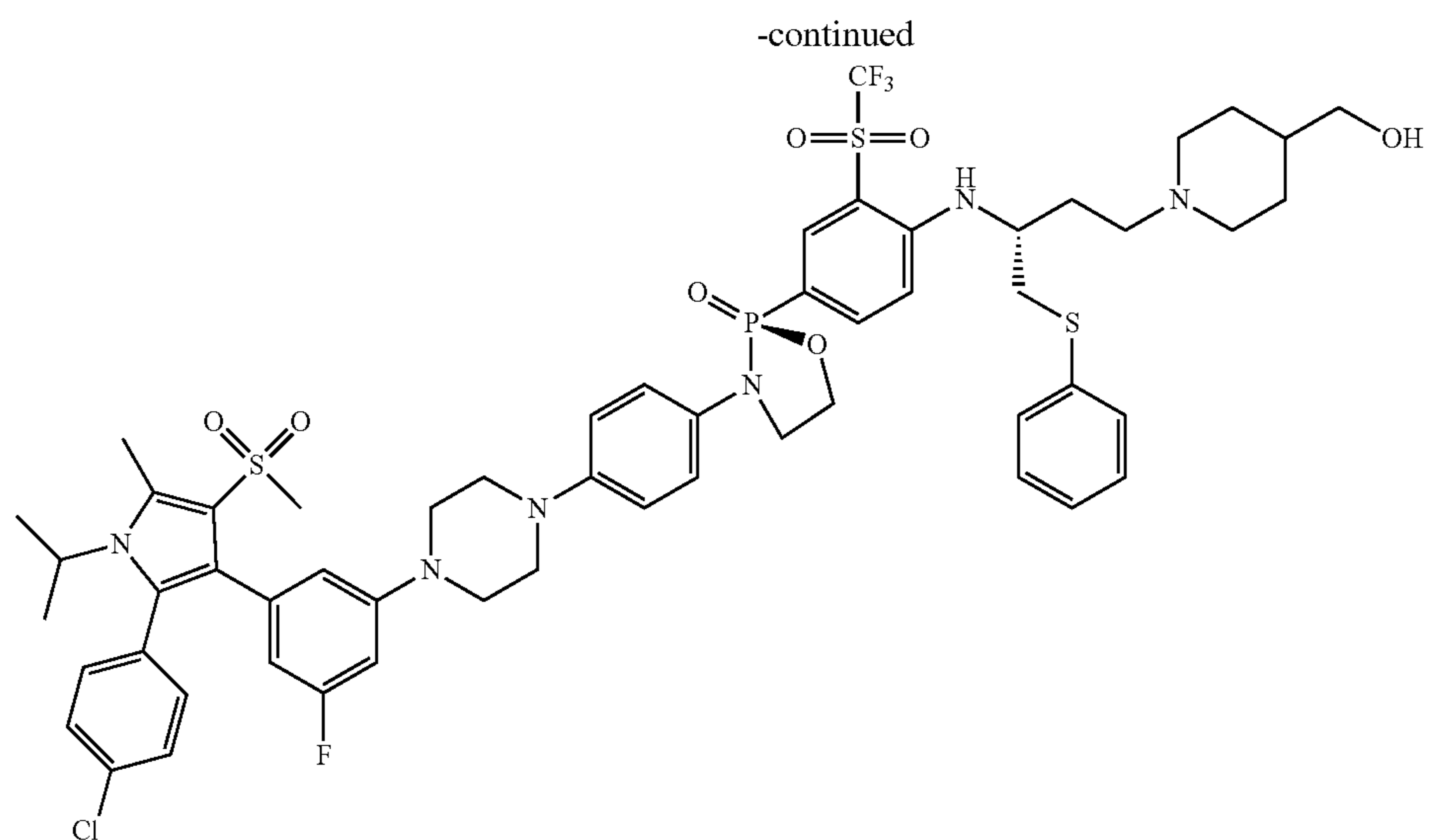
(S)-3-(4-(4-(3-(2-(4-chlorophenyl)-1-isopropyl-5-methyl-4-(methylsulfonyl)-1H-pyrrol-3-yl)-5-fluorophenyl)piperazin-1-yl)phenyl)-2-(4-(((R)-4-(4-hydroxymethyl)piperidin-1-yl)-1-(phenylthio)butan-2-yl)amino)-3-((trifluoromethyl)sulfonyl)phenyl)-1,3,2-oxazaphospholidine 2-oxide
