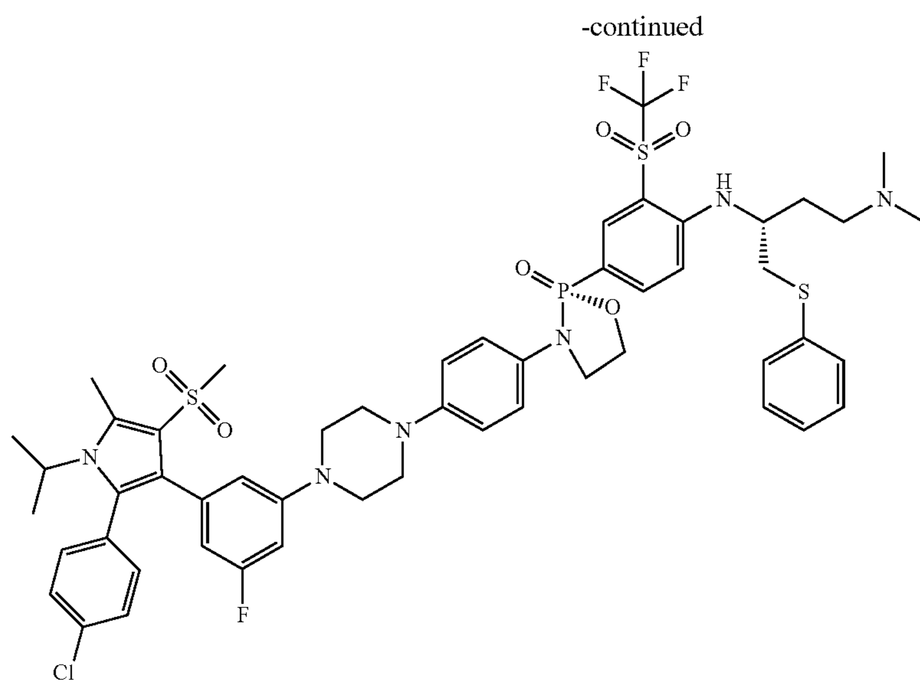
(R)-3-(4-(4-(3-(2-(4-chlorophenyl)-1-isopropyl-5-methyl-4-(methylsulfonyl)-1H-pyrrol-3-yl)-5-fluorophenyl)piperazin-1-yl)phenyl)-2-(4-((R)-4-(dimethylamino)-1-(phenylthio)butan-2-yl)amino)-3-(trifluoromethylsulfonyl)phenyl)-1,3,2-oxazaphospholidine 2-oxide
