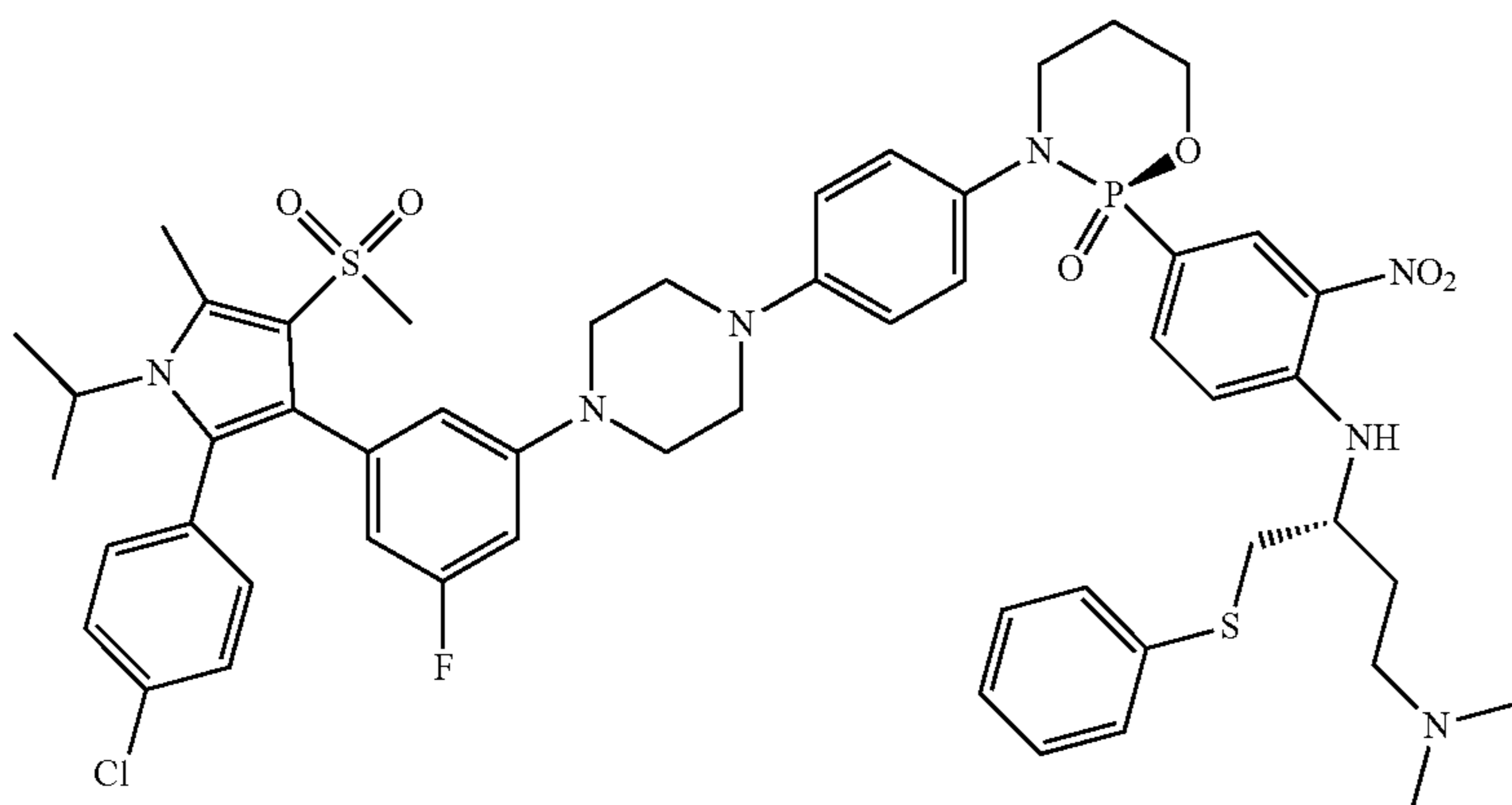
(R)-3-(4-(4-(3-(2-(4-chlorophenyl)-1-isopropyl-5-methyl-4-(methylsulfonyl)-1H-pyrrol-3-yl)-5-fluorophenyl)piperazin-1-yl)phenyl)-2-(4-(((R)-4-(dimethylamino)-1-(phenylthio)butan-2-yl)amino)-3-nitrophenyl)-1,3,2-oxazaphosphinane 2-oxide
