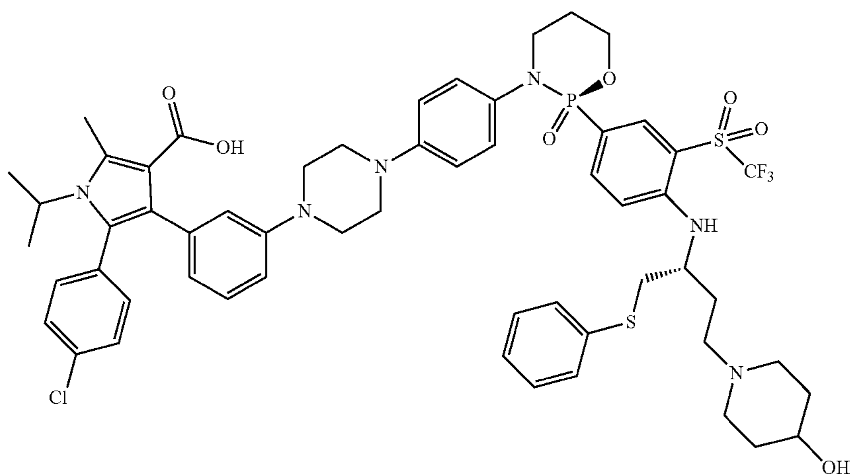
5-(4-chlorophenyl)-4-(3-(4-(4-((R)-2-4-(((R)-4-(4-hydroxypiperidin-1-yl)-1-(phenylthio)butan-2-yl)amino)-3-((trifluoromethyl)sulfonyl)phenyl)-2-oxido-1,3,2-oxazaphosphinan-3-yl)phenyl)piperazin-1-yl)phenyl)-1-isopropyl-2-methyl-1H-pyrrole-3-carboxylic acid
