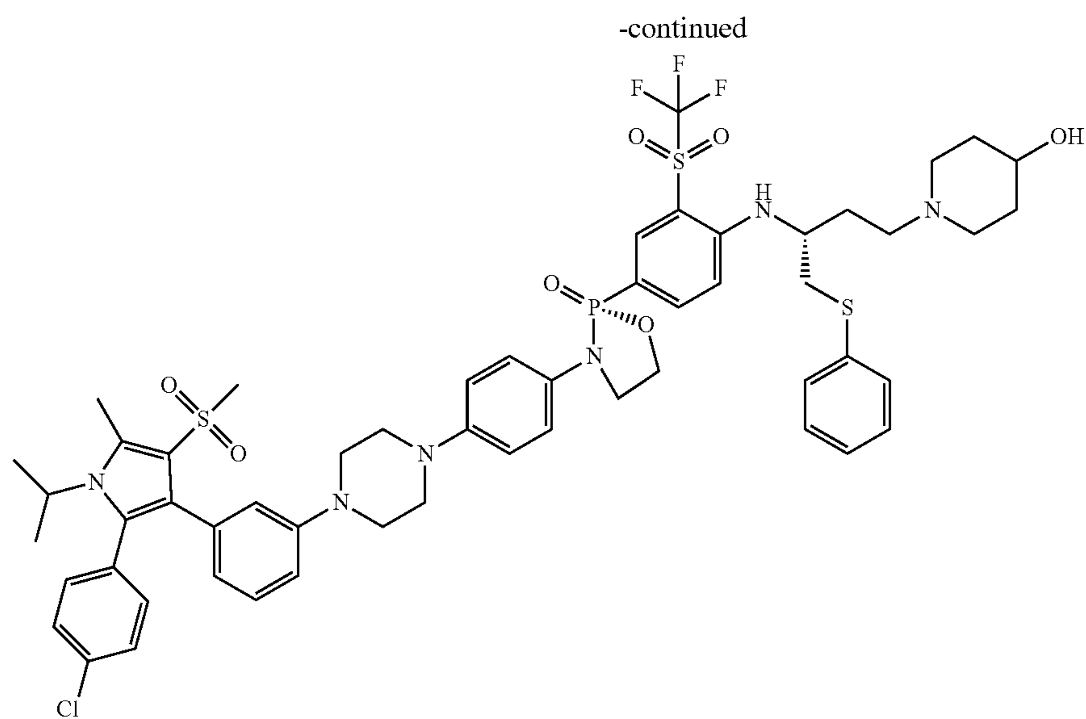
(R)-3-(4-(4-(3-(2-(4-chlorophenyl)-1-isopropyl-5-methyl-4-(methylsulfonyl)-1H-pyrrol-3-yl)phenyl)piperazin-1-yl)phenyl)-2-(4-(((R)-4-(4-(hydroxypiperidin-1-yl)-1-(phenylthio)butan-2-yl)amino)-3-(trifluoromethyl)sulfonyl)phenyl)-1,3,2-oxazaphospholidine 2-oxide
