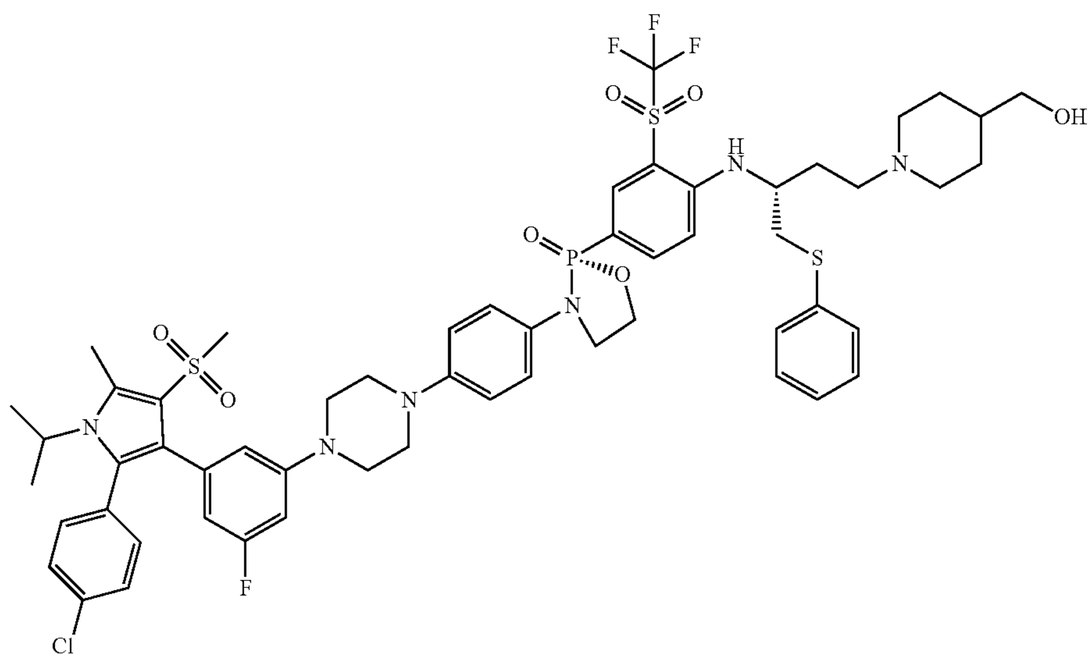
(R)-3-(4-(4-(3-(2-(4-chlorophenyl)-1-isopropyl-5-methyl-4-(methylsulfonyl)-1H-pyrrol-3-yl)-5-fluorophenyl)piperazin-1-yl)phenyl)-2-(4-(((R)-4-(4-(hydroxymethyl)piperidin-1-yl)-1-(phenylthio)butan-2-yl)amino)-3-(trifluoromethyl)sulfonyl)phenyl)-1,3,2-oxazaphospholidine 2-oxide
