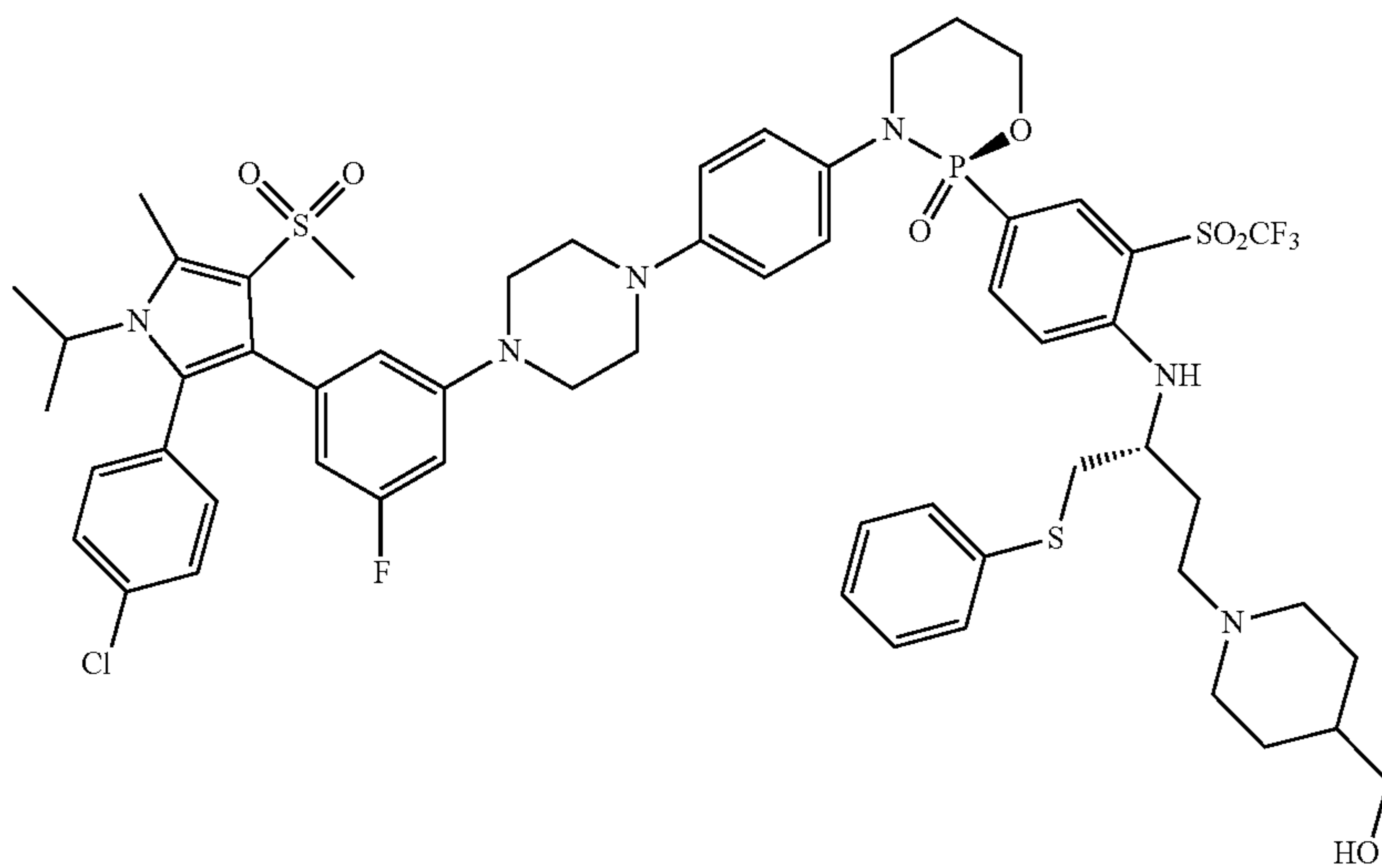
(R)-3-(4-(4-(3-(2-(4-chlorophenyl)-1-isopropyl-5-methyl-4-(methylsulfonyl)-1H-pyrrol-3-yl)-5-fluorophenyl)piperazin-1-yl)phenyl)-2-(4-(((R)-4-(4-hydroxypiperidin-1-yl)-1-(phenylthio)butan-2-yl)amino)-3-((trifluoromethyl)sulfonyl)phenyl)-1,3,2-oxazaphosphinane 2-oxide
