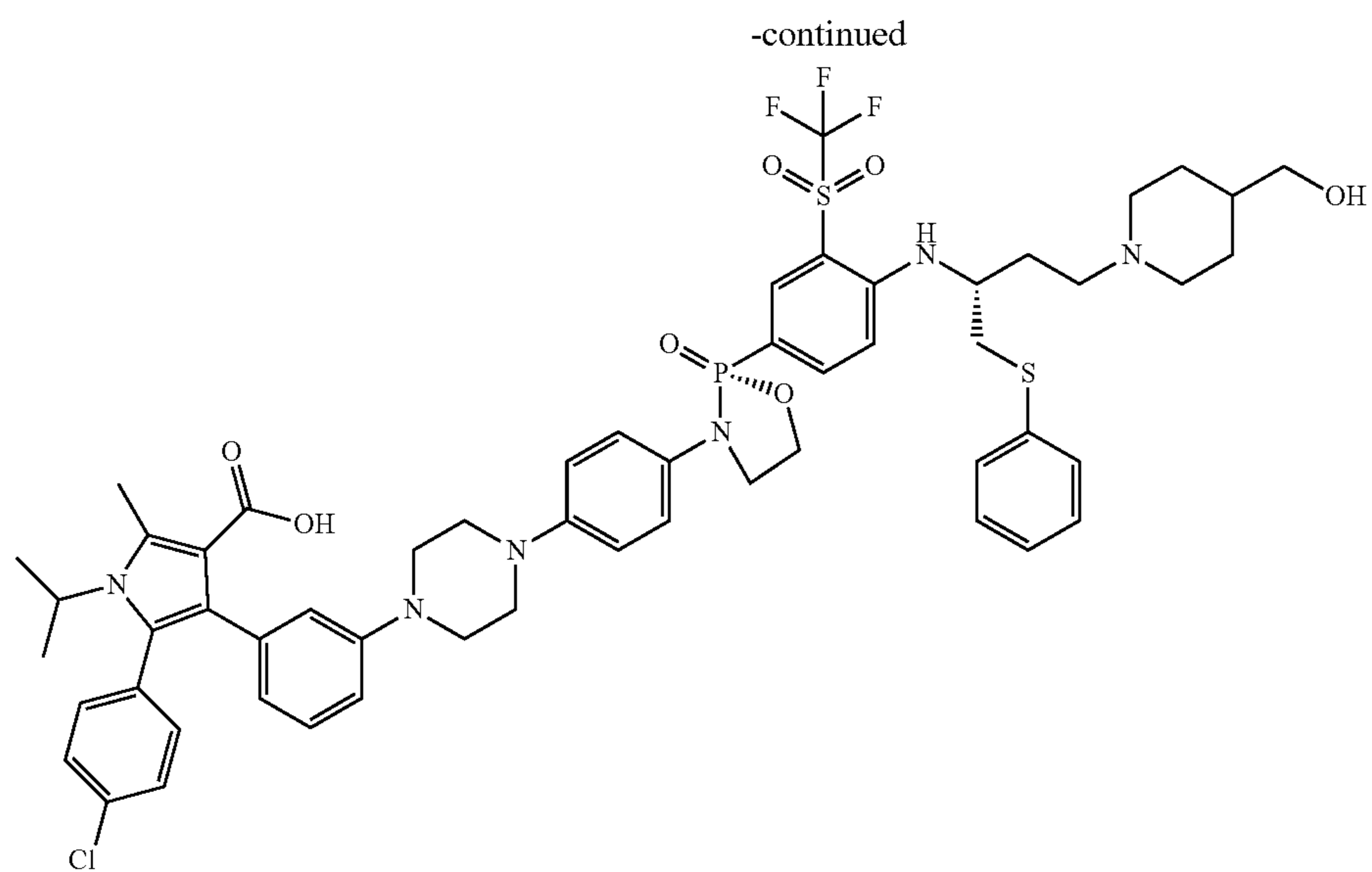
5-(4-chlorophenyl)-4-(3-(4-(4-((R)-2-(4-((R)-4-(4-hydroxymethyl)piperidin-1-yl)-1-(phenylthio)butan-2-yl)amino)-3-(trifluoromethyl)sulfonyl)phenyl)-2-oxido-1,3,2-oxazaphospholidin-3-yl)phenyl)piperazin-1-yl)phenyl)-1-isopropyl-2-methyl-1H-pyrrole-3-carboxylic acid
