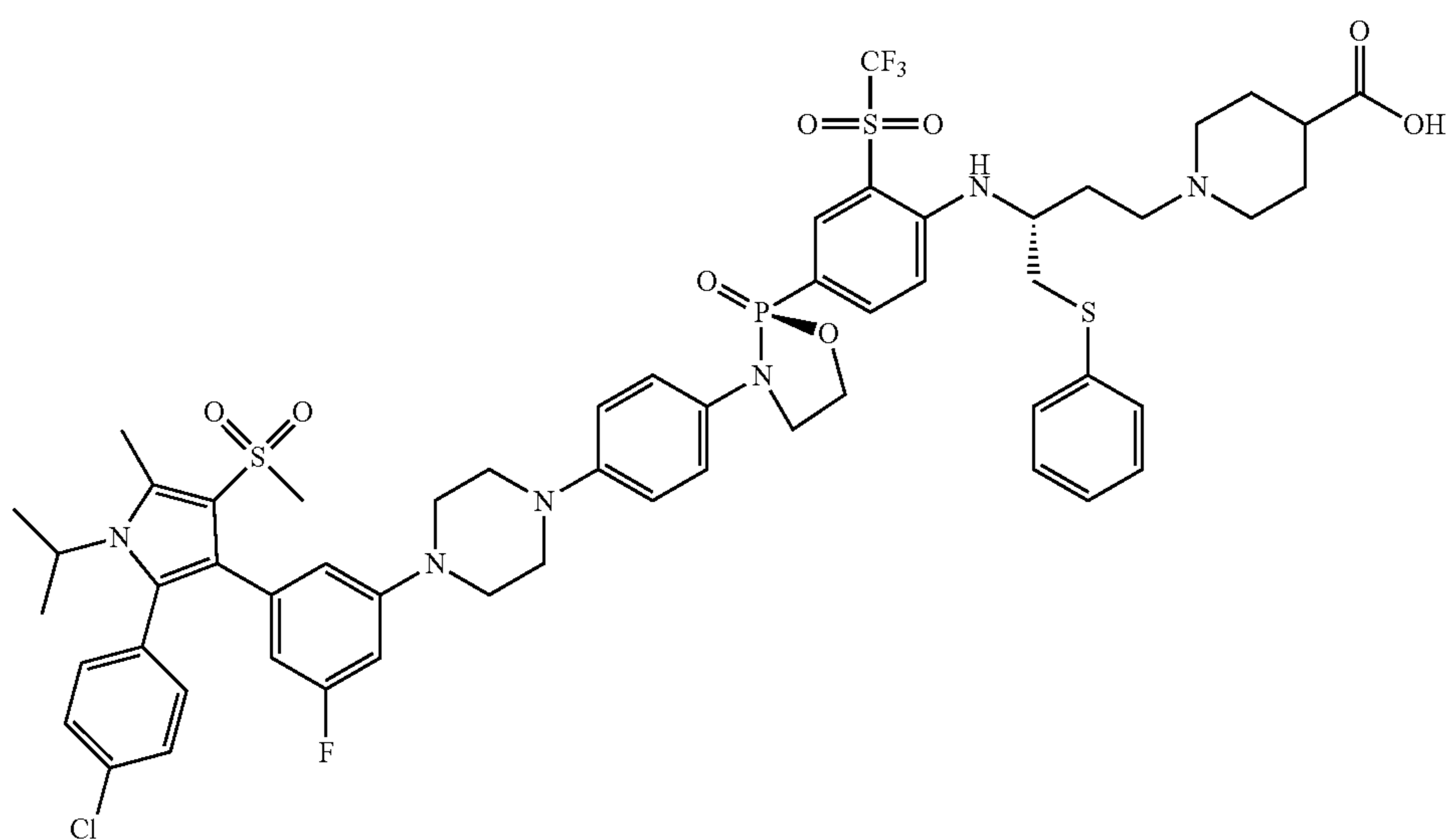
1-((R)-3-((4-((S)-3-(4-(4-(3-(2-(4-chlorophenyl)-1-isopropyl-5-methyl-4-(methylsulfonyl)-1H-pyrrol-3-yl)phenyl)piperazin-1-yl)phenyl)-2-oxido-1,3,2-oxazaphospholidin-2-yl)-2-((trifluoromethyl)sulfonyl)phenyl)amino)-4-(phenylthio)butyl)piperidine-4-carboxylic acid
