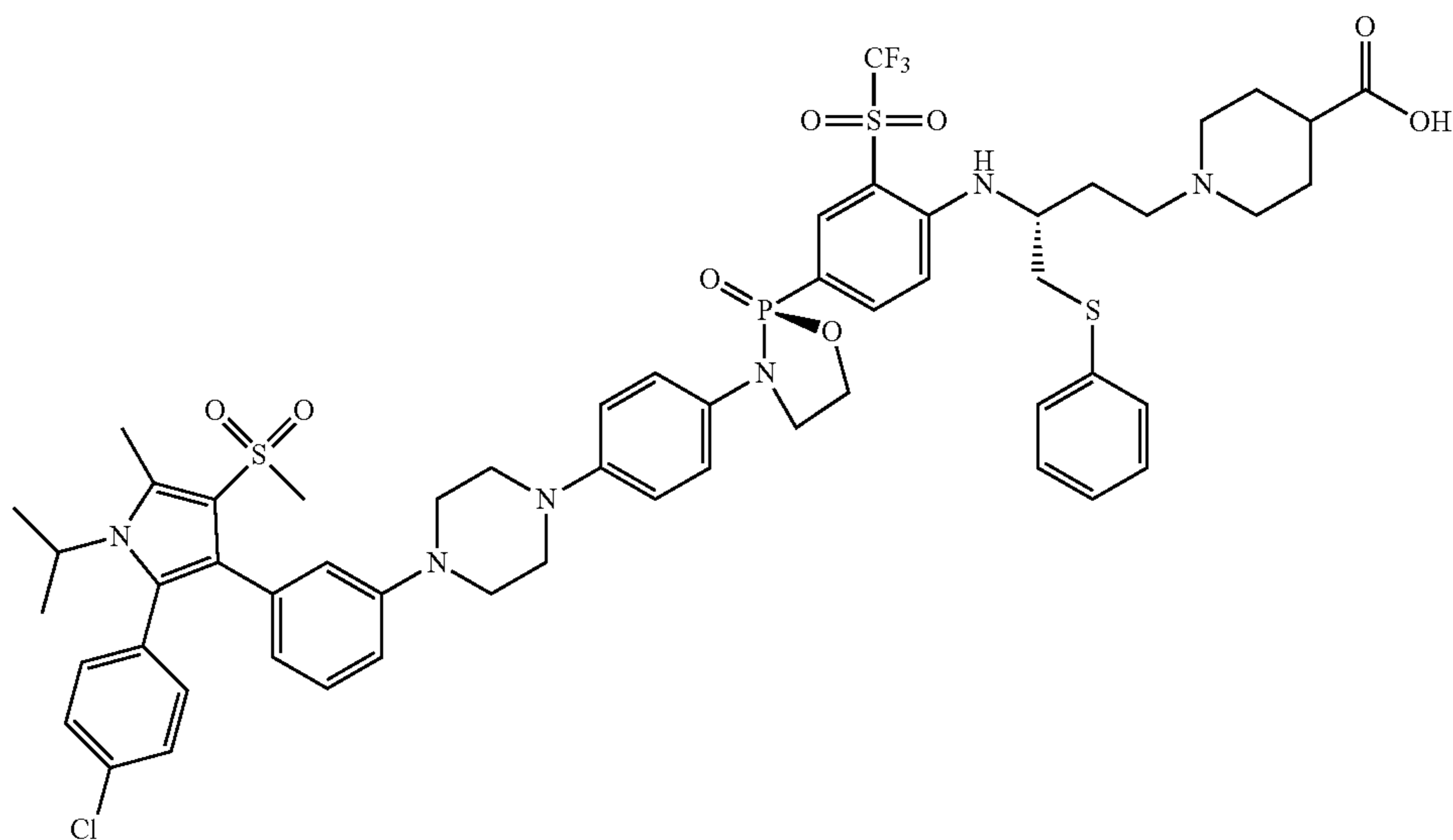
1-((R)-3-((4-((S)-3-(4-(4-(3-(2-(4-chlorophenyl)-1-isopropyl-5-methyl-4-(methylsulfonyl)-1H-pyrrol-3-yl)phenyl)piperazin-1-yl)phenyl)-2-oxido-1,3,2-oxazaphospholidin-2-yl)-2-(trifluoromethyl)sulfonyl)phenyl)amino)-4-(phenylthio)butyl)piperidine-4-carboxylic acid
