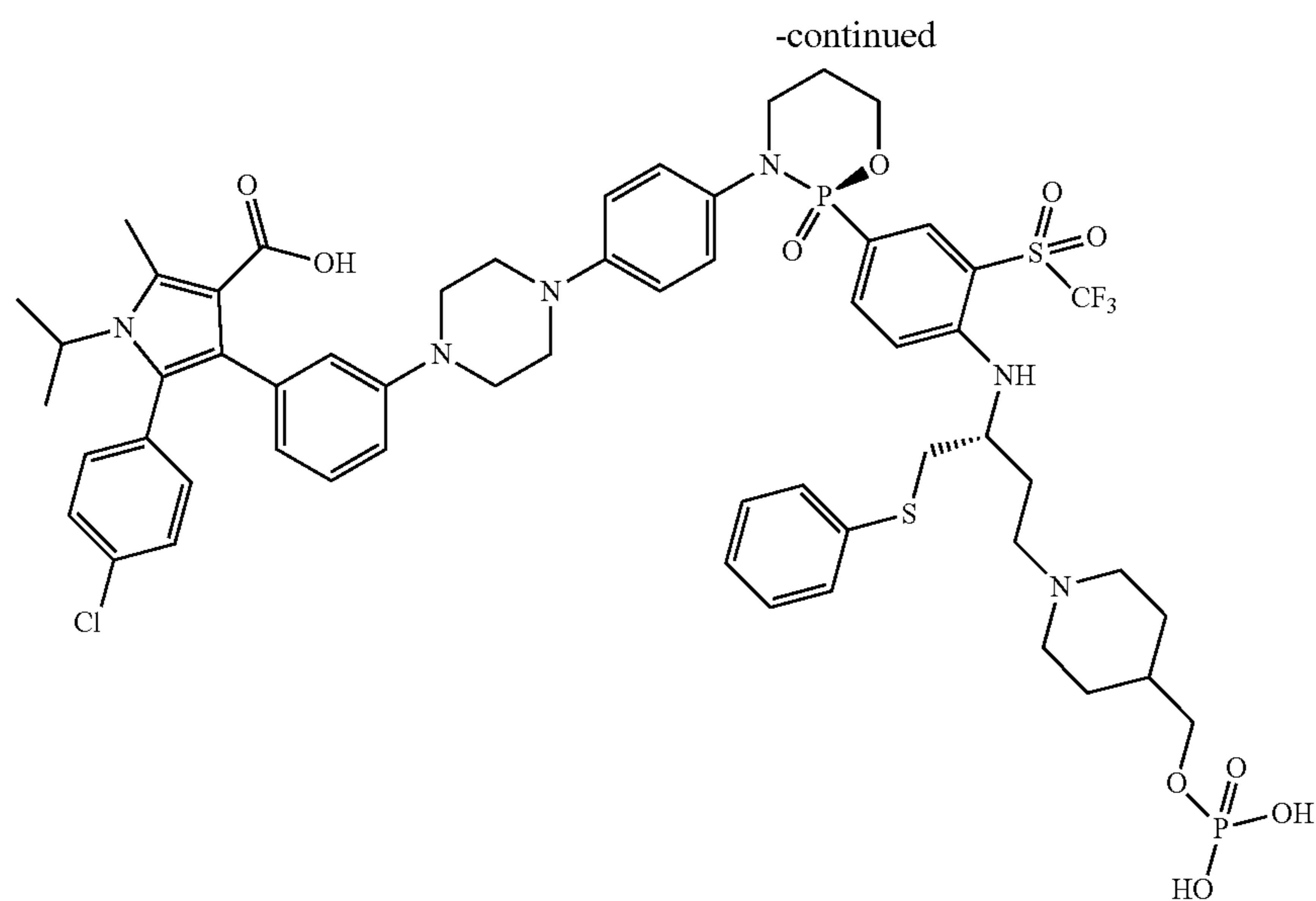
5-(4-chlorophenyl)-1-isopropyl-2-methyl-4-(3-(4-(4-((R)-2-oxido-2-(4-(((R)-1-(phenylthio)-4-(4-((phosphonooxy)methyl)piperidin-1-yl)butan-2-yl)amino)-3-((trifluoromethyl)sulfonyl)phenyl)-1,3,2-oxazaphosphinan-3-yl)phenyl)piperazin-1-yl)phenyl)-1H-pyrrole-3-carboxylic acid
