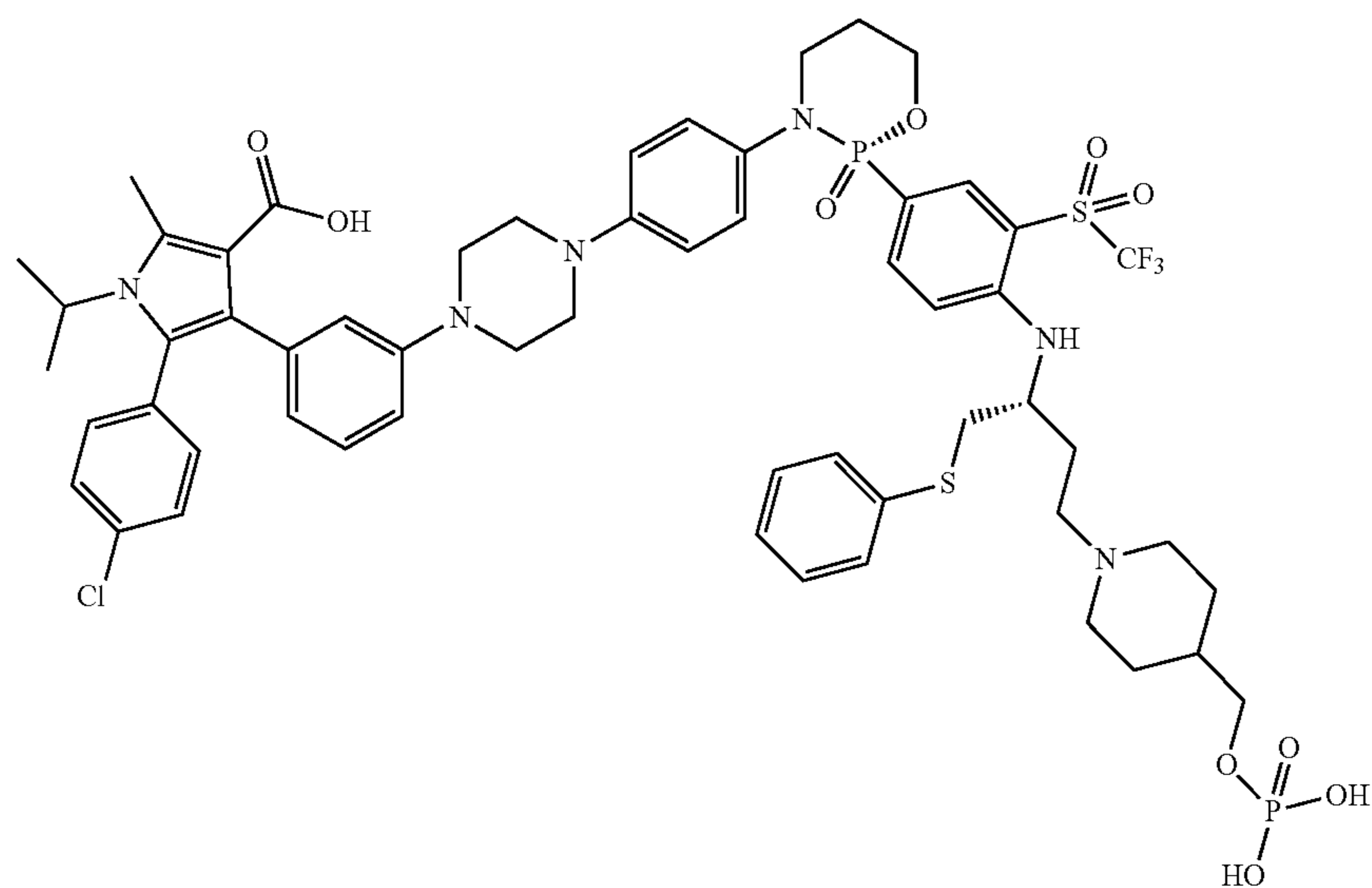
5-(4-chlorophenyl)-1-isopropyl-2-methyl-4-(3-(4-(4-((S)-2-oxido-2-(4-(((R)-1-(phenylthio)-4-(4-((phosphonooxy)methyl)piperidin-1-yl)butan-2-yl)amino)-3-((trifluoromethyl)sulfonyl)phenyl)-1,3,2-oxazaphosphinan-3-yl)phenyl)piperazin-1-yl)phenyl)-1H-pyrrole-3-carboxylic acid
