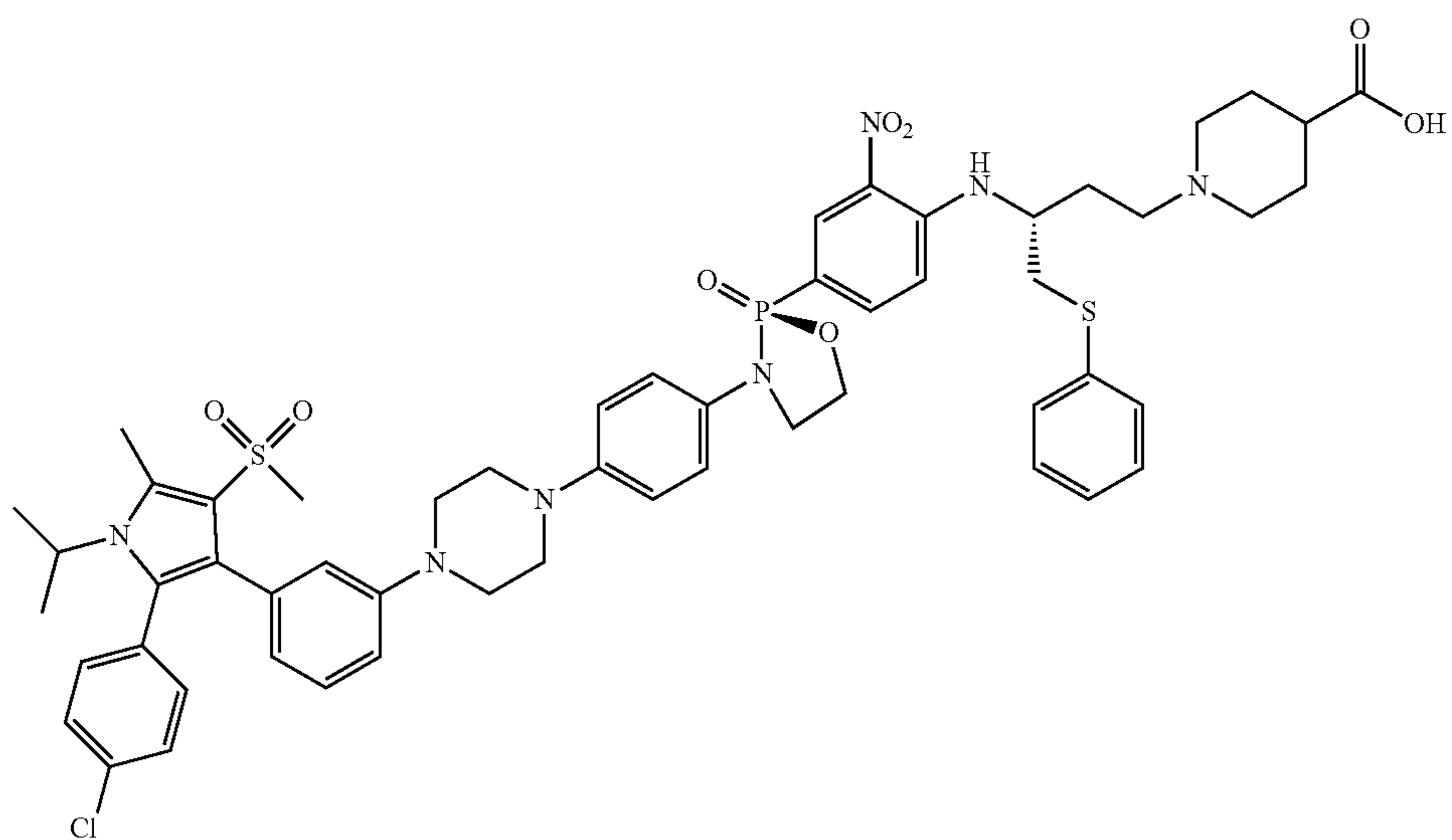
1-((S)-3-((4-((R)-3-(4-(4-(3-(2-(4-chlorophenyl)-1-isopropyl-5-methyl-4-(methylsulfonyl)-1H-pyrrol-3-yl)phenyl)piperazin-1-yl)phenyl)-2-oxido-1,3,2-oxazaphospholidin-2-yl)-2-nitrophenyl)amino)-4-(phenylthio)butyl)piperidine-4-carboxylic acid
