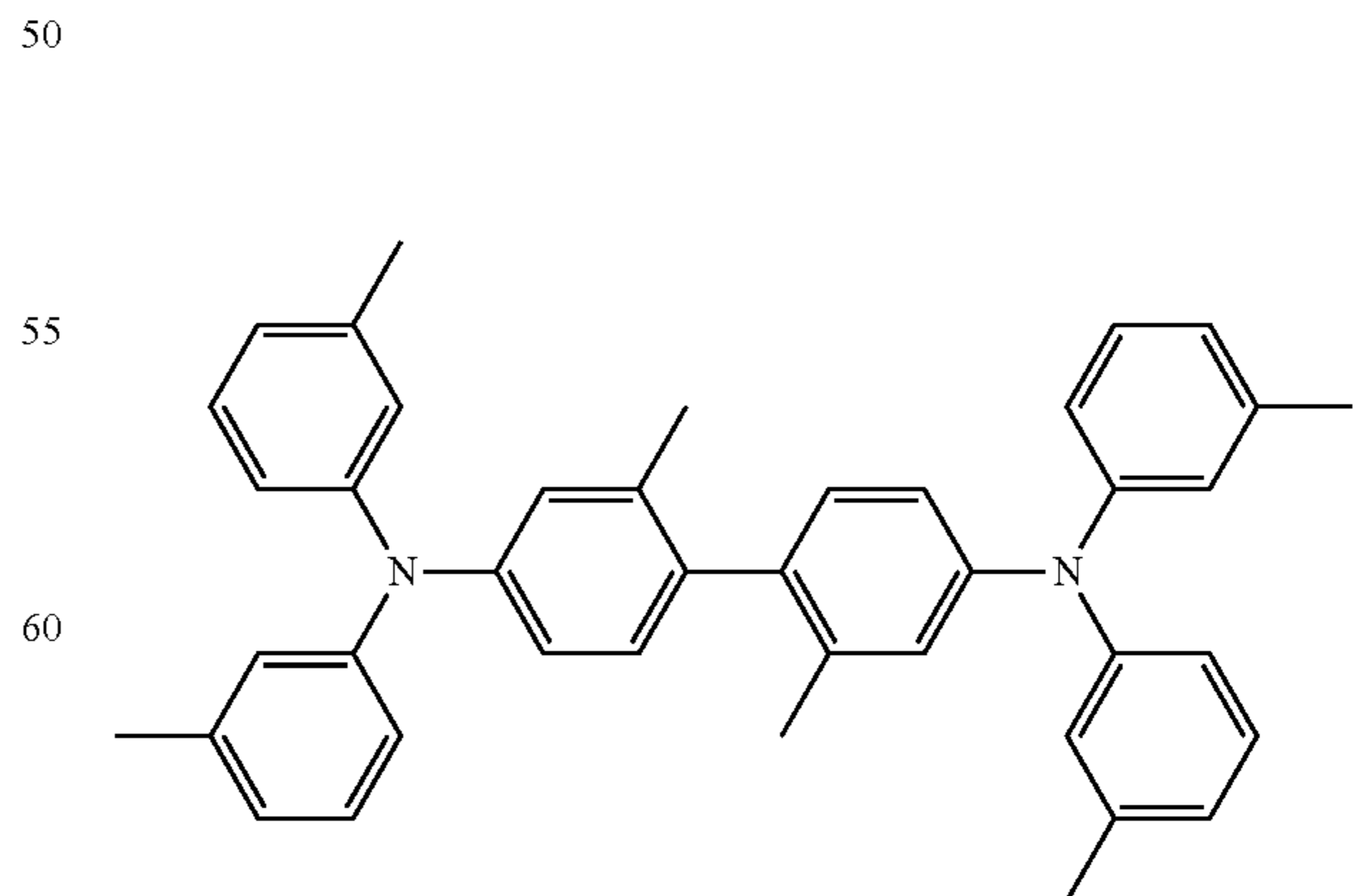
HMTPD
