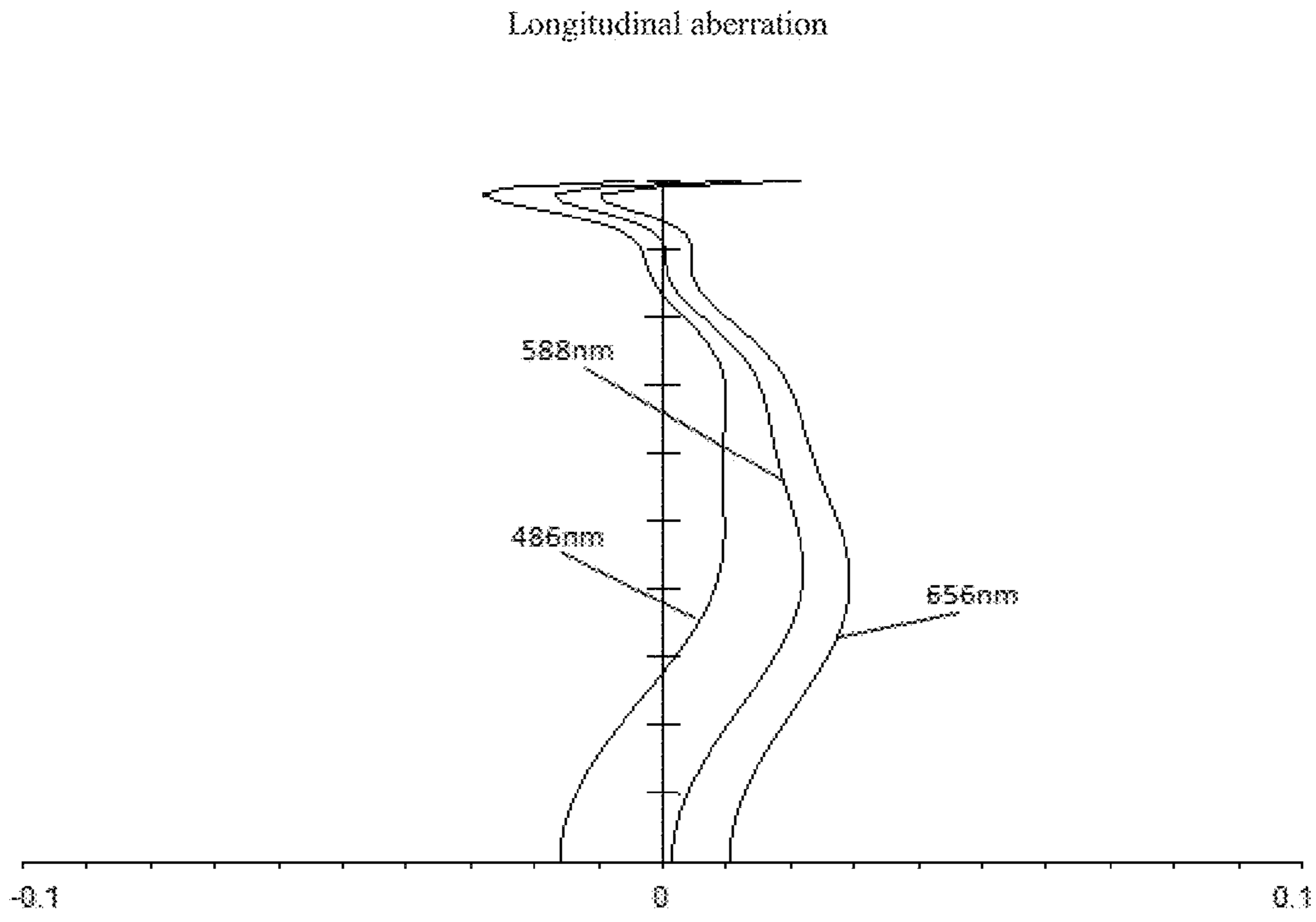
millimeter Fig. 2
