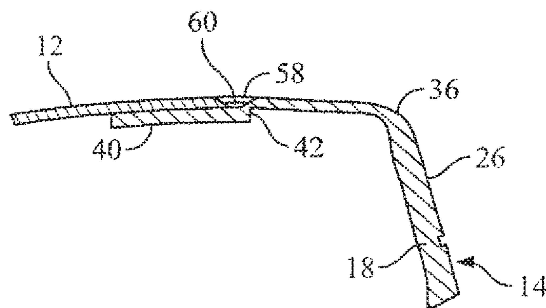
FIG. 10C
