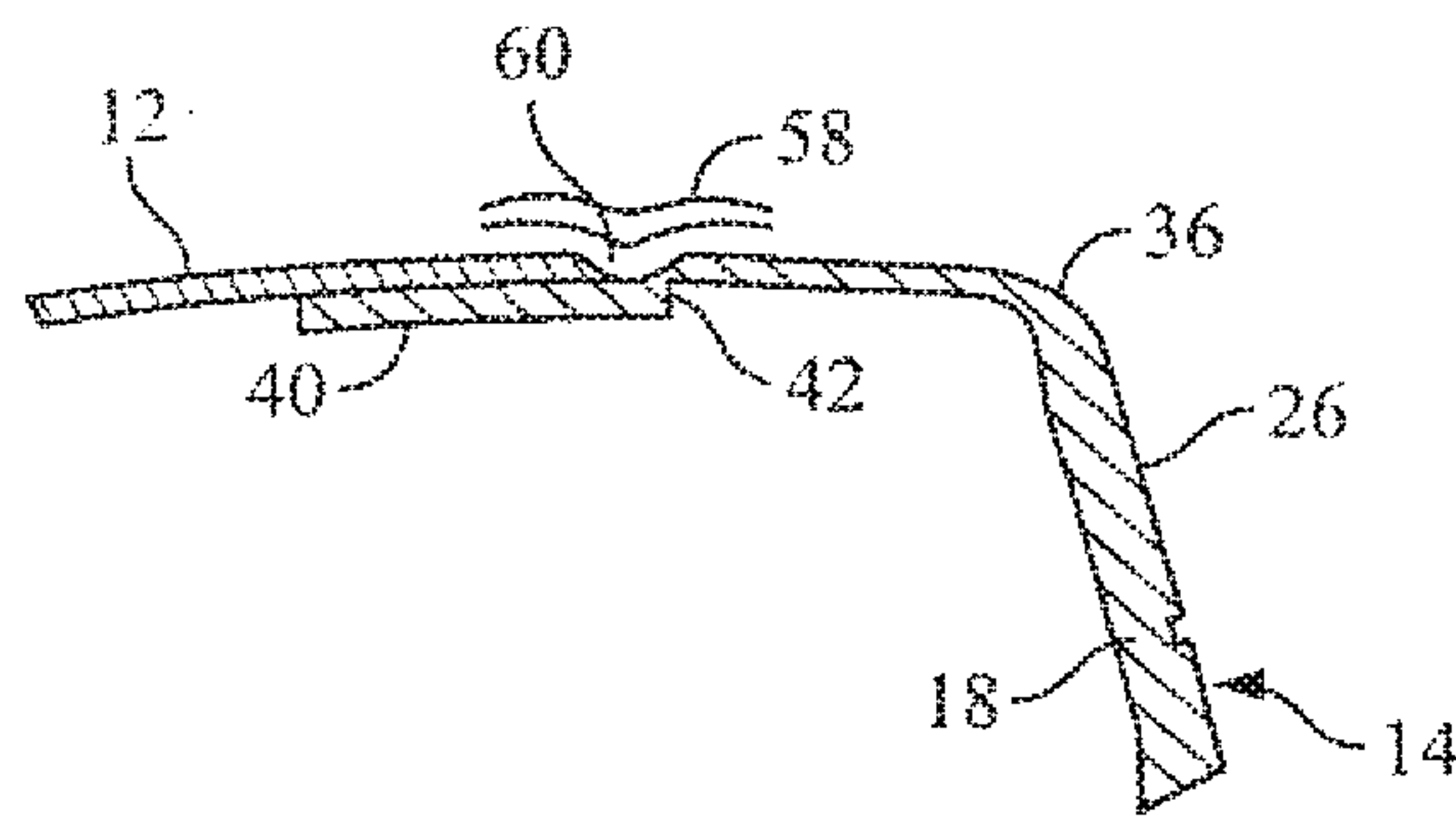
FIG. 10B
