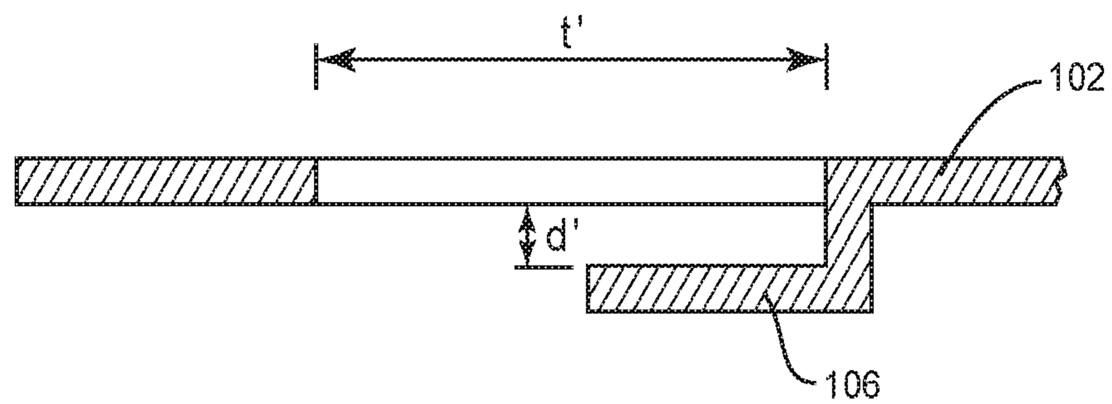
FIG. 3
