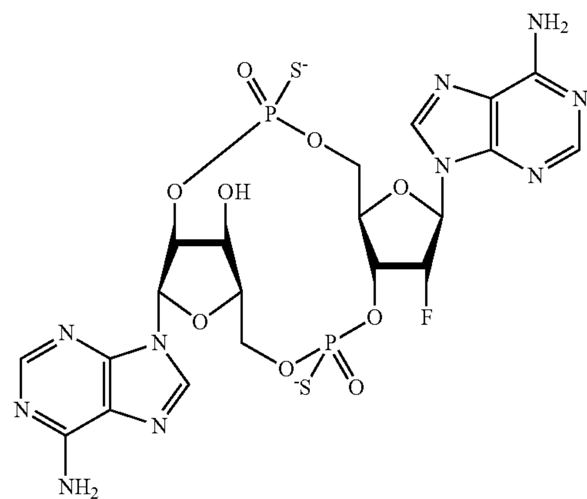
1a - Isomer 1 1b - Isomer 2
