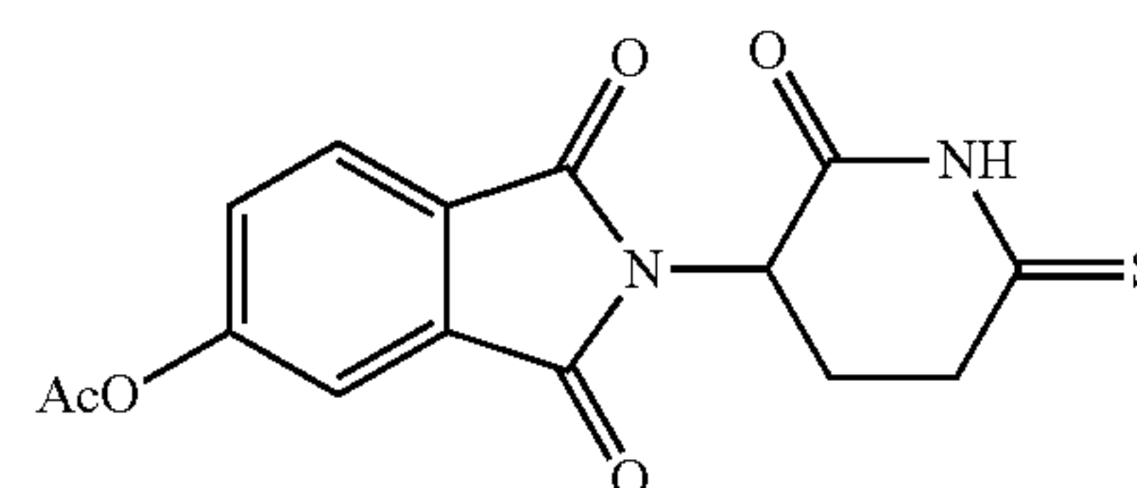
19: C 15 H 12 N 2 O 5 S MW 332.33
