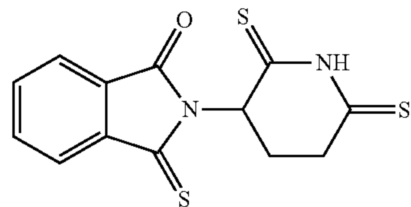
4: C 13 H 10 N 2 O 3 S MW 306.43
