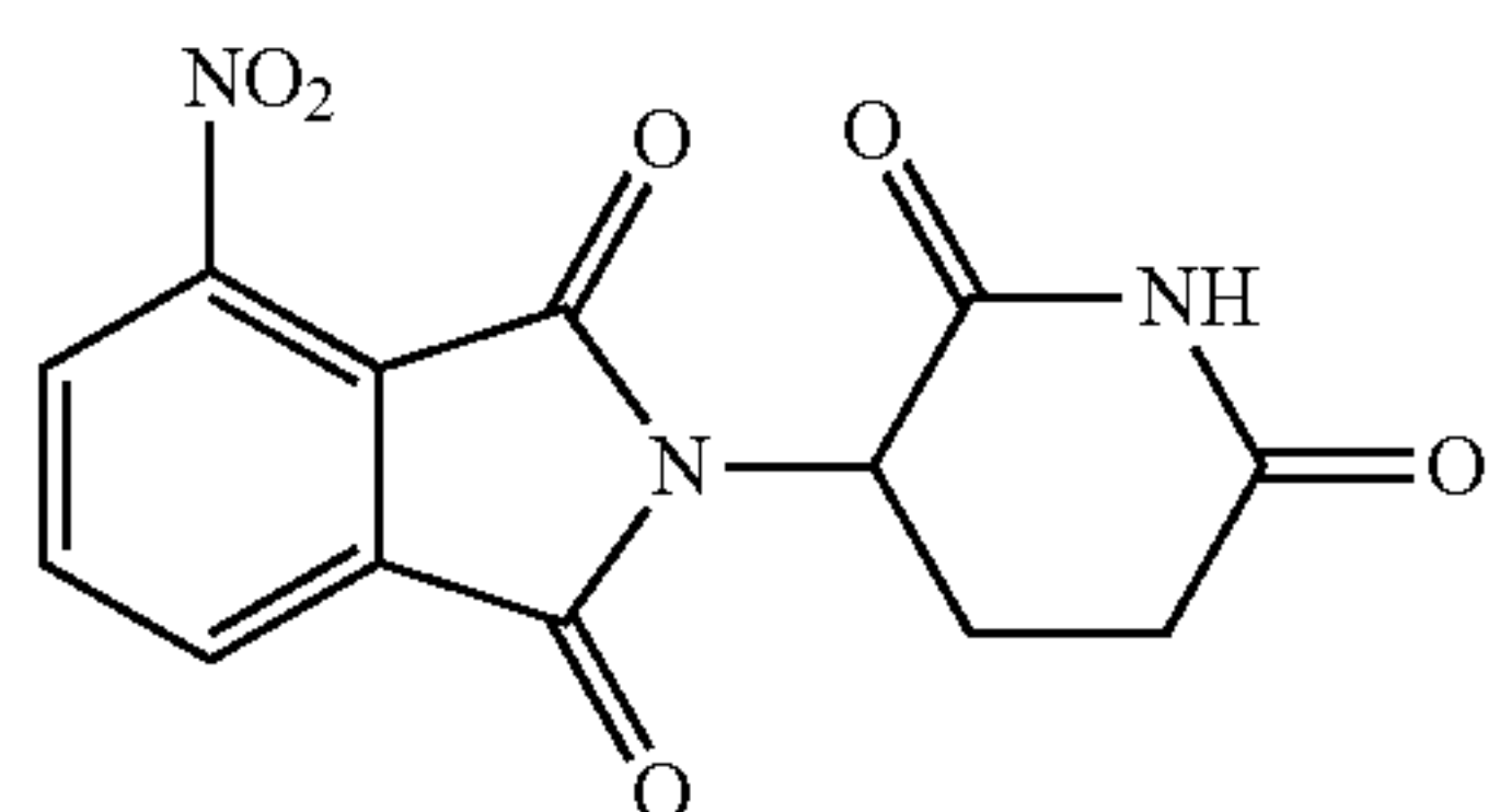
5: C 13 H 9 N 3 O 6 MW 303.23
