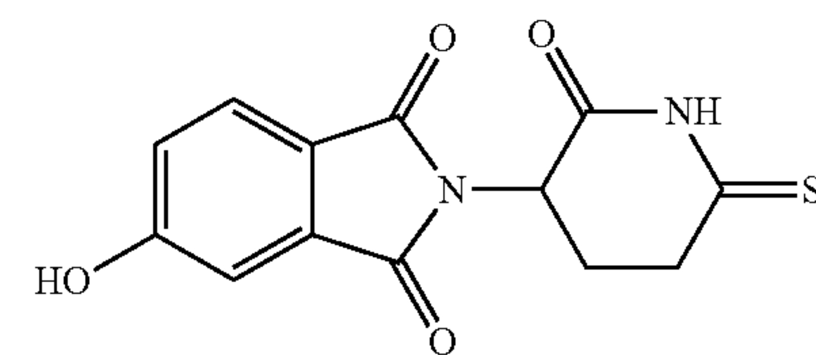
17: C 13 H 10 N 2 O 4 S MW 290.29
