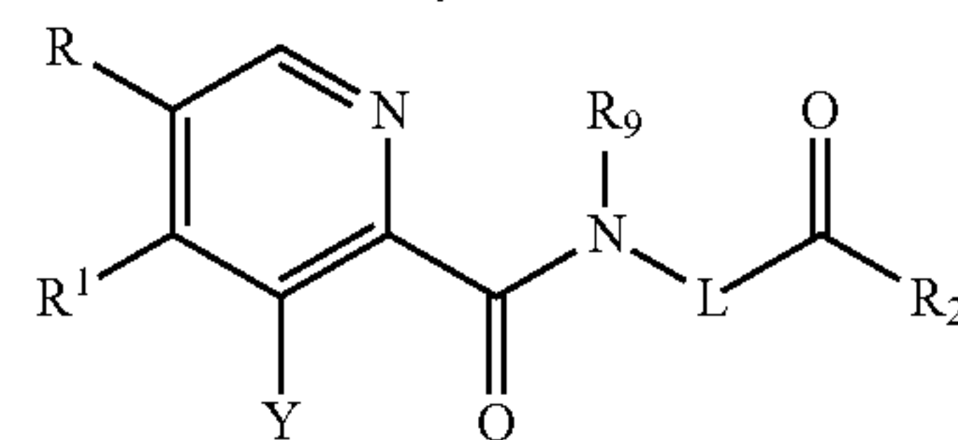
2-amidopyridines
