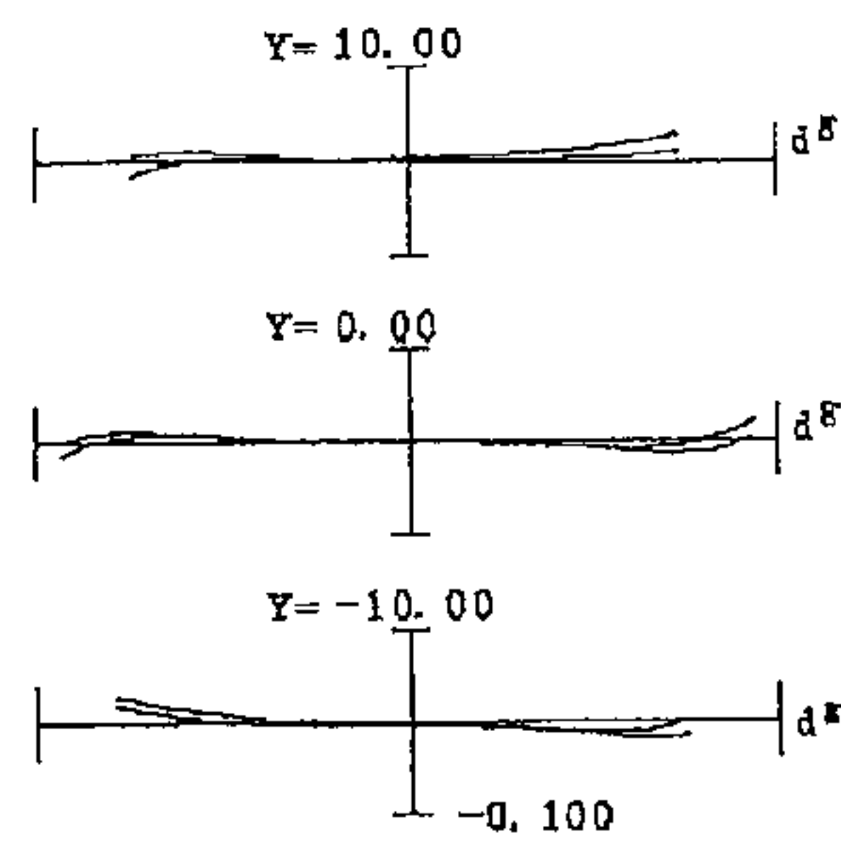
COMA ABERRATION
