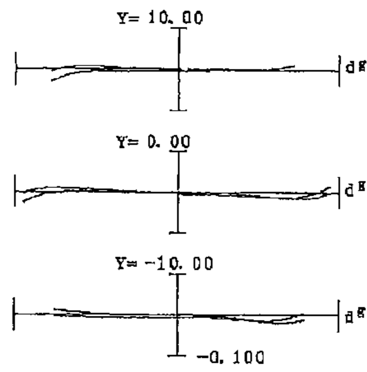
COMA ABERRATION
