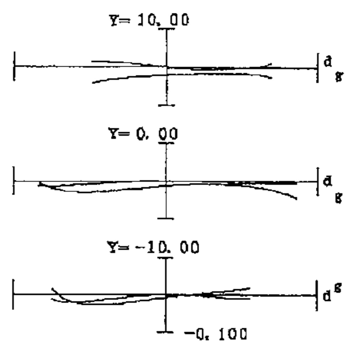
COMA ABERRATION
