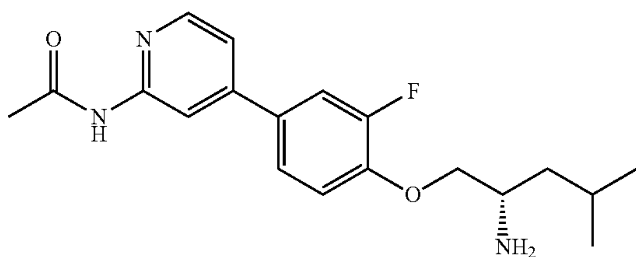
Part E: (S)—N-(4-(4-((2-amino-4-methylpentyl)oxy)-3-fluorophenyl)pyridin-2-yl)acetamide
