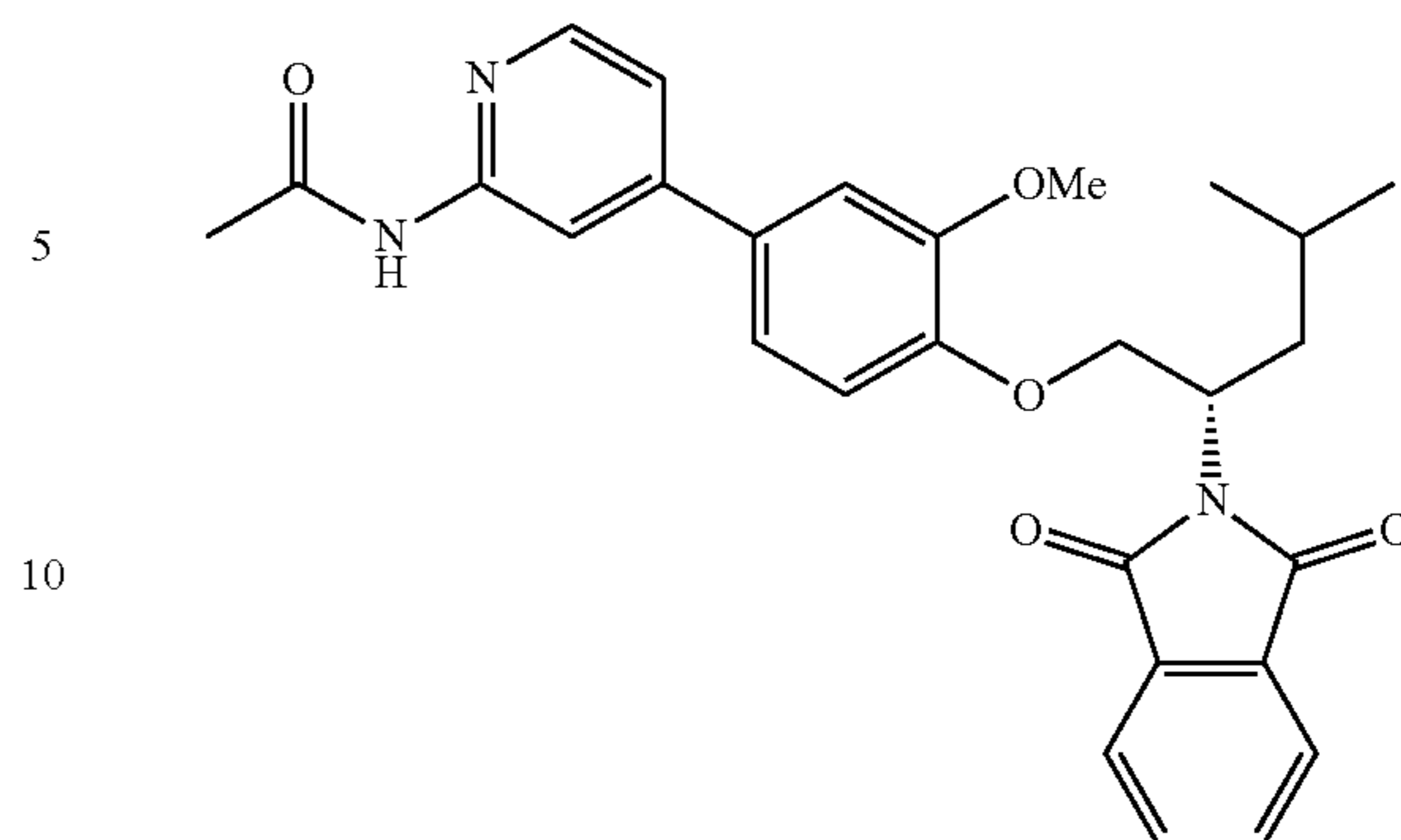
Part B: (S)—N-(4-(4-((2-(1,3-dioxisoindolin-2-yl)-4-methylpentyl)oxy)-3-methoxyphenyl)pyridin-2-yl)acetamide
