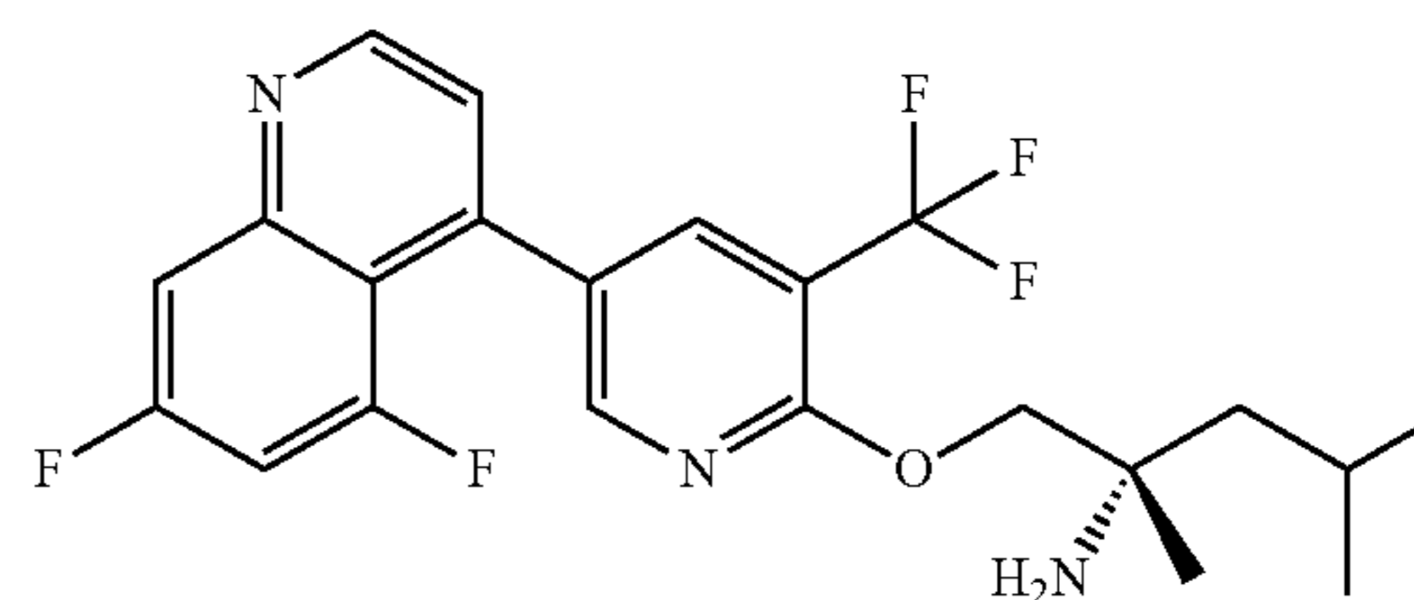
Part D: (S)-1-((5-(5,7-difluoroquinolin-4-yl)-3-(trifluoromethyl)pyridin-2-yl)oxy)-2,4-dimethylpentan-2-amine
