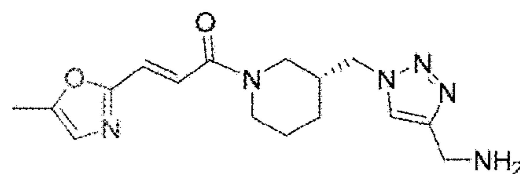
(R,E)-1-(3-((4-(aminomethyl)-1H-1,2,3-triazol-1-yl)methyl)piperidin-1-yl)-3-(5-methyloxazol-2-yl)prop-2-en-1-one
