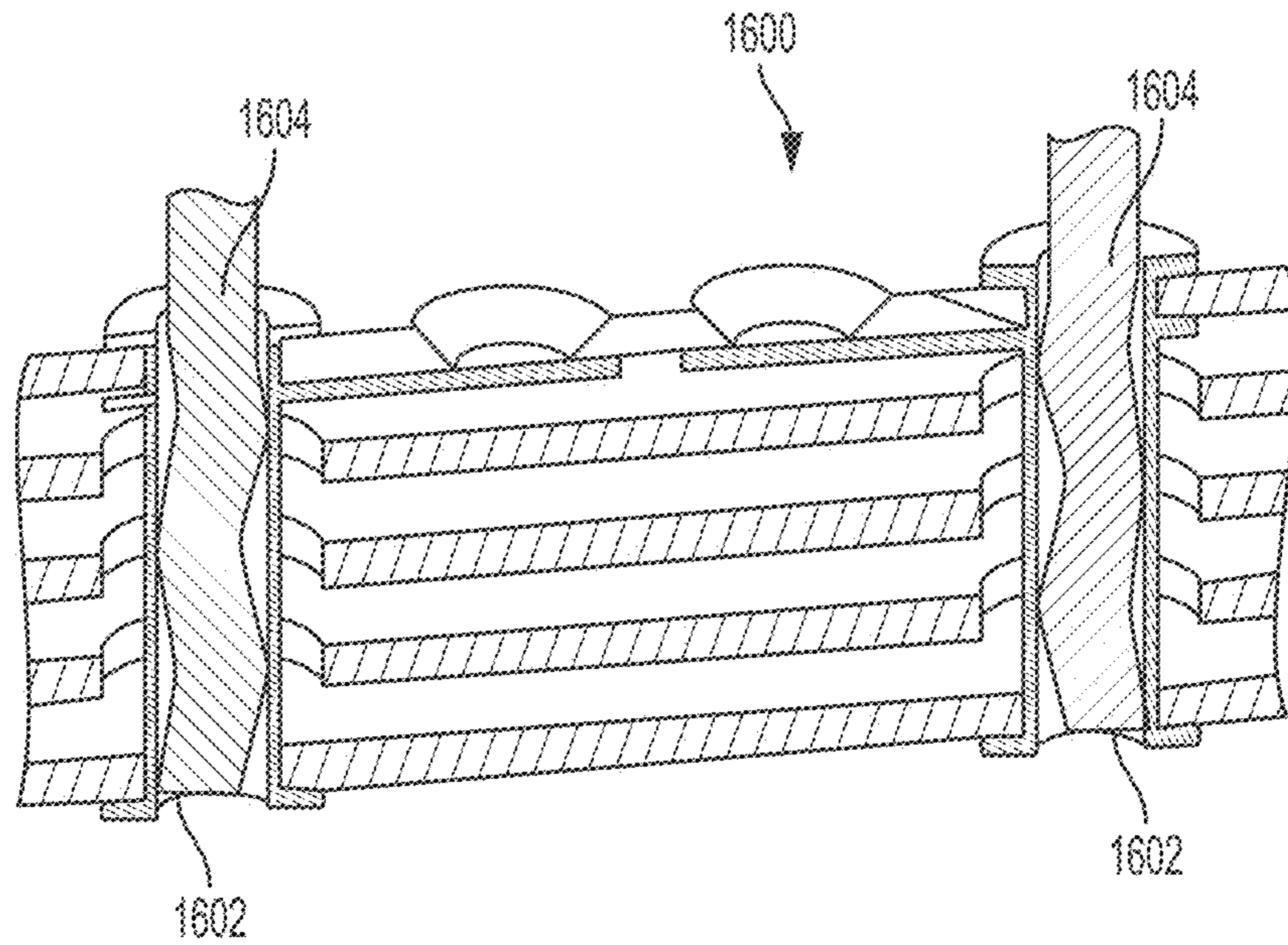
FIG. 16B
