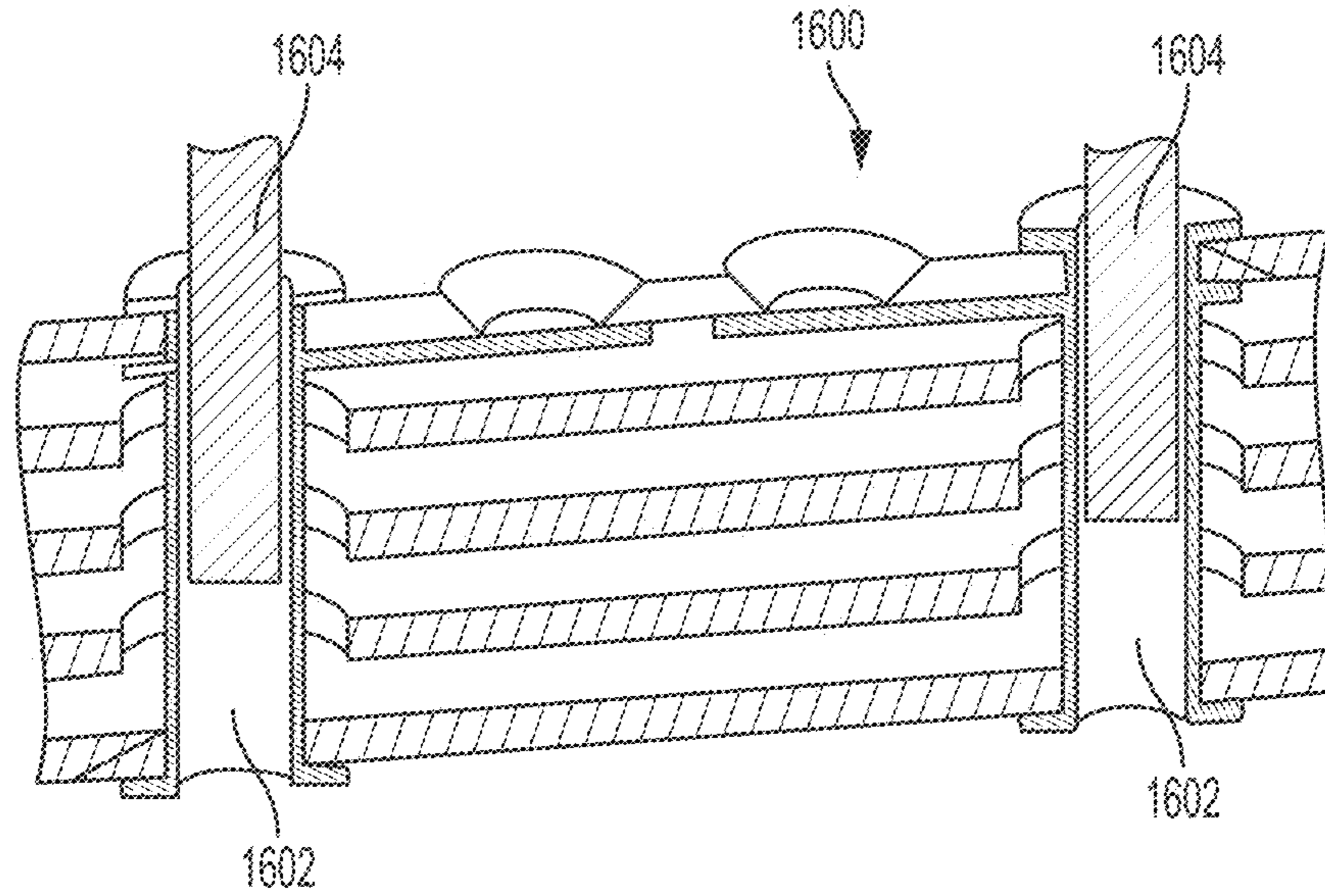
FIG. 16A
