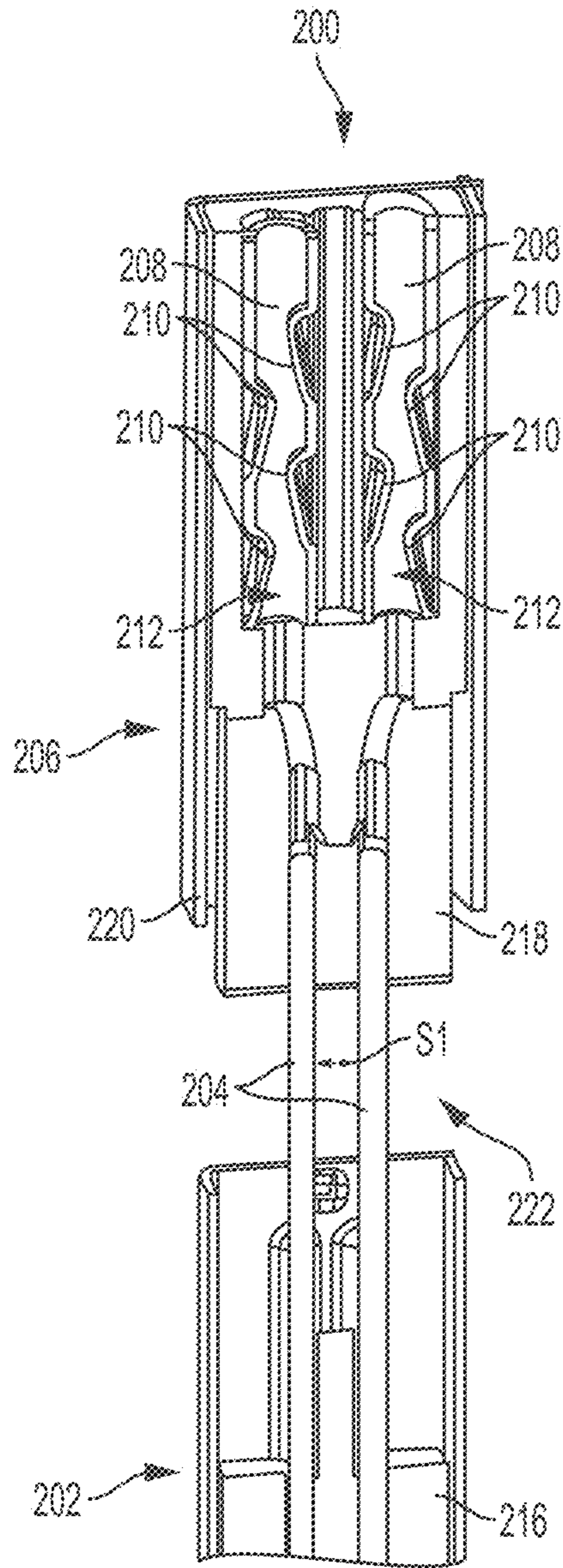
FIG. 2A
