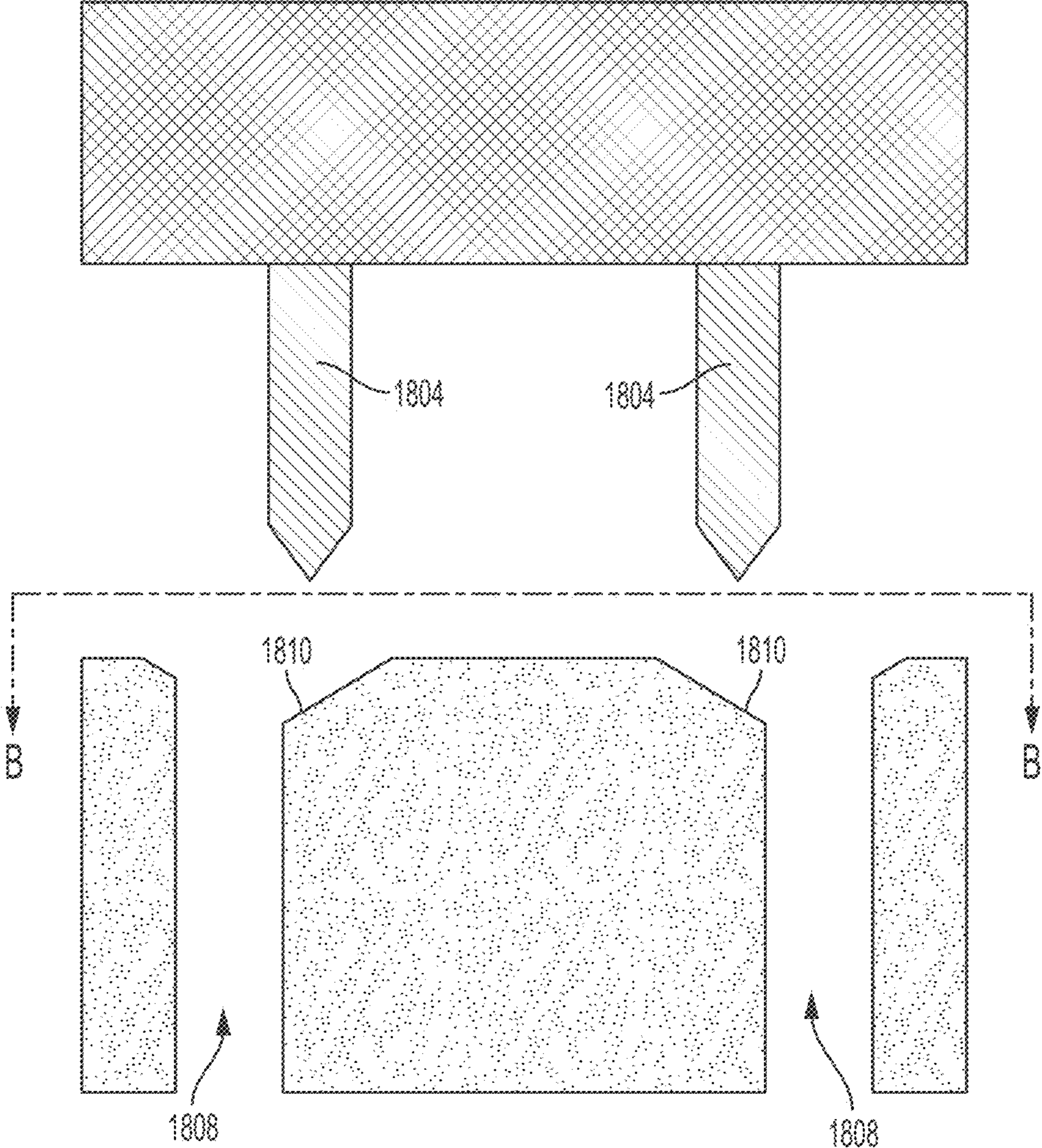
FIG. 18A
