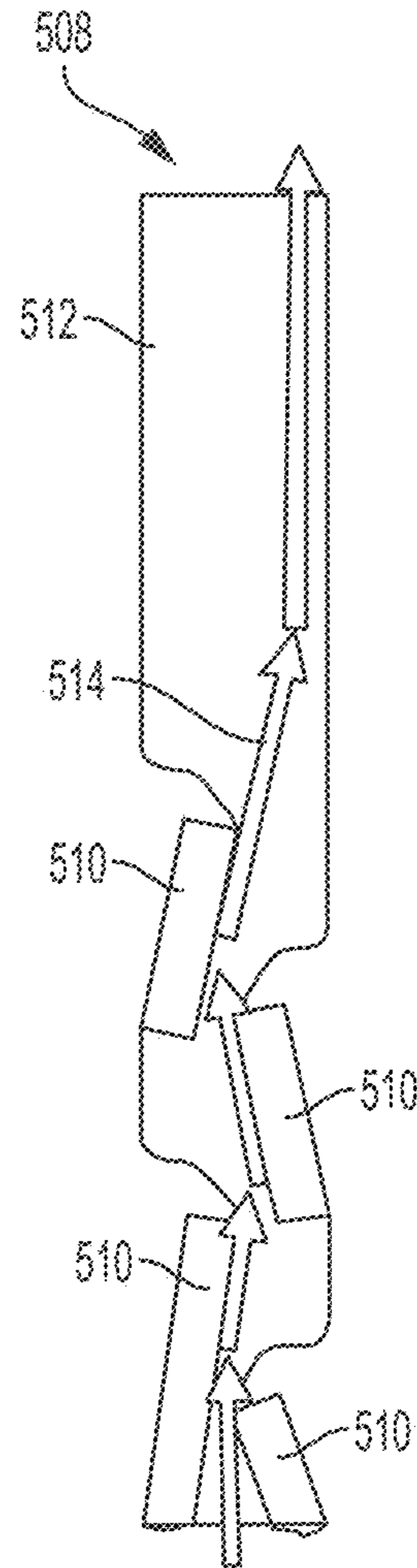
FIG. 5B
