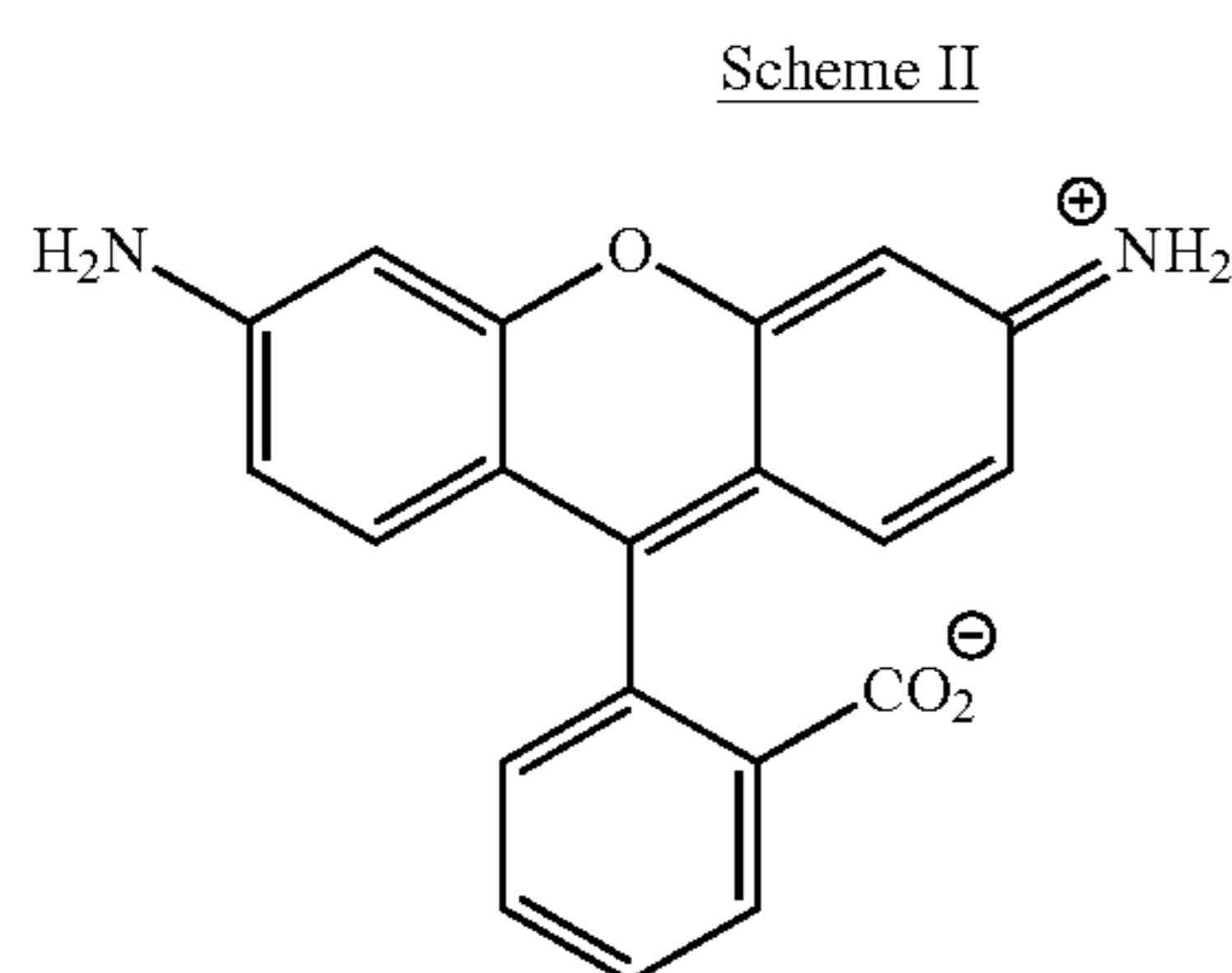
Rhodamine 110
