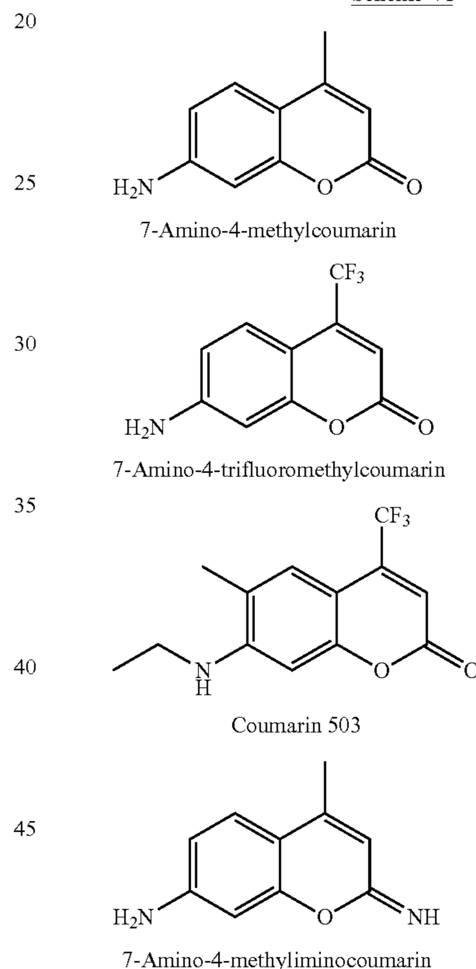
Scheme VI
