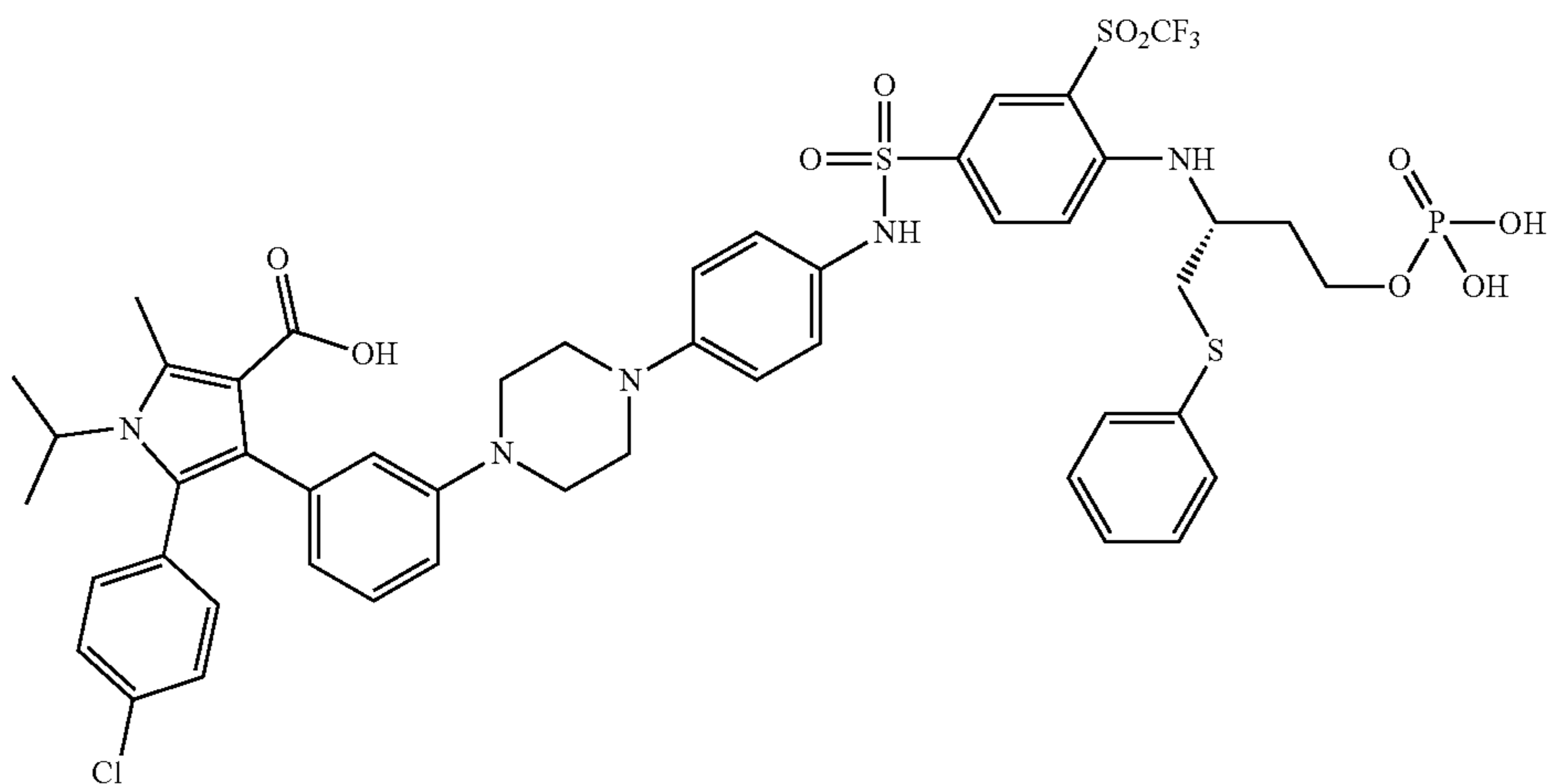
(R)-5-(4-chlorophenyl)-1-isopropyl-2-methyl-4-(3-(4-(4-((1-(phenylthio)-4-(phosphonooxy)butan-2-yl)amino)-3-((trifluoromethyl)sulfonyl)phenyl)sulfonamido)phenyl)piperazin-1-yl)phenyl)-1H-pyrrole-3-carboxylic acid
