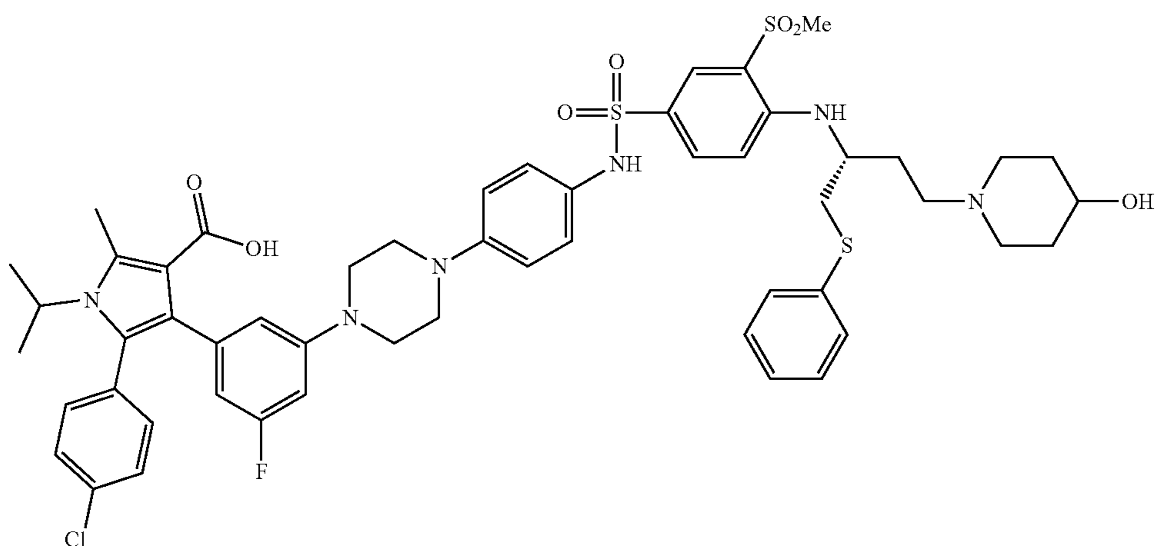
(R)-5-(4-chlorophenyl)-4-(3-fluoro-5-(4-(4-((4-(4-hydroxypiperidin-1-yl)-1-(phenylthio)butan-2-yl)amino)-3-(methylsulfonyl)phenyl)sulfonamido)phenyl)piperazin-1-yl)phenyl)-1-isopropyl-2-methyl-1H-pyrrole-3-carboxylic acid
