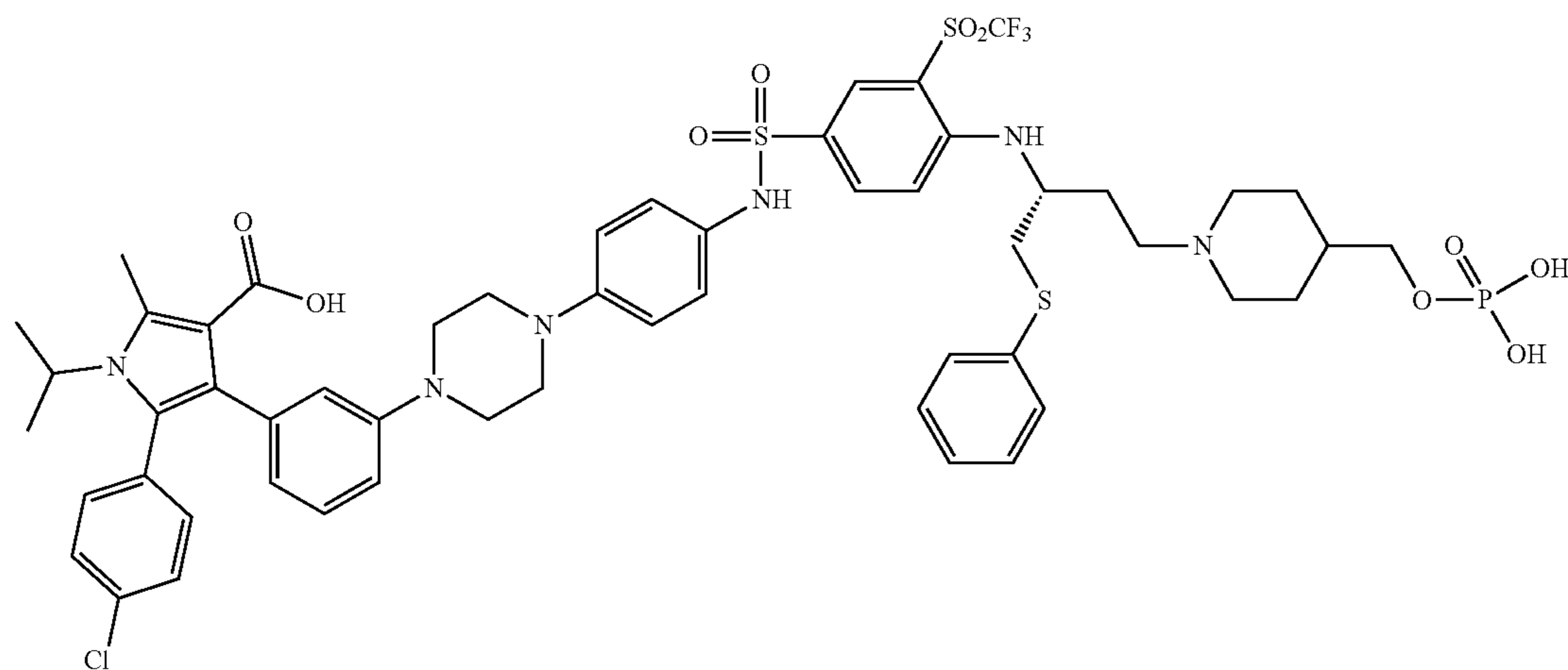
(R)-5-(4-chlorophenyl)-1-isopropyl-2-methyl-4-(3-(4-(4-((1-(phenylthio)-4-(4-((phosphonooxy)methyl)piperidin-1-yl)butan-2-yl)amino)-3-((trifluoromethyl)sulfonyl)phenyl)sulfonamido)phenyl)piperazin-1-yl)phenyl)-1H-pyrrole-3-carboxylic acid
