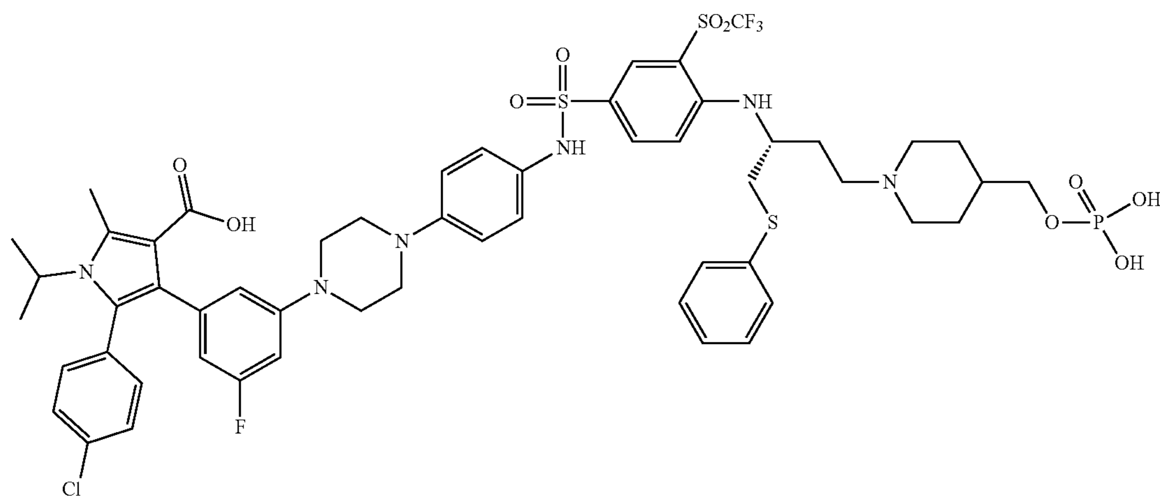
(R)-5-(4-chlorophenyl)-4-(3-fluoro-5-(4-(4-((1-(phenylthio)-4-(4-((phosphonooxy)methyl)piperidin-1-yl)butan-2-yl)amino)-3-((trifluoromethyl)sulfonyl)phenyl)sulfonamido)phenyl)piperazin-1-yl)phenyl)-1-isopropyl-2-methyl-1H-pyrrole-3-carboxylic acid
