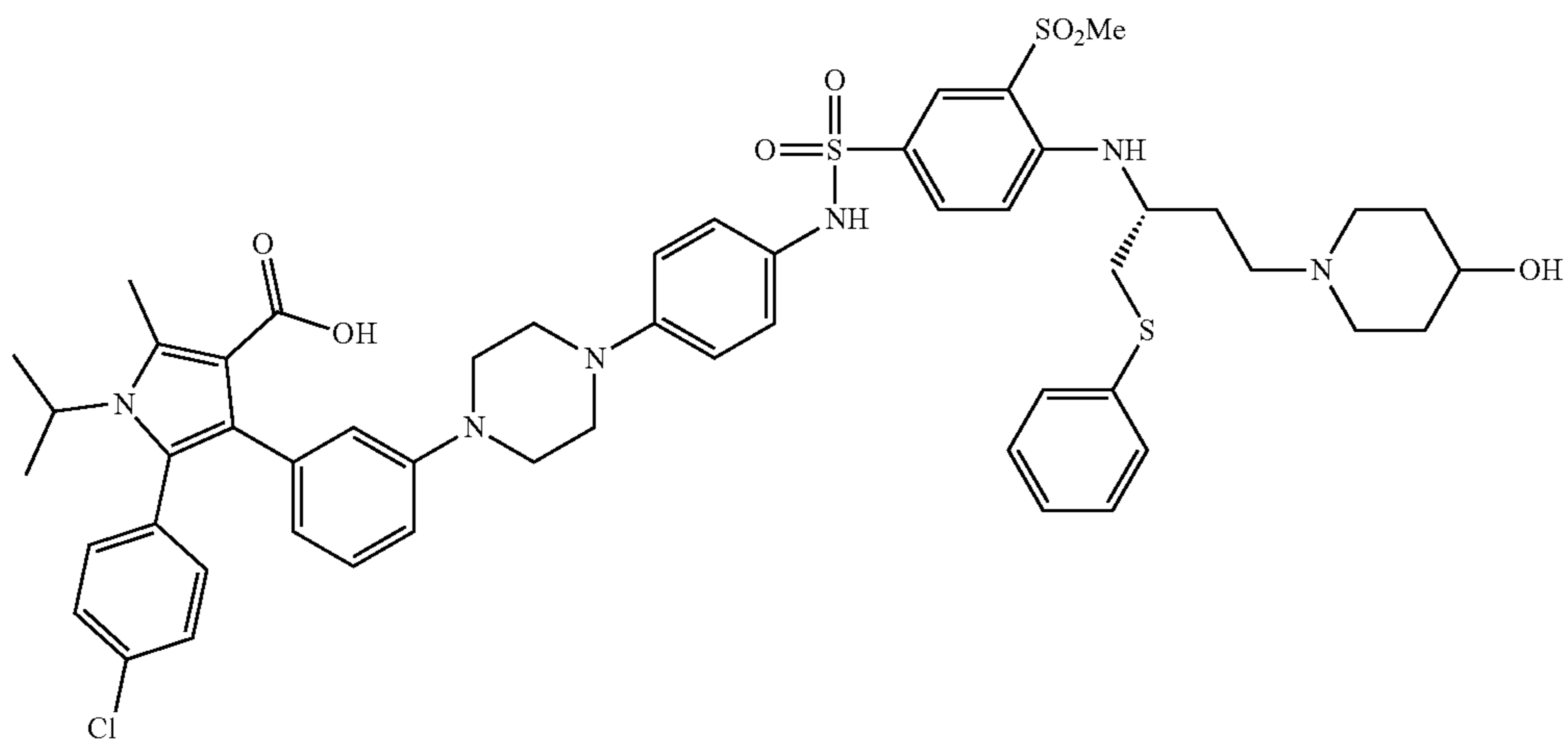
(R)-5-(4-chlorophenyl)-4-(3-(4-(4-((4-(4-hydroxypiperidin-1-yl)-1-(phenylthio)butan-2-yl)amino)-3-(methylsulfonyl)phenyl)sulfonamido)phenyl)piperazin-1-yl)phenyl)-1-isopropyl-2-methyl-1H-pyrrole-3-carboxylic acid
