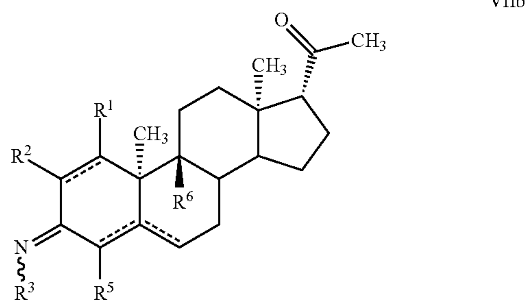
VIIb
