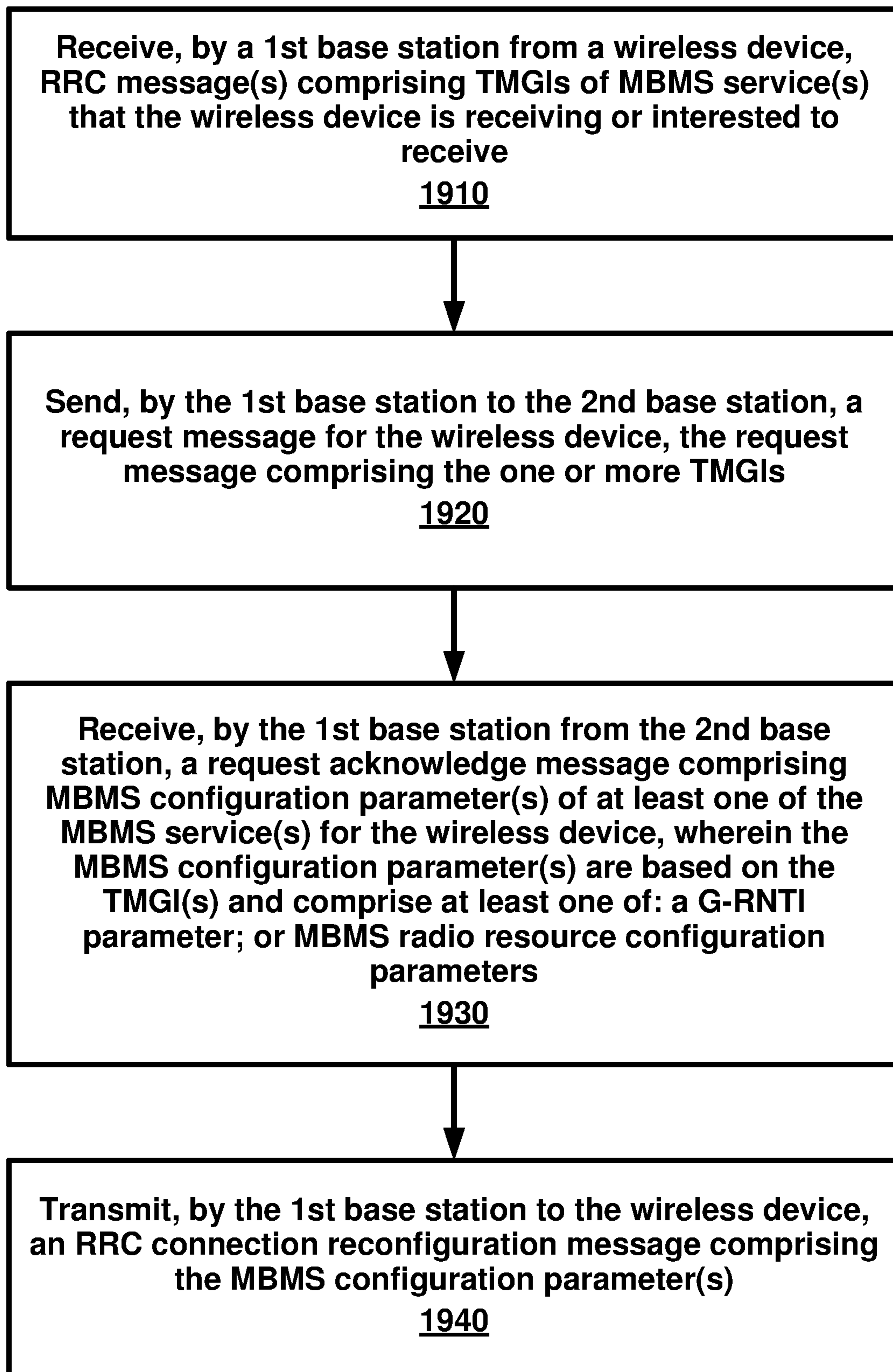
FIG. 19
