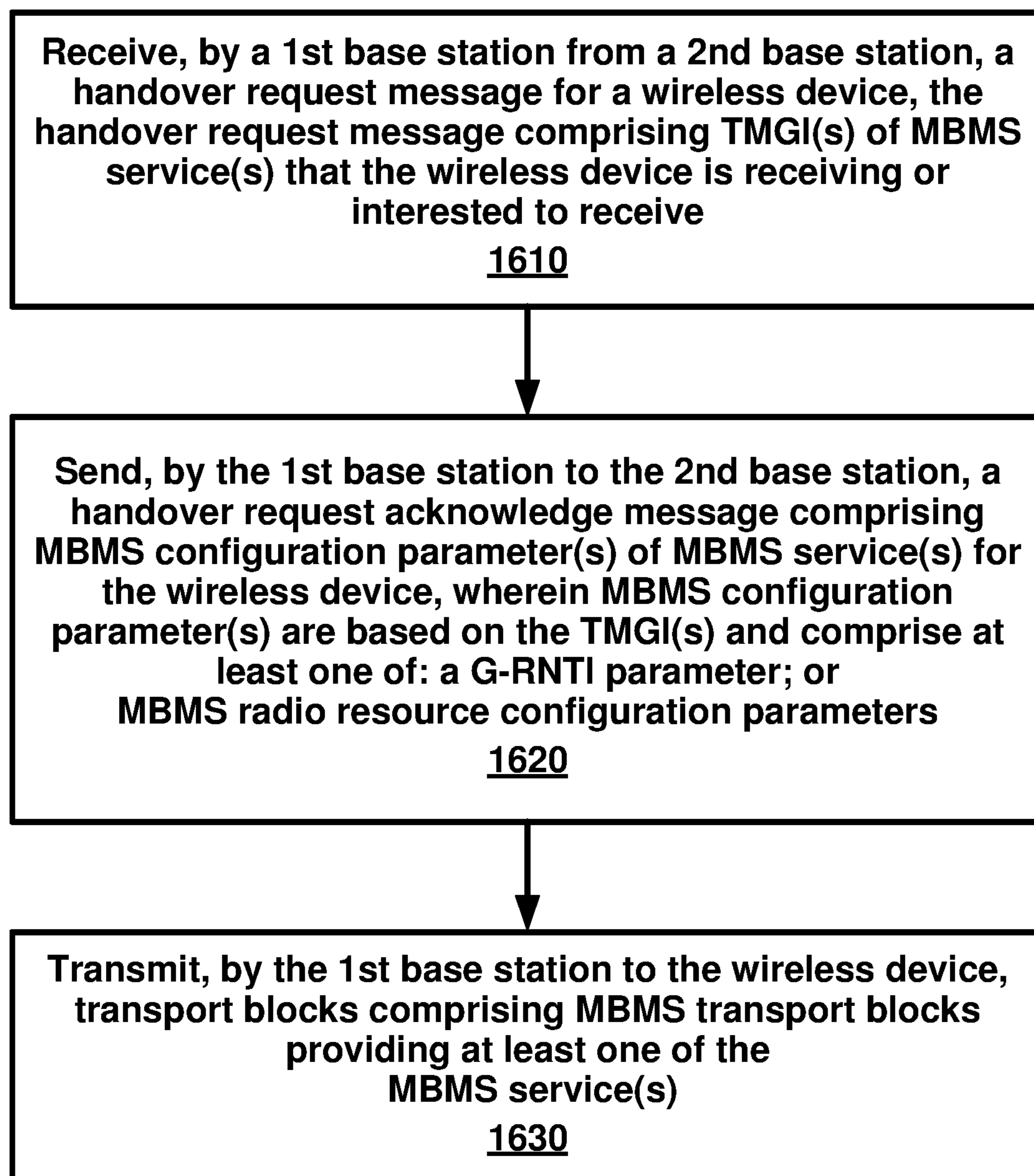
FIG. 16
