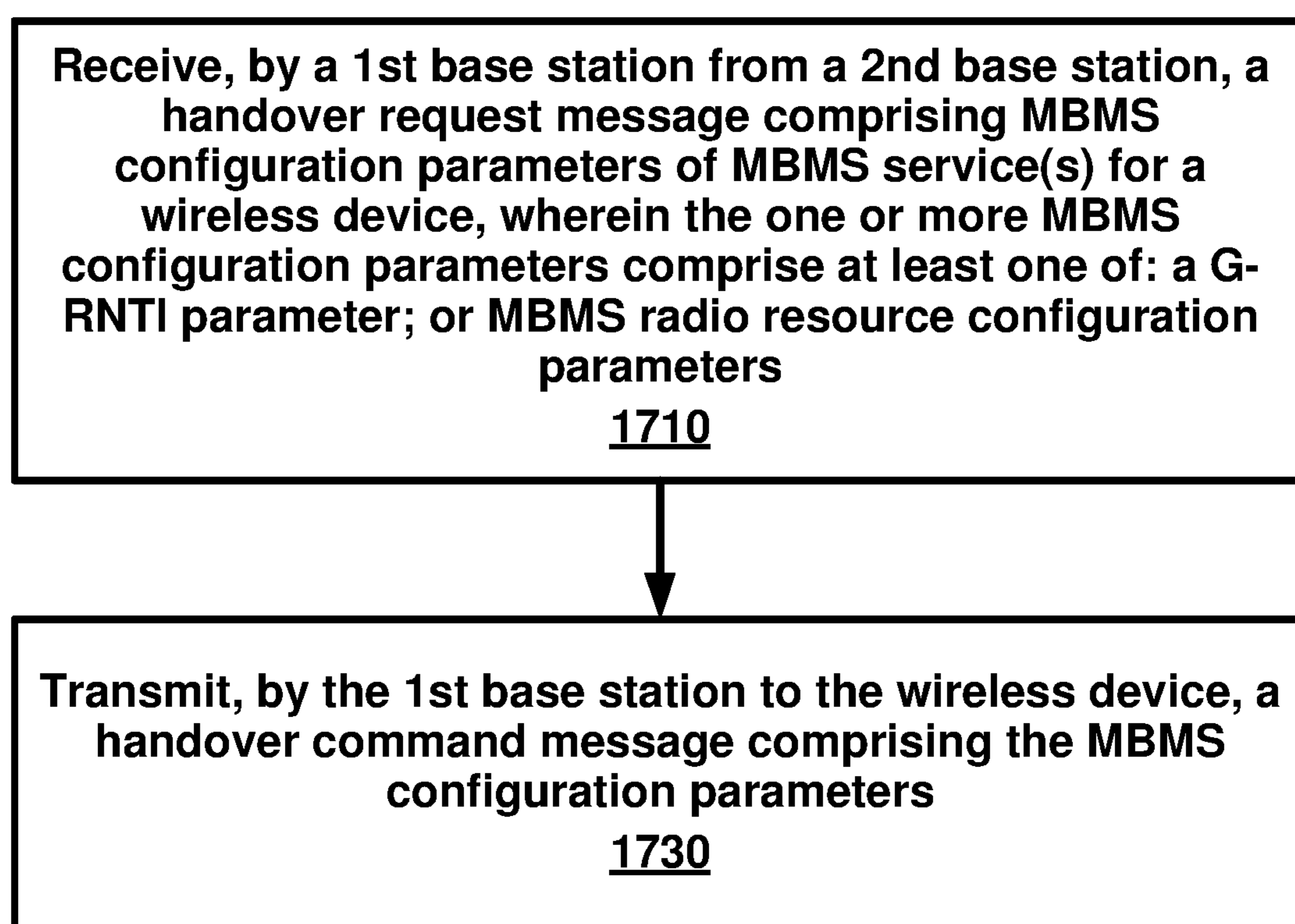
FIG. 17
