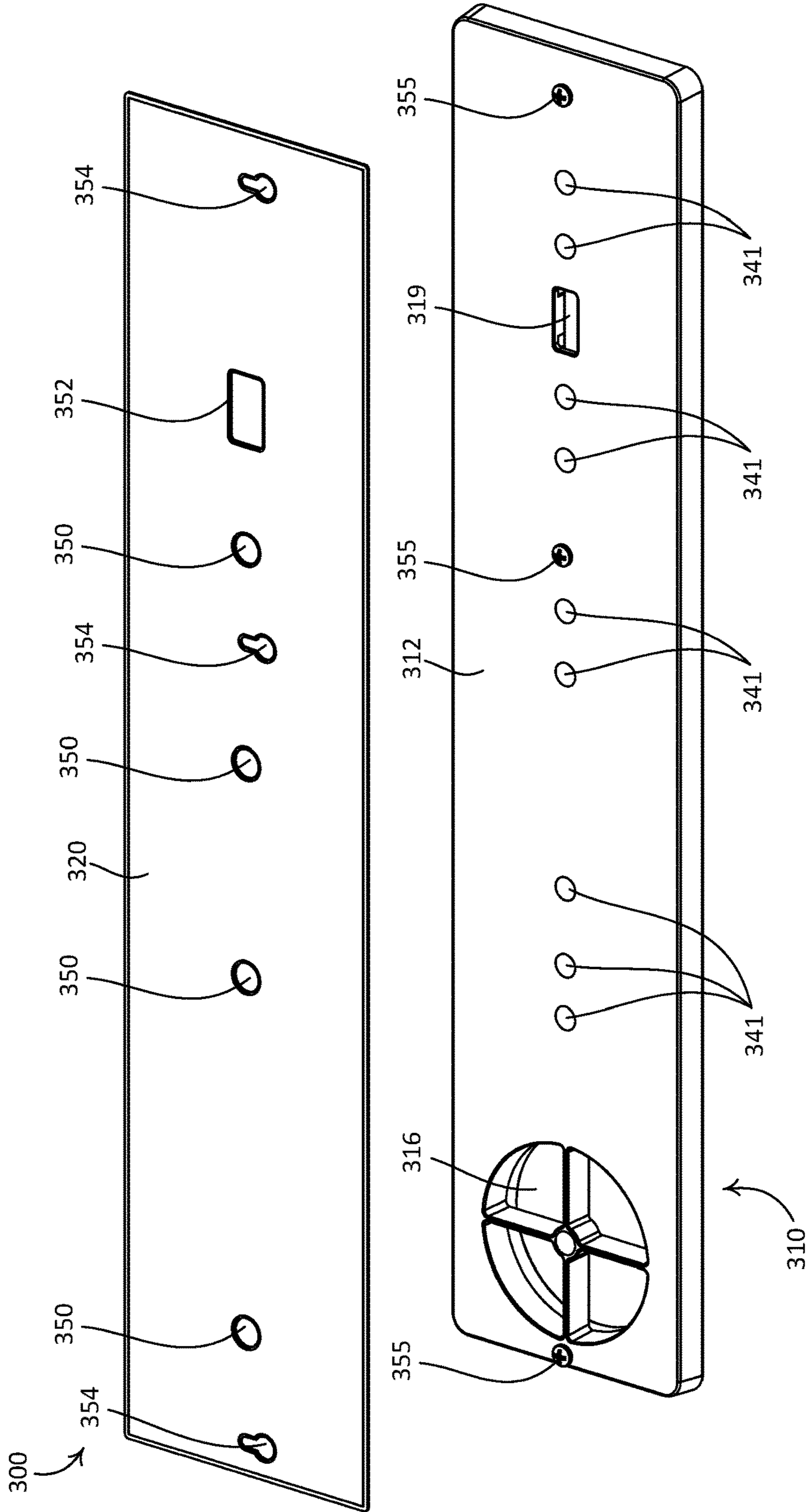
FIG. 3C
