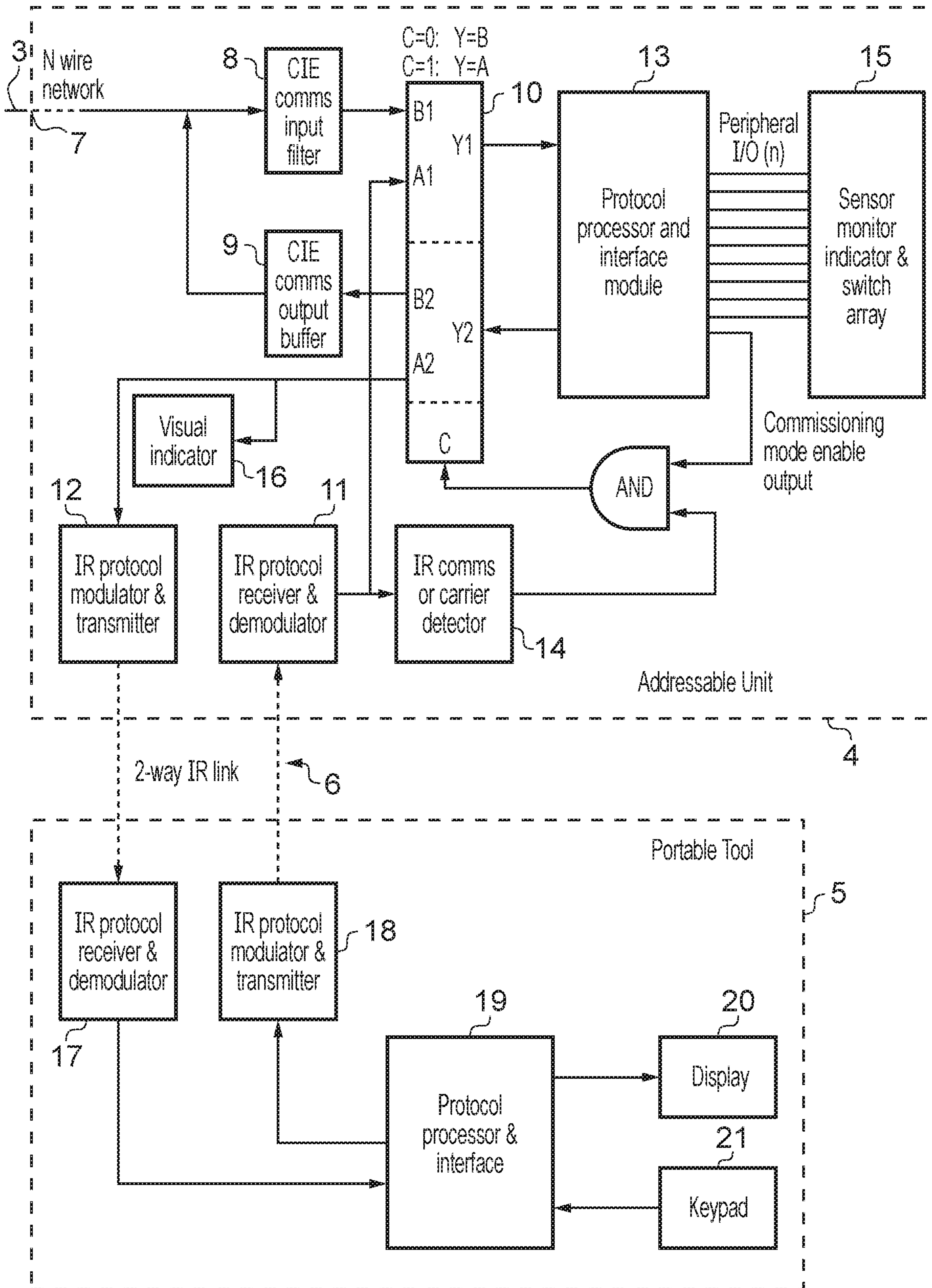
Block diagram of IR link modules
