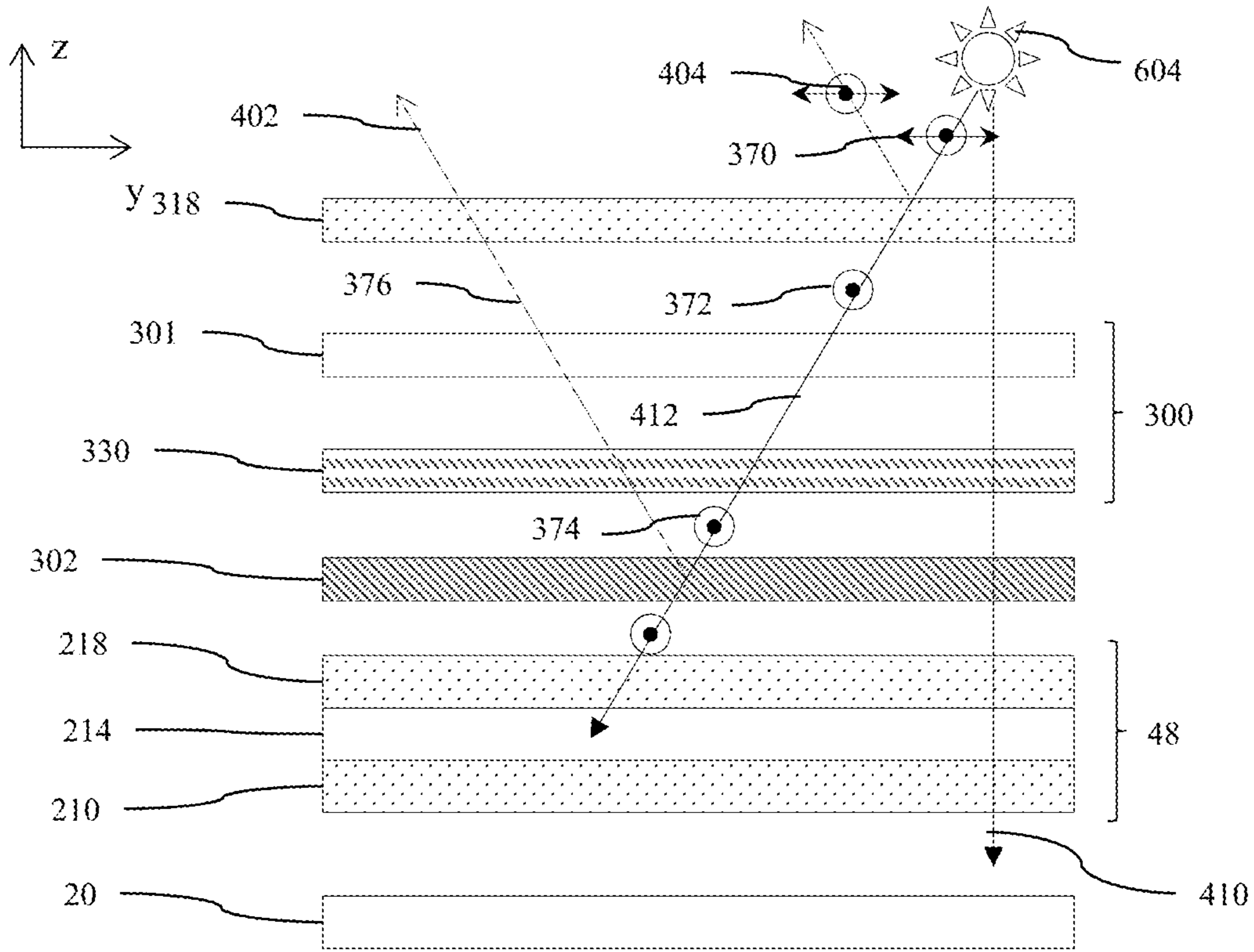
FIG. 9D Reflectivity
