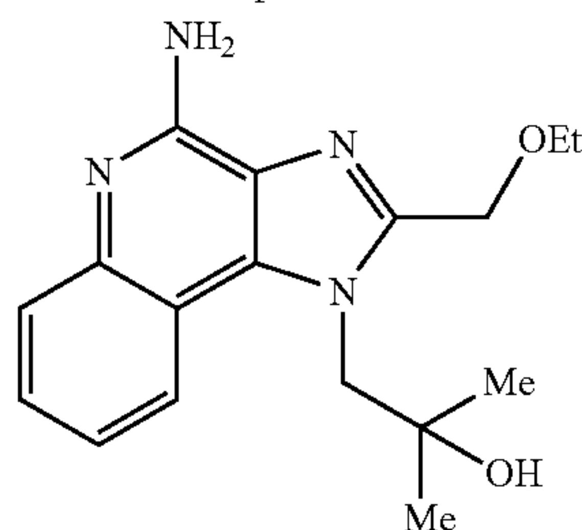
Resiquimod
