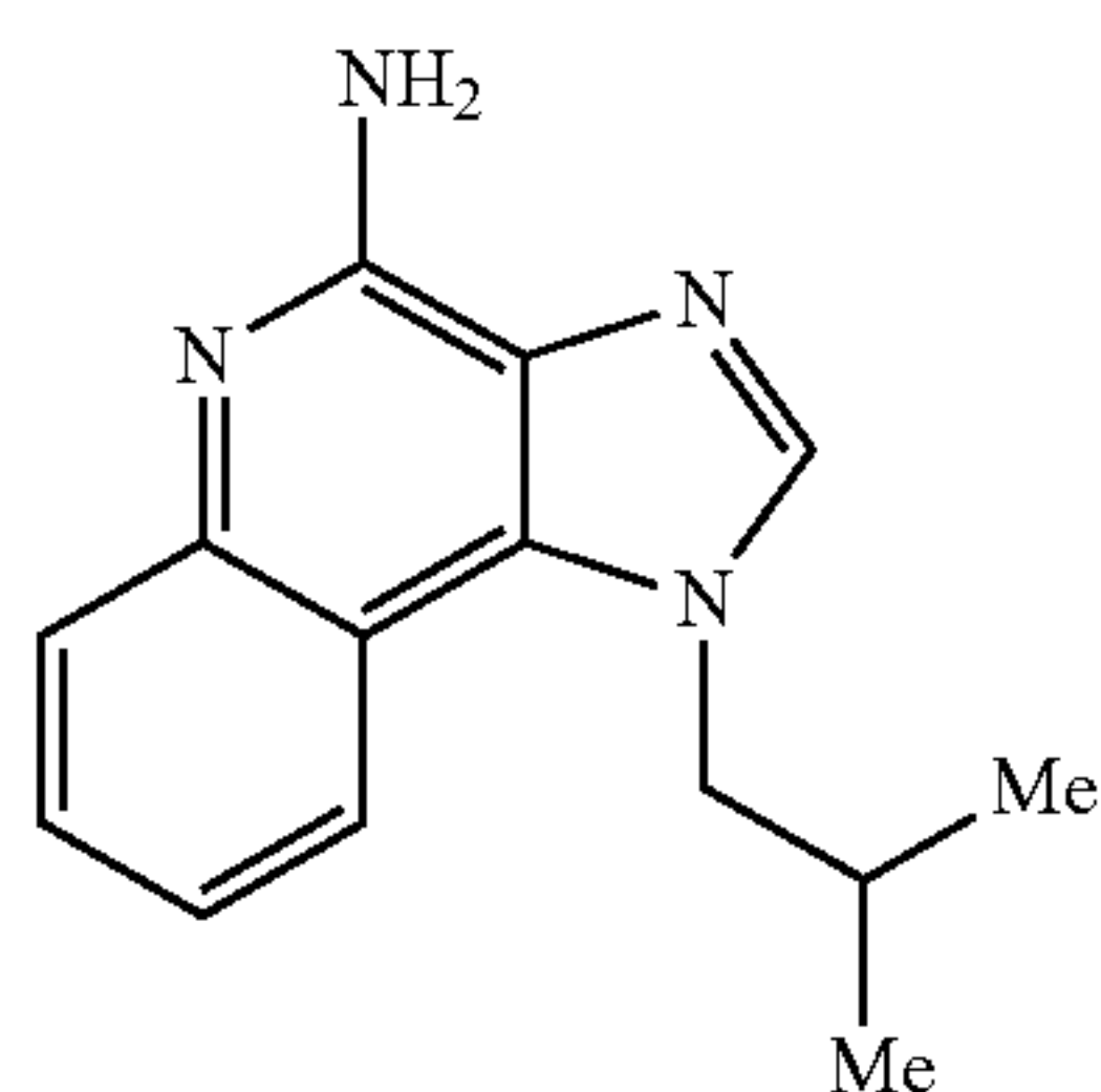
Imiquimod
