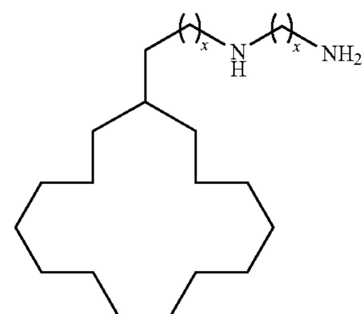
x = 3; 3HCl (MotuCH 2 CH 2 33)
