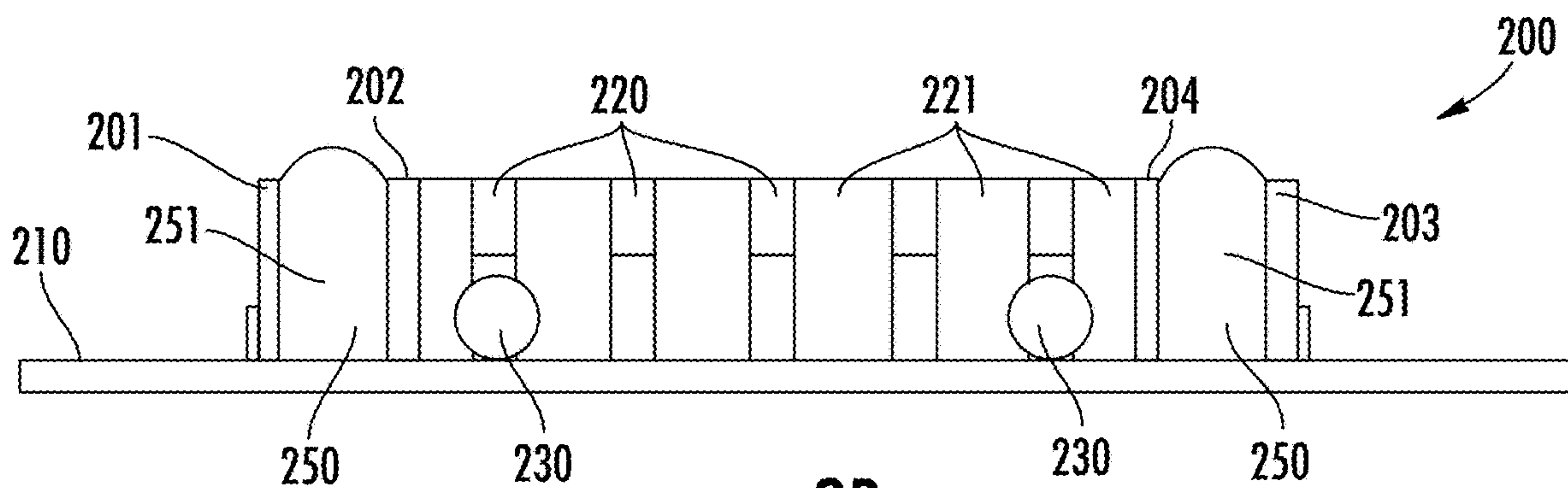
FIG. 2B
