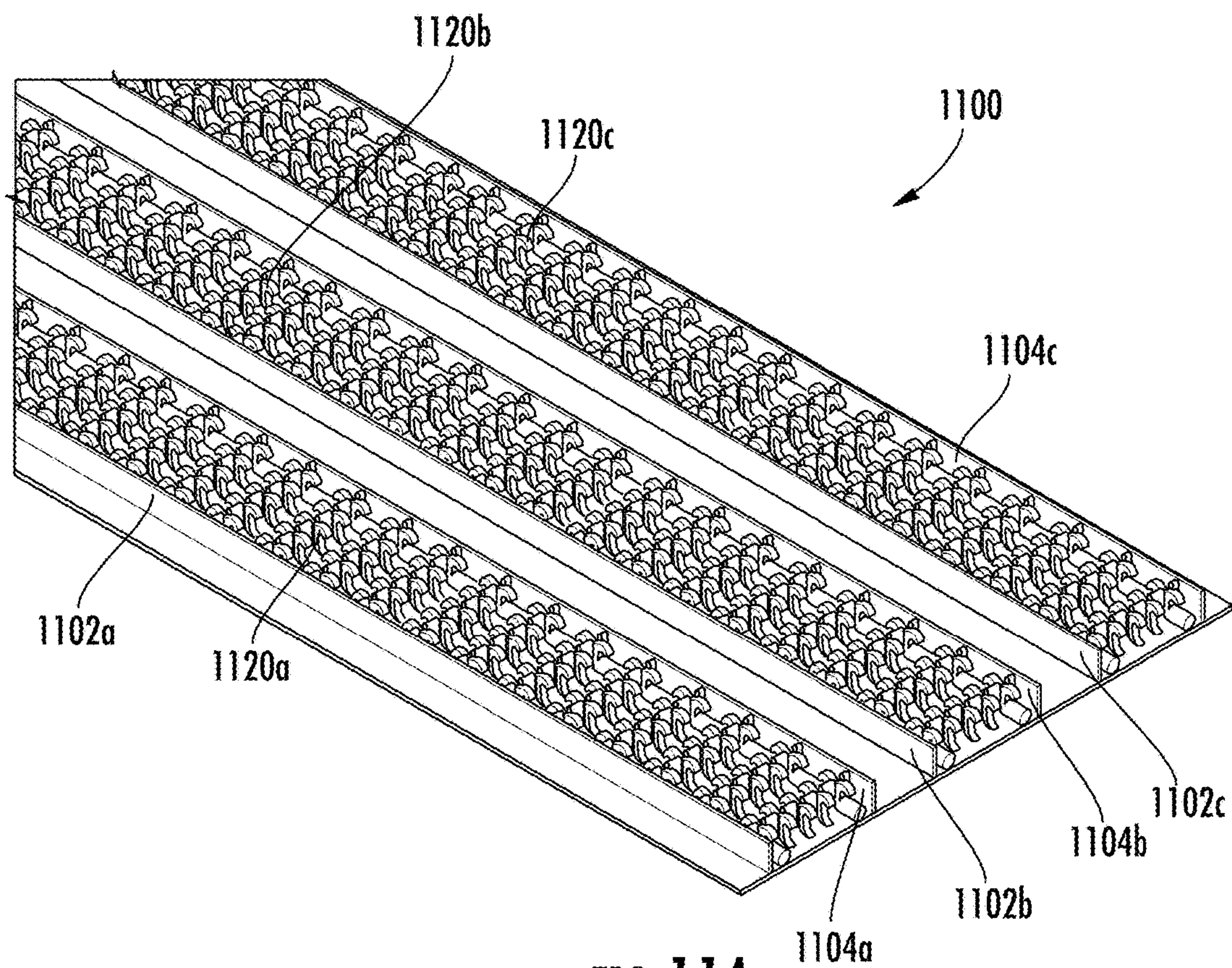
FIG. 11A
