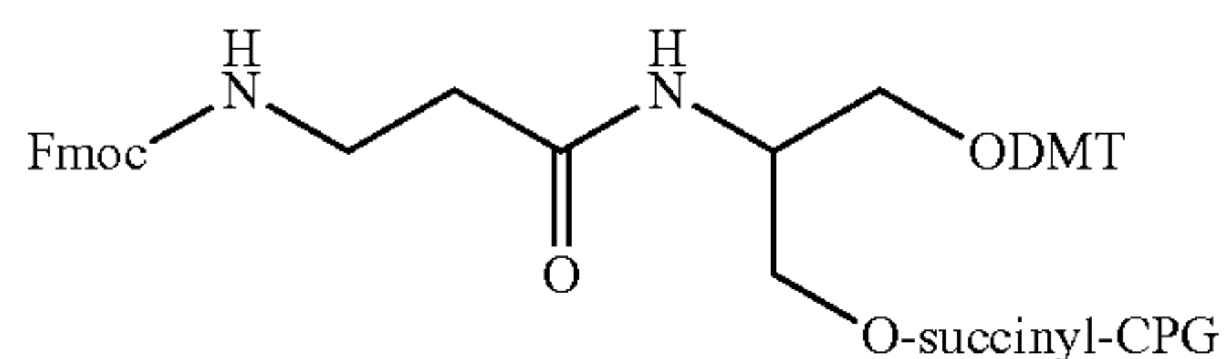
3'-Amino-Modifier Serinol CPG
