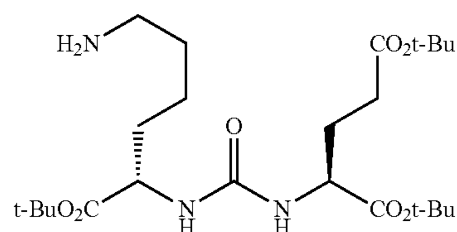
(S)-di-tert-butyl 2-(3-((S)-6-amino-1-tert-butoxy-1-oxohexan-2-yl)ureido)pentanedioate (12)
