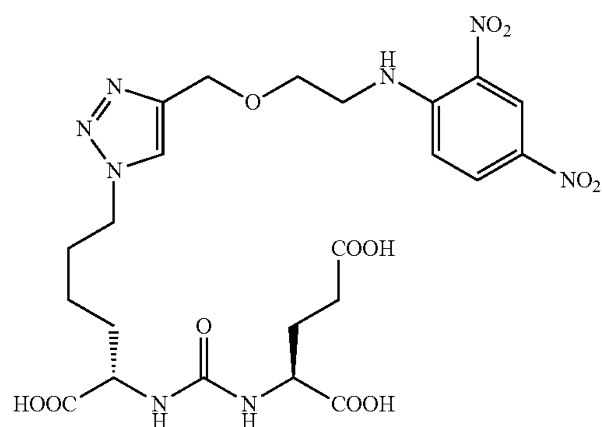
(S)-2-(3-((S)-1-carboxy-5-(4-((2-(2,4-dinitrophenylamino)ethoxy)methyl)-1H-1,2,3-triazol-1-yl)pentyl)ureido)pentanedioic acid (2)
