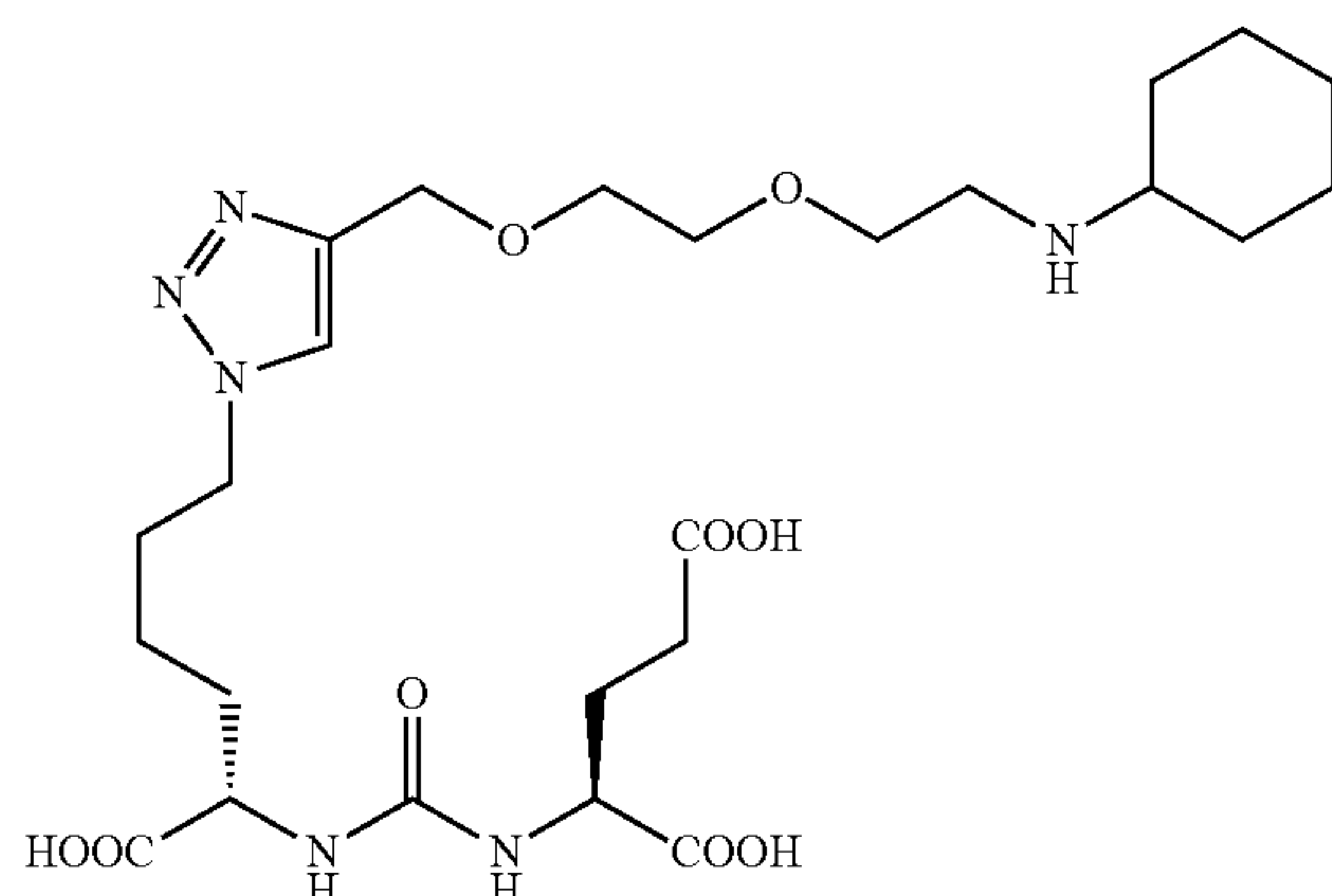
(S)-2-(3-((S)-1-carboxy-5-(4-((2-(2-(cyclohexylamino)ethoxy)ethoxy)methyl)-1H-1,2,3-triazol-1-yl)pentyl)ureido)pentanedioic acid (17)
