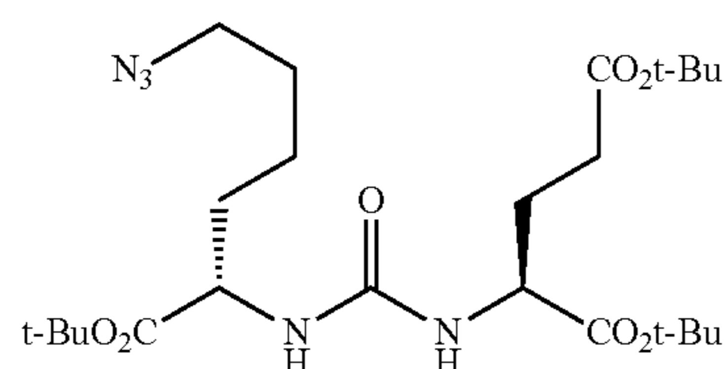
(S)-di-tert-butyl 2-(3-((S)-6-azido-1-tert-butoxy-1-oxohexan-2-yl)ureido)pentanedioate (14)
