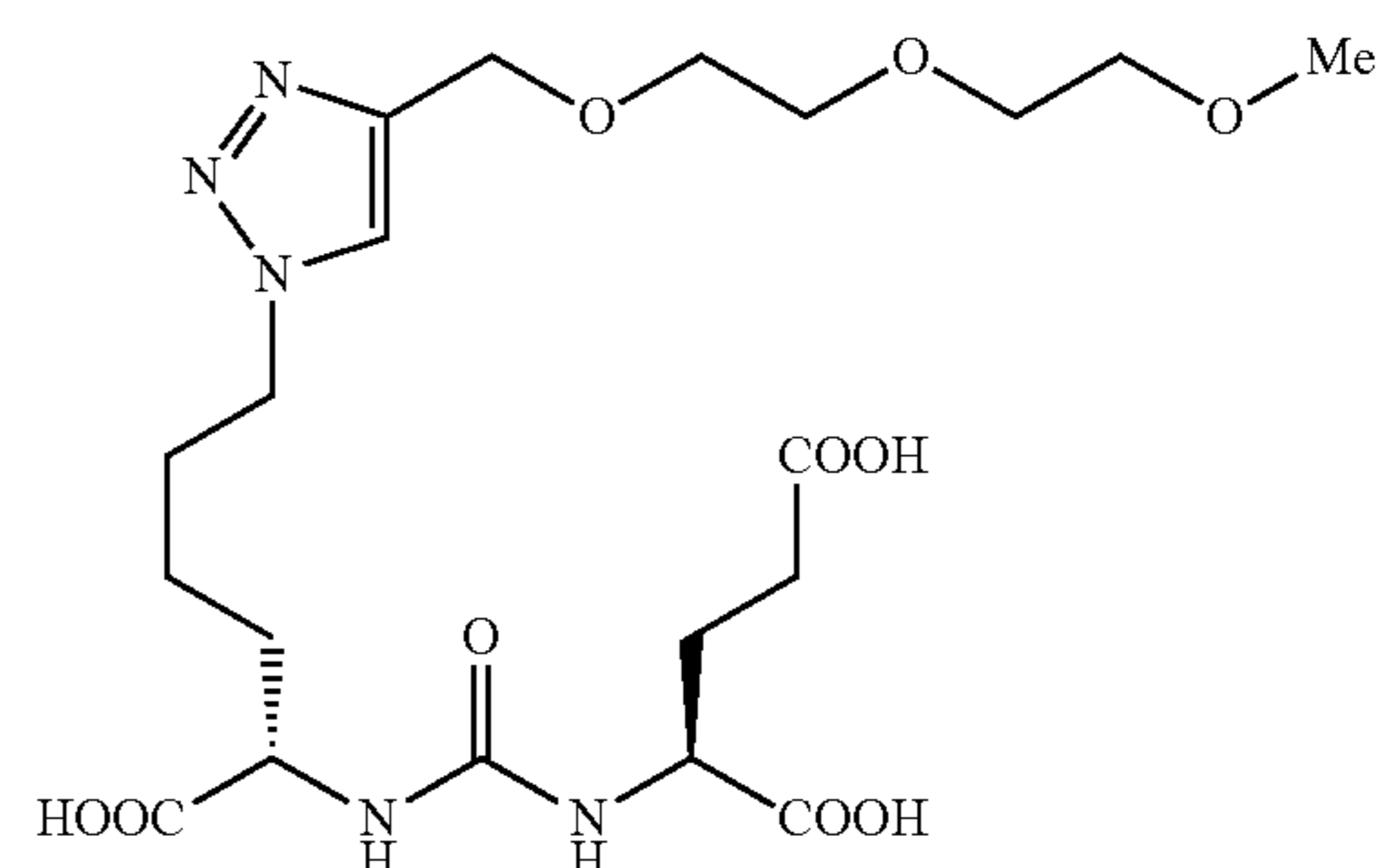
(S)-2-(3-((S)-1-carboxy-5-(4-((2-(2-methoxyethoxy)ethoxy)methyl)-1H-1,2,3-triazol-1-yl)pentyl)ureido)pentanedioic acid (9)
