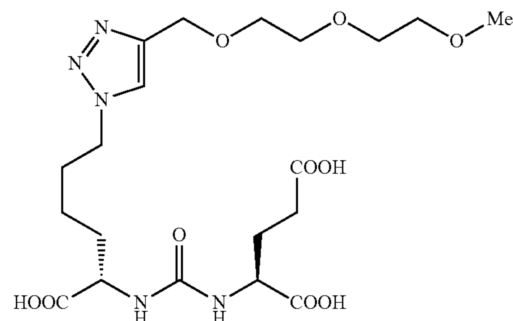
(S)-2-(3-((S)-1-carboxy-5-(4-((2-(2-methoxyethoxy)ethoxy)methyl)-1H-1,2,3-triazol-1-yl)pentyl)ureido)pentanedioic acid (9)
