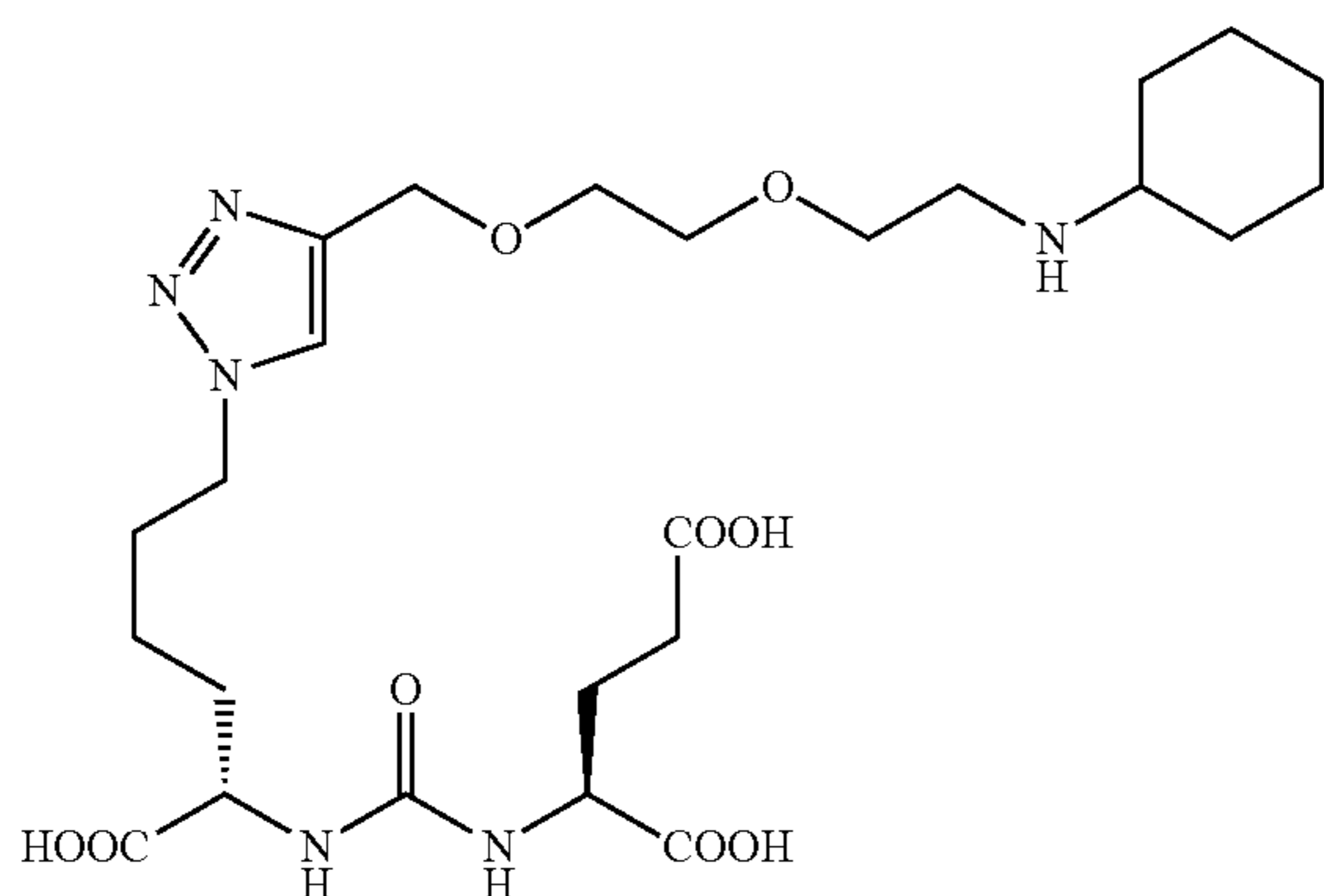
(S)-2-(3-((S)-1-carboxy-5-(4-(2-(2-(cyclohexylamino)ethoxy)ethoxy)methyl)-1H-1,2,3-triazol-1-yl)pentyl)ureido)pentanedioic acid (17)
