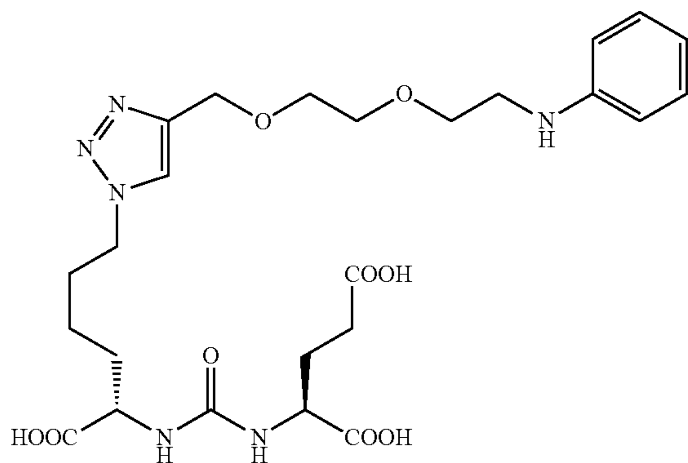
(S)-2-(3-((S)-1-carboxy-5-(4-((2-(2-(phenylamino)ethoxy)ethoxy)methyl)-1H-1,2,3-triazol-1-yl)pentyl)ureido)pentanedioic acid (15)
