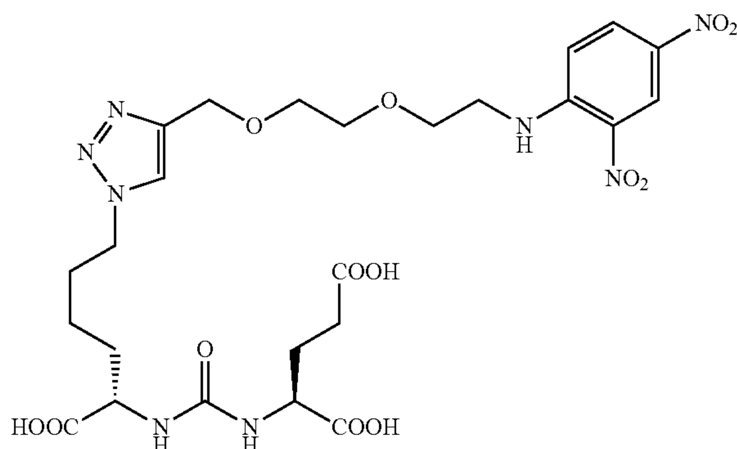
(S)-2-(3-((S)-1-carboxy-5-(4-((2-(2-(2,4-dinitrophenylamino)ethoxy)ethoxy)methyl)-1H-1,2,3-triazol-1-yl)pentyl)ureido)pentanedioic acid (3)
