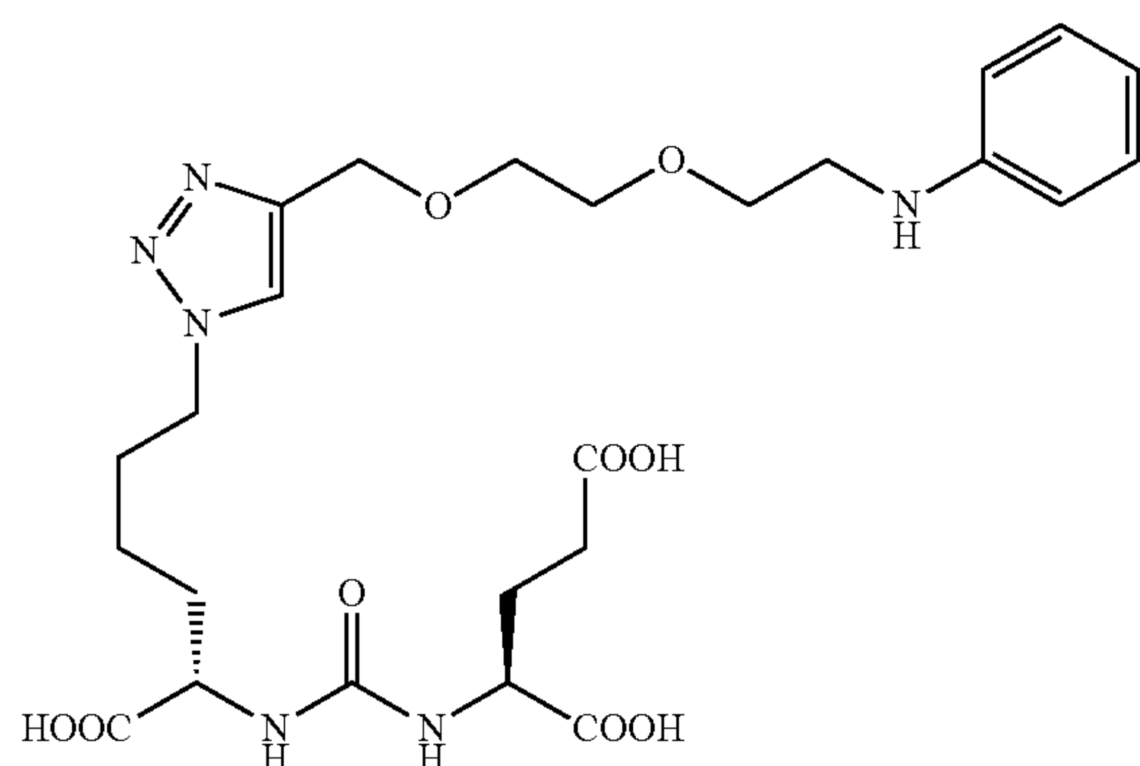
(S)-2-(3-((S)-1-carboxy-5-(4-((2-(2-(phenylamino)ethoxy)ethoxy)methyl)-1H-1,2,3-triazol-1-yl)pentyl)ureido)pentanedioic acid (15)
