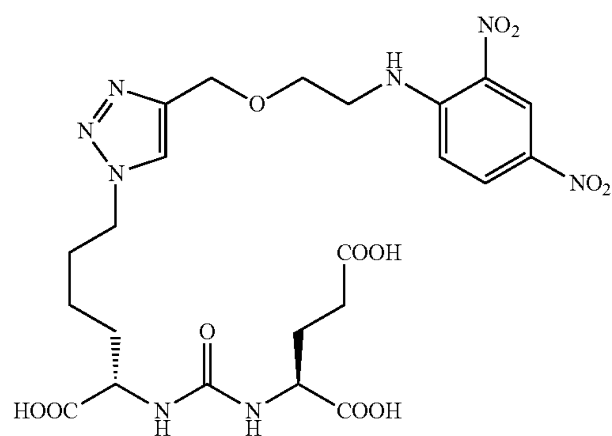
(S)-2-(3-((S)-1-carboxy-5-(4-((2-(2,4-dinitrophenylamino)ethoxy)methyl)-1H-1,2,3-triazol-1-yl)pentyl)ureido)pentanedioic acid (2)
