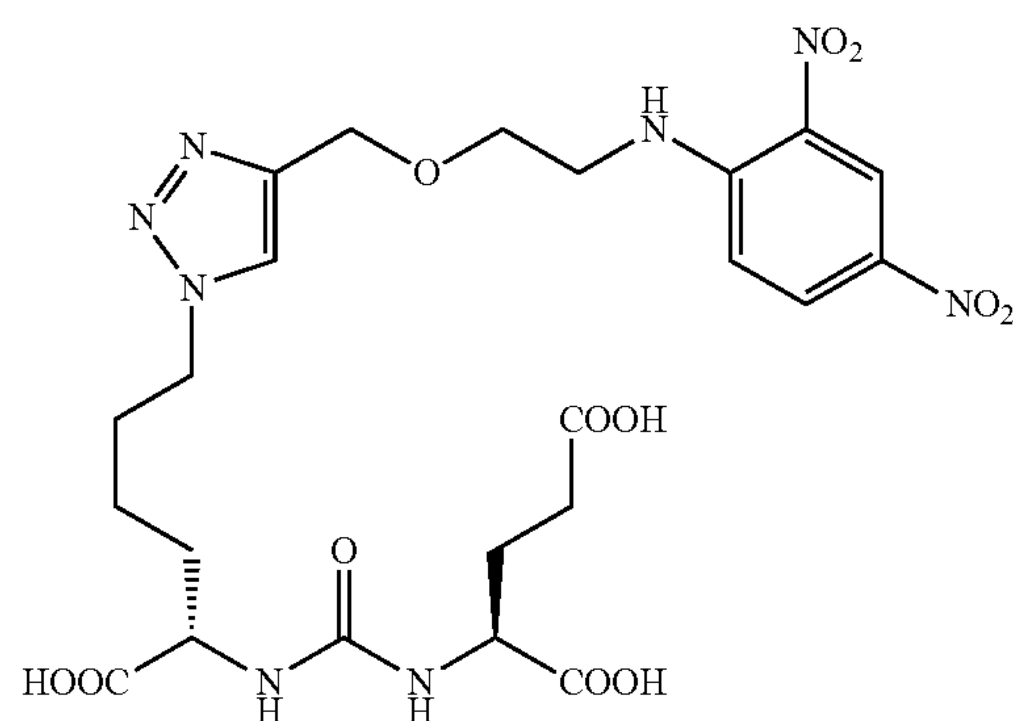
(S)-2-(3-((S)-1-carboxy-5-(4-((2-(2,4-dinitrophenylamino)ethoxy)methyl)-1H-1,2,3-triazol-1-yl)pentyl)ureido)pentanedioic acid (2)
