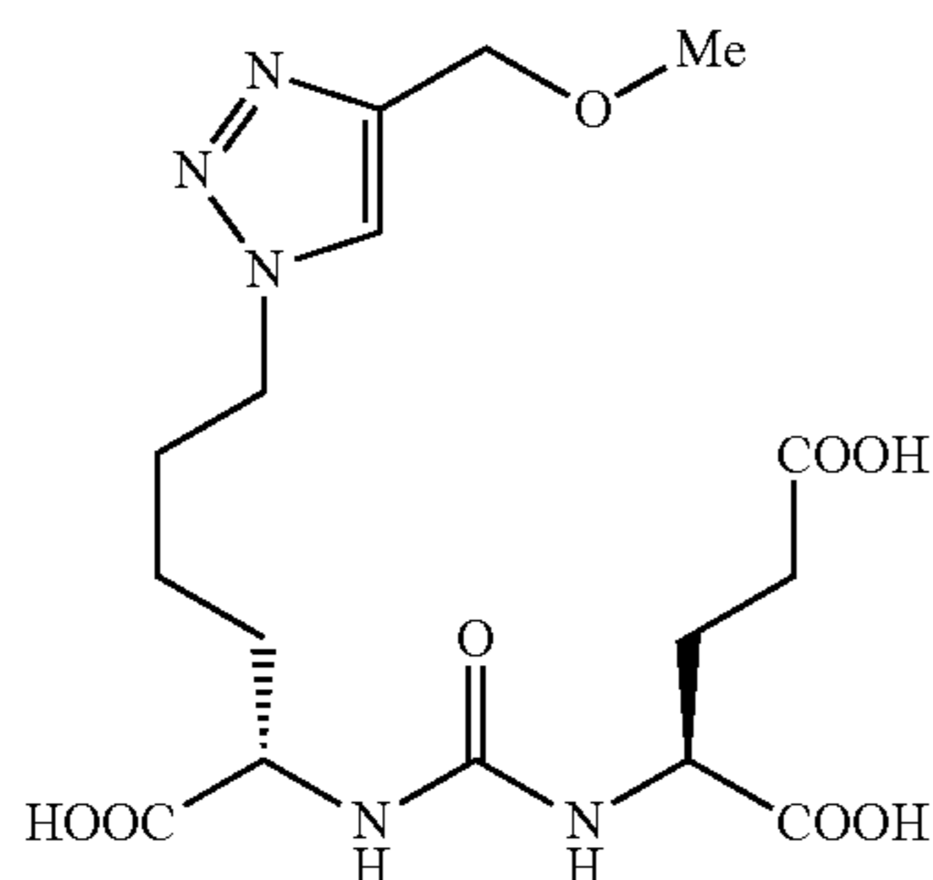
(S)-2-(3-((S)-1-carboxy-5-(4-(methoxymethyl)-1H-1,2,3-triazol-1-yl)pentyl)ureido)pentanedioic acid (8)
