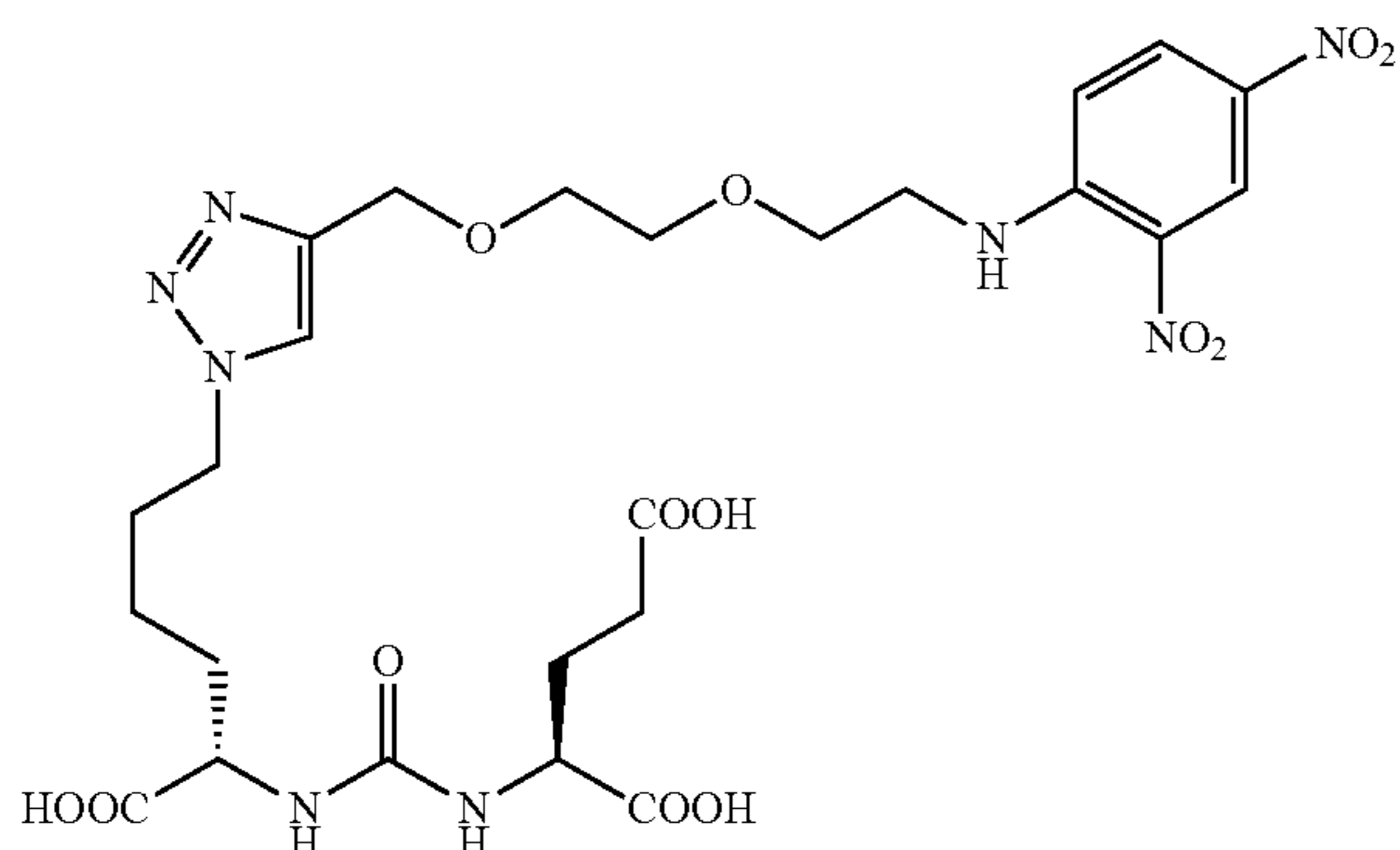
(S)-2-(3-((S)-1-carboxy-5-(4-((2-(2-(2,4-dinitrophenylamino)ethoxy)ethoxy)methyl)-1H-1,2,3-triazol-1-yl)pentyl)ureido)pentanedioic acid (3)
