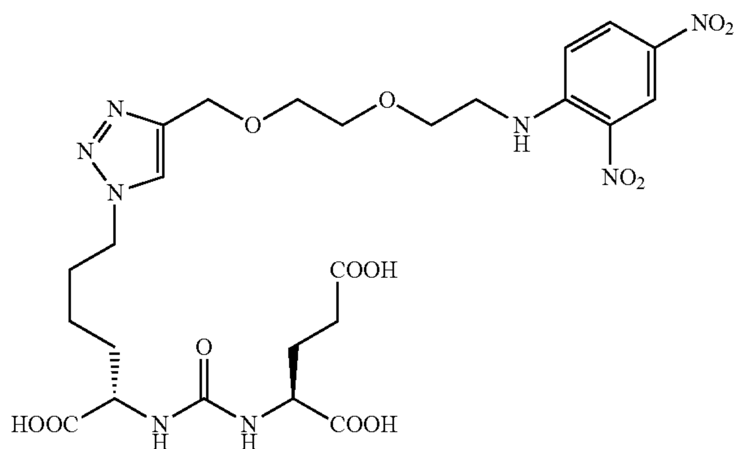
(S)-2-(3-((S)-1-carboxy-5-(4-((2-(2-(2,4-dinitrophenylamino)ethoxy)ethoxy)methyl)-1H-1,2,3-triazol-1-yl)pentyl)ureido)pentanedioic acid (3)
