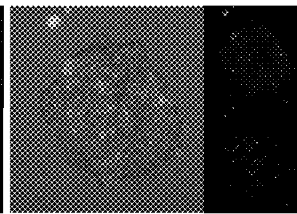
FIG. 16C: Oleandrin [10 ug/ml]
