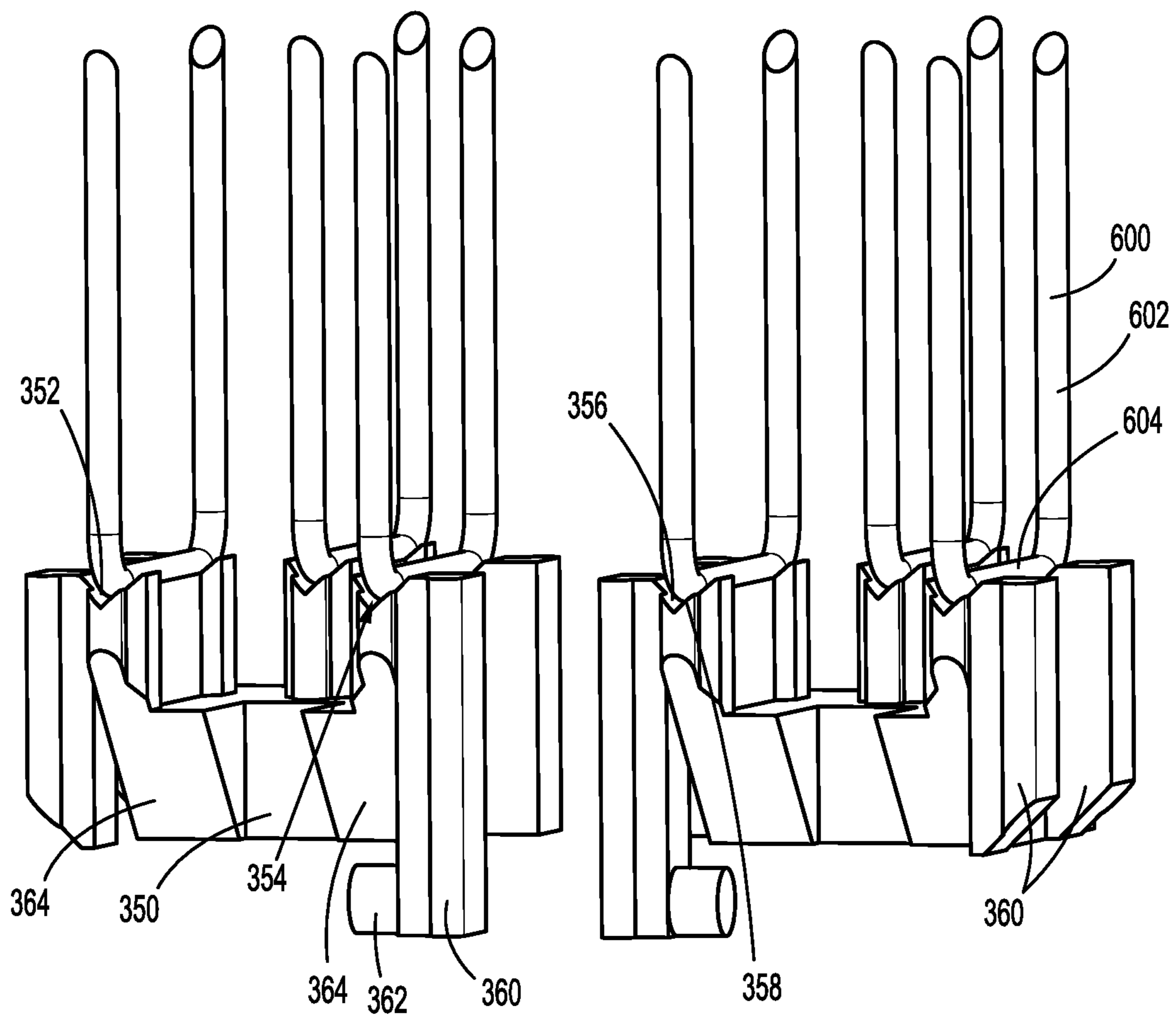
FIG. 5G
