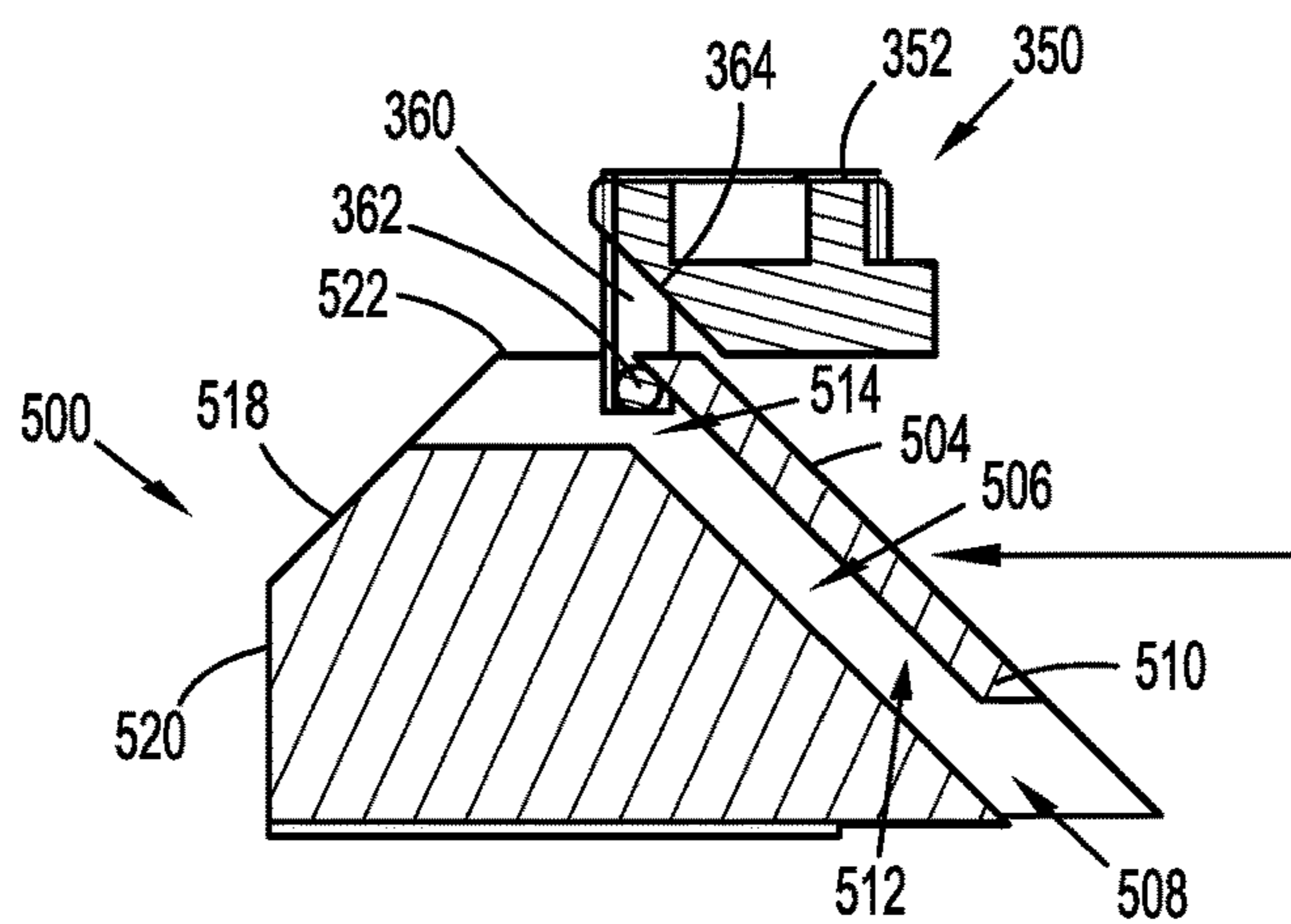
FIG. 15
