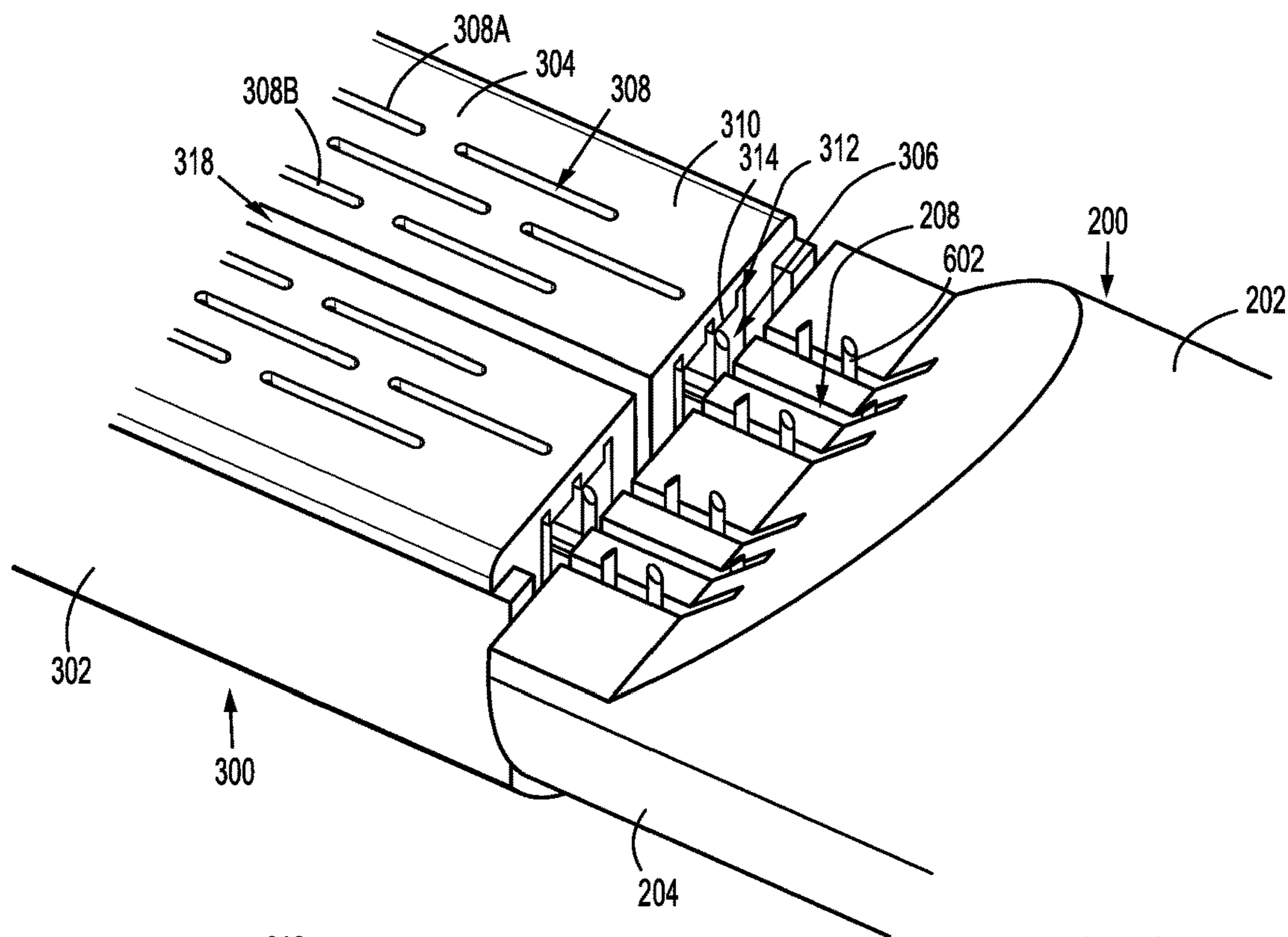
FIG. 3B
