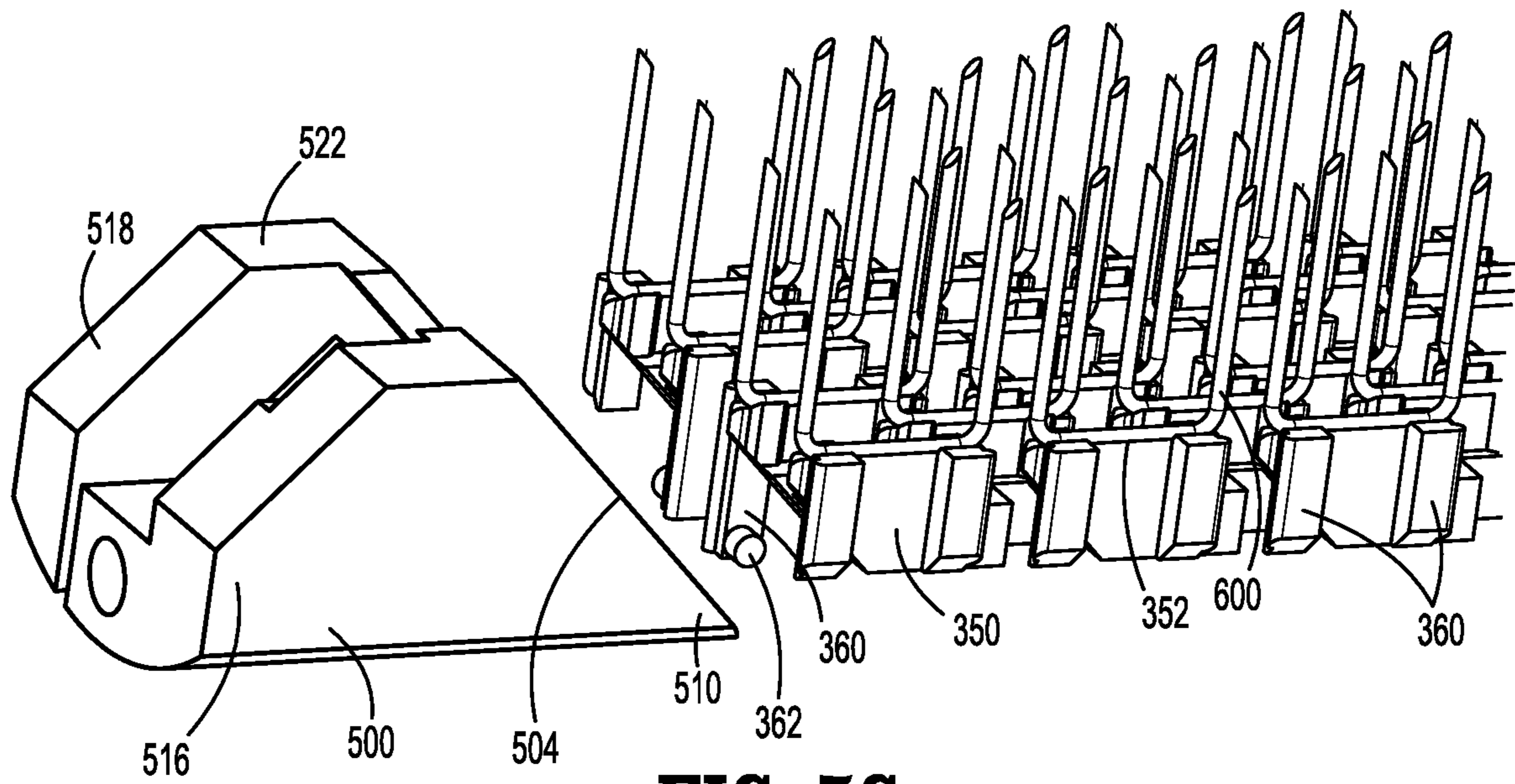
FIG. 5C
