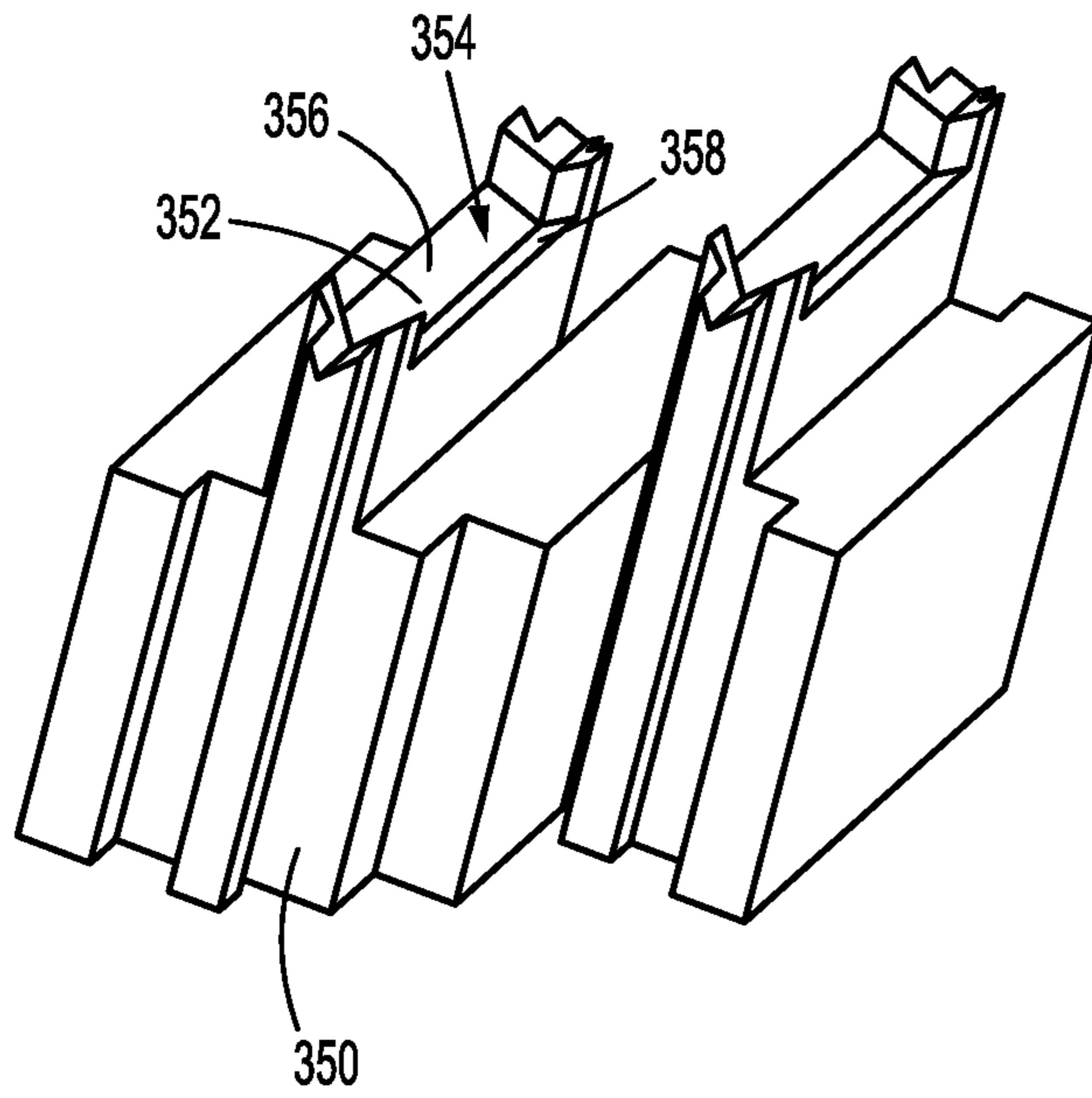
FIG. 6A
