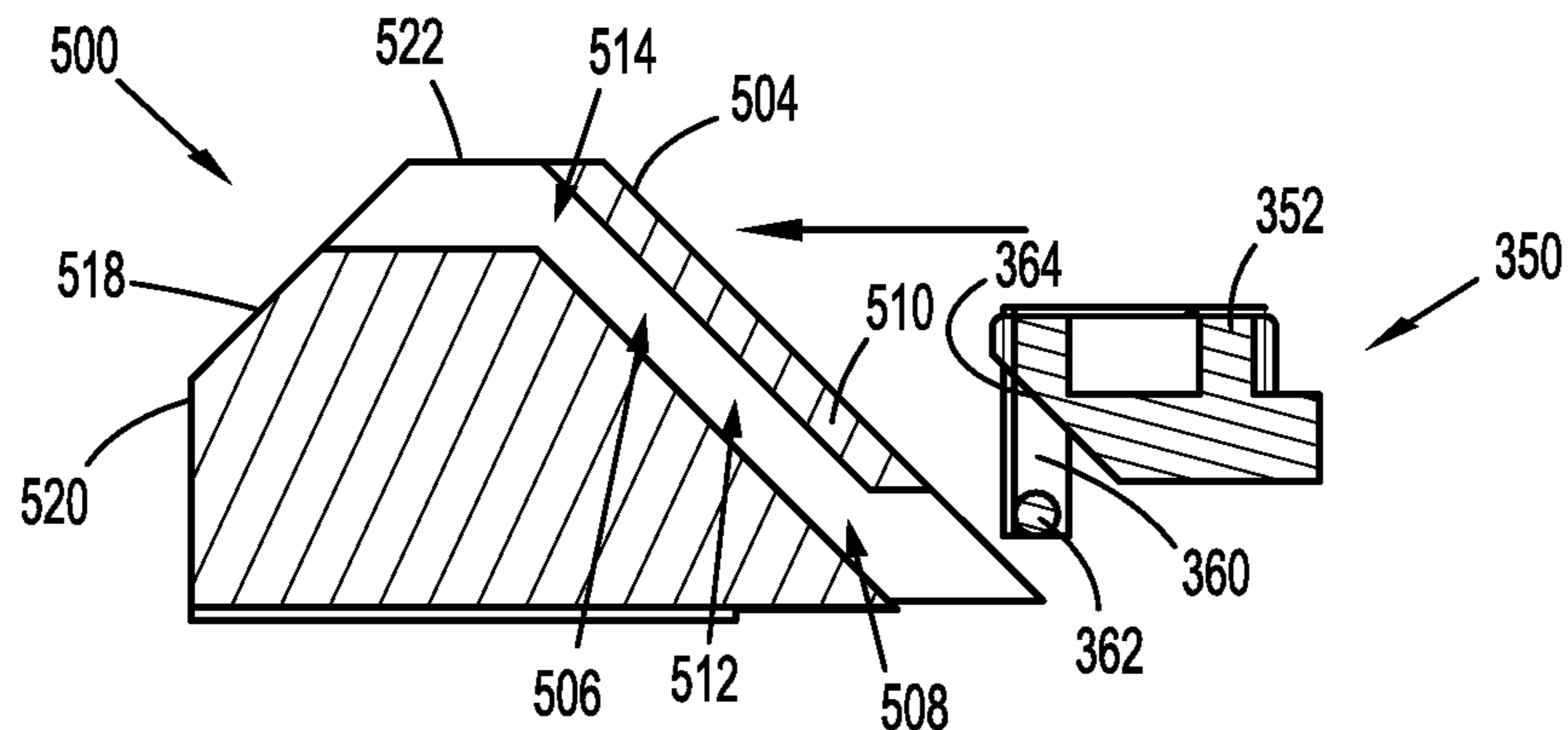
FIG. 18
