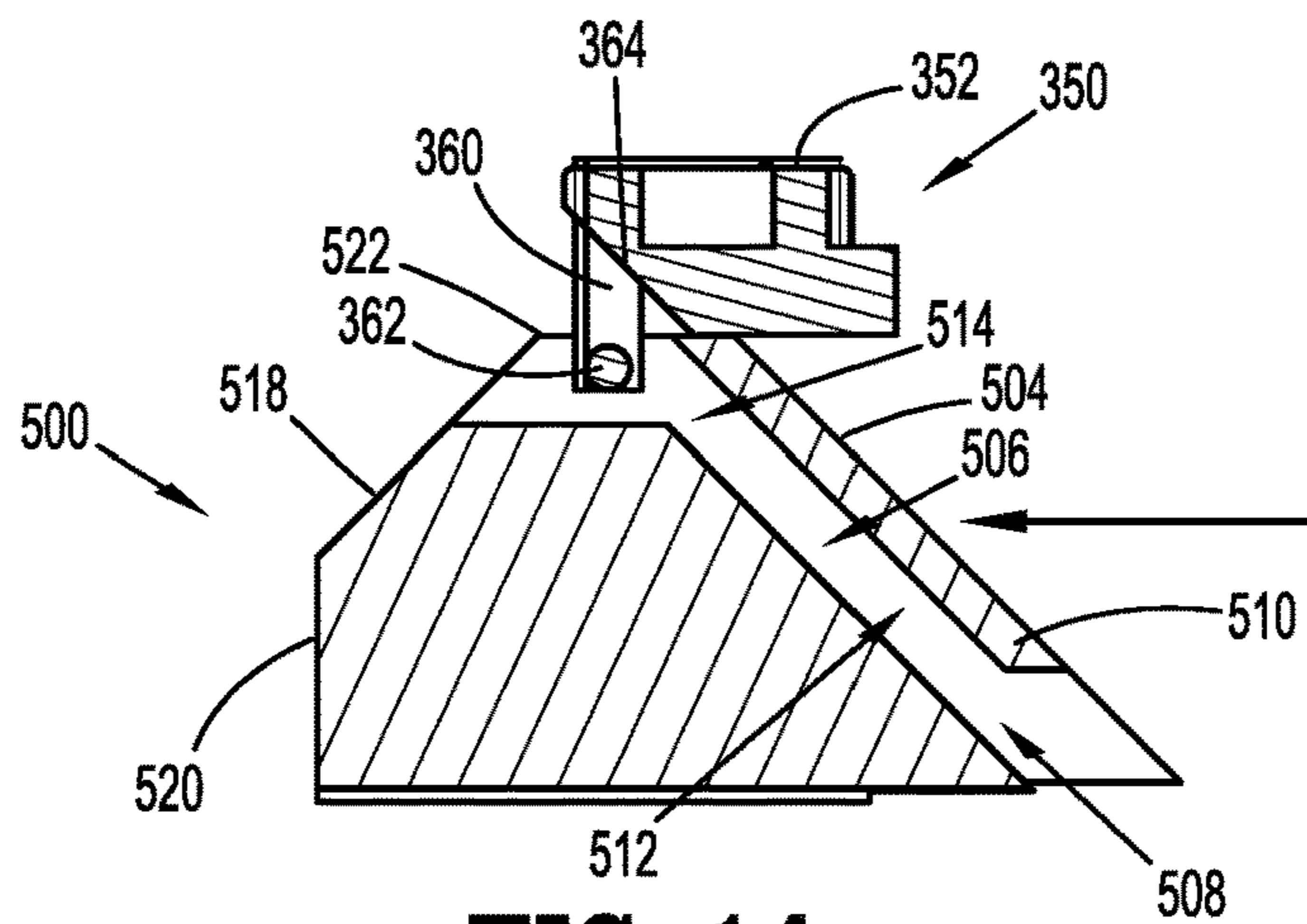
FIG. 14
