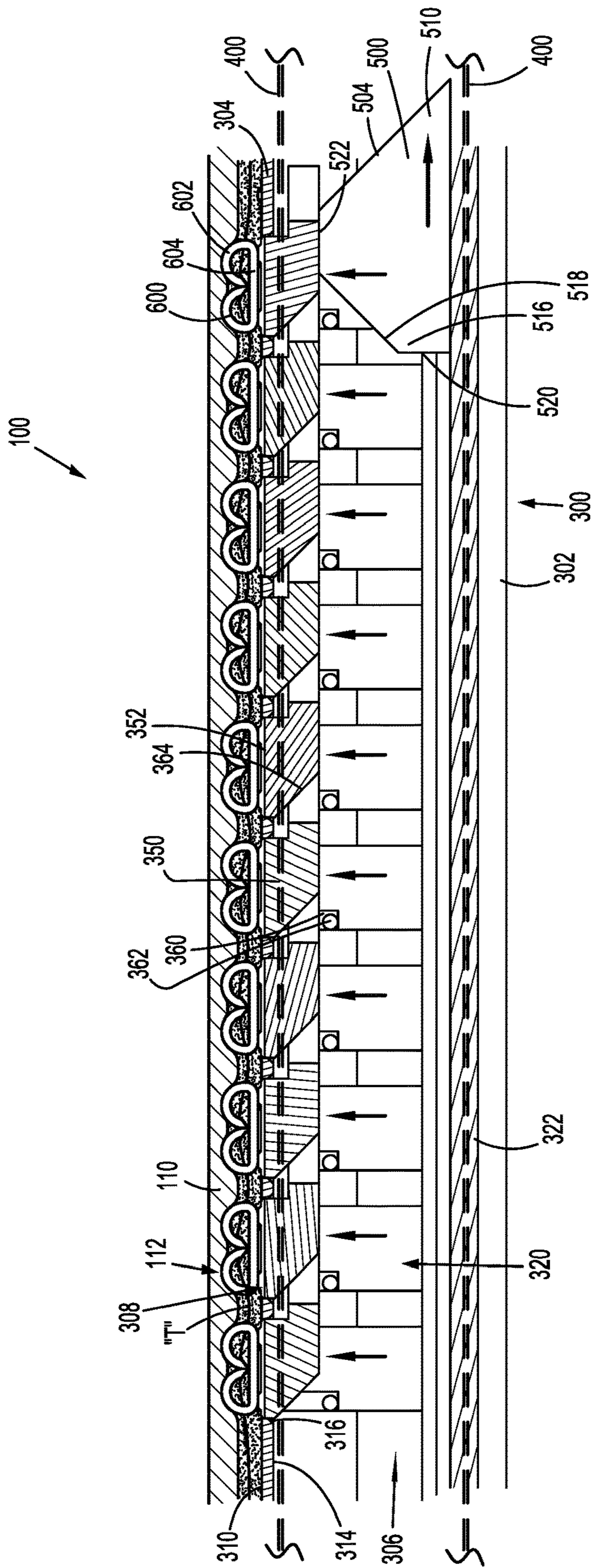
FIG. 19
