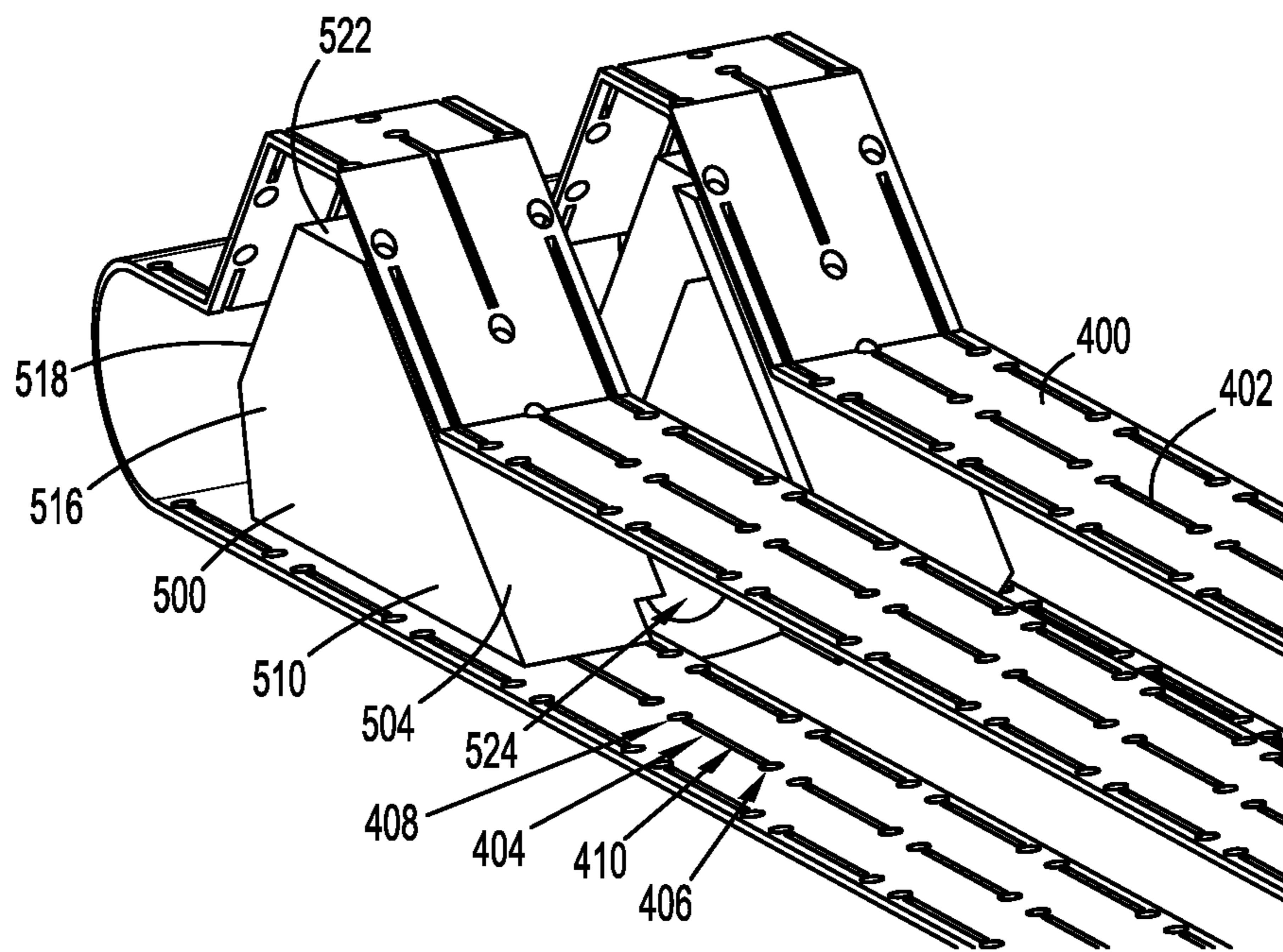
FIG. 5D
