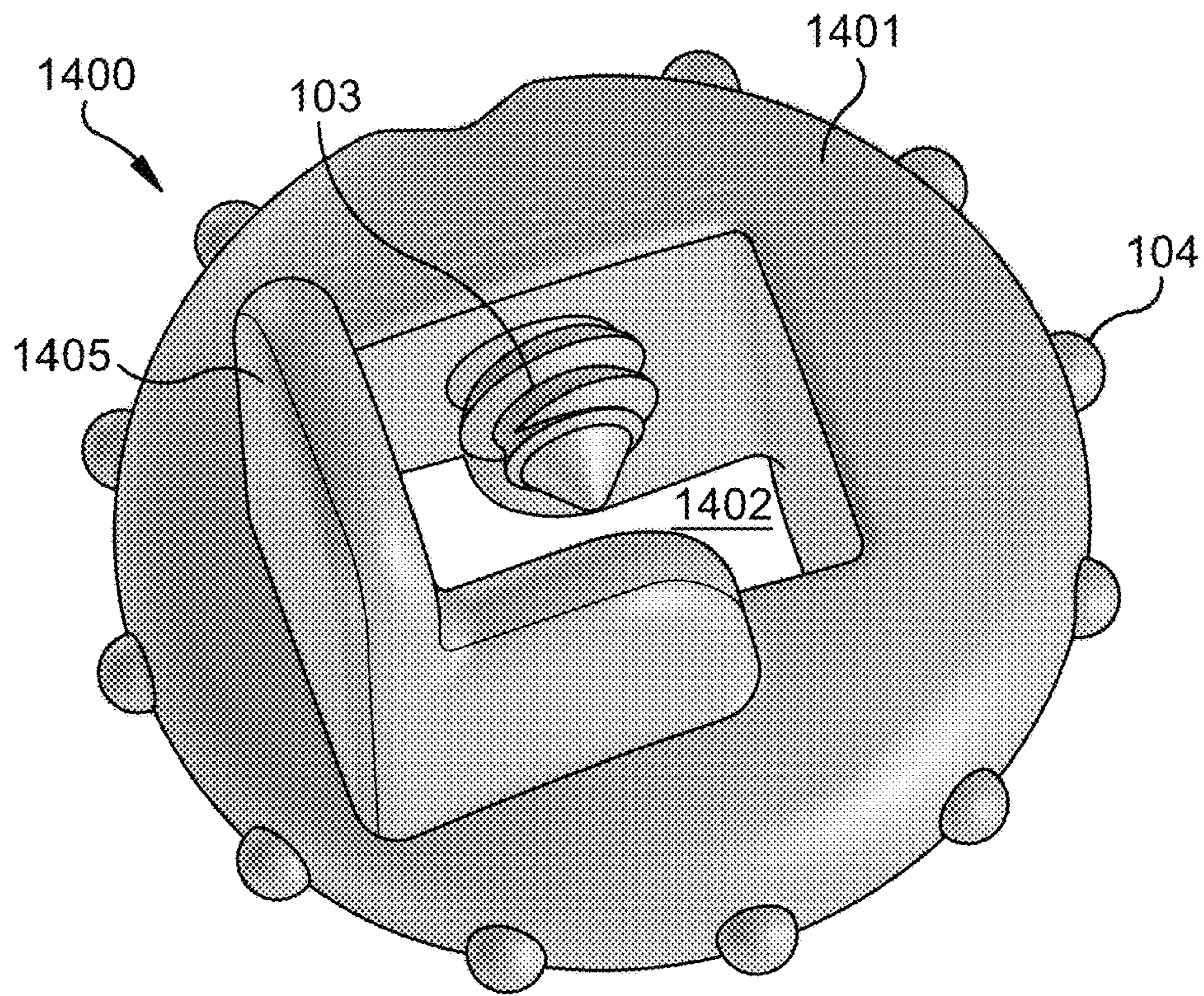
FIG. 14
