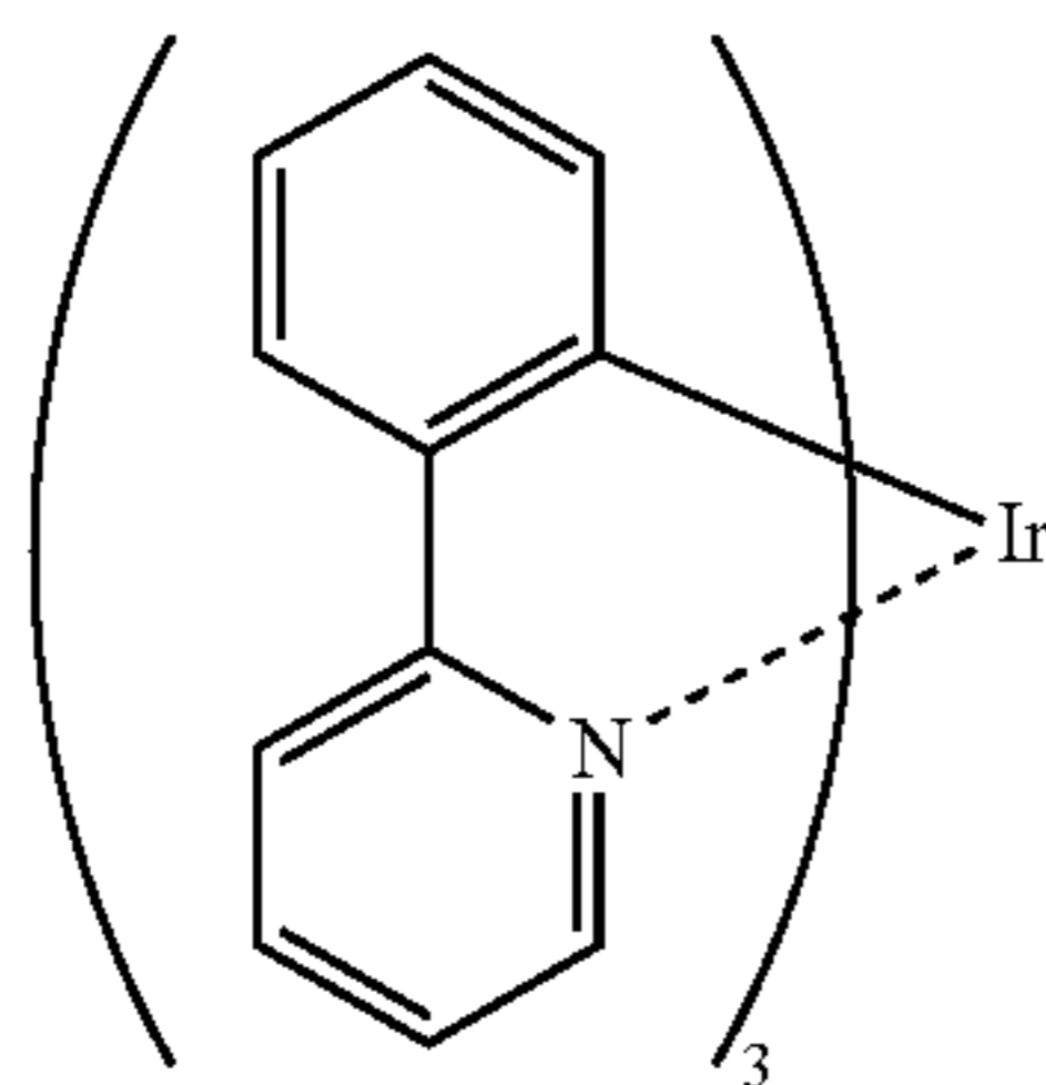
Ir(ppy) 3
