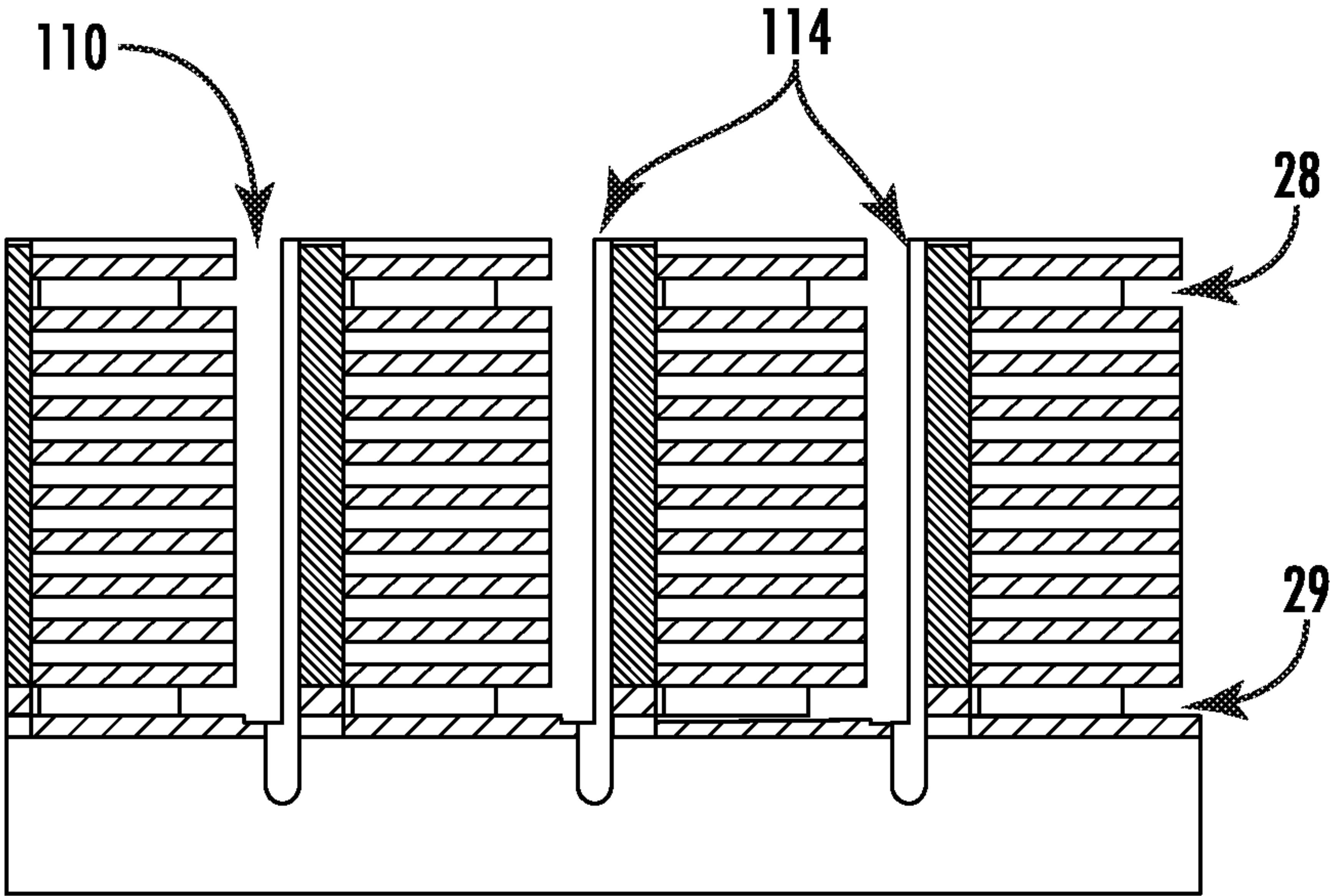
FIG. 11B
