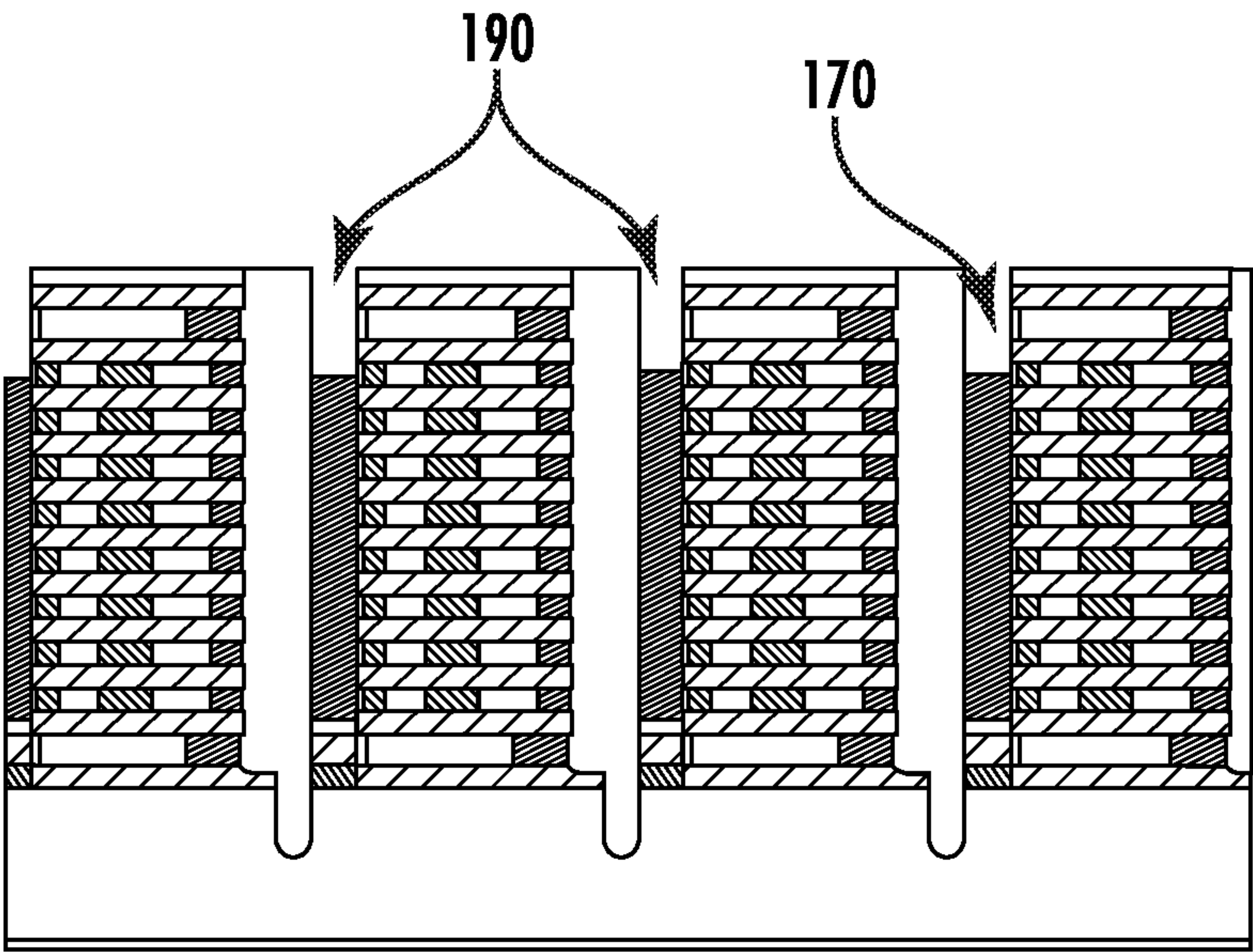
FIG. 19B
