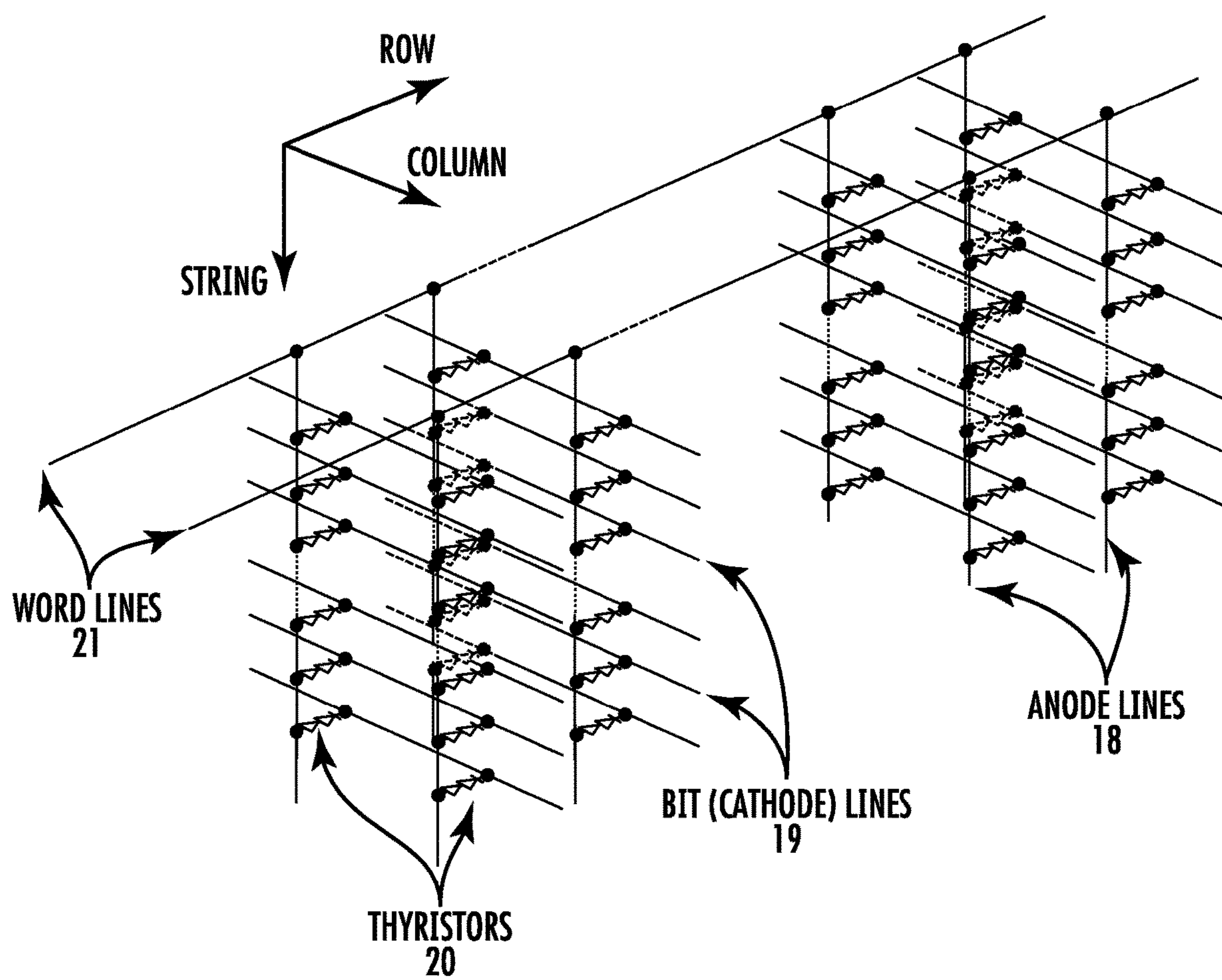
FIG. 3A
