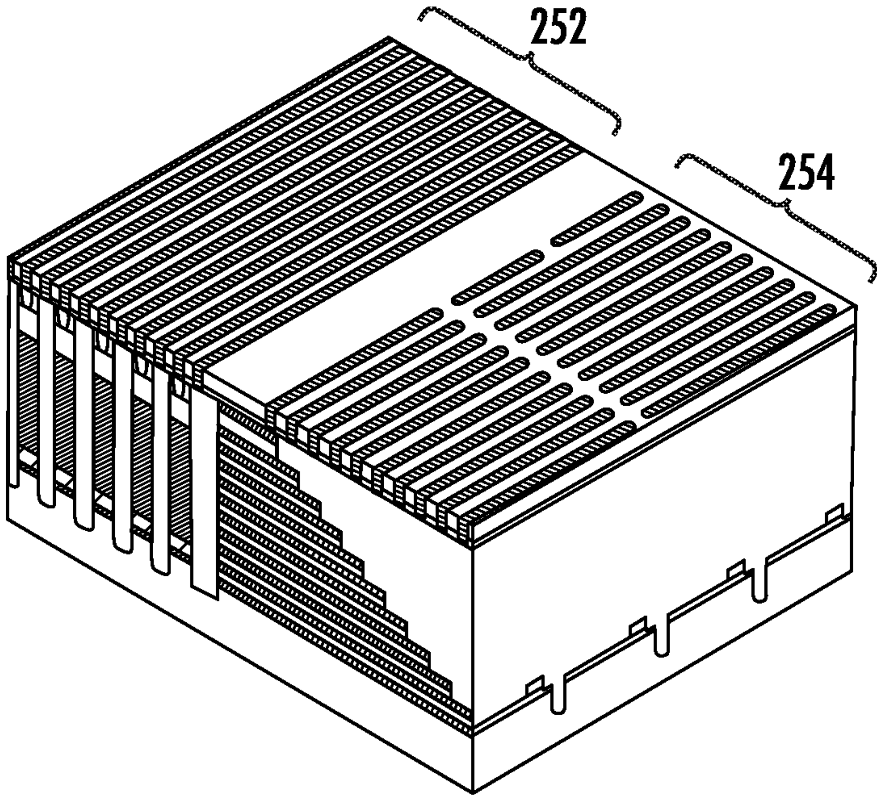
FIG. 25
