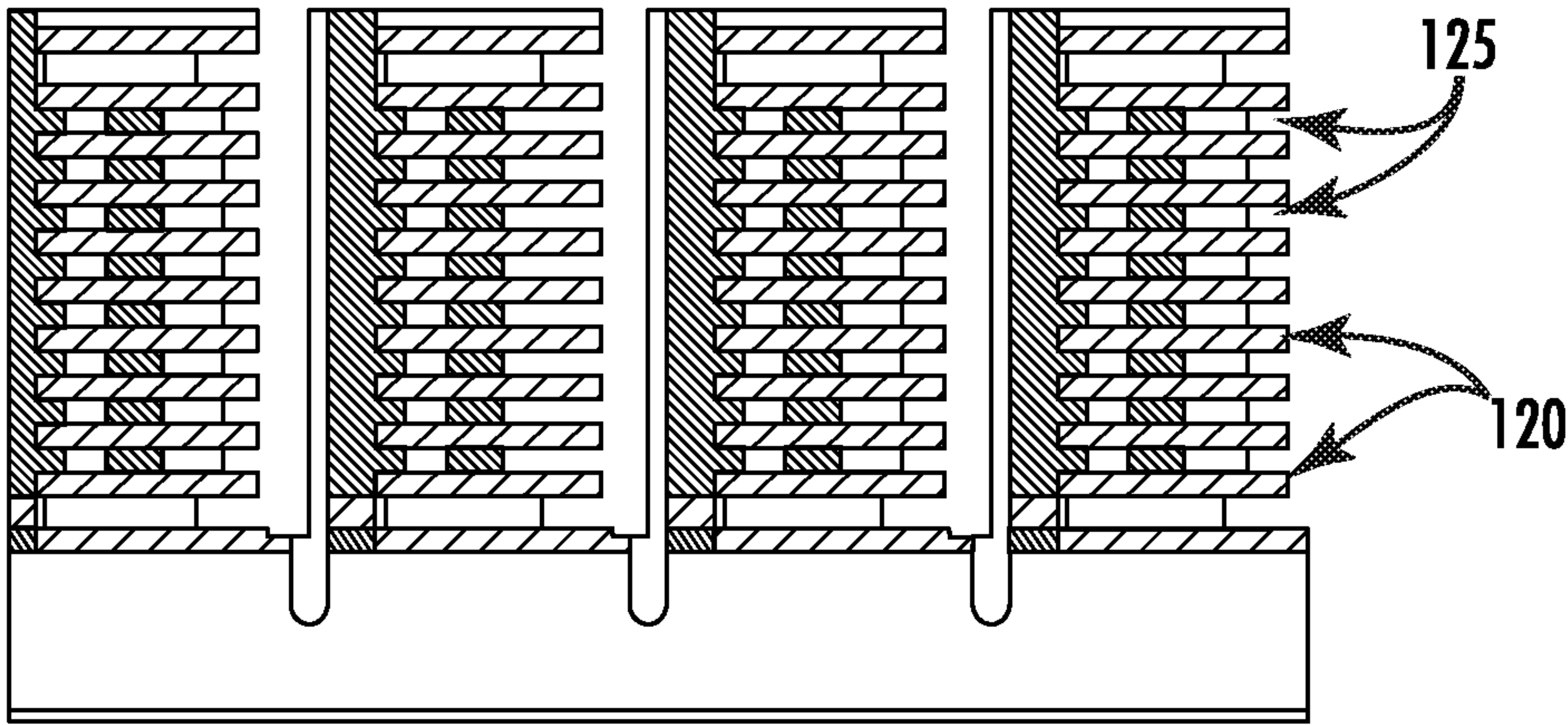
FIG. 13B
