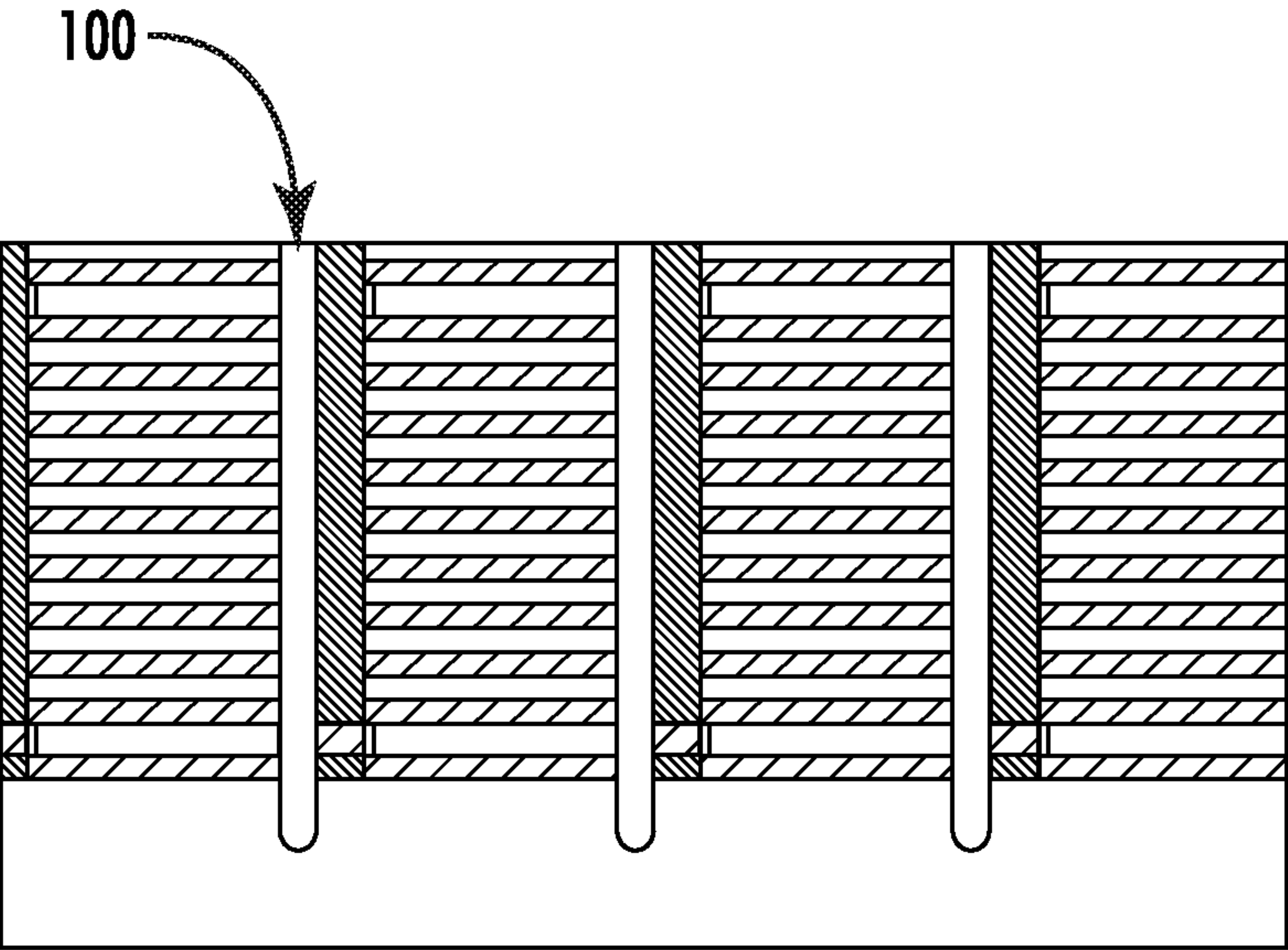
FIG. 10B
