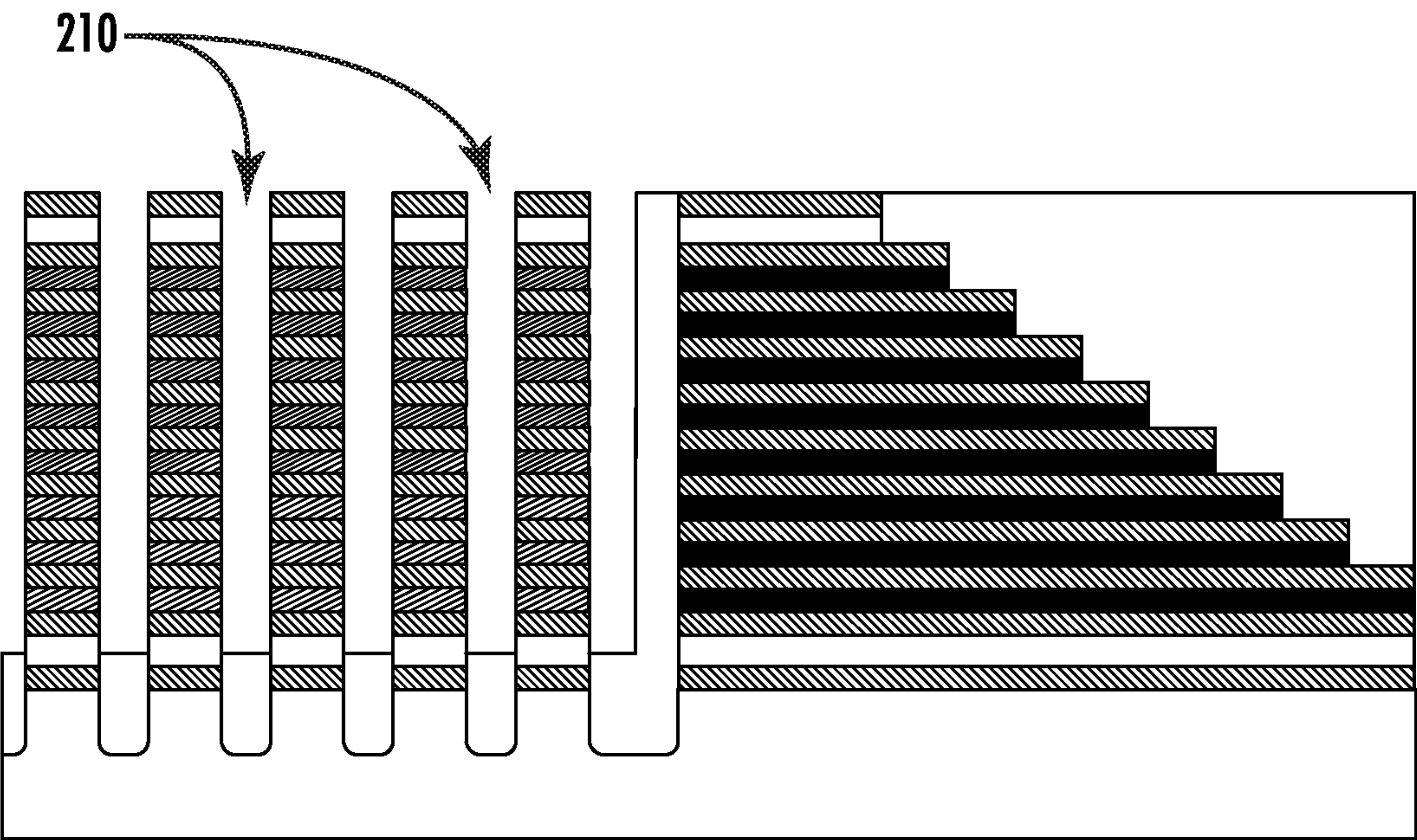
FIG. 21B
