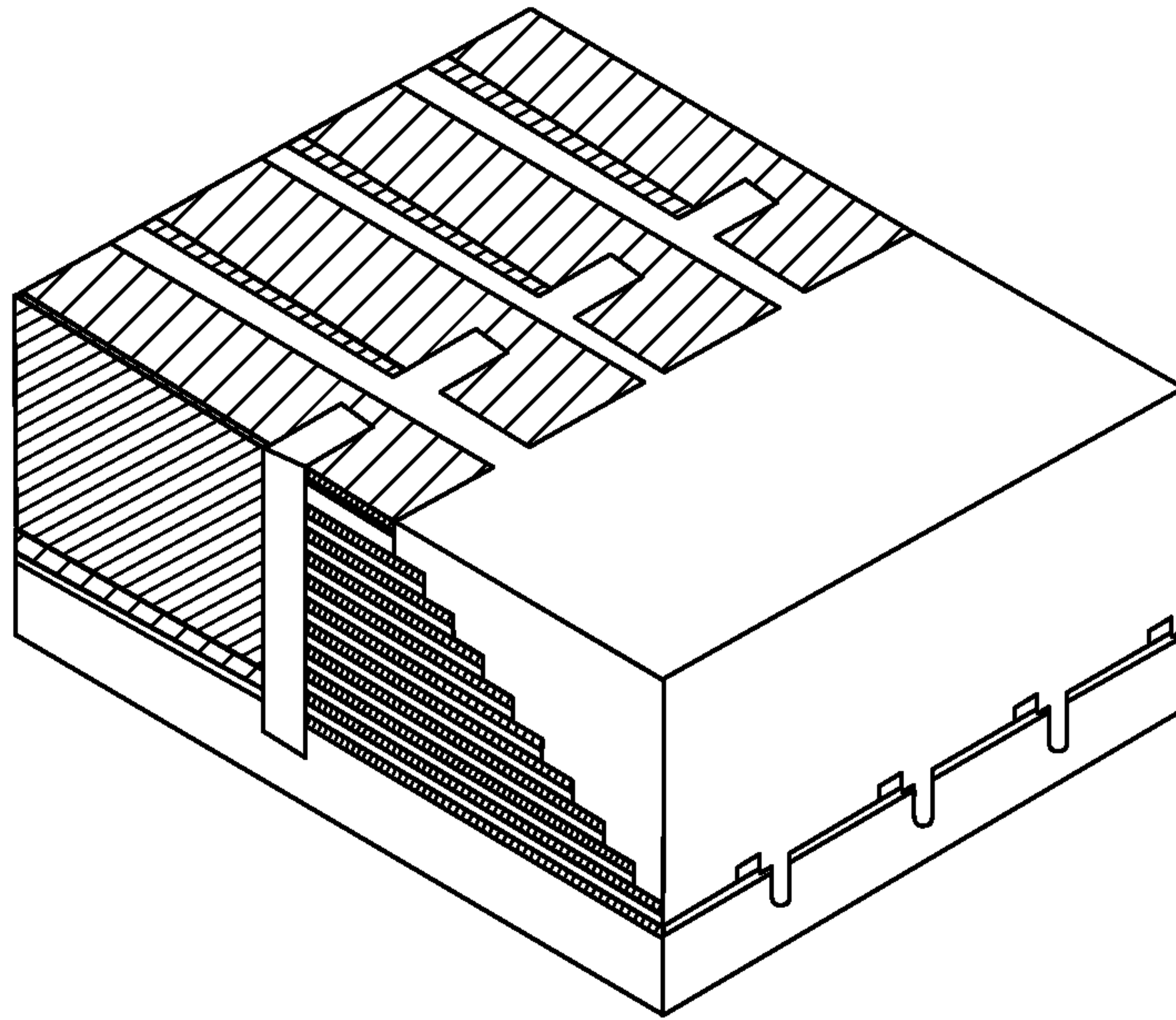
FIG. 15
